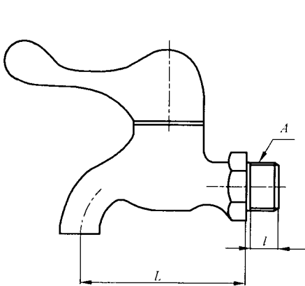
图 A.1 普通洗涤水嘴
