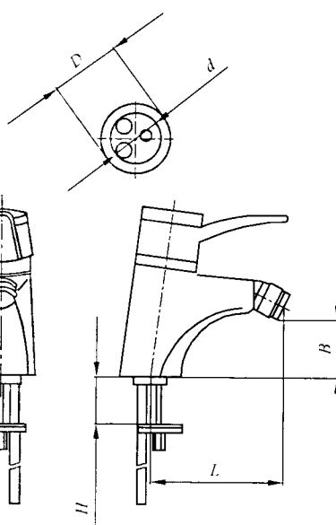
图 A.17 台式明装单柄双控净身水嘴
