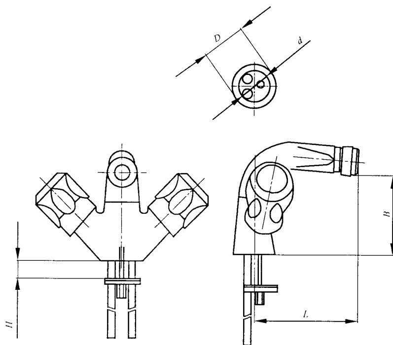
图 A.16 台式明装双柄双控净身水嘴
