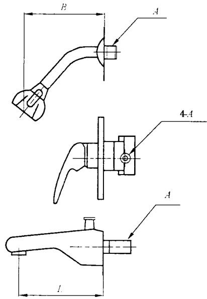
图 A.9 壁式暗装单柄双控浴缸/淋浴水嘴
