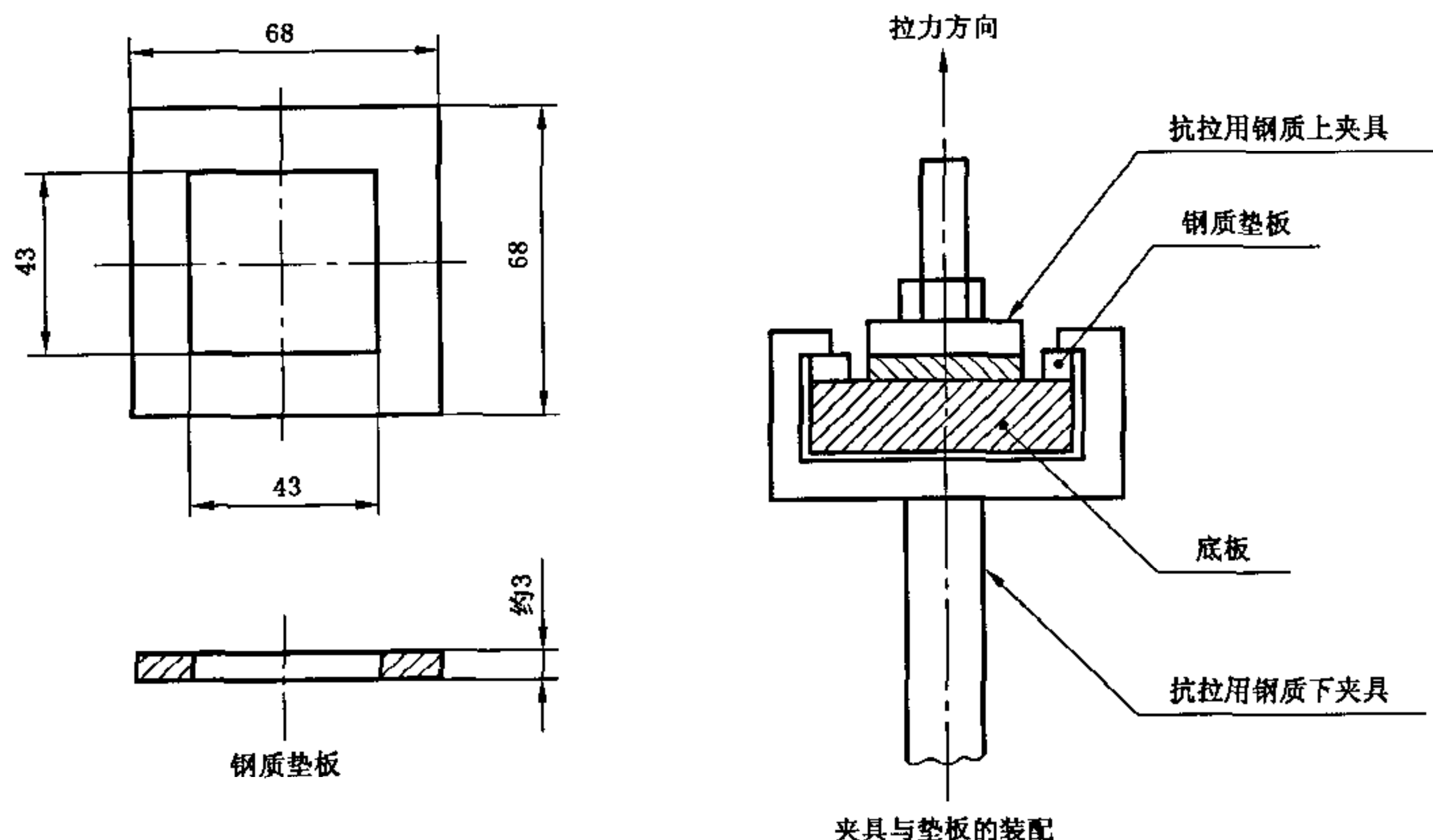
图 5 钢质下夹具和钢质垫板的装配
