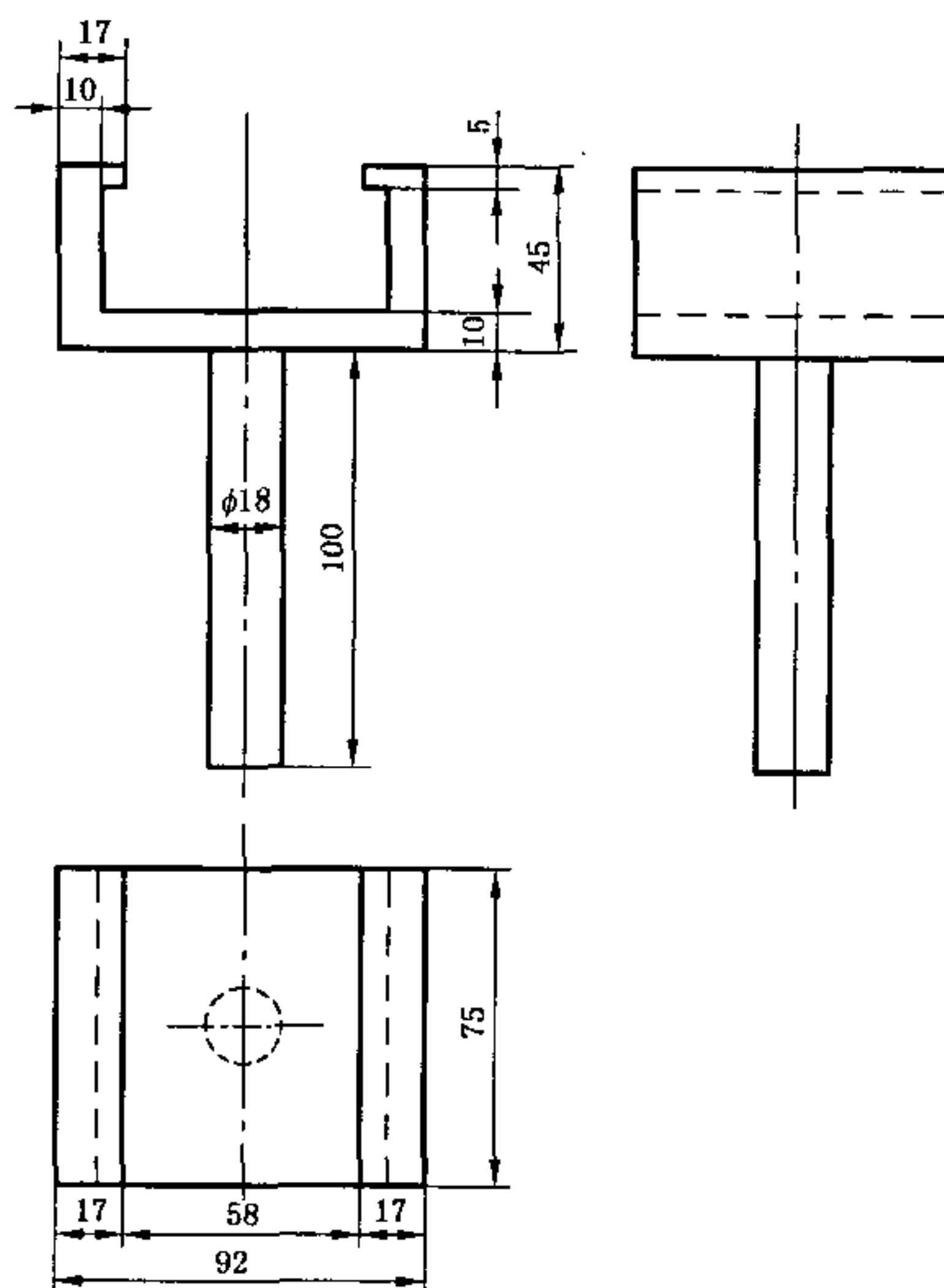
图 4 抗拉用钢质下夹具
