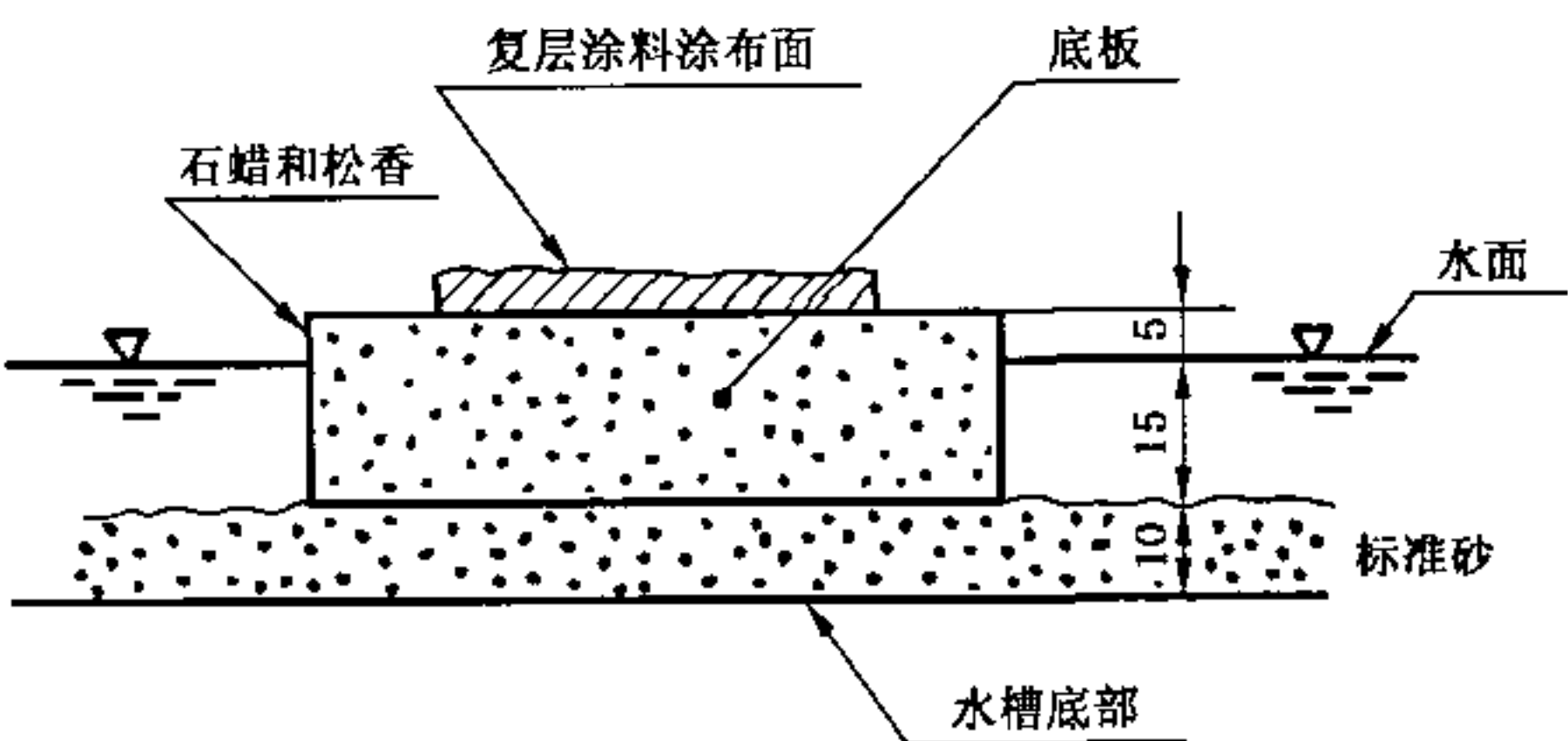
图 6 浸水后粘结强度试验用装置
