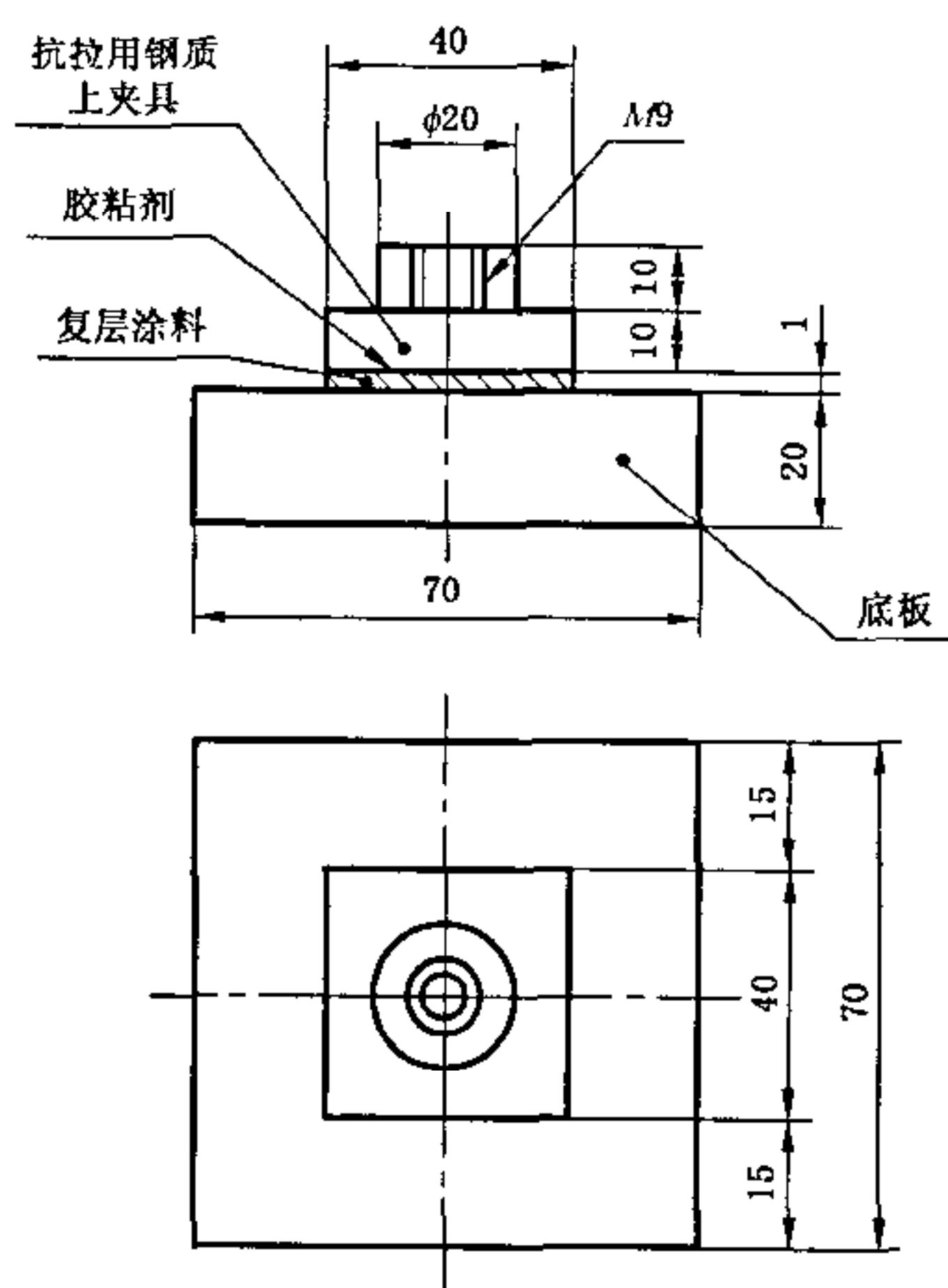
图 3 抗拉用钢质上夹具
