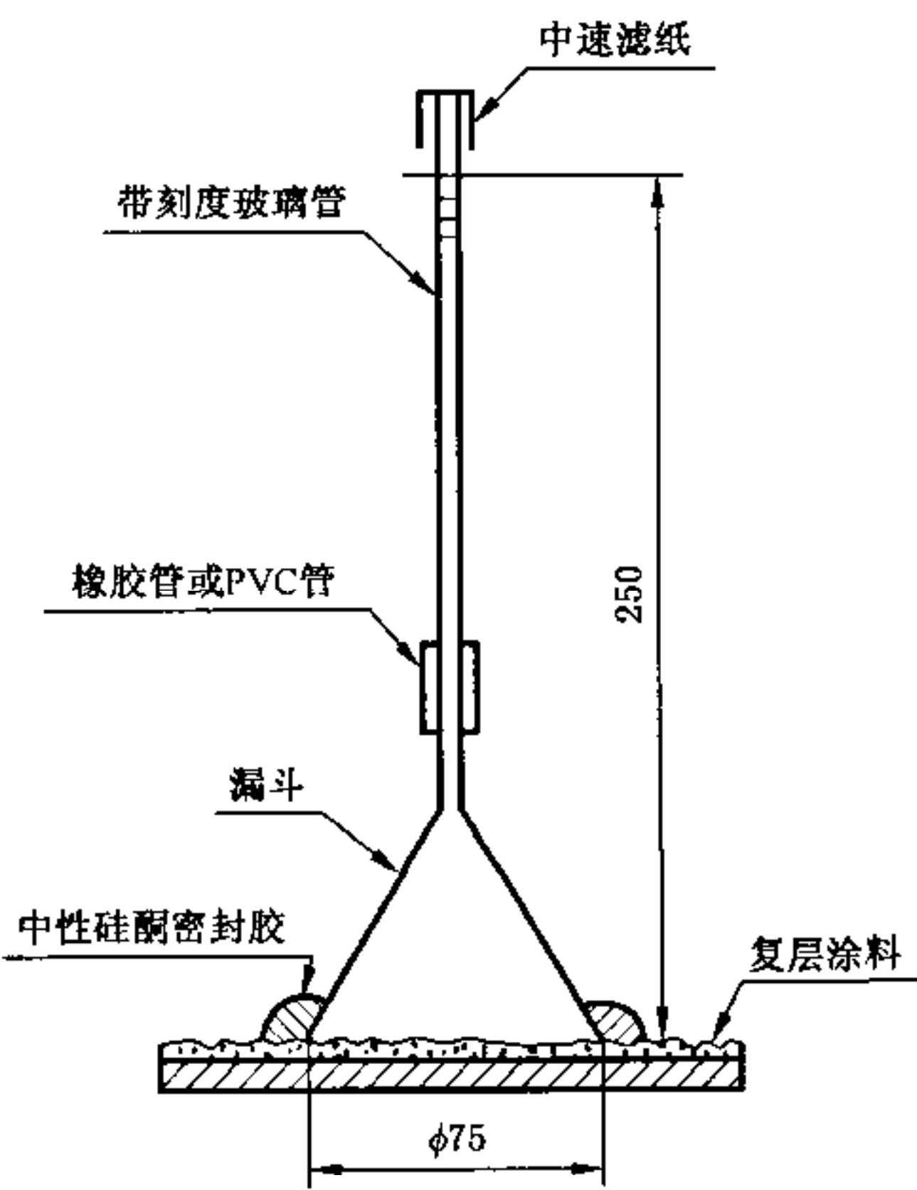
图 7 透水性试验用装置
