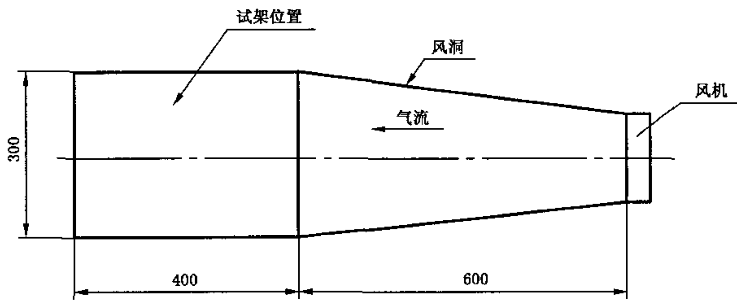
图 1 初期干燥抗裂性试验用仪器
