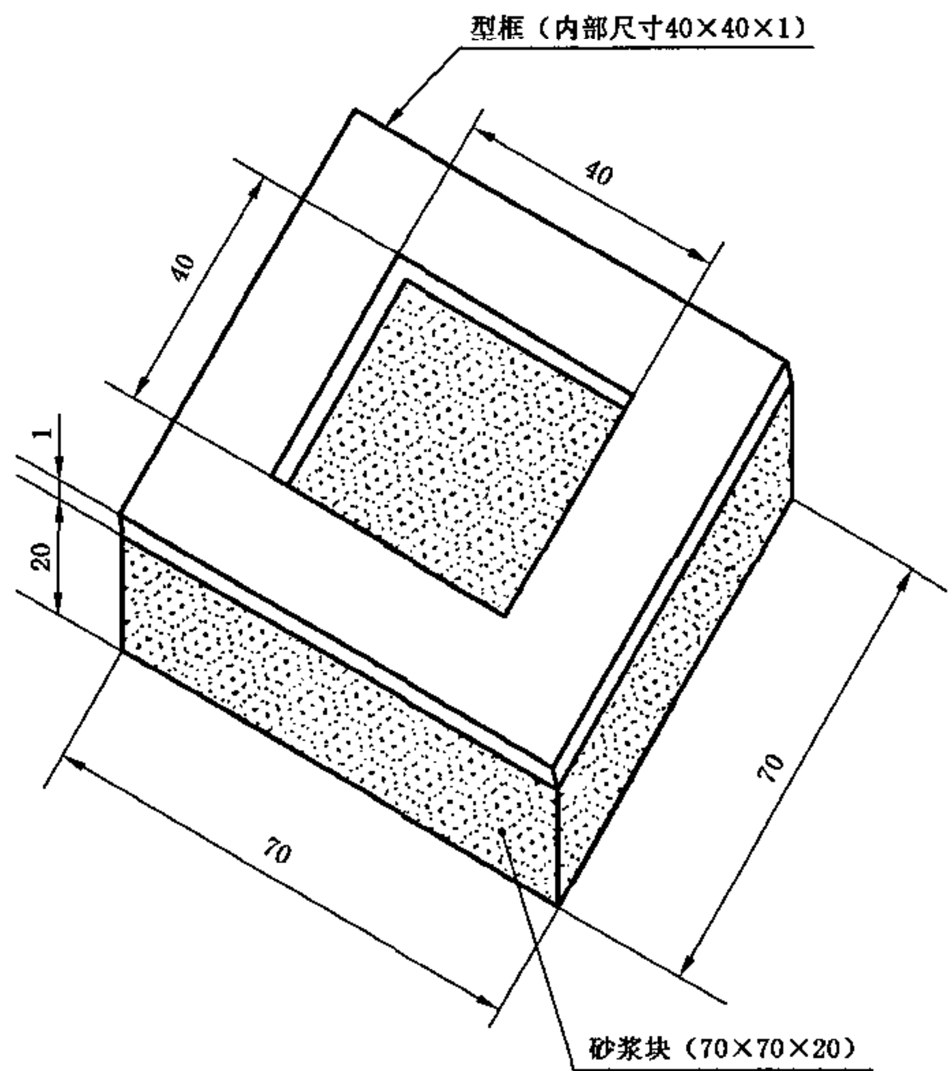
图 2 硬聚氯乙烯或金属型框
