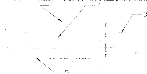
1—砂壁状建筑涂料; 2—砂浆块; 3—水面; 4—标准砂; 5—水槽底部
