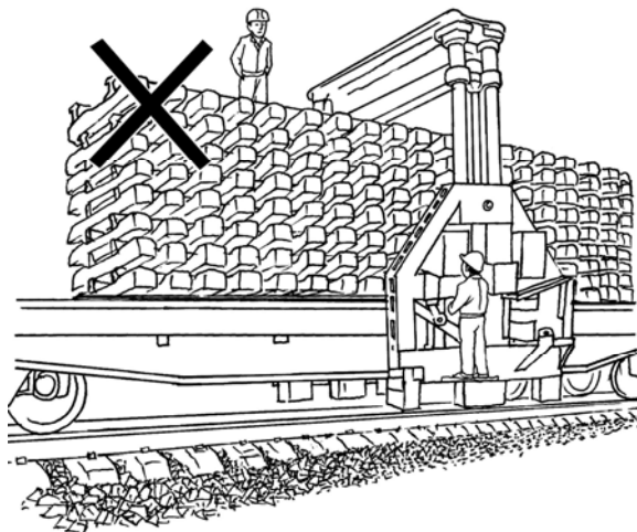
图 7.3.4 换装时人员不应站在轨节上
