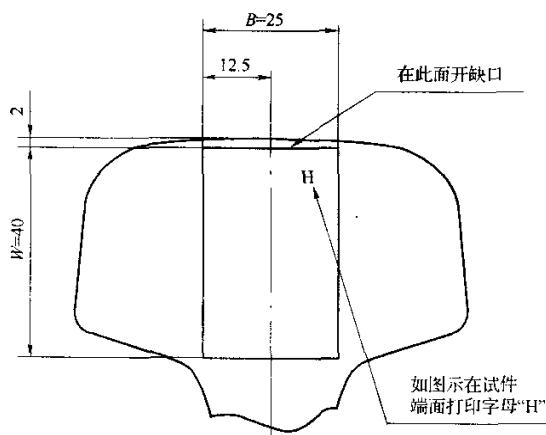
图 D.1 断裂韧性试样的取样部位
