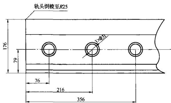
b) 60 kg/m钢轨螺栓孔布置图
