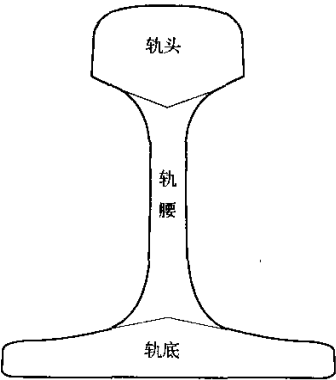
图 C. 1 钢轨横断面分区定义
