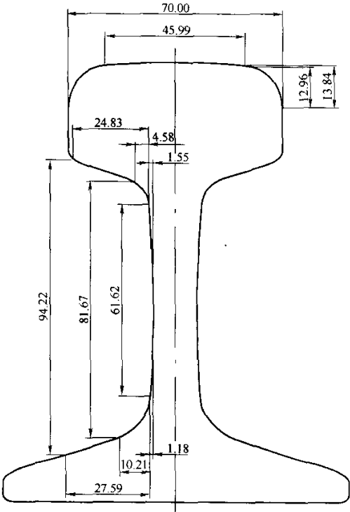
图 A.2 43 kg/m 钢轨断面过渡尺寸
