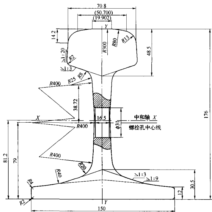
a) 60 kg/m钢轨断面图
