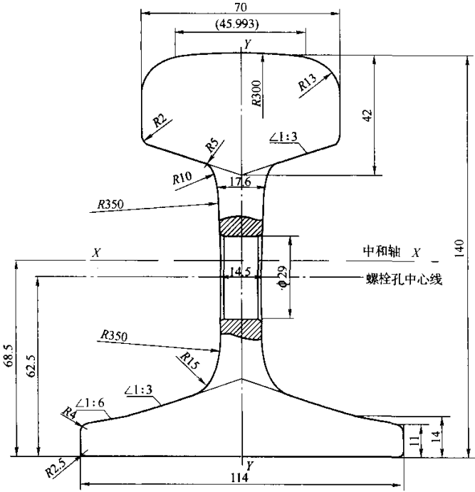
a) 43 kg/m 钢轨断面图
