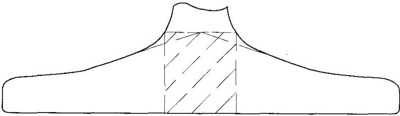
图 8 钢轨轨底超探区域(阴影部分)
