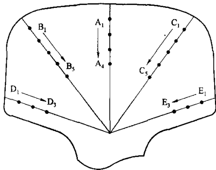
图 3 横断面硬度测点位置示意图
