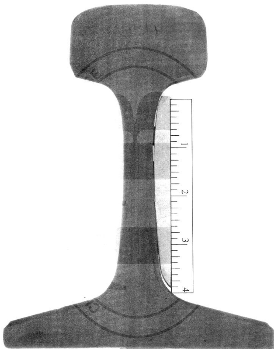
图 C. 11 由放射状条纹、裂纹、中间裂纹以及转折裂纹发展的轨头内大于 3 mm 的条纹
