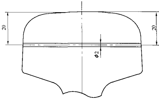
c) 钢轨轨头人工缺陷位置 3
