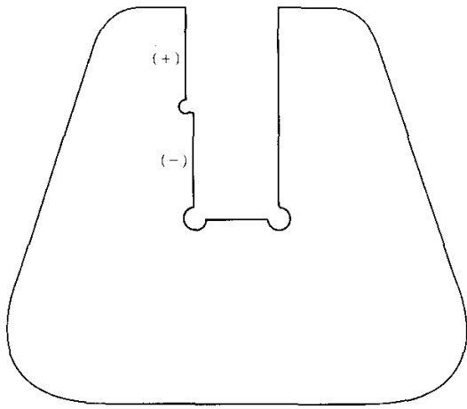
图 B.8 轨腰厚度
