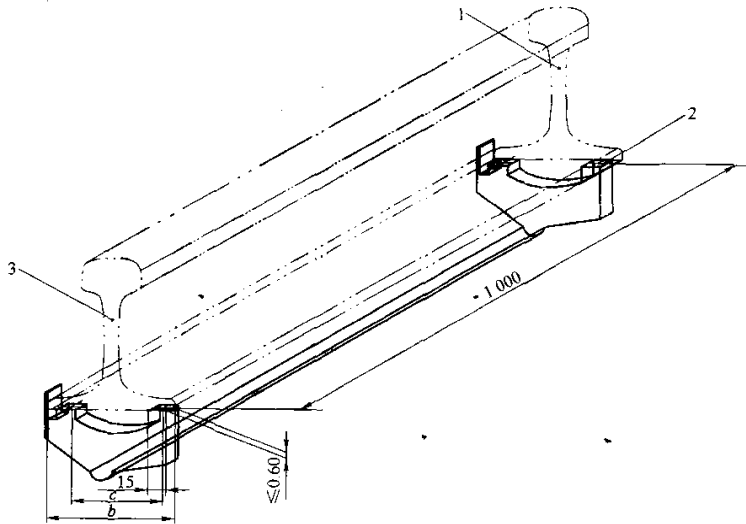
图 1 钢轨平直度测量示意图
