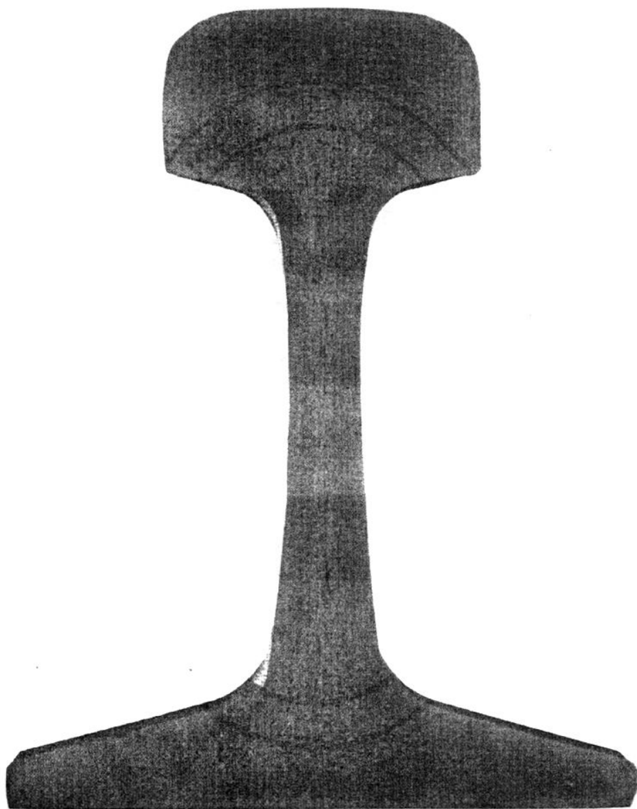
图 C. 8 延伸至轨头或轨底超过 25 mm 的分散分布的偏析
