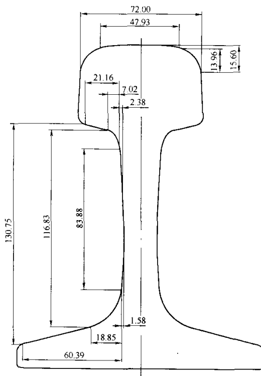
图 A.8 75 kg/m 钢轨断面过渡尺寸
