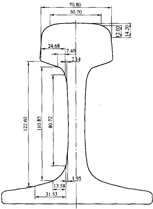
图 A. 6 60 kg/m 钢轨断面过渡尺寸
