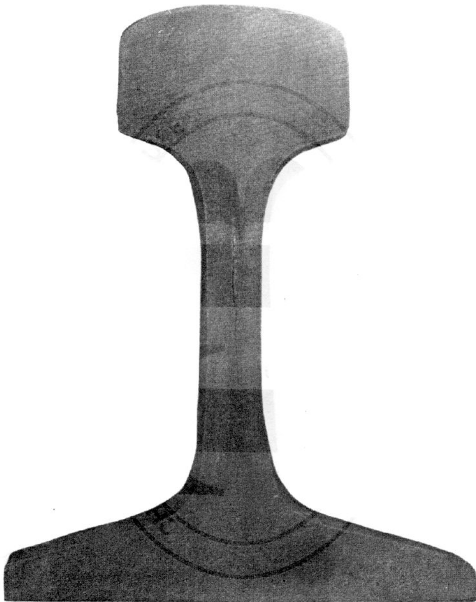
图 C.3 任何尺寸的缩孔
