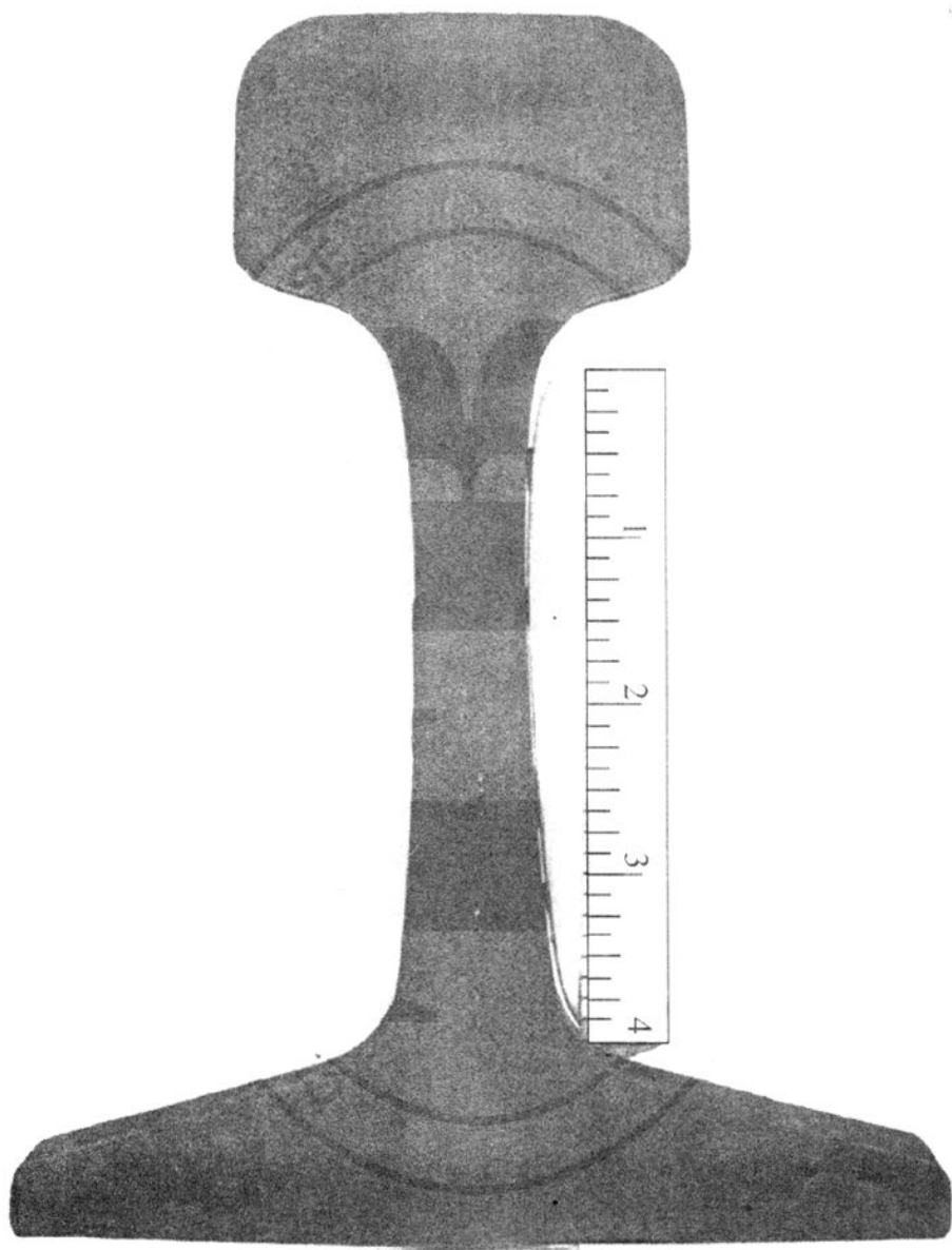
图 C. 12 引起钢轨早期失效的其他缺陷(如炉渣、耐火材料)
