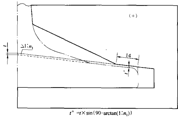
a) 正量规图
