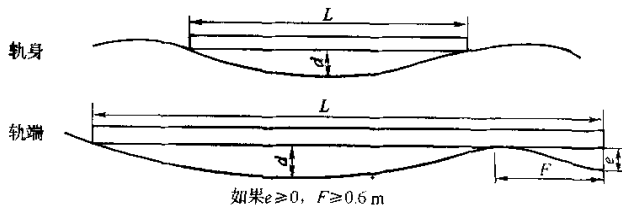
图 1 钢轨平直度测量示意图
