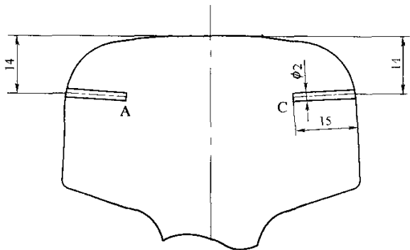
a) 钢轨轨头人工缺陷位置 1
