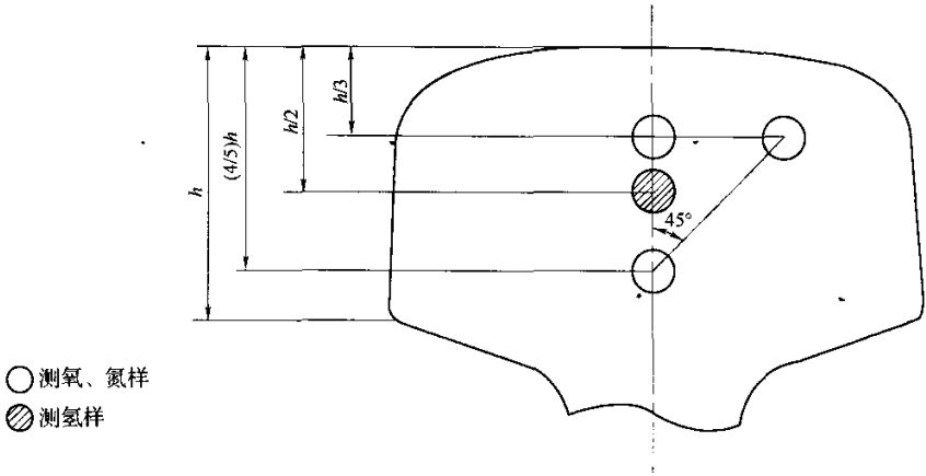
图 6 测定总氧、氮含量和氢含量试样的取样位置
