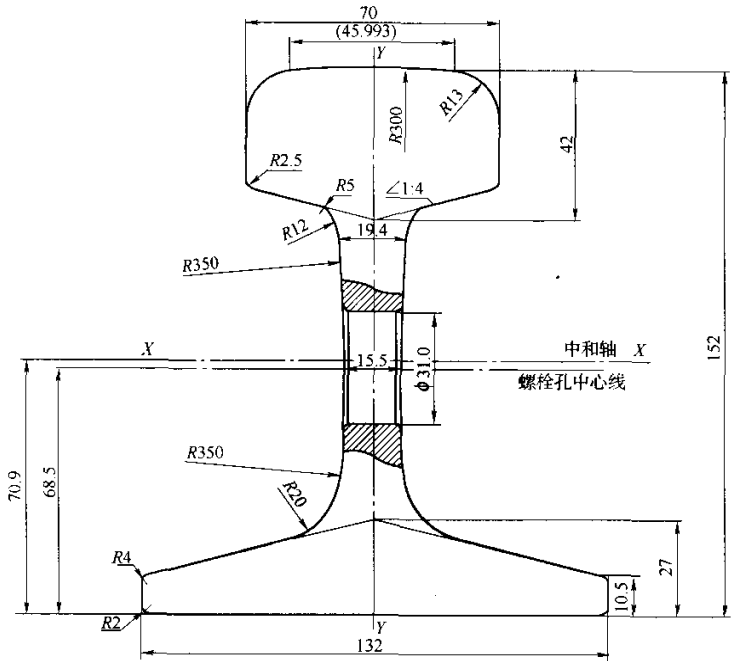
a) 50 kg/m钢轨断面图
