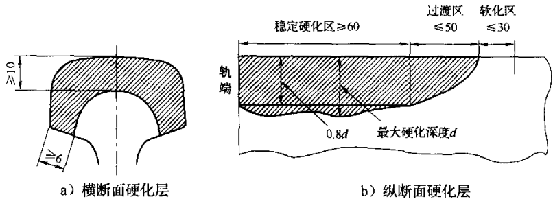
图 E.1 硬化层形状及尺寸
