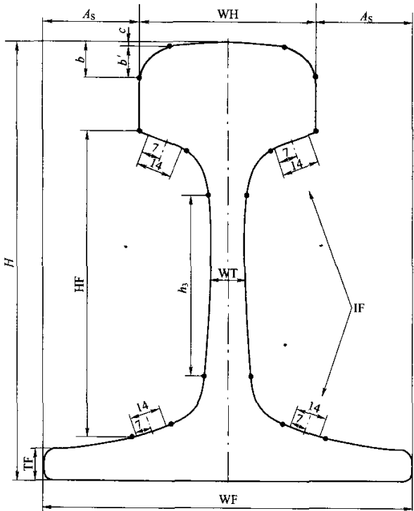
图 B.1 钢轨几何尺寸公差数据基准点
