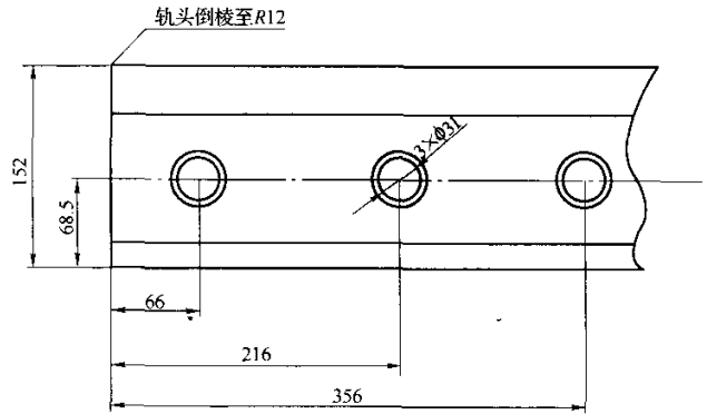
b) 50 kg/m钢轨螺栓孔布置图
