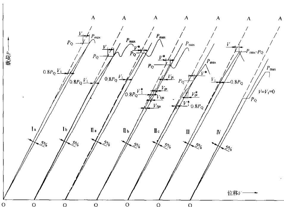
图 D.3 载荷—裂纹张开曲线
