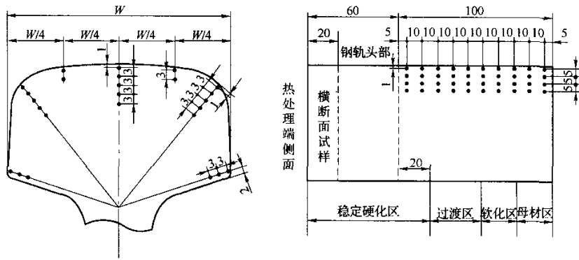
图 E.2 钢轨横断面及纵断面硬化层硬度分布测定位置
