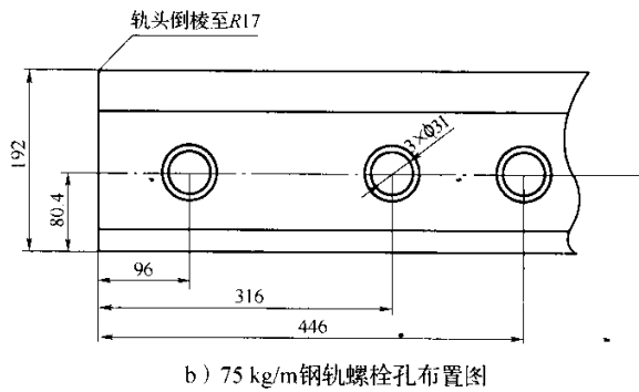
图 A. 7 75 kg/m 钢轨型式尺寸
