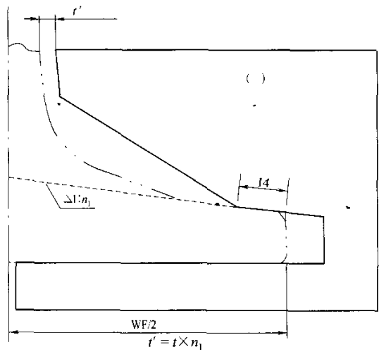
a) 正量规图
