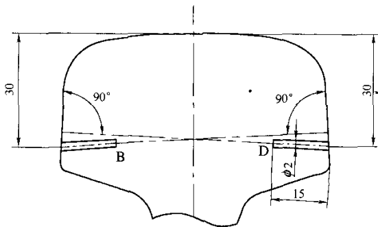
b) 钢轨轨头人工缺陷位置 2
