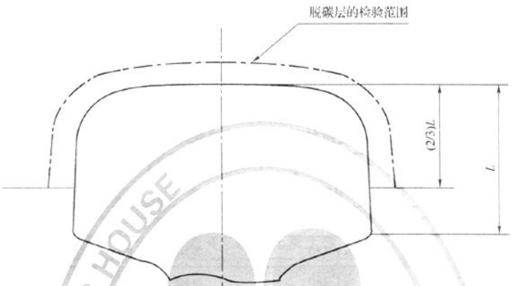
图 4 轨头表面脱碳层检验范围
