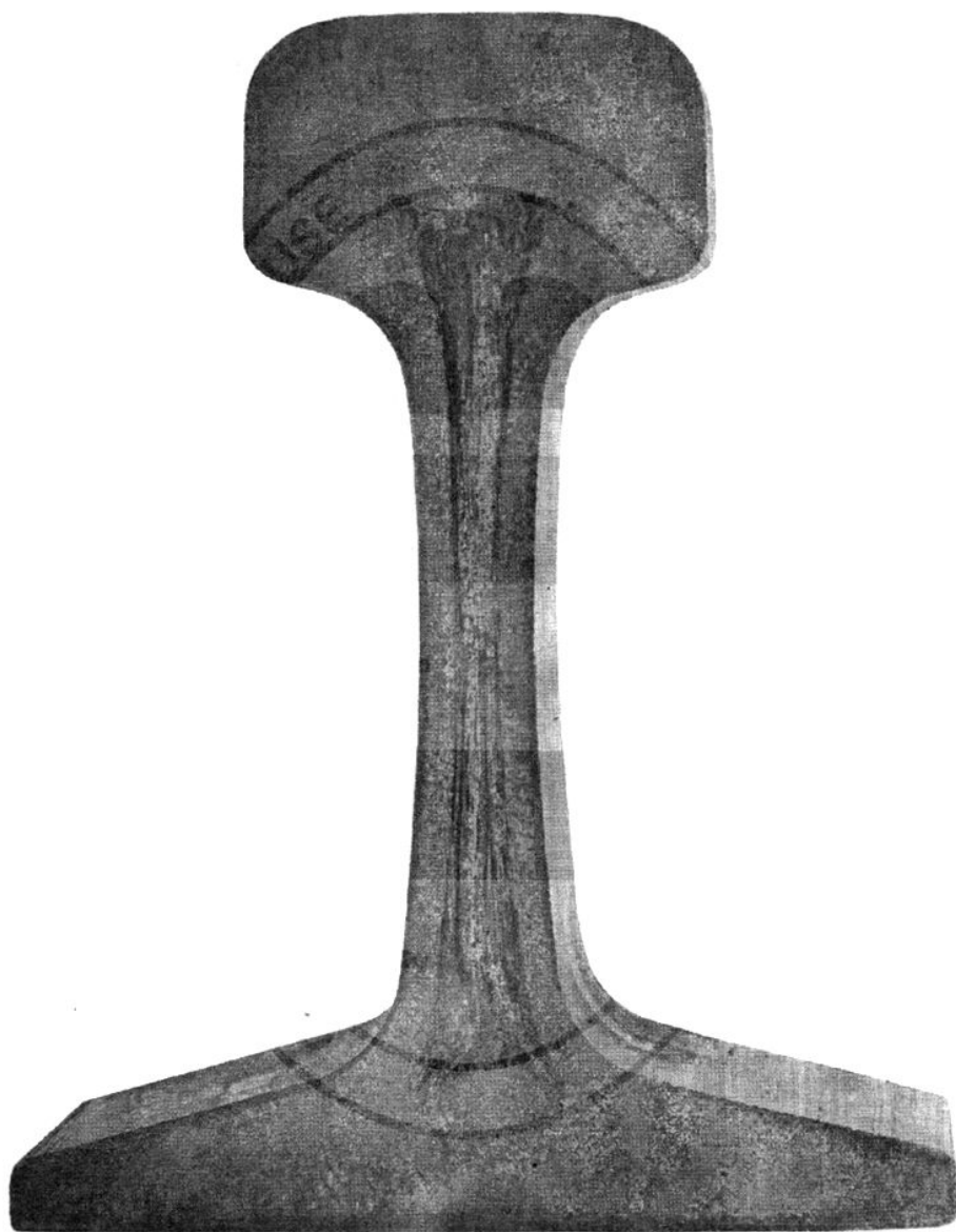
图 C. 10 宽度大于 6 mm 并延伸到轨头或轨底内 13 mm 以上的正偏析或负偏析
