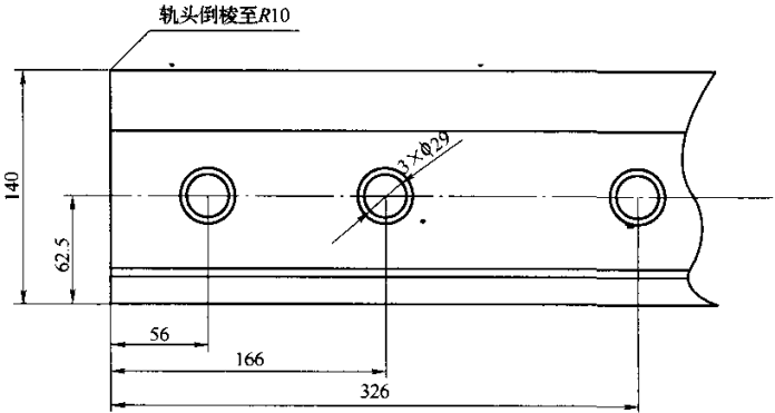
b) 43 kg/m 钢轨螺栓孔布置图
