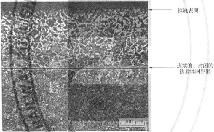
图 5 轨头表面允许的脱碳层深度金相图(100 ×)
