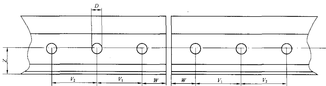
b) 螺栓孔布置示意图
