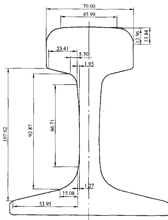
图 A.4 50 kg/m 钢轨断面过渡尺寸
