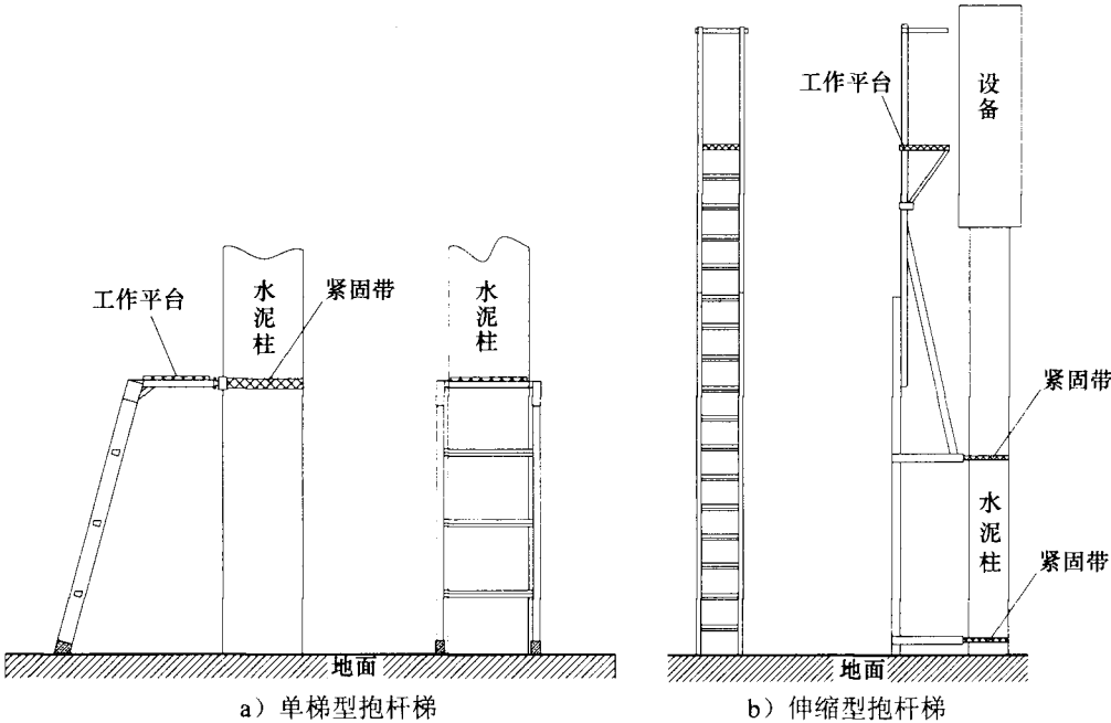
图 1 抱杆梯结构示意图
