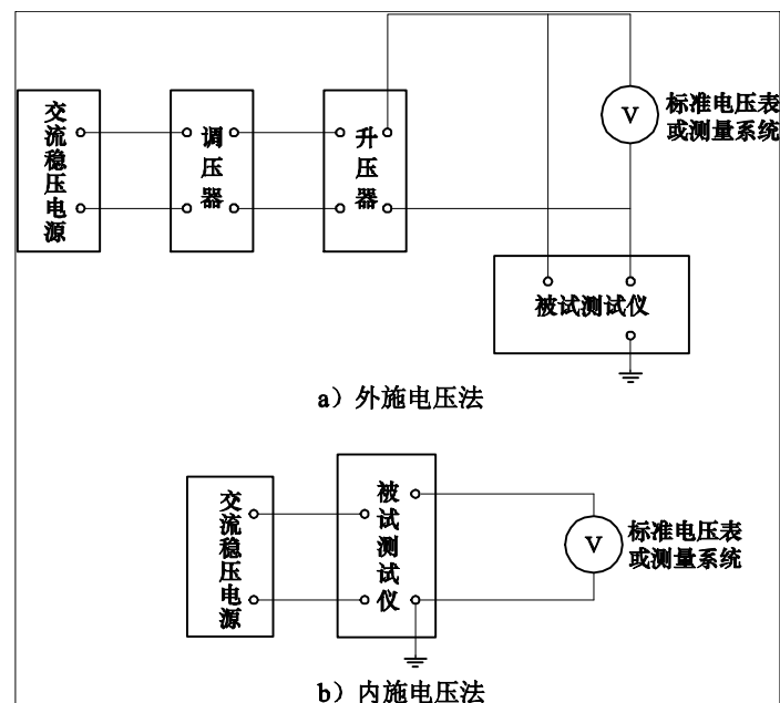
图 2 电压示值误差试验原理接线图
