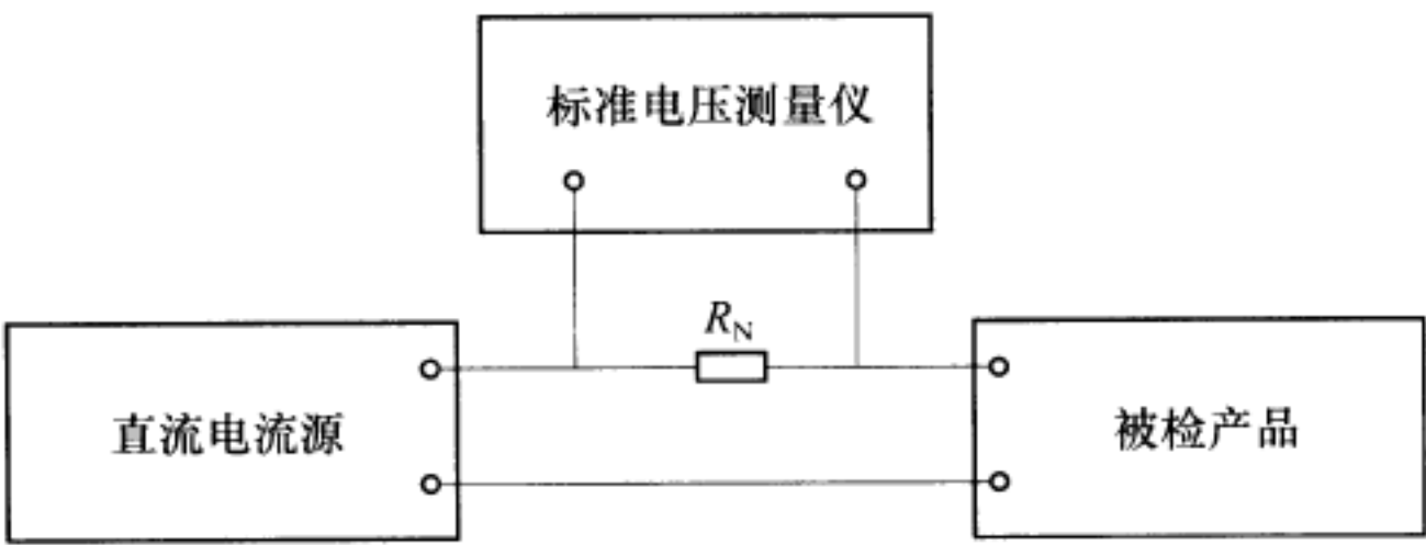
图 5 标准数字电压表法接线
