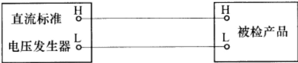
图 2 直流电压标准源法接线
