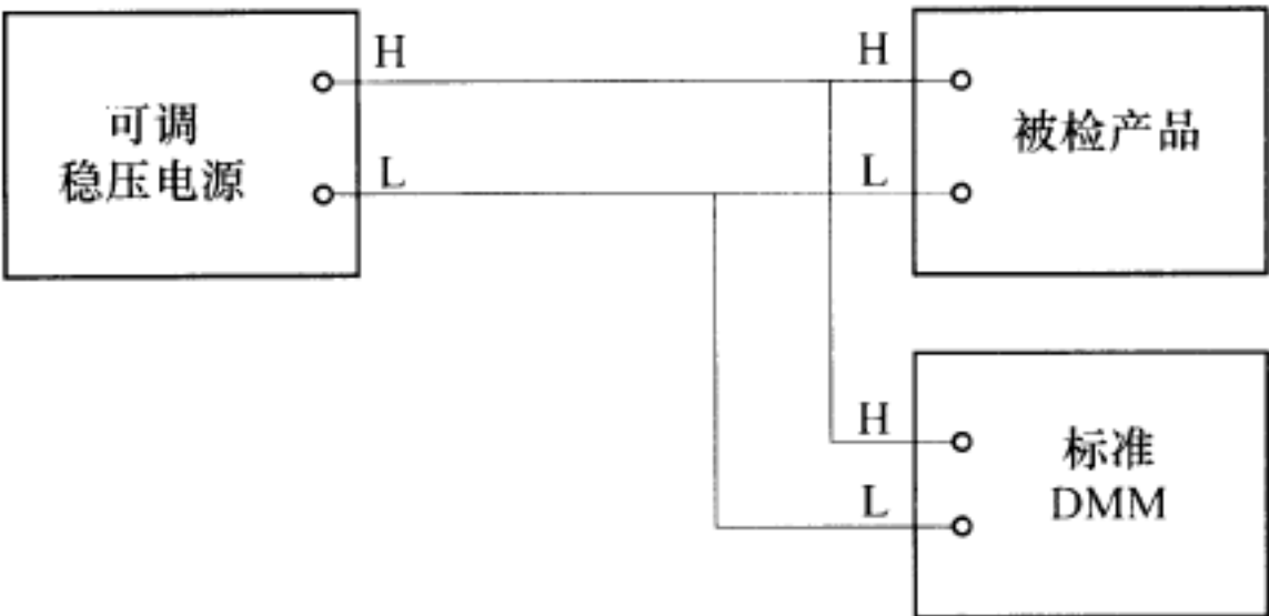
图 3 直流电压直接比较法接线
