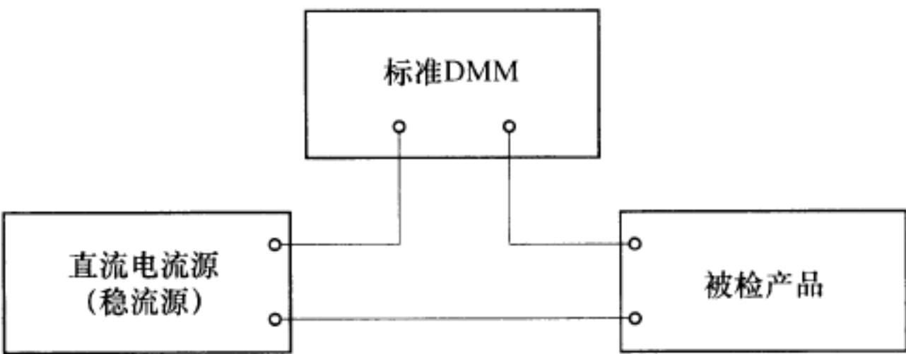
图 4 直流电流直接比较法接线
