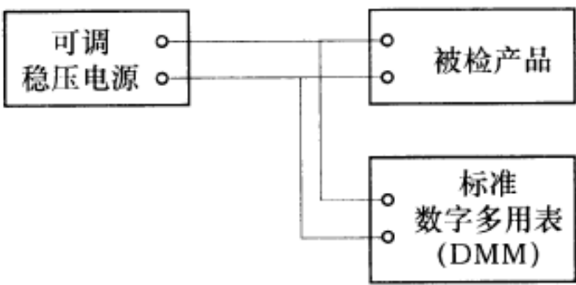
图 1 交流电压直接比较法接线
