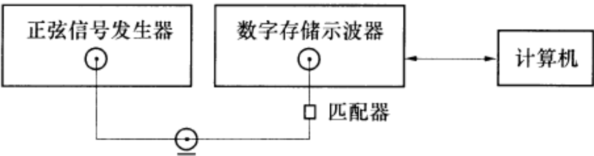
图 6 数字存储示波器校准接线
