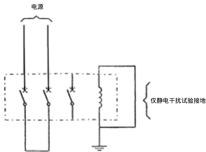
图F1 验证低频，静电和电磁场骚扰影响的试验电路
