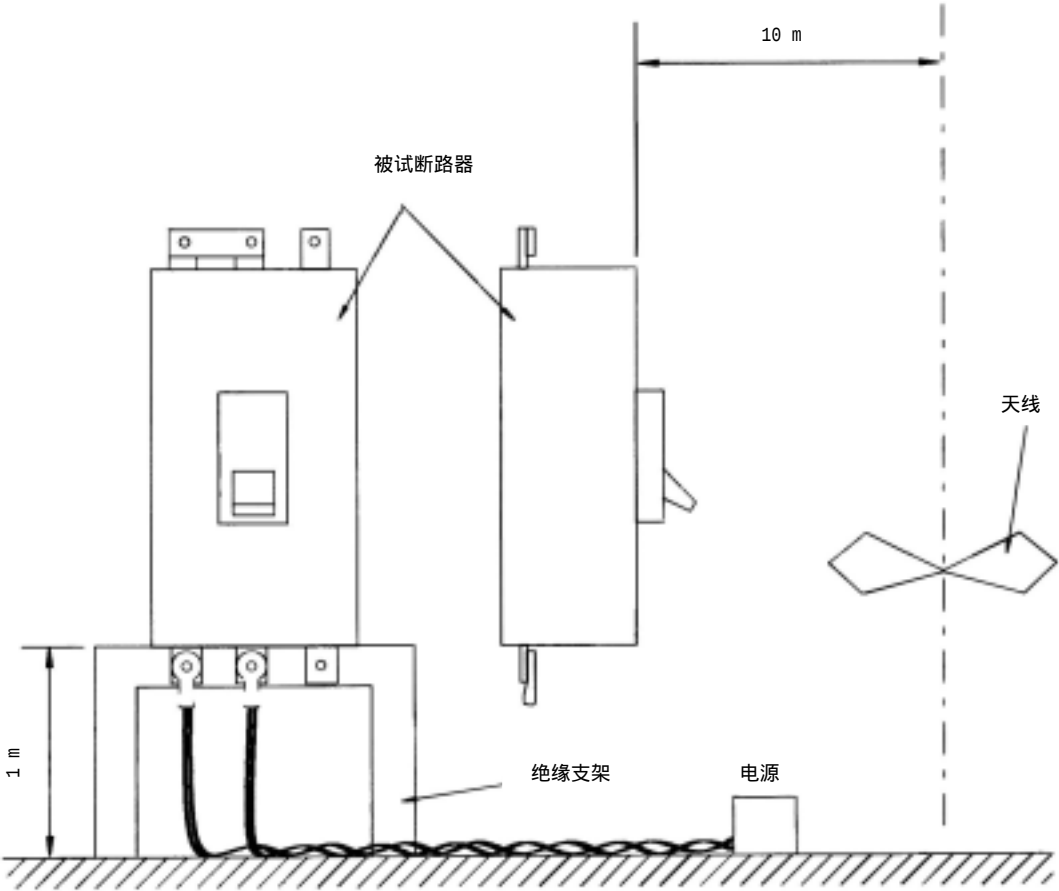
图F9 验证无线电射频发射的试验装置
