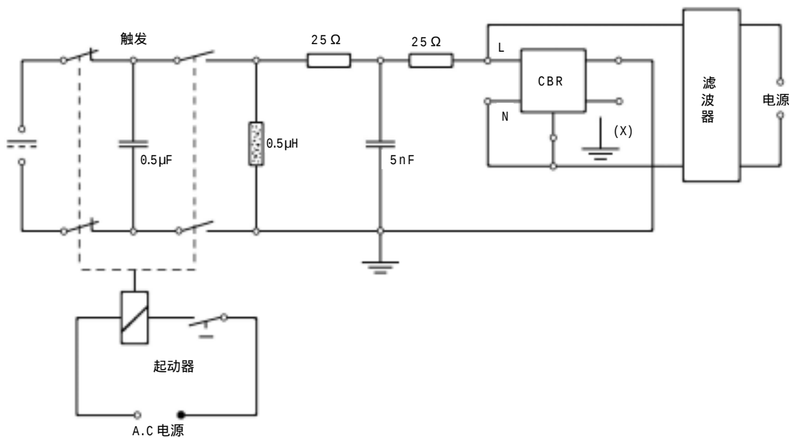
图 B4 电流振荡波 0.5 μs/100 kHz
