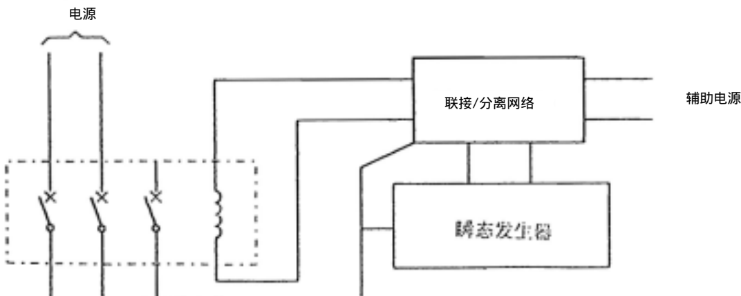
图F5 验证辅助电路瞬变影响的试验电路（共模式）
