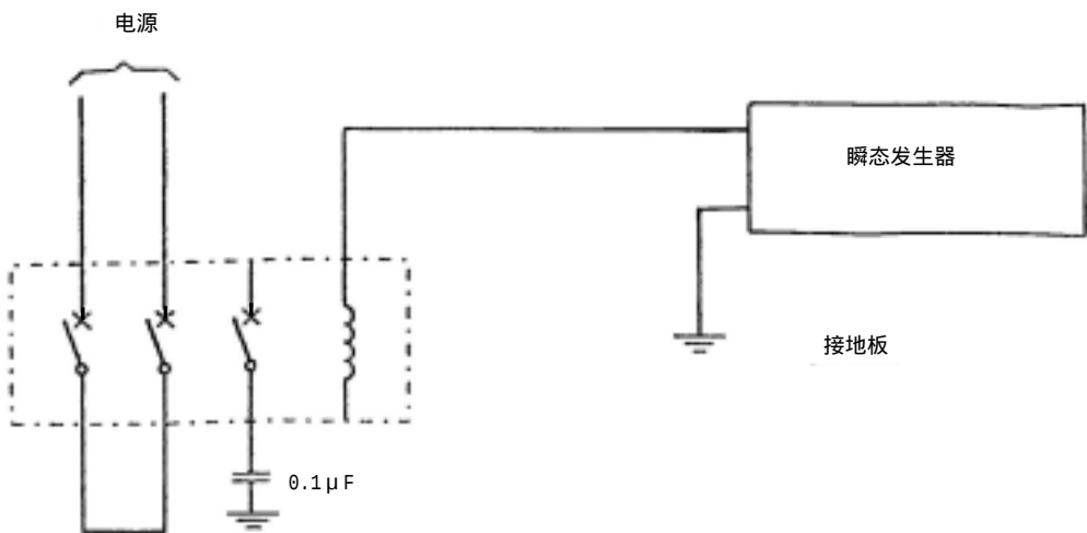
图F5 验证辅助电路瞬变影响的试验电路（共模式）
