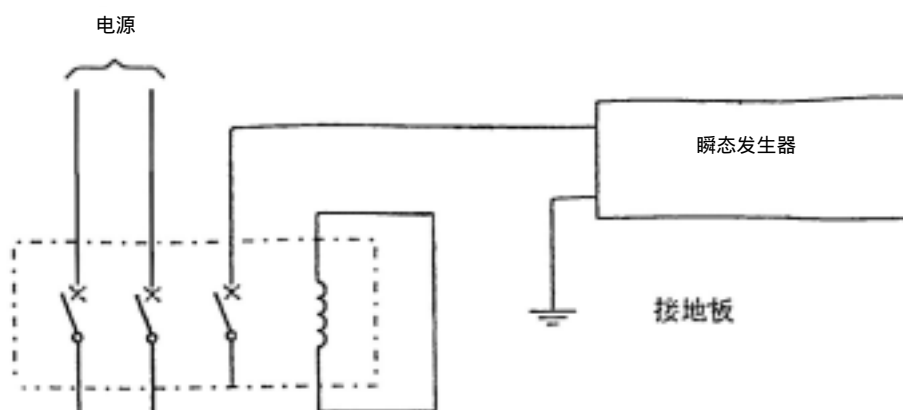
图F2 验证电流骤降和分断影响的试验电路
