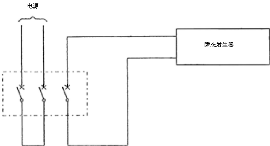
图F4 验证主电路瞬变影响的试验电路（差模式）
