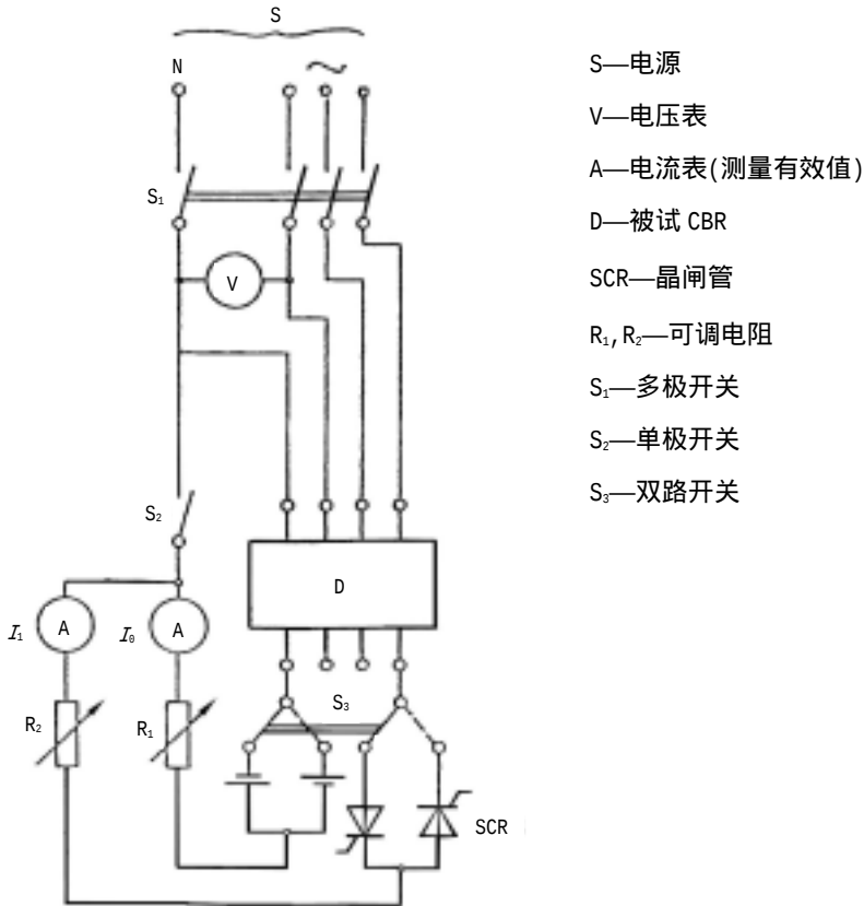
图B9 在剩余脉冲直流叠加平滑剩余直流（见B8.7.2.4）情况下 验证 CBR 动作正确性的试验电路
