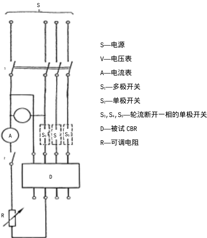
图 B3 验证按 B3.1.2.2.1（见 B8.9）分类 CBR 特性的试验电路
