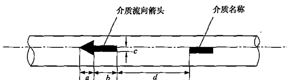
图 C.1 管道介质名称和介质流向箭头的位置和形状
