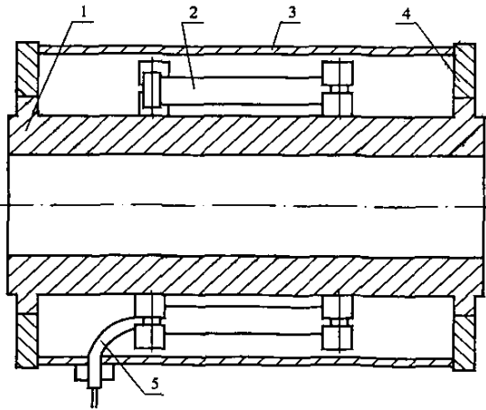
1—钢筒；2—差动电阻式应变计；3—护壳；4—护盘；5—引出电缆
