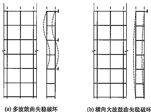
图 1 作业脚手架失稳破坏示意
