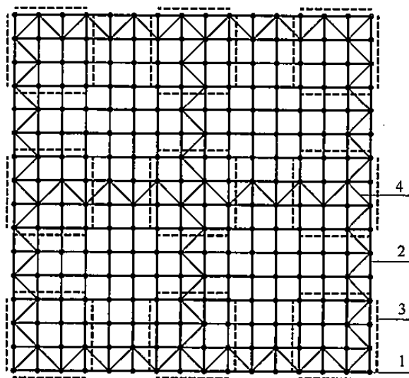
图 8.3.5-3 竖向塔形桁架、水平斜撑杆布置示意
