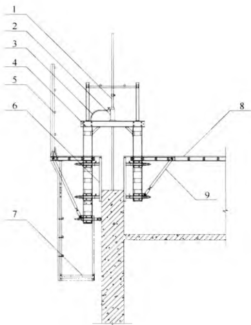
图 2 高层建筑滑模装置剖面图
