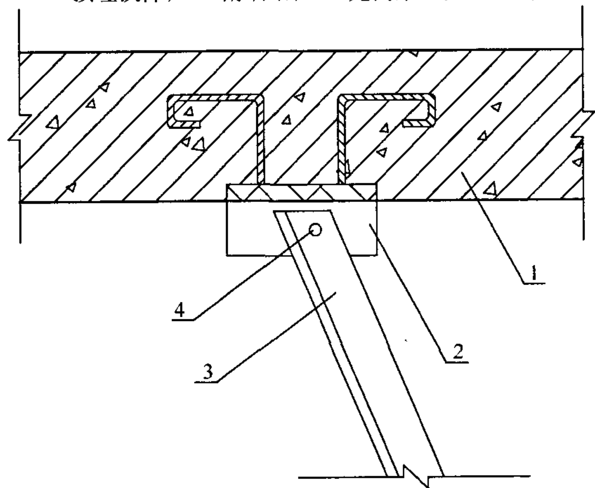
图 A.0.1-2 节点详图
