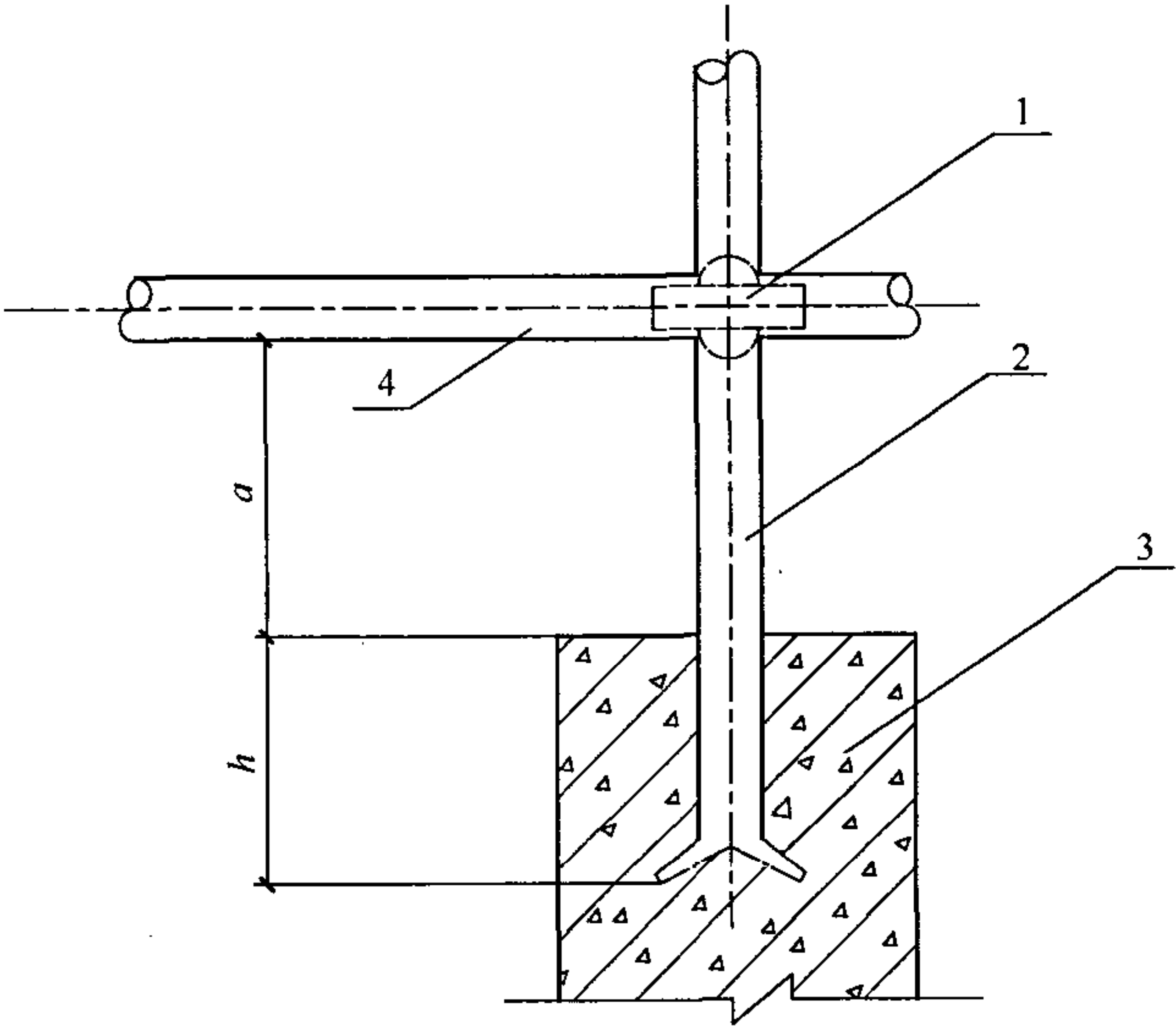
图 A.0.2 钢管附墙架与预埋钢管连接
