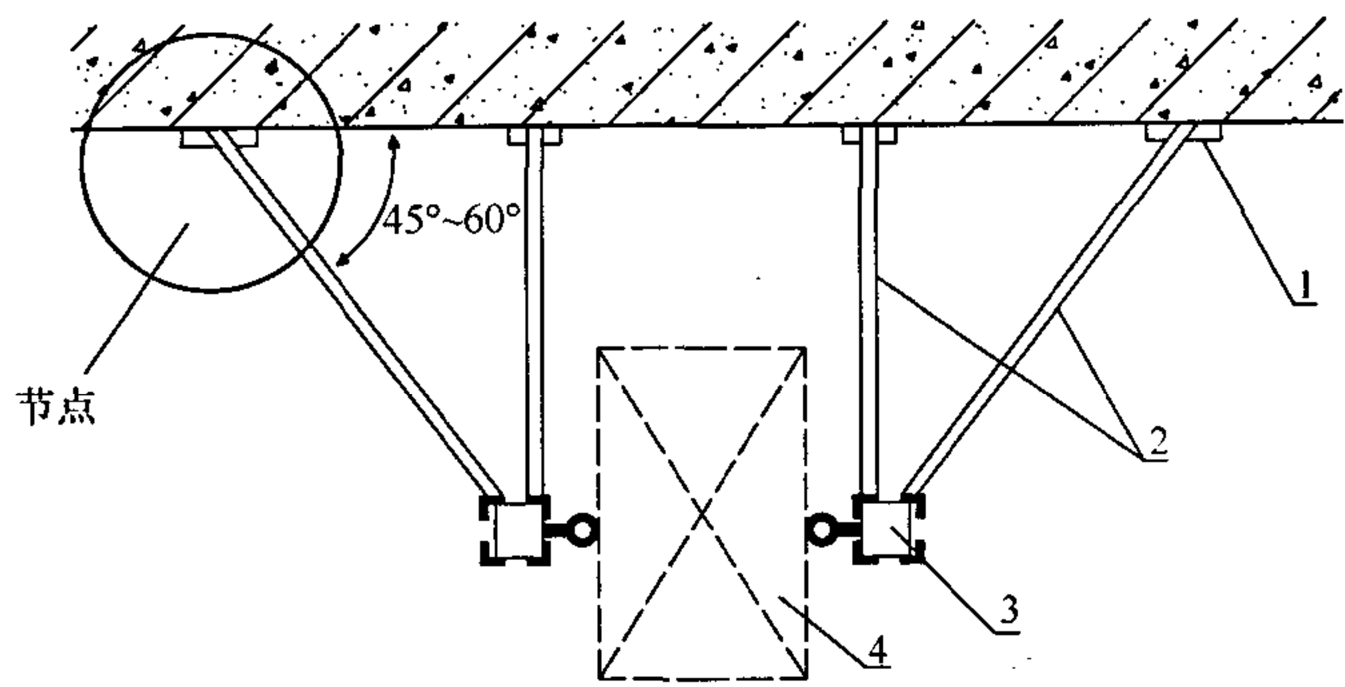
图 A.0.1-1 型钢附墙架与埋件连接
