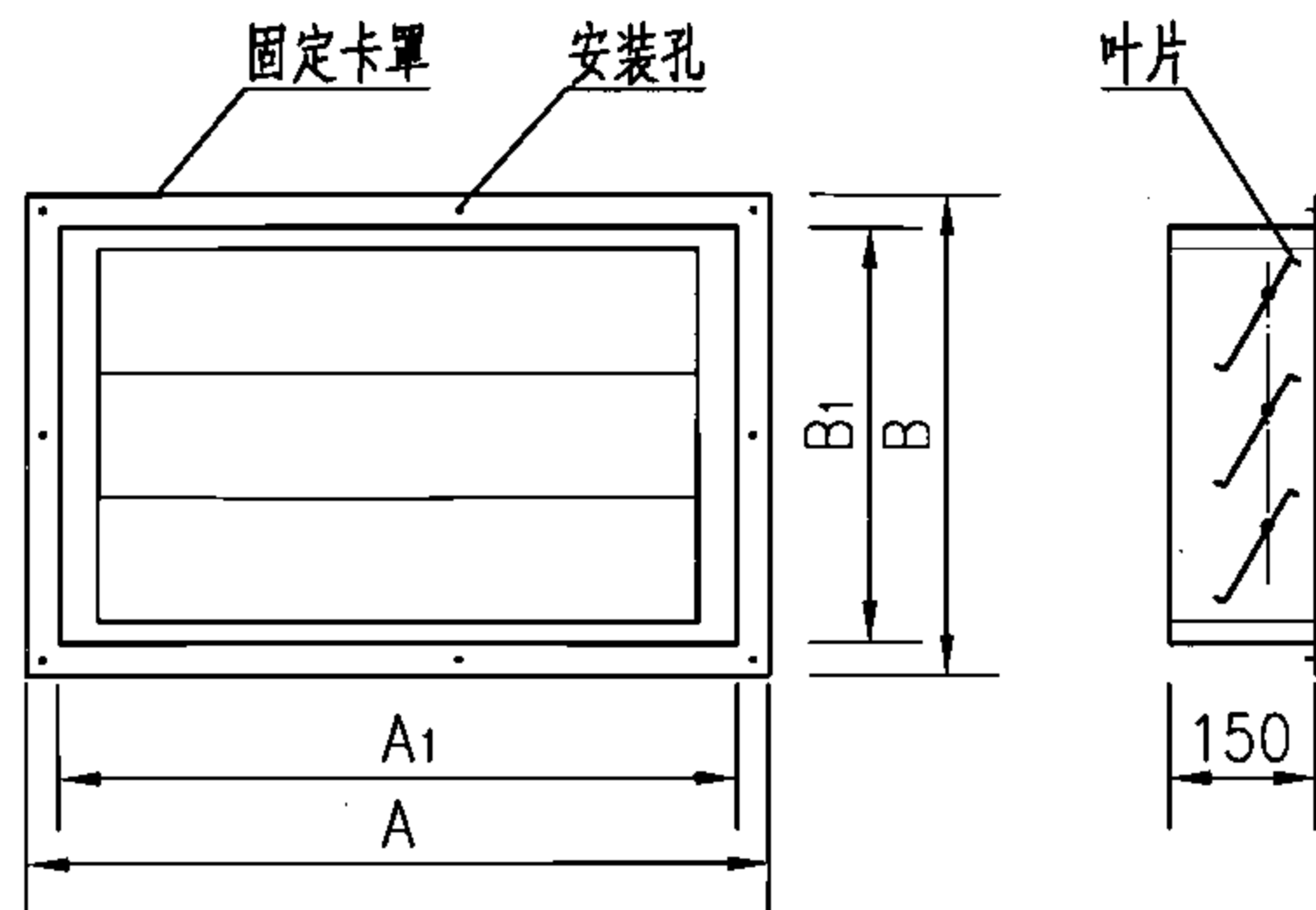
XYK系列机械式开启泄压阀外形图
