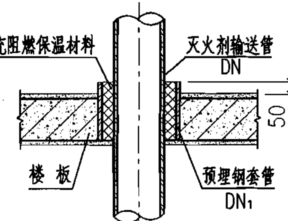
管道穿楼板敷设安装图
