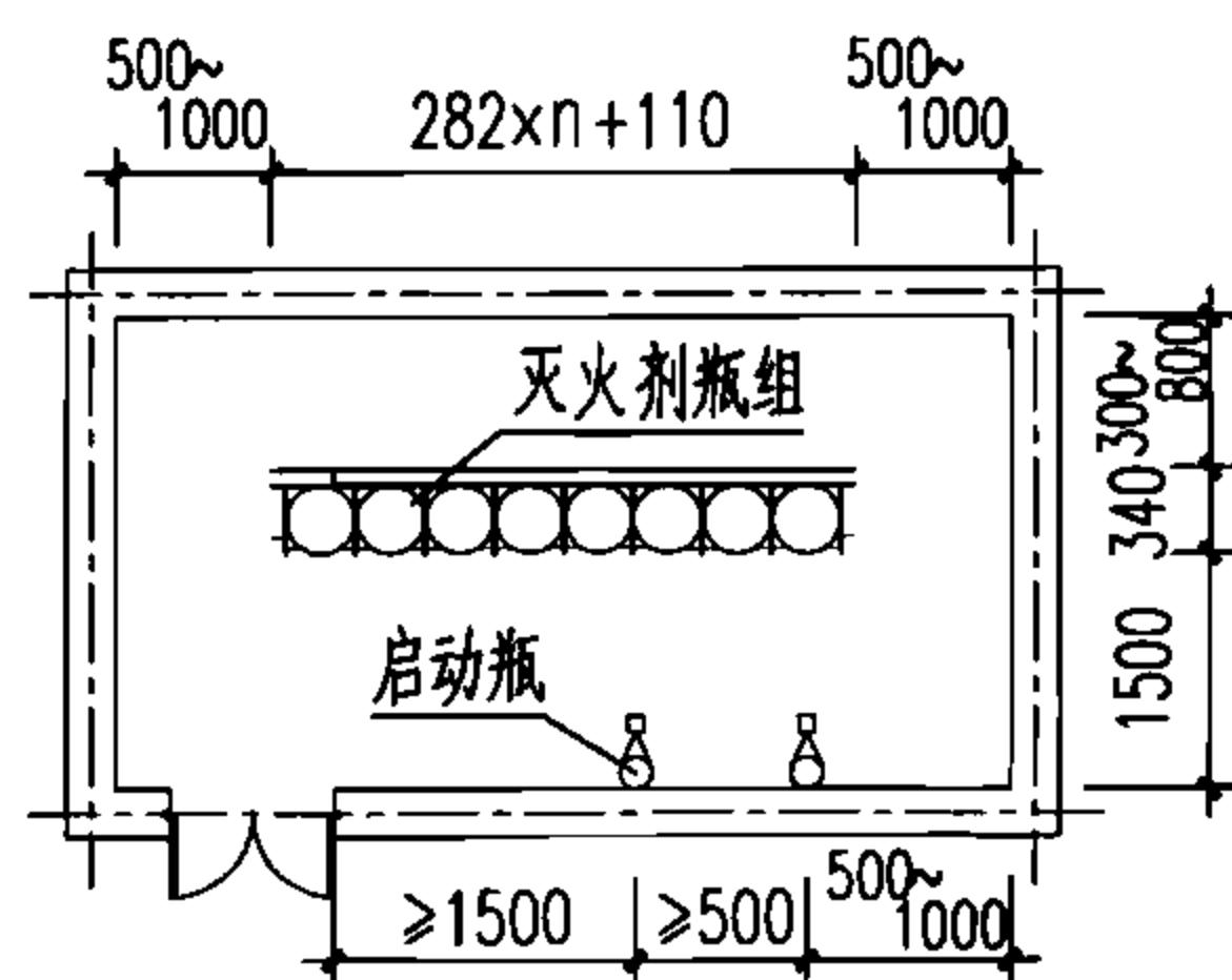
单排储瓶布置图
