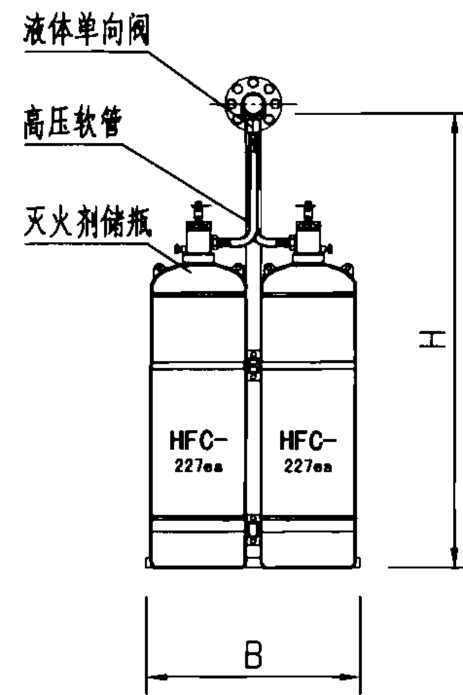
双排钢瓶侧视图
