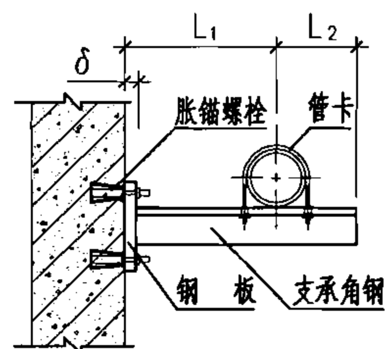
沿墙（柱）安装单管托架图 (DN15~DN50)
