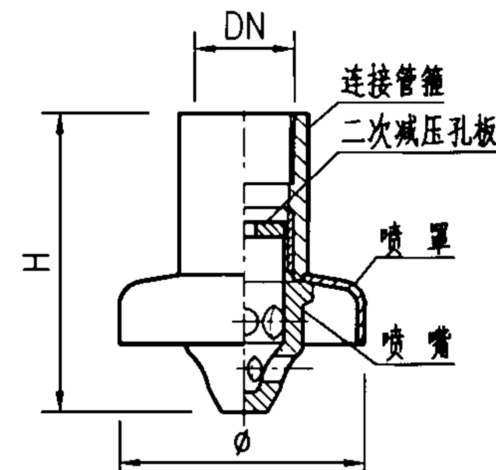
带喷罩的喷嘴
