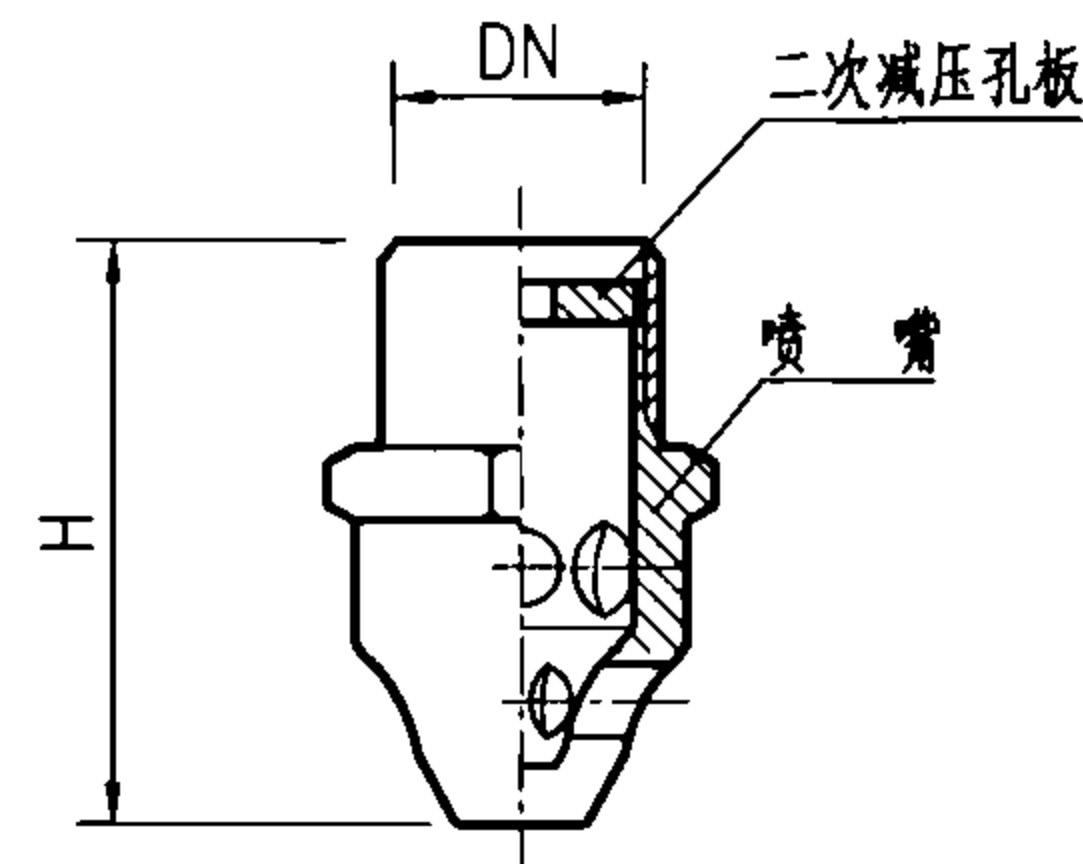
不带喷罩的喷嘴
