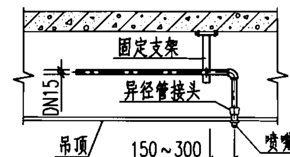
防护区有吊顶喷嘴安装图
