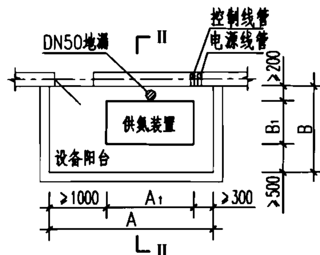
平面布置图
