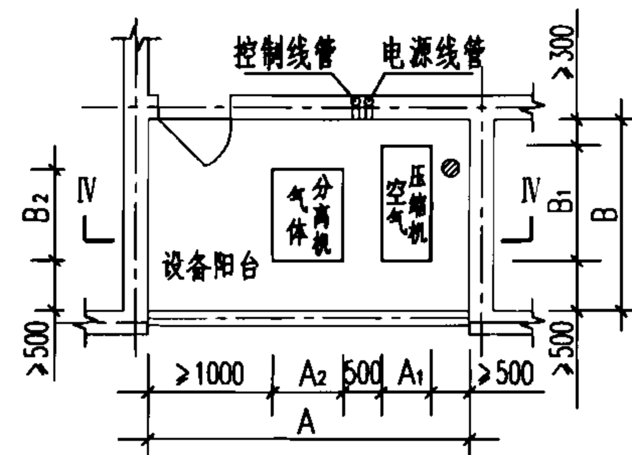
平面布置图
