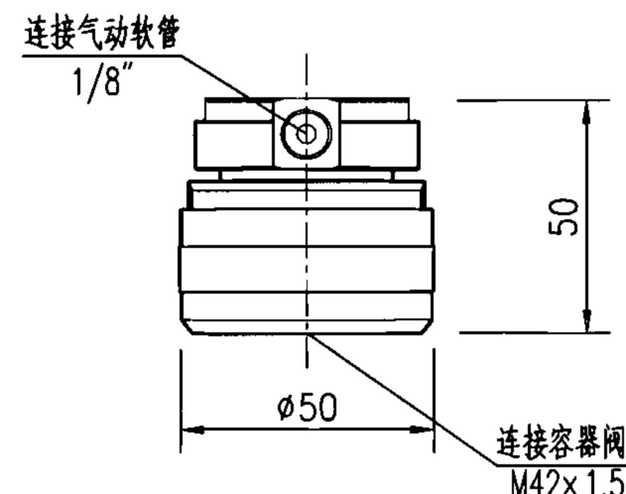
电磁启动阀
