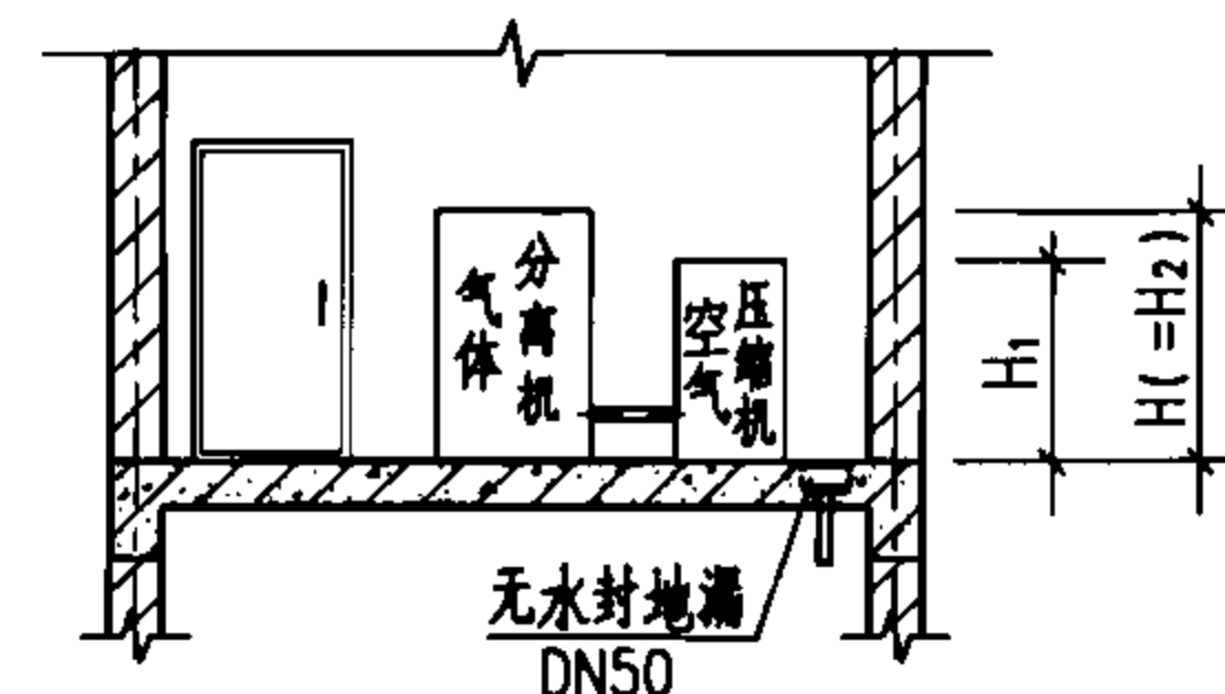
IV-IV 剖面图
