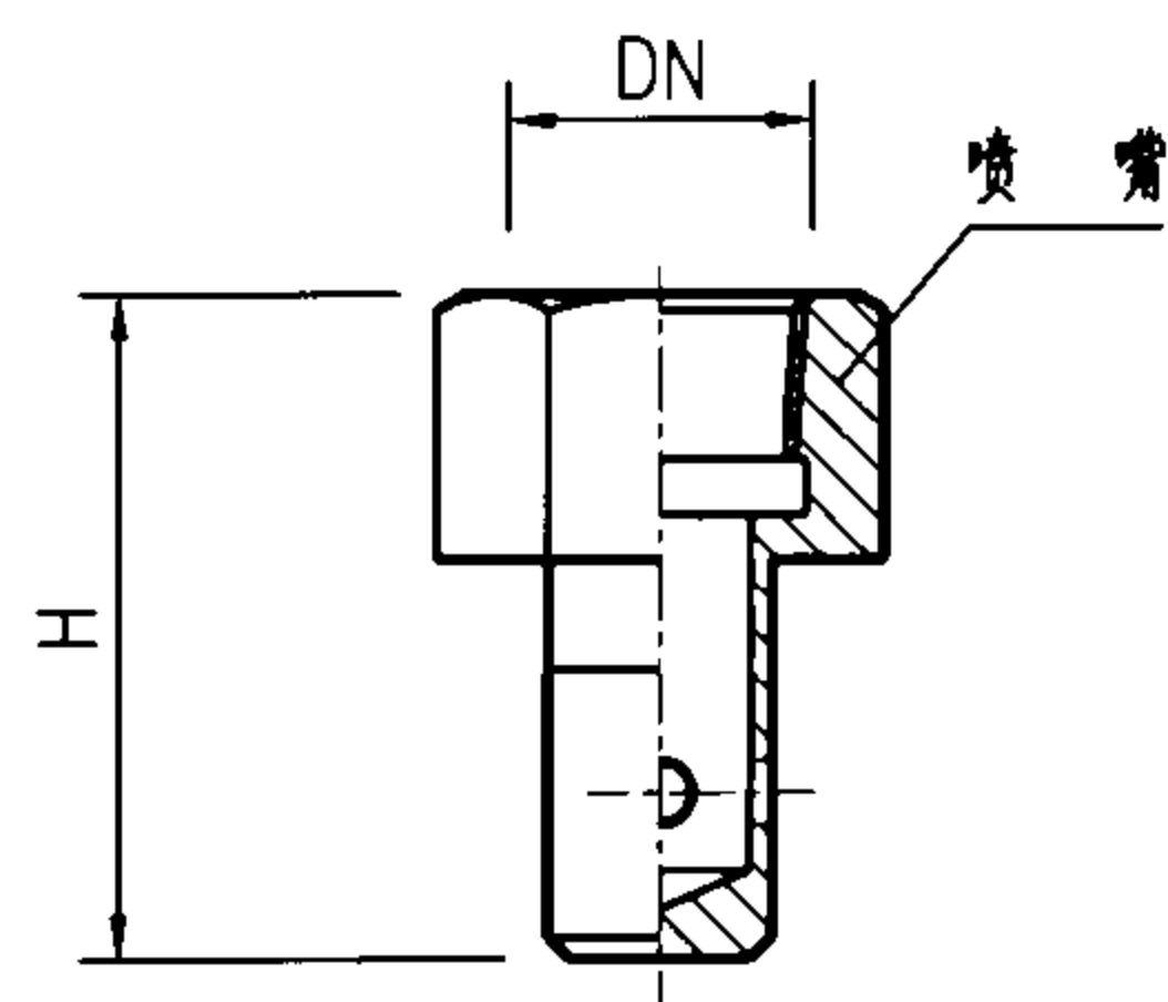
不带喷罩的喷嘴
