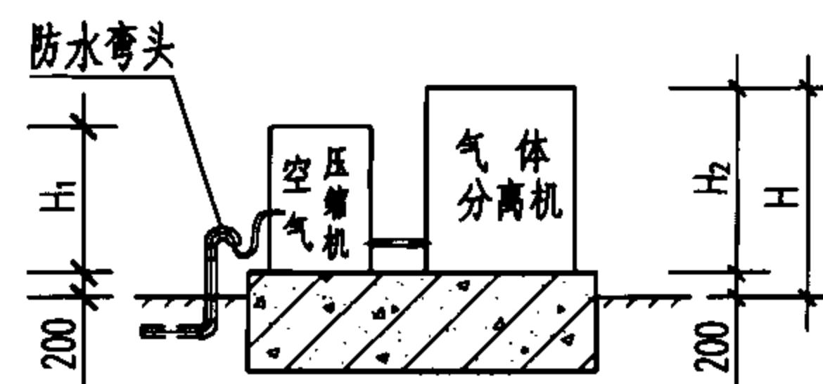
III-III 剖面图
