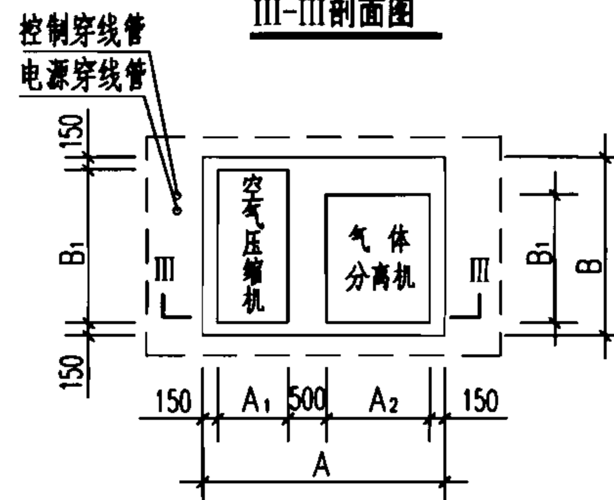
平面布置图
