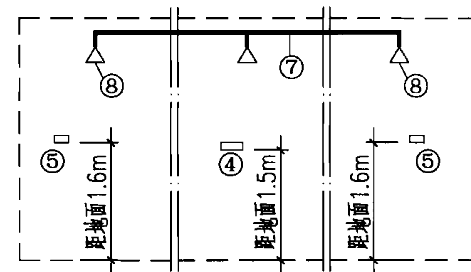
主控制器、氧浓度探测器、注氮管路立面布置图
