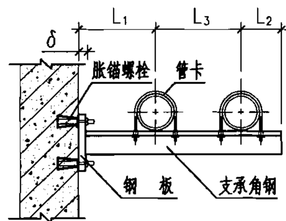
沿墙（柱）安装双管托架图 (DN15~DN40)
