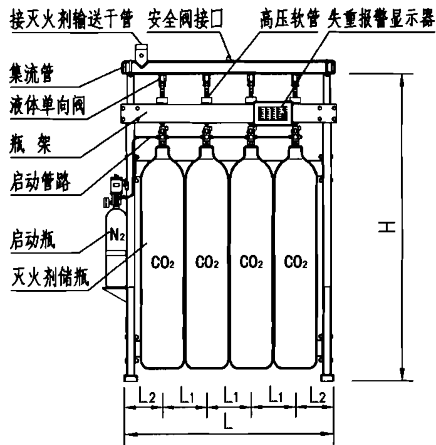
单元独立系统储存装置外形图
