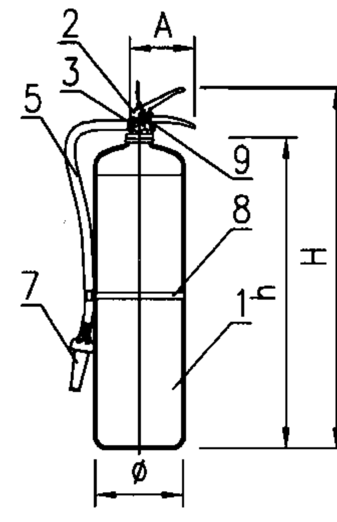
水基型灭火器外形图 (MSZ/AR3~9、MPZ/AR3~9)
