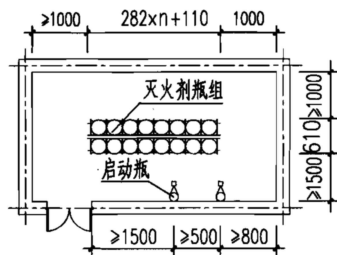
双排储瓶布置图
