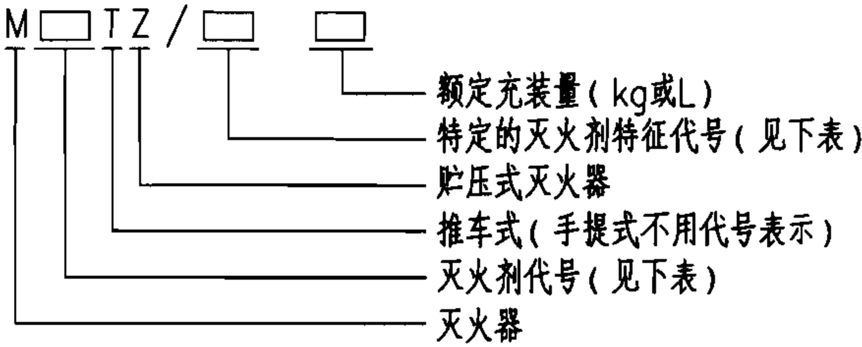
灭火剂代号和特定的灭火剂特征代号
