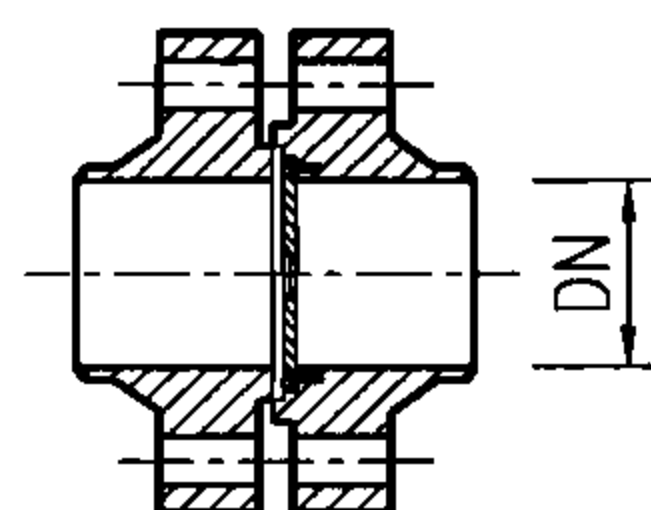
法兰连接减压装置 (DN80~150)
