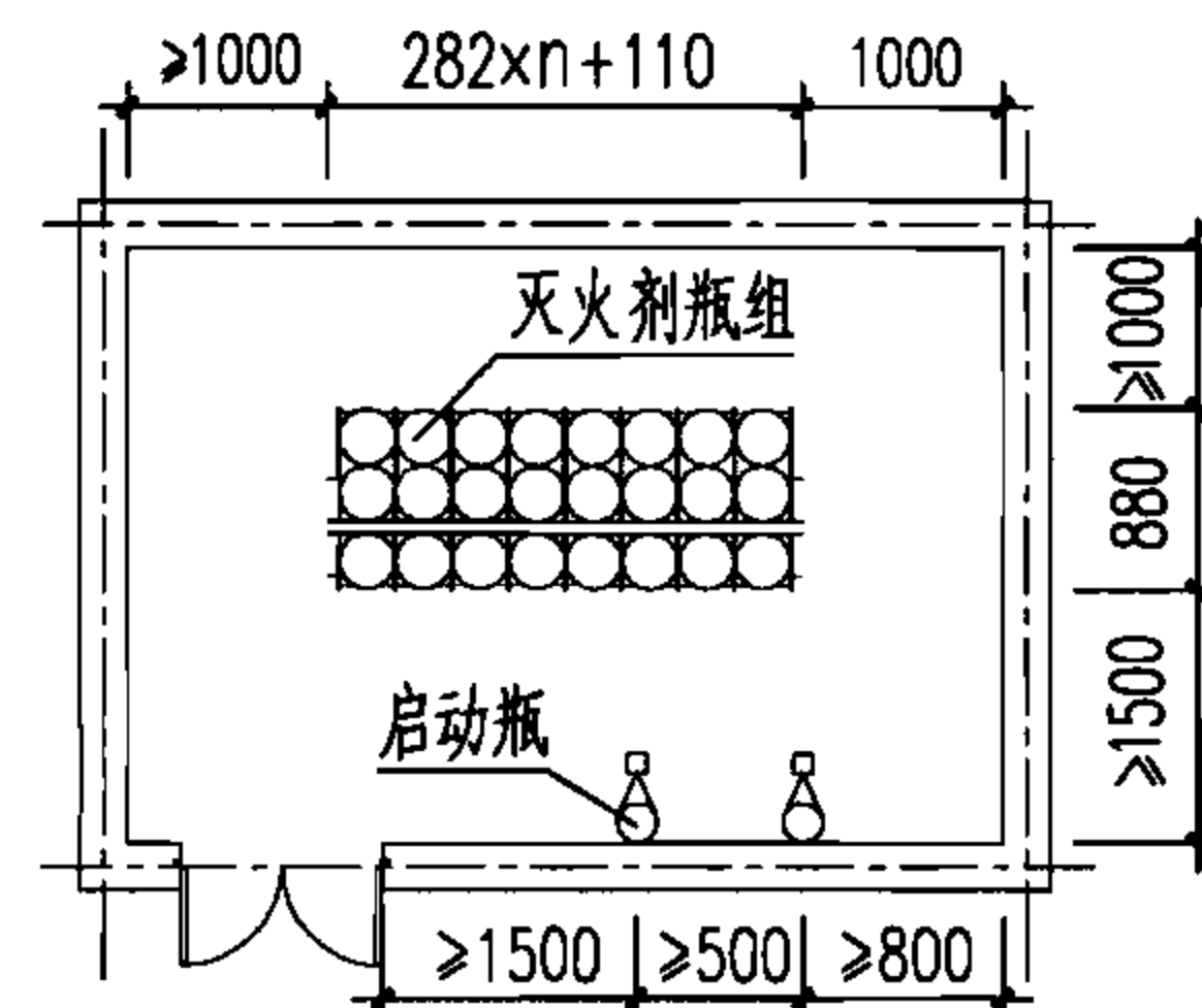
三排储瓶布置图
