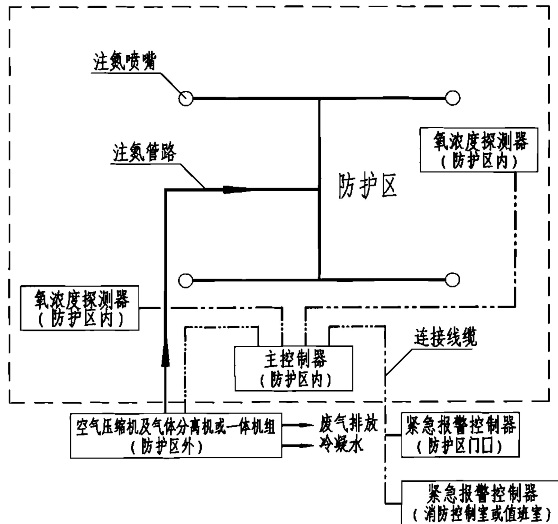
单元独立系统原理图
