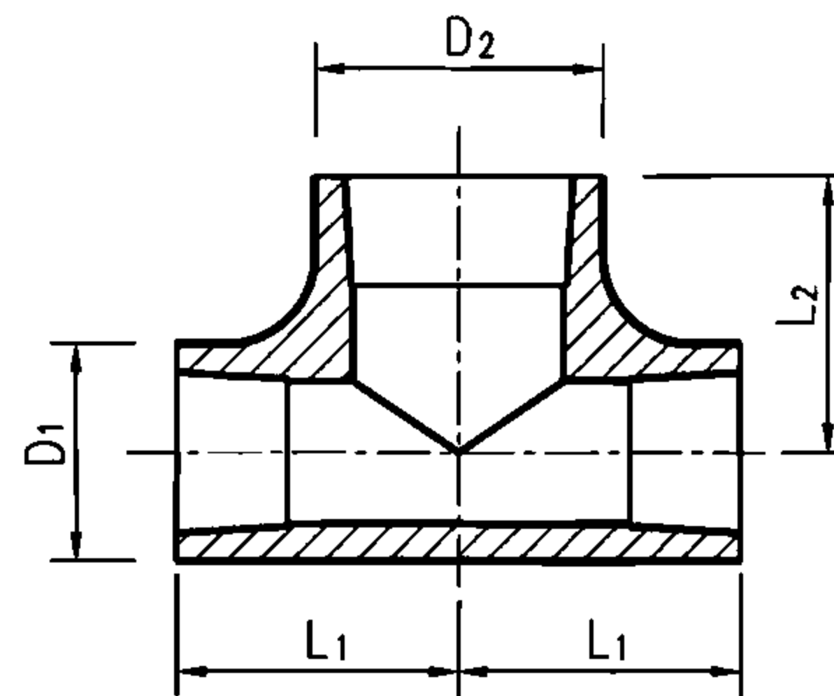
异径三通
