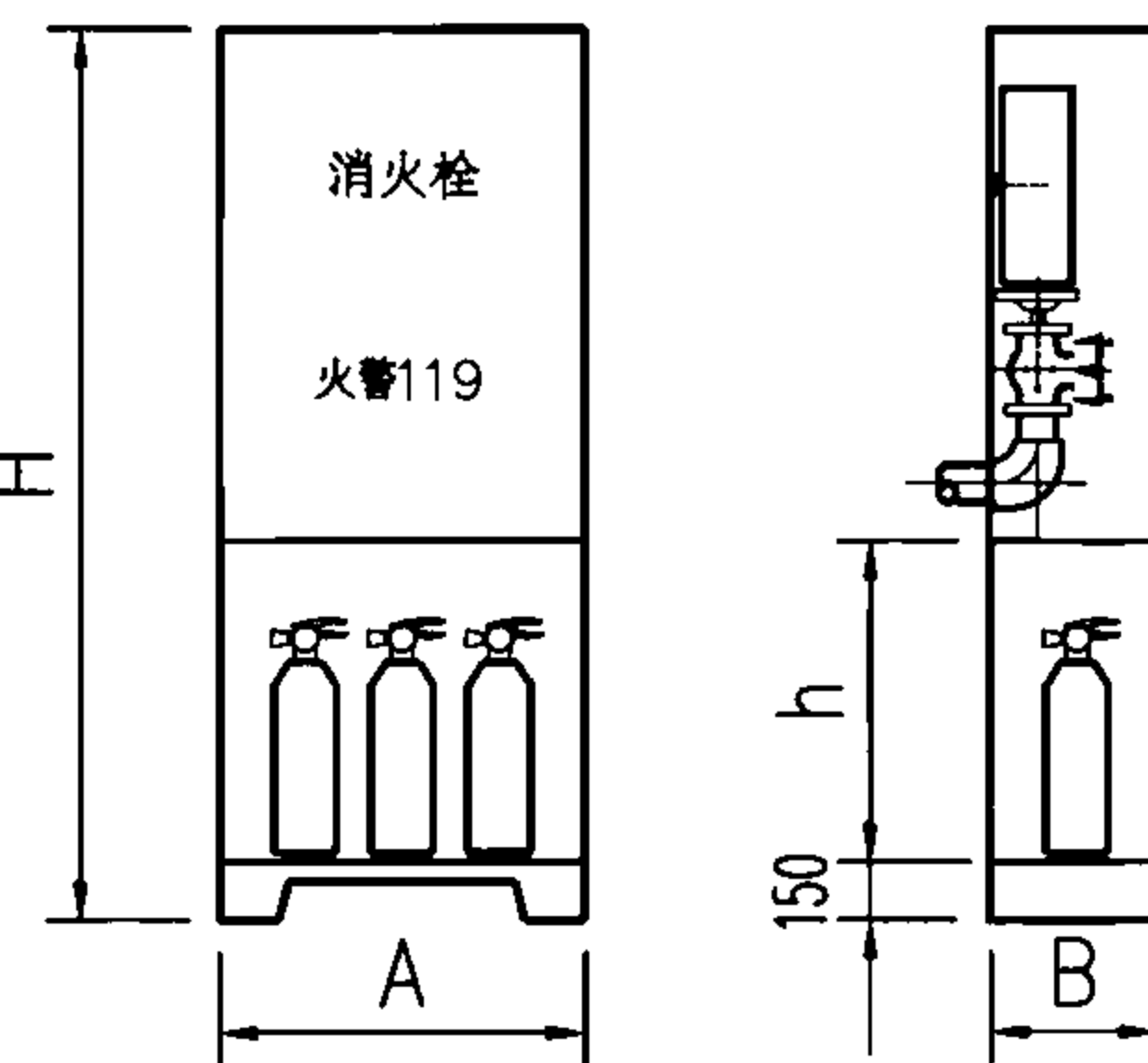
落地型带灭火器箱组合式消防柜外形图
