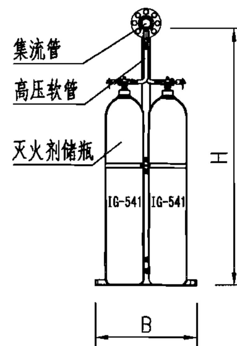
双排瓶组钢瓶侧视图
