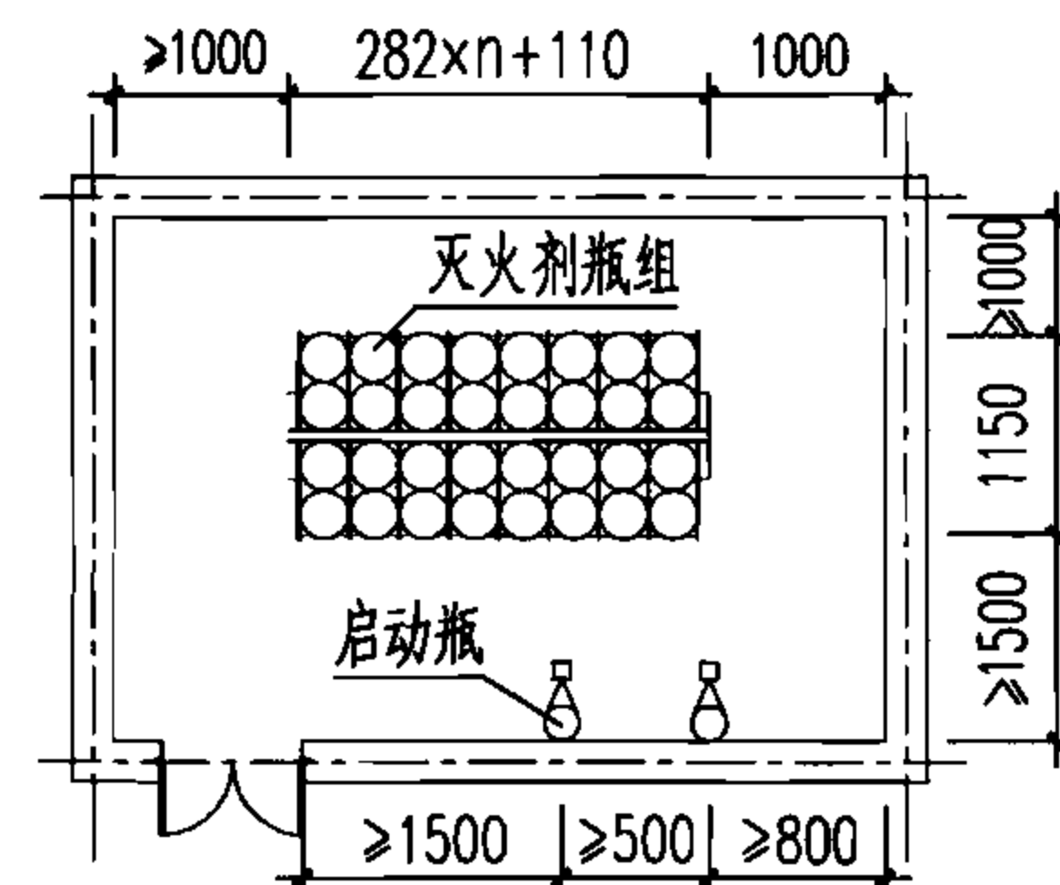
四排储瓶布置图
