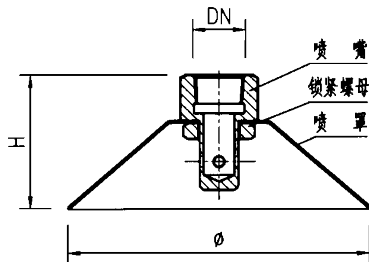
带喷罩的喷嘴
