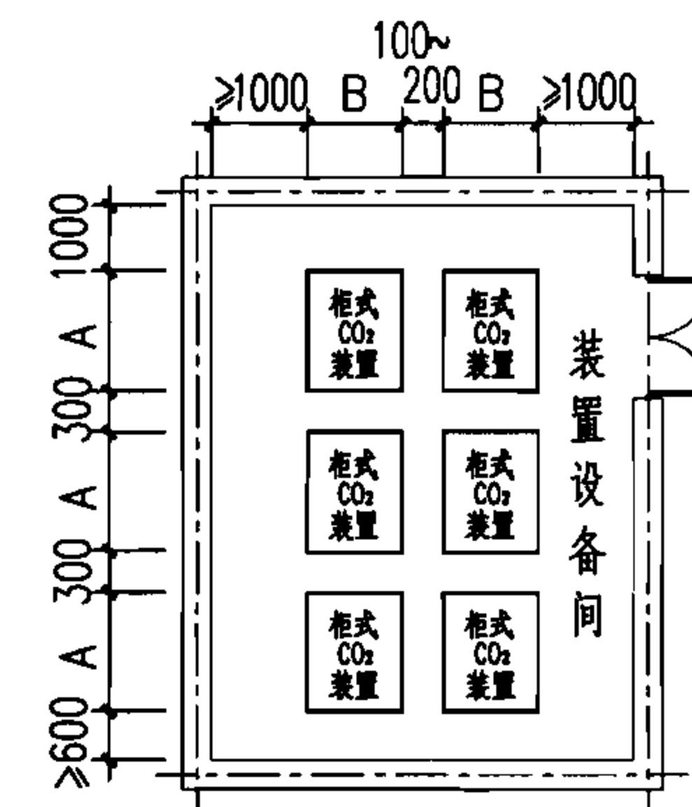
柜式低压CO 2 装置设备间布置图
