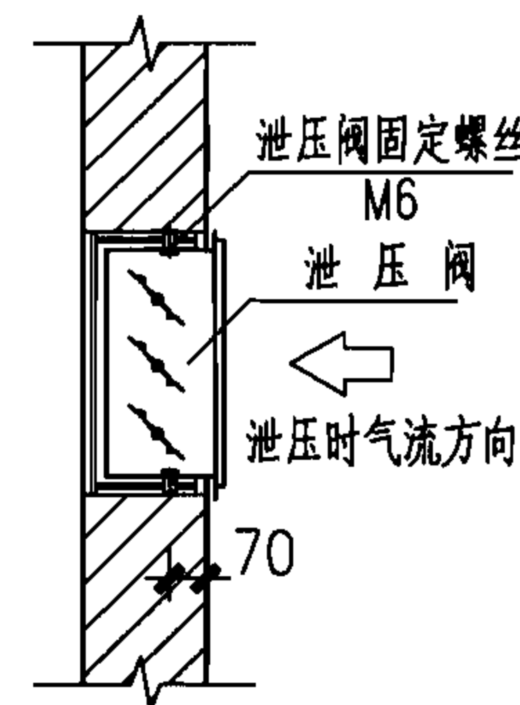
泄压阀安装图 (以 FXY-III 型为例)
