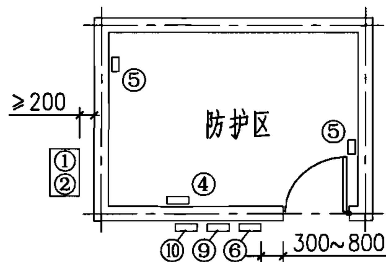
无管网系统组件平面布置图
