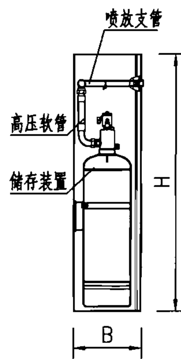
三氟甲烷装置剖视图
