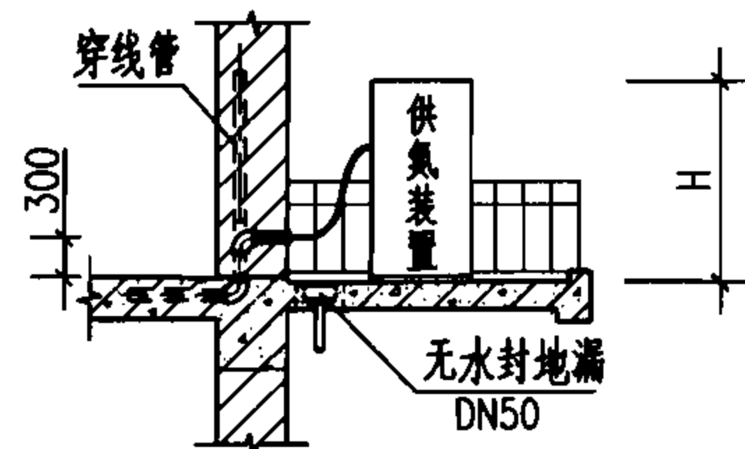
II-II 剖面图
