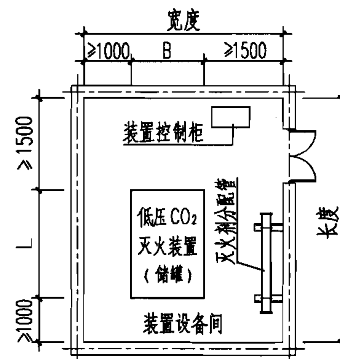
储罐式、整体式低压CO 2 装置设备间布置图
