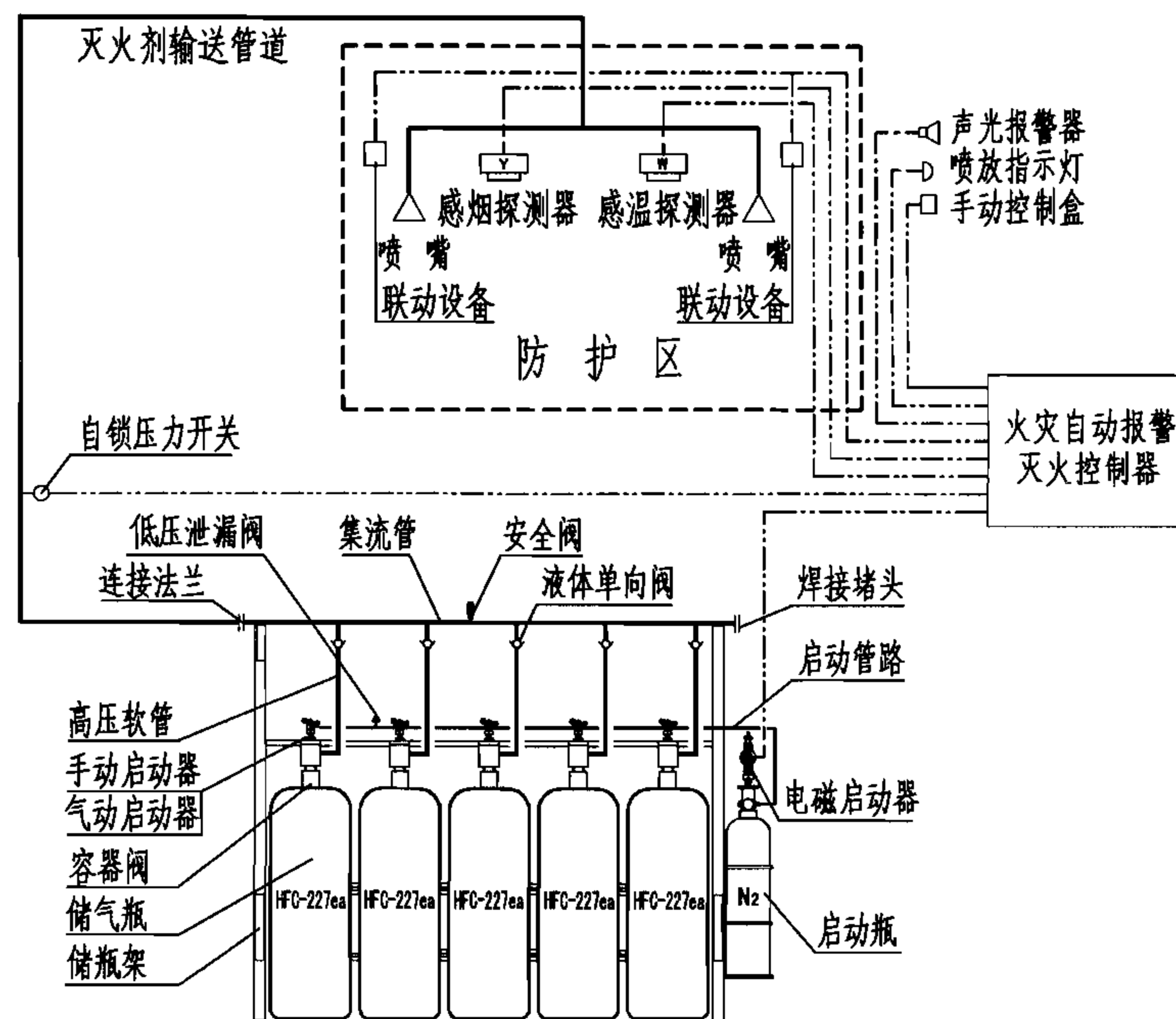
七氟丙烷单元独立系统原理图
