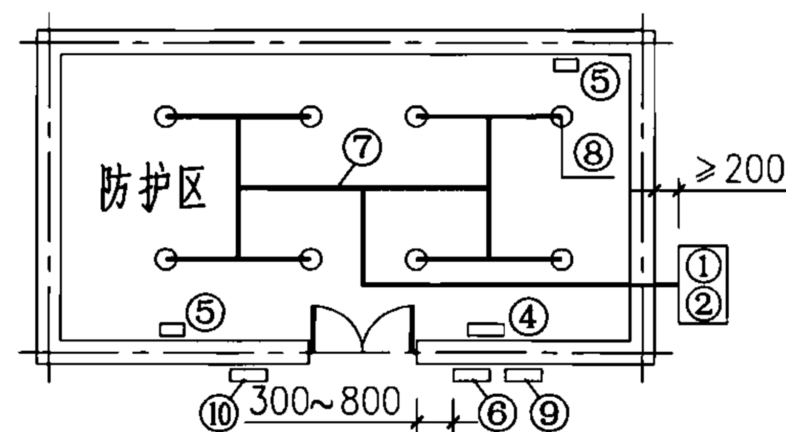
有管网系统组件平面布置图
