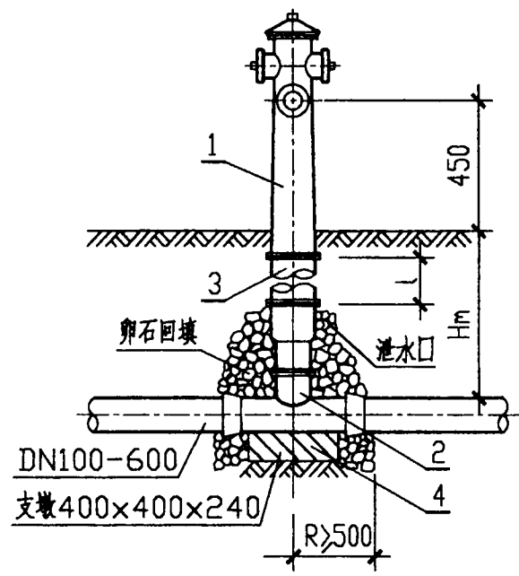
1-1 剖面图
