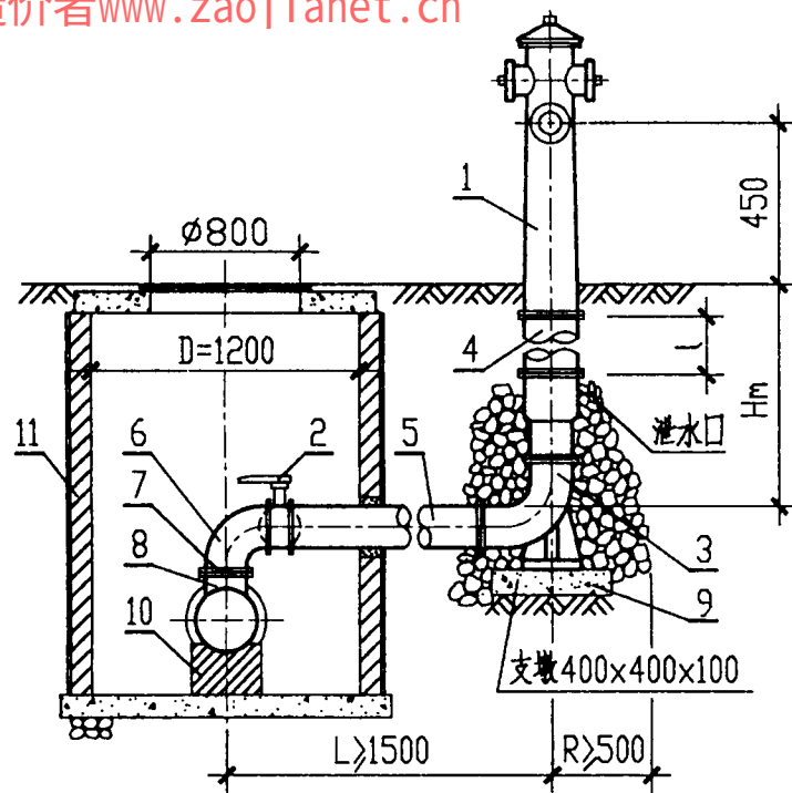
1-1 剖面图
