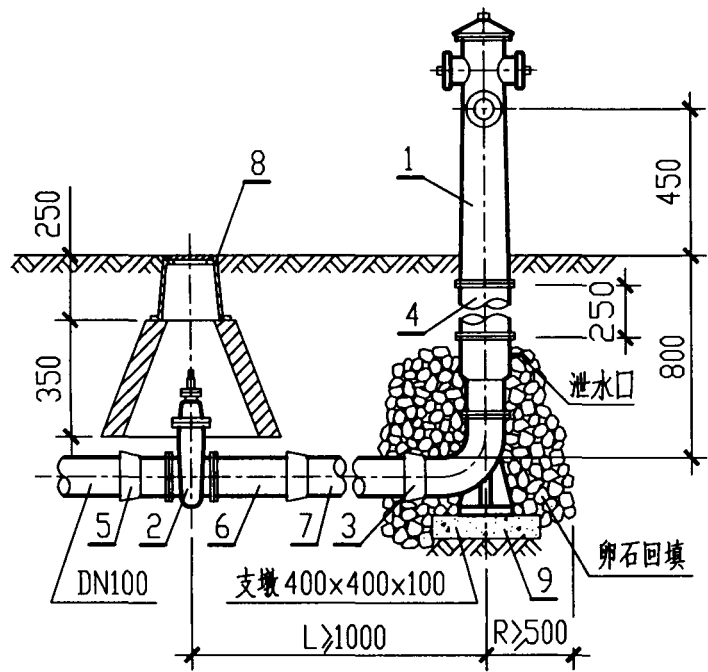
1-1 剖面图
