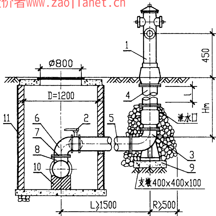
1-1 剖面图
