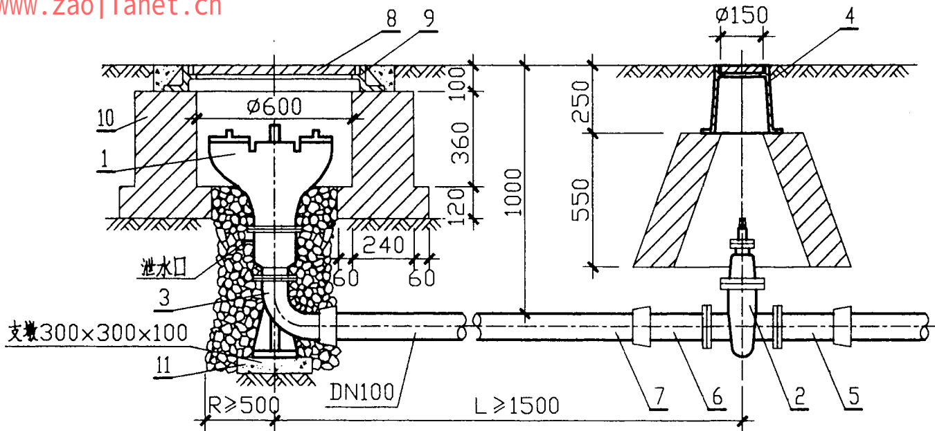
1-1 剖面图
