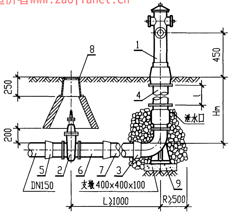
1-1 剖面图
