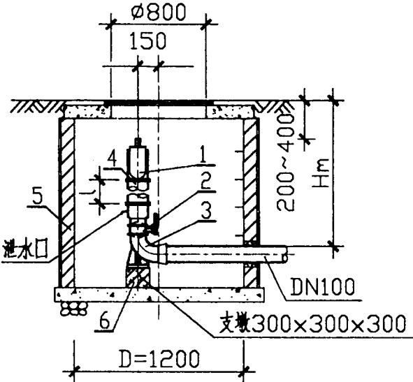
1-1 剖面图
