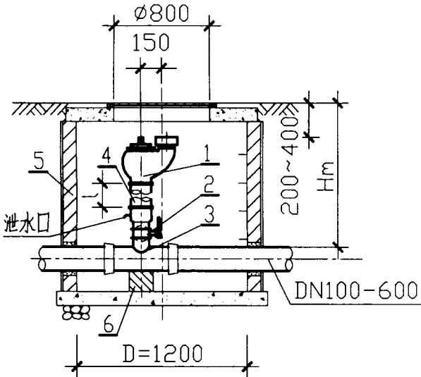
1-1 剖面图
