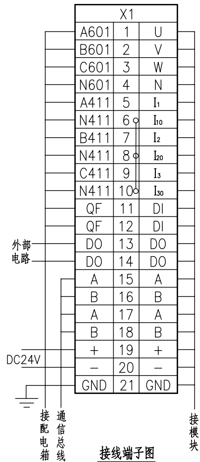
三相有中性线风机、泵类电压电流监测电路图
