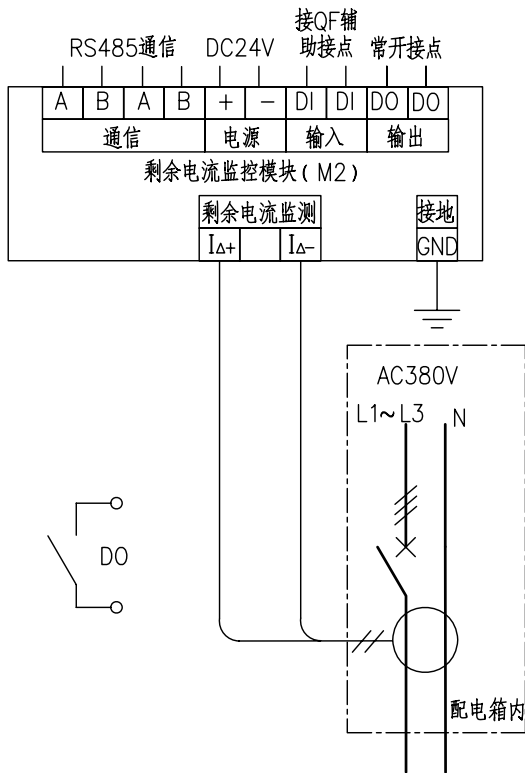
原理图 (三相有中性线)
