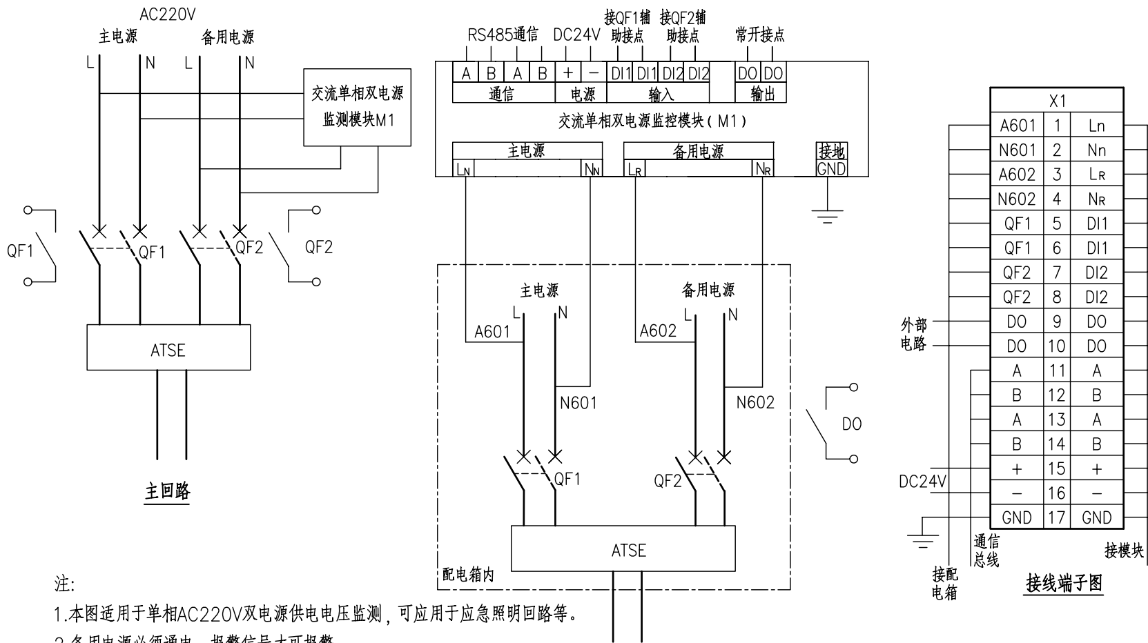
原理图
