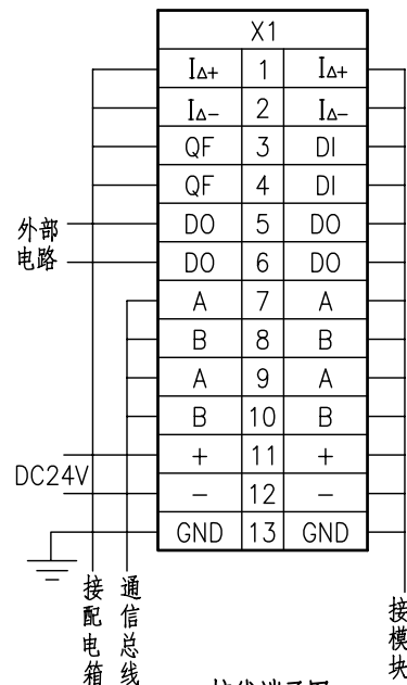
接线端子图
