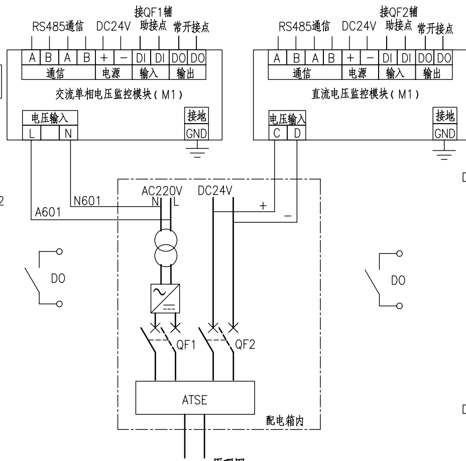
原理图
