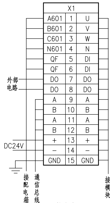
接线端子图
