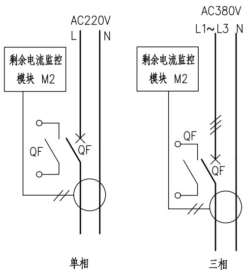
主回路
