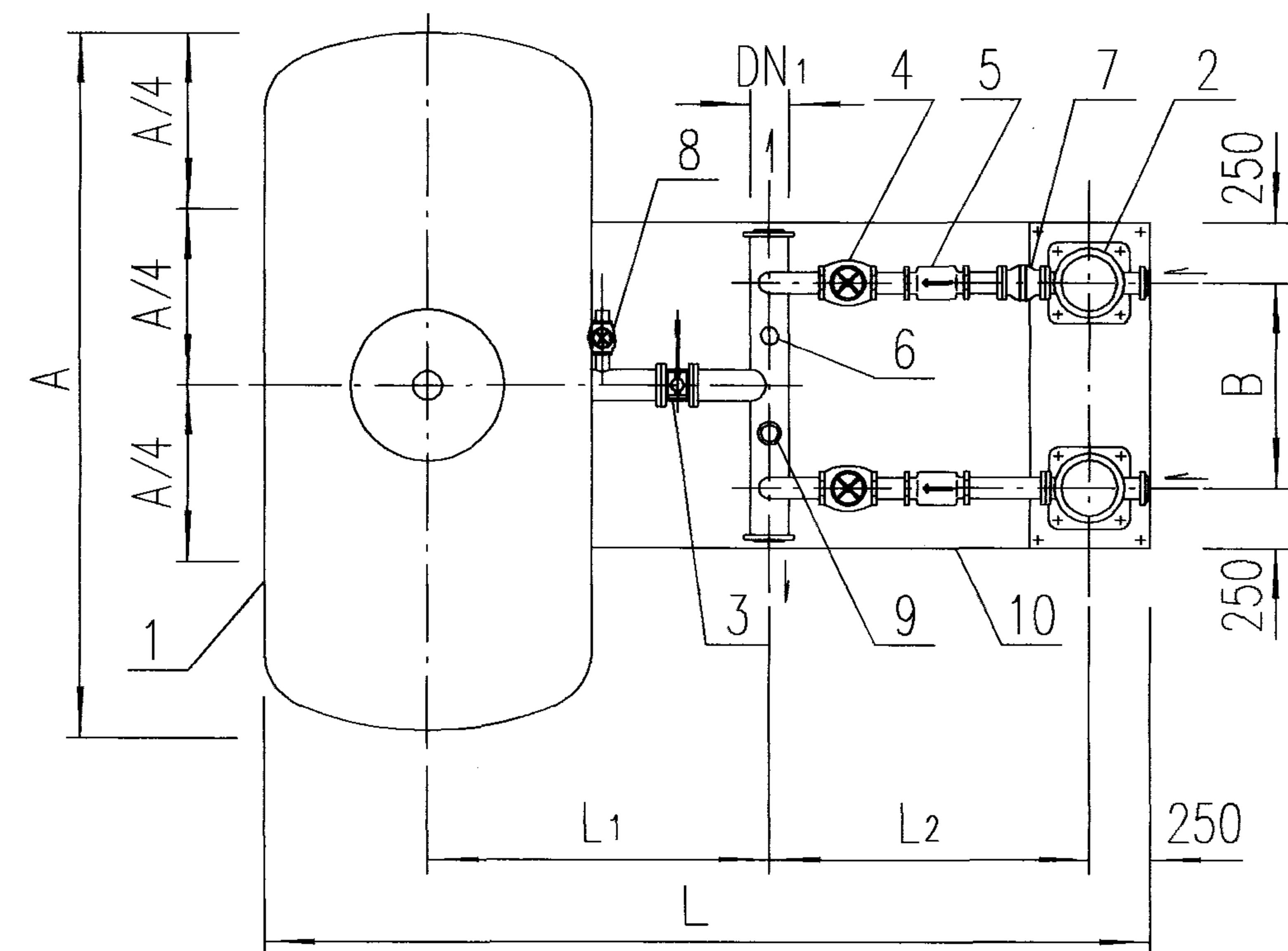
平面图
