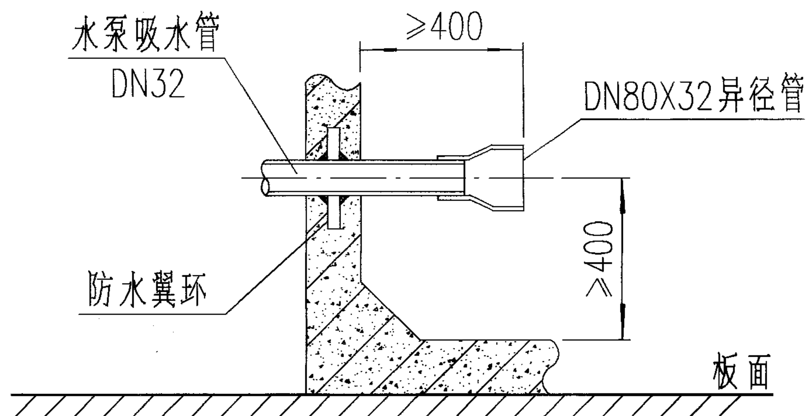
(a) 适用于钢筋混凝土水池
