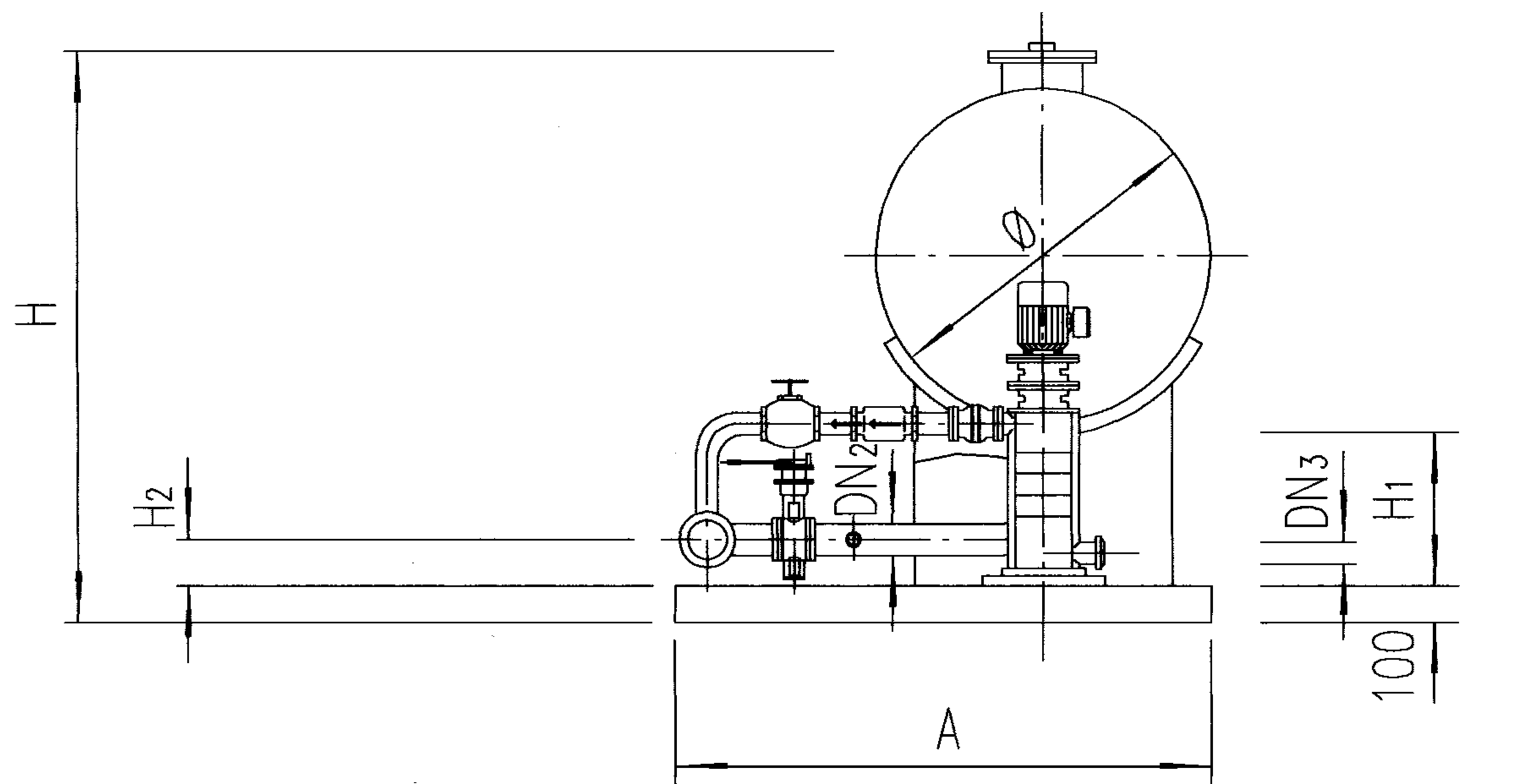
右立视图
