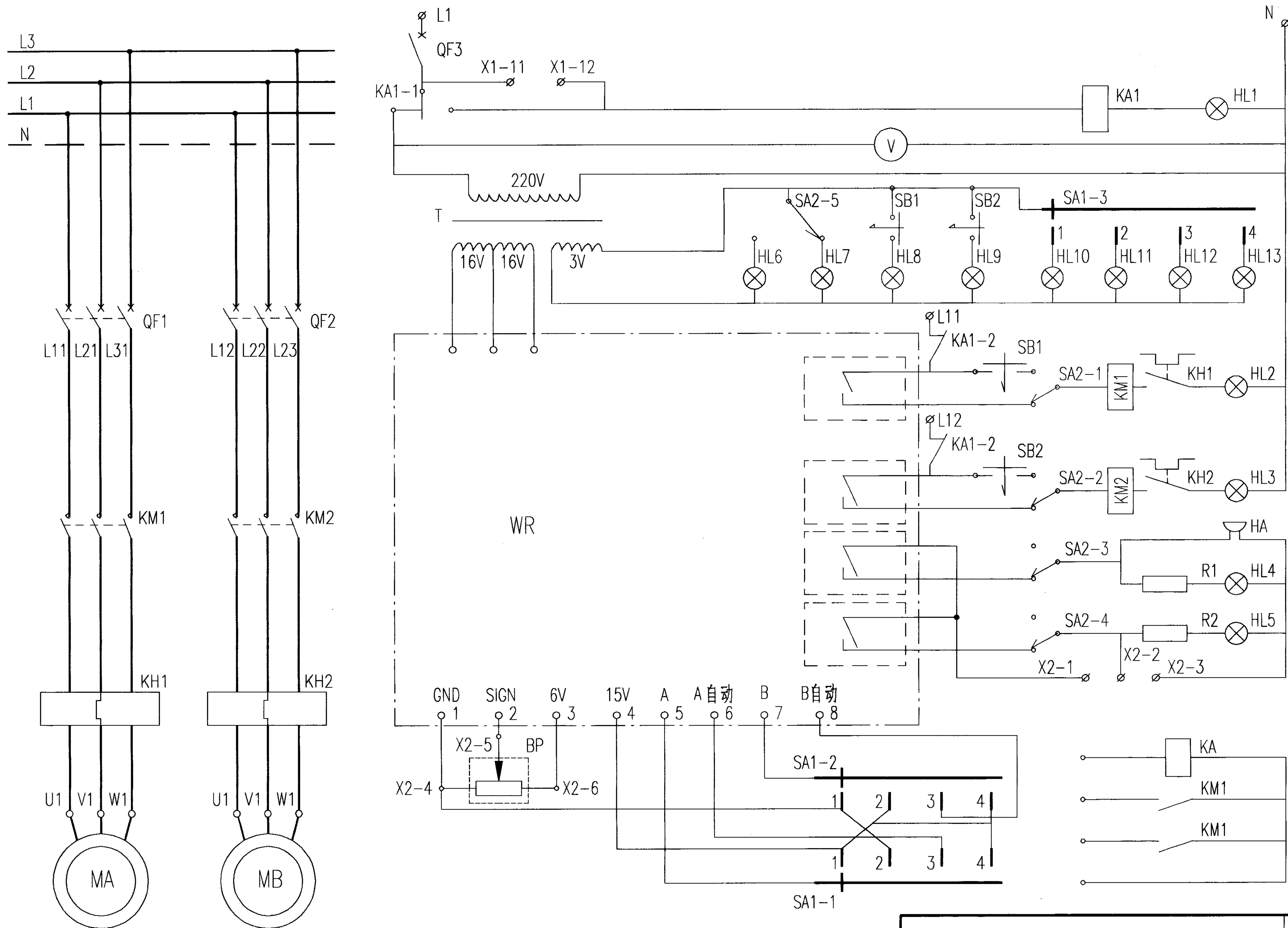
增压稳压泵自动控制电气原理图
