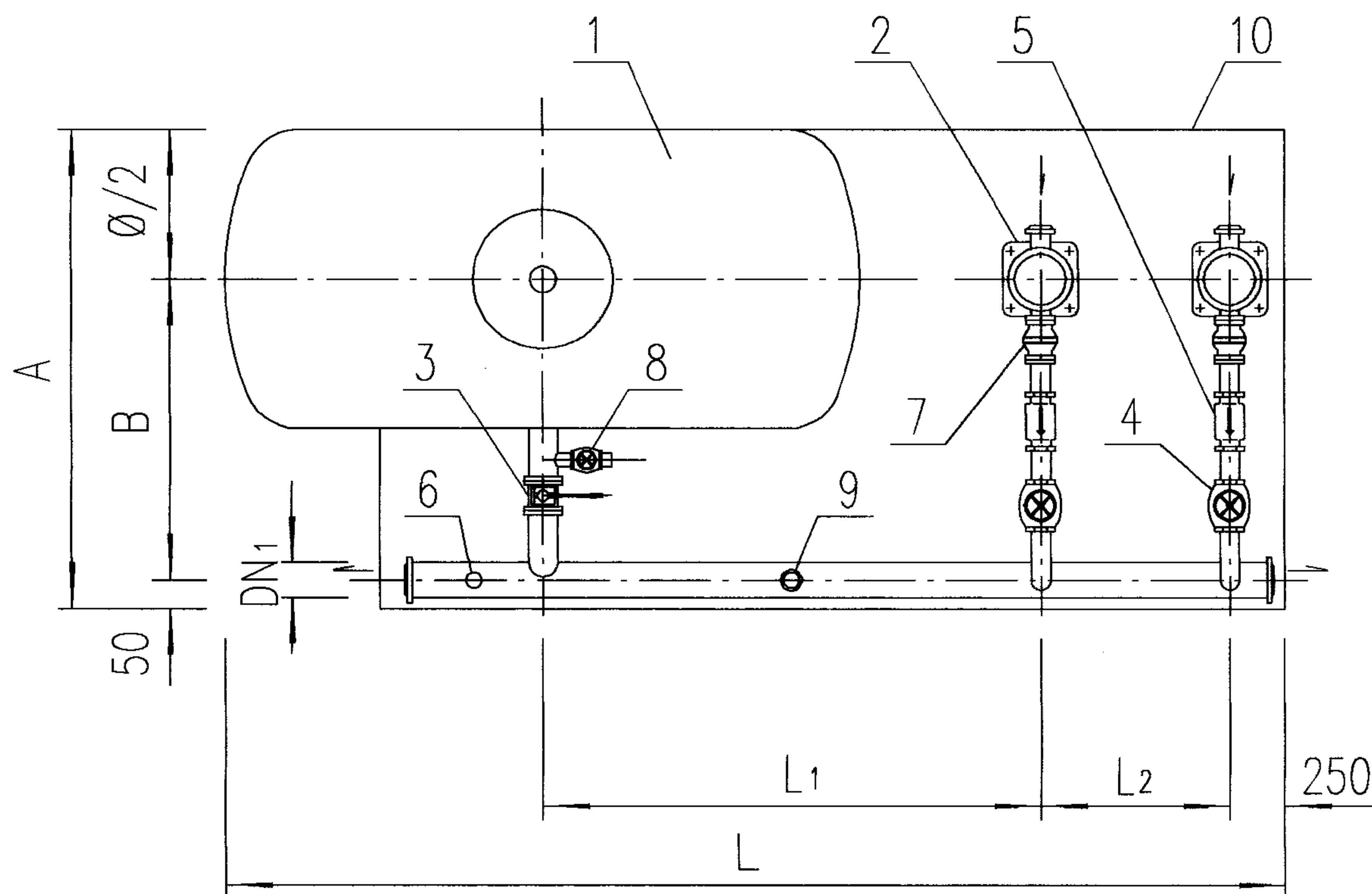
平面图
