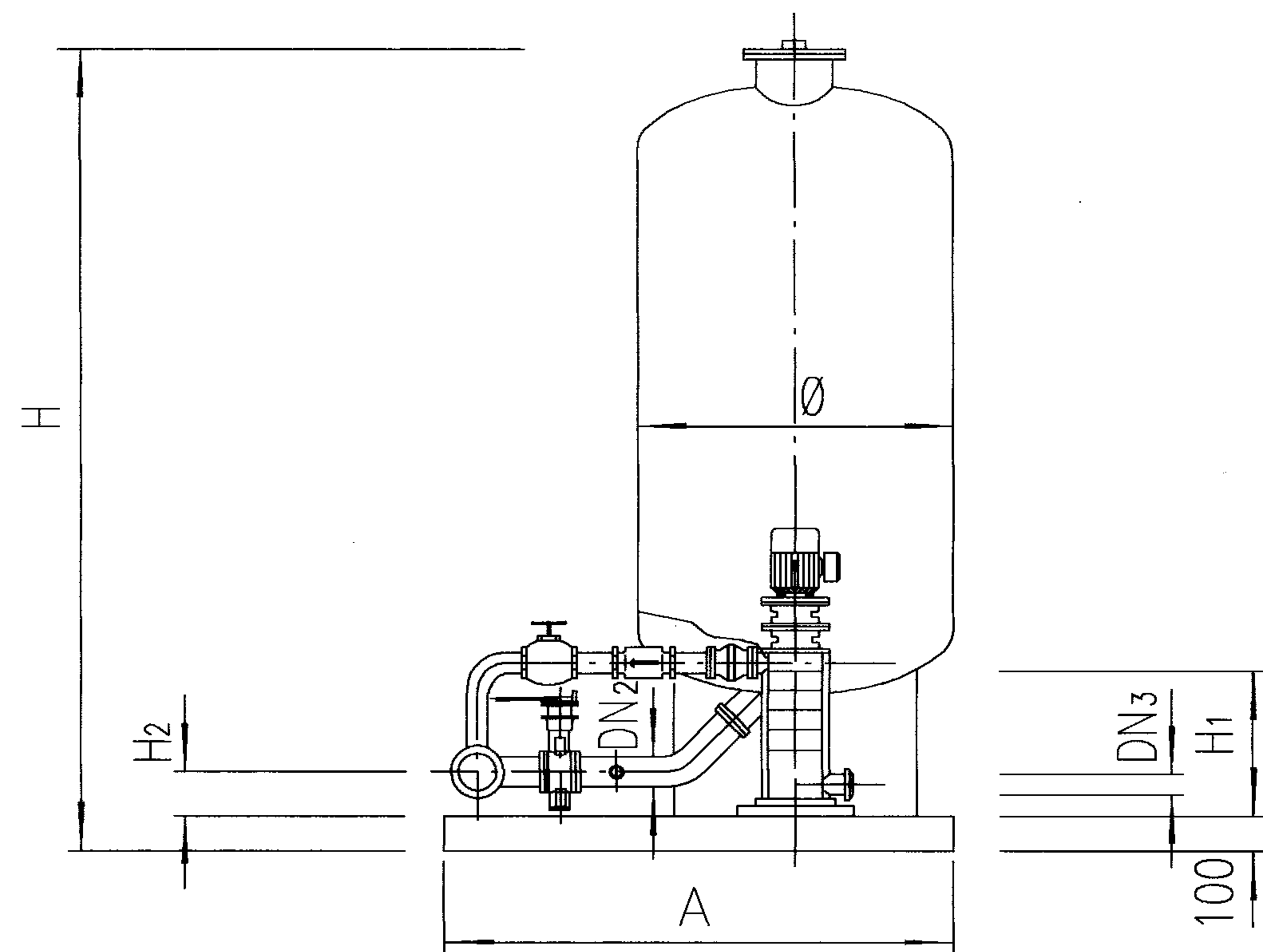
右立视图
