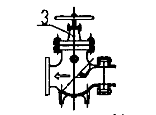
SQS-E 型阀组
