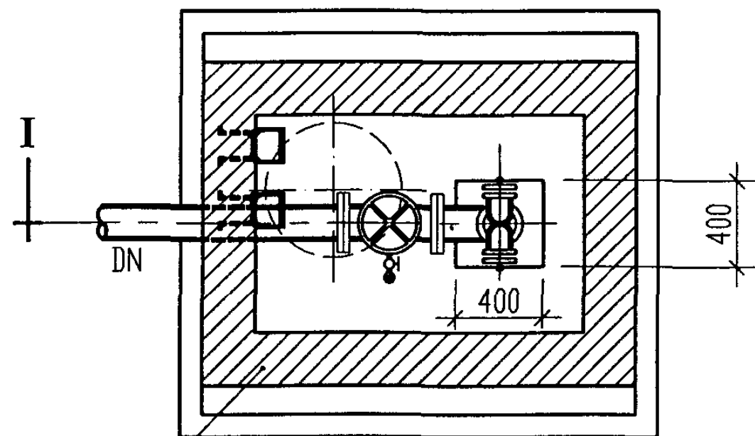
II-II 平面图
