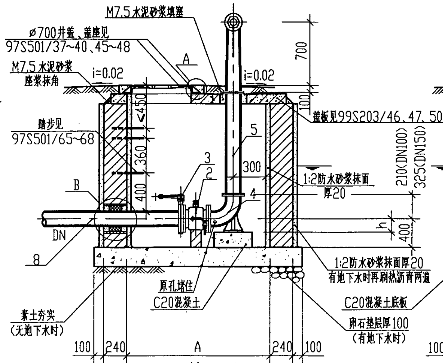
I-I 剖面图
