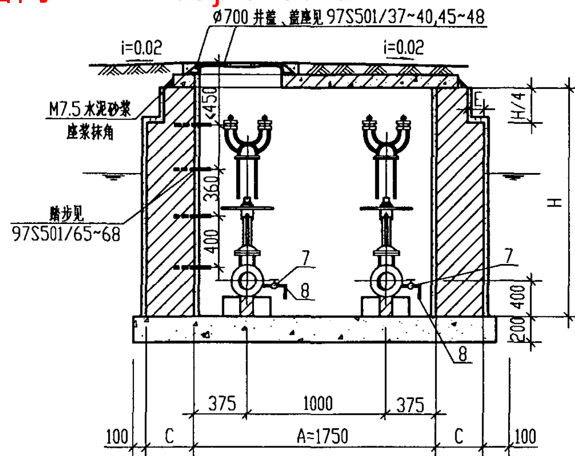
I—I 剖面图
