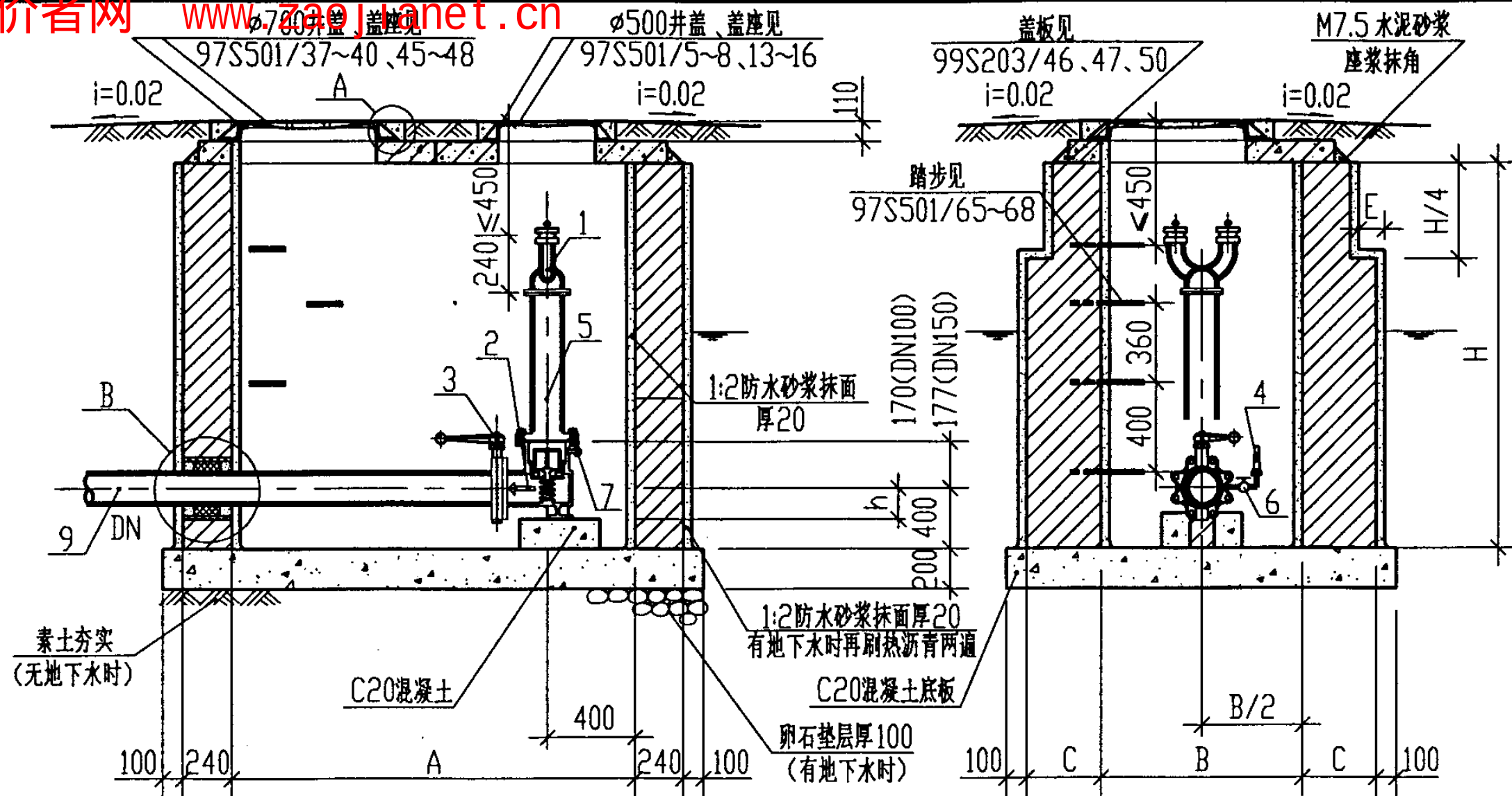
I-I 剖面图
