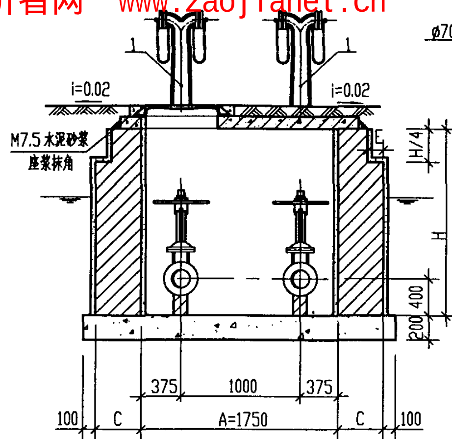
I-I 剖面图
