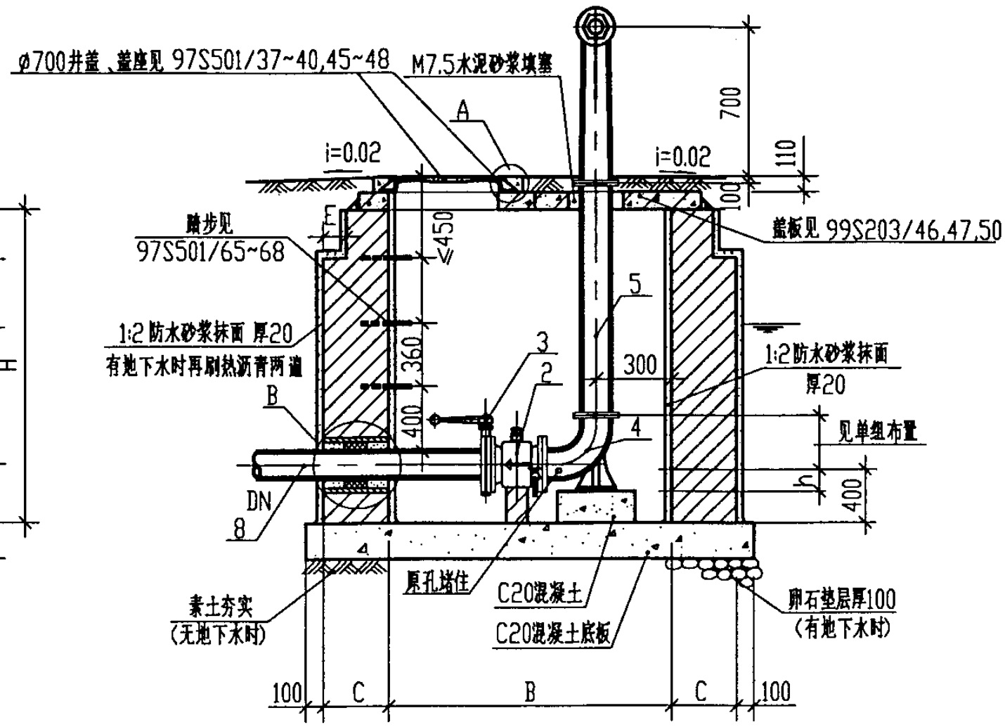
II-II 剖面图
