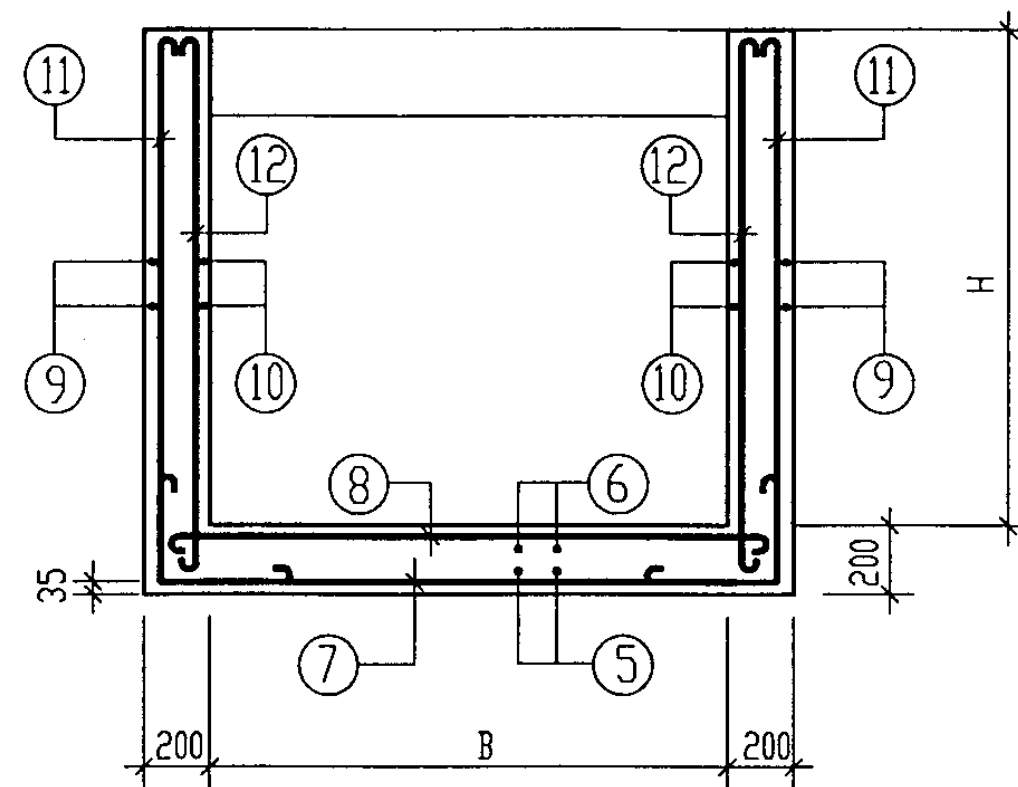
II-II 剖面图
