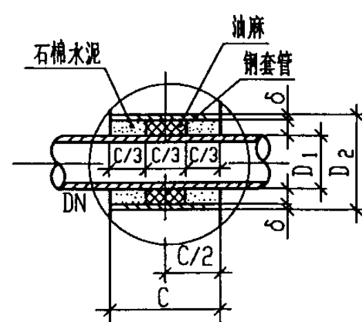
节点 B
