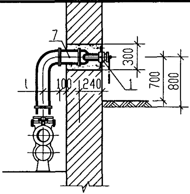
I-I 剖面图
