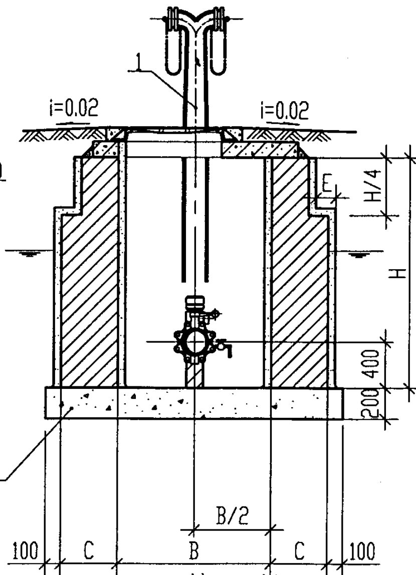
II-II 剖面图
