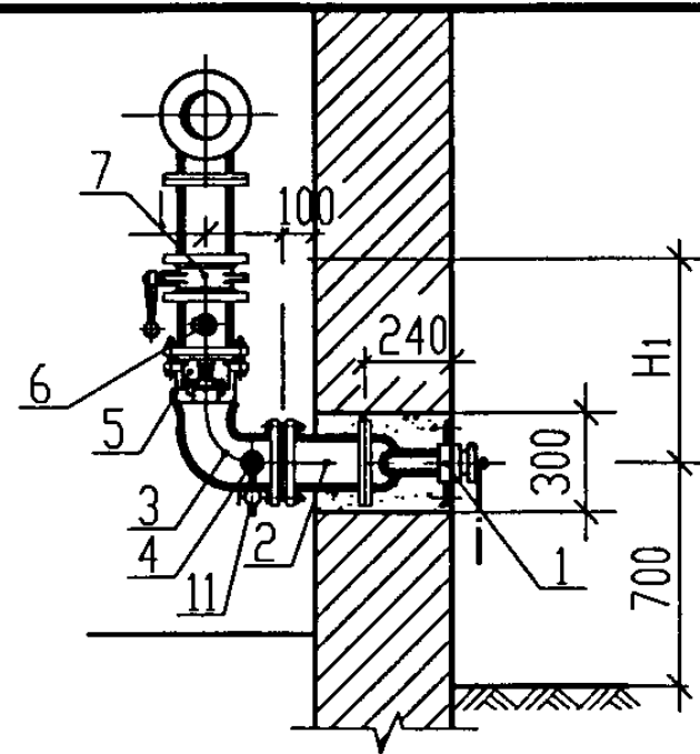
II-II剖面图
