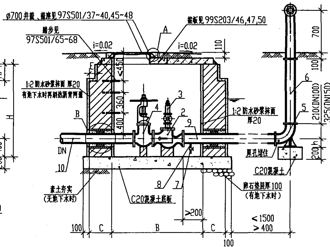
II-II 剖面图
