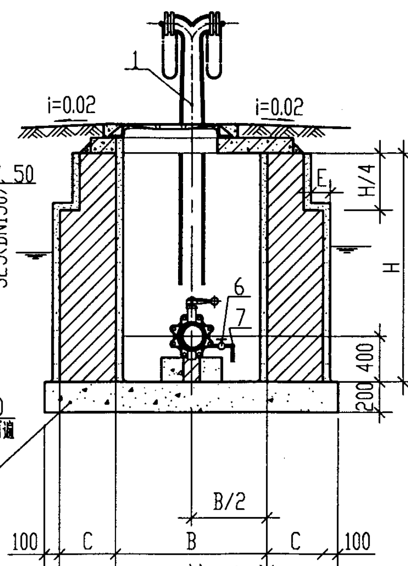
II-II 剖面图
