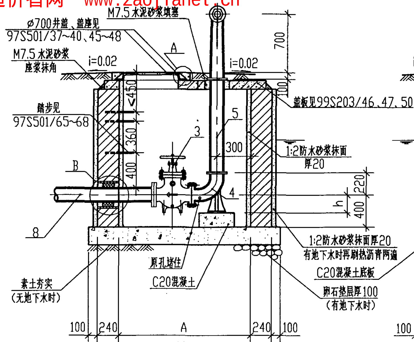
I-I 剖面图
