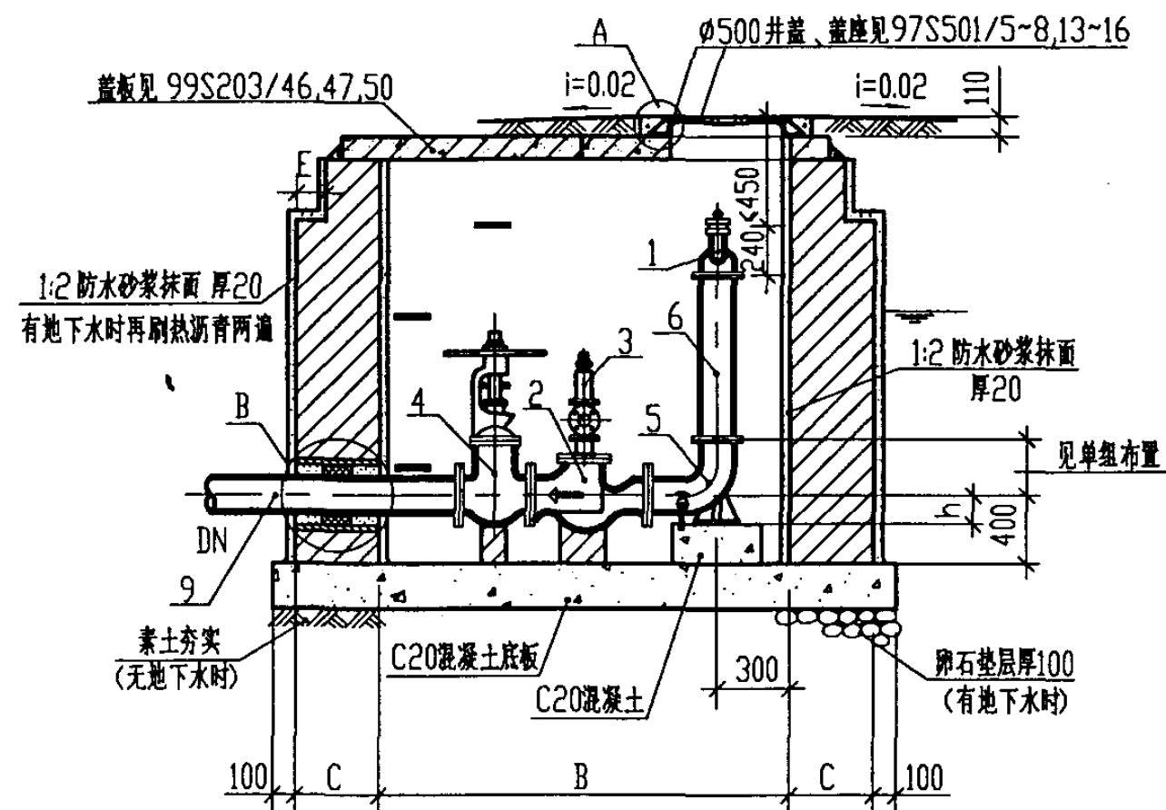
II-II 剖面图
