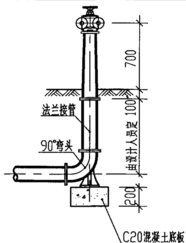
I-I 剖面图
