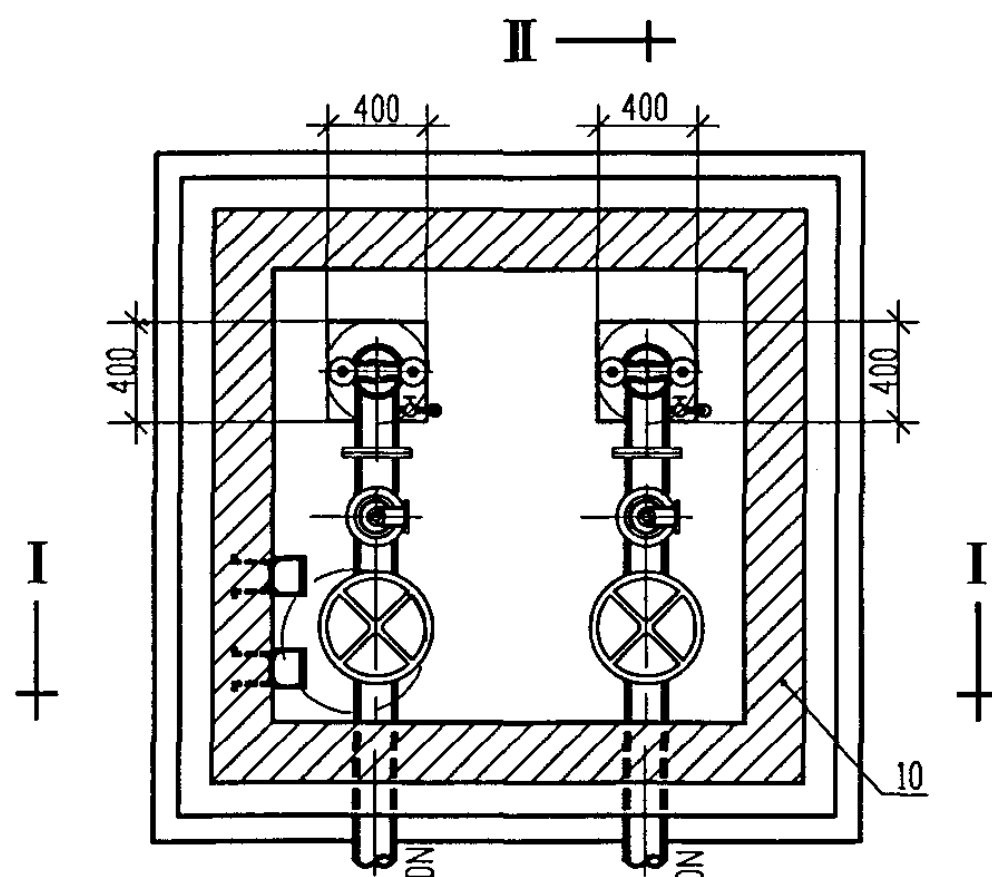
II — 平面图
