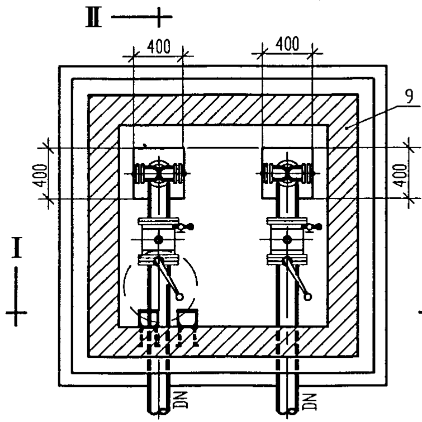
平面图
