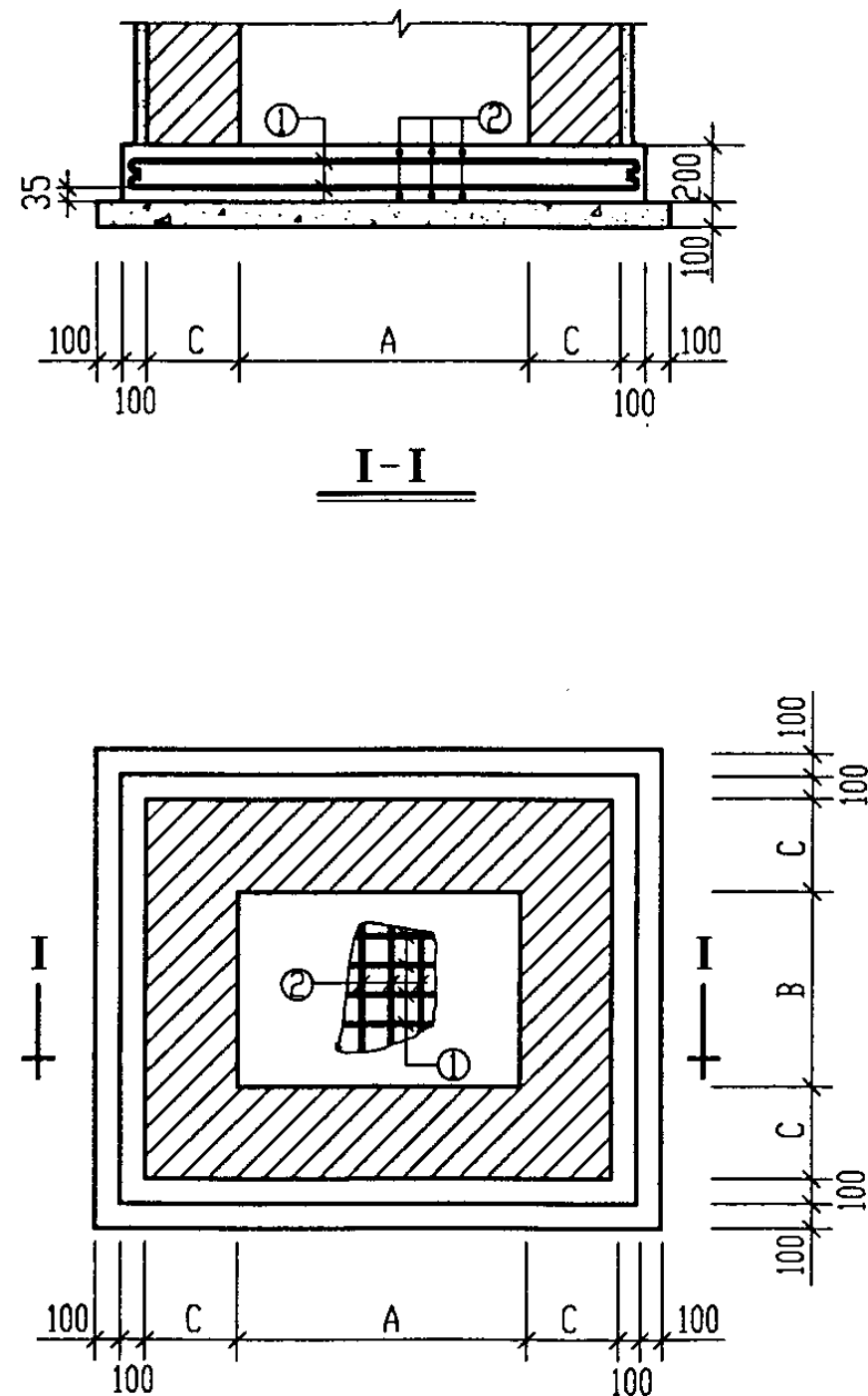
底板配筋图
