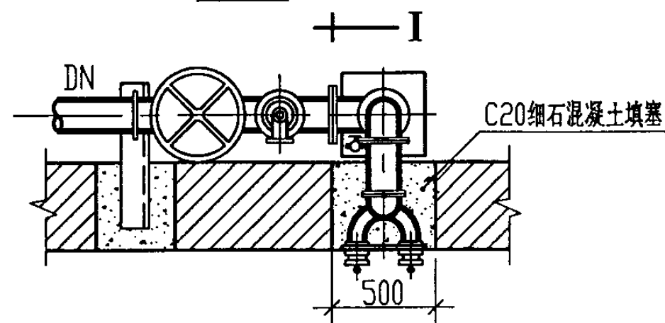
立面图
