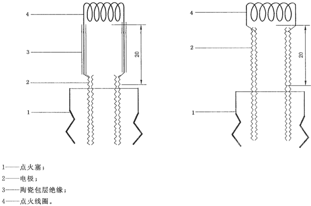
图 A.2 火花塞
