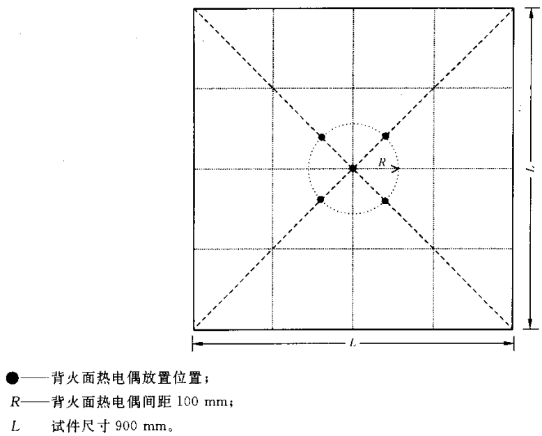
图 A.2 背火面热电偶布置图
