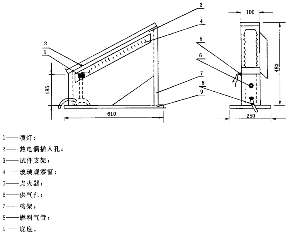
图 B.1 隧道炉
