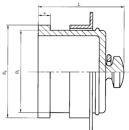
图 5 KMK 型网盖
