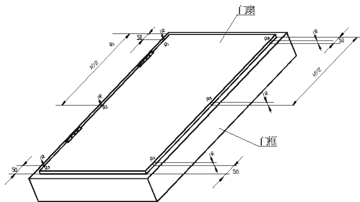
图 15 门框与门扇平面高低差测量位置示意图
