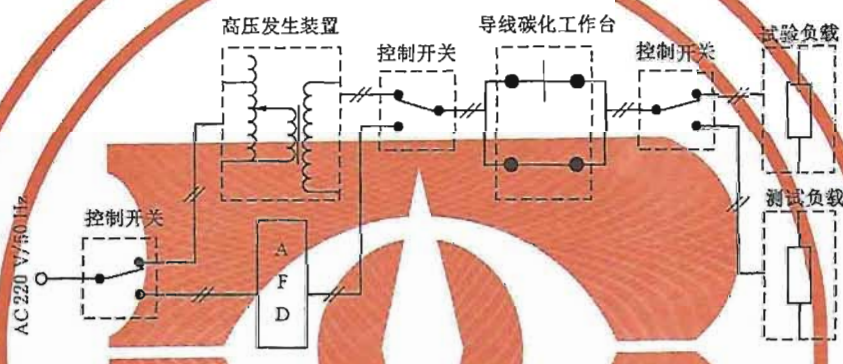
图 2 串联碳化路径电弧试验线路示意图
