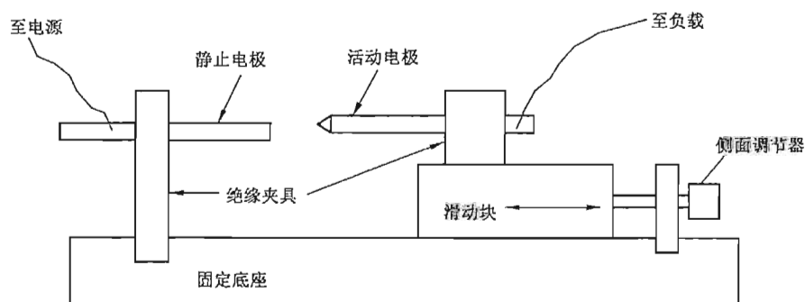
图 11 电弧发生装置
