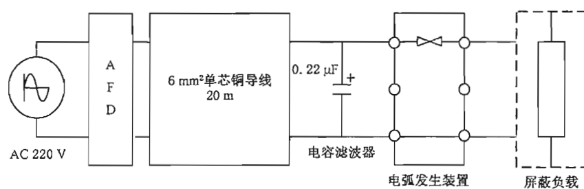
图 9 电容滤波器抑制试验
