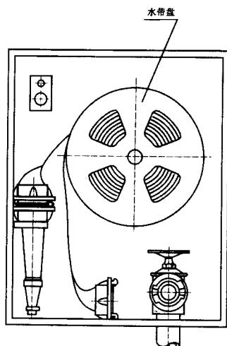
图 2 盘卷式栓箱
