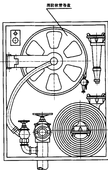
图 3 卷置式栓箱(配置消防软管卷盘)
