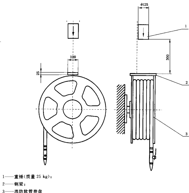
图 6 消防软管卷盘的抗冲击性能试验
