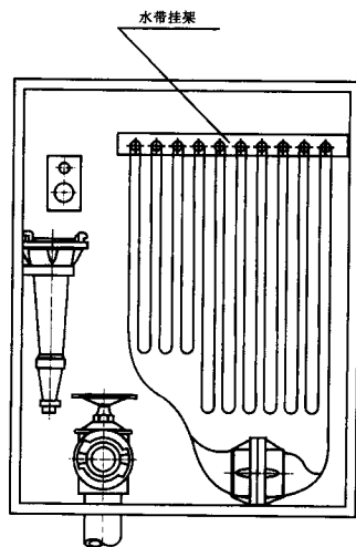
图 1 挂置式栓箱
