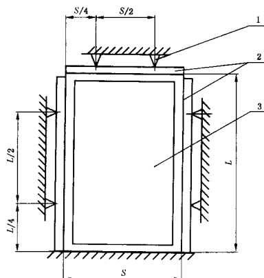
图 5 刚度试验台
