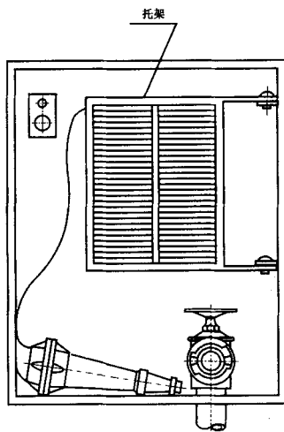
图 4 托架式栓箱
