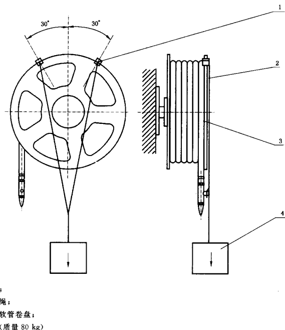
图7 消防软管卷盘的负荷性能试验
