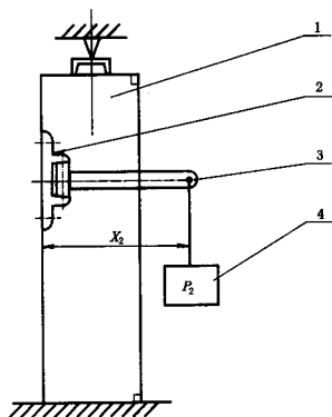
图 9 托架式栓箱的刚度试验
