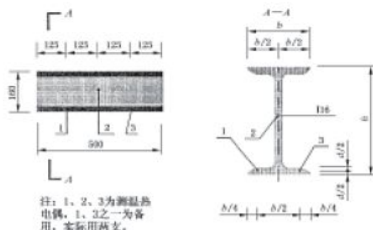
图 1 附加耐火试验热电偶埋设图(单位:mm)
