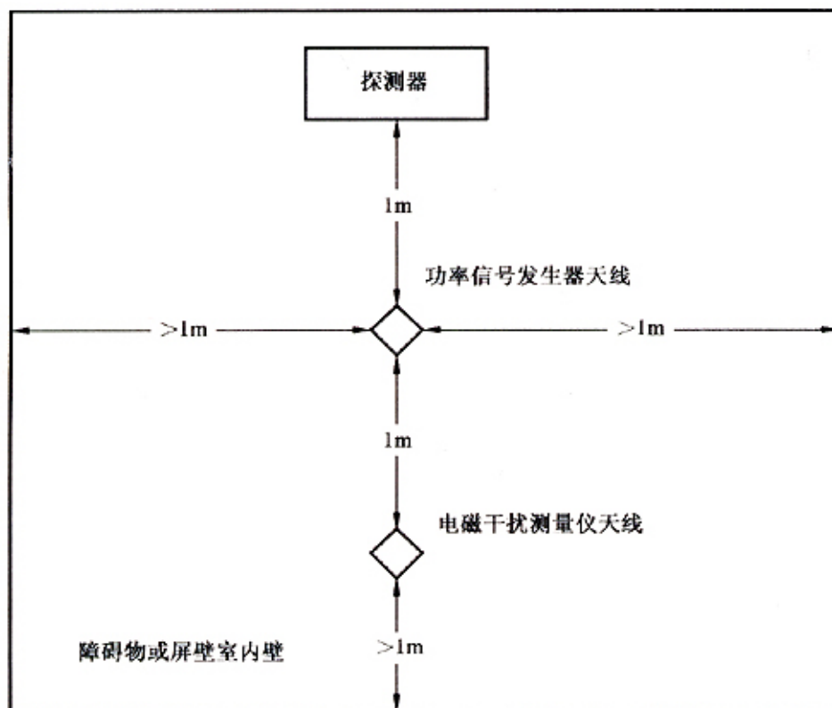
图 2 天线位置图
