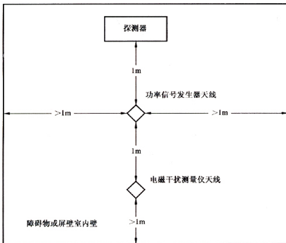
图 2 天线位置图
