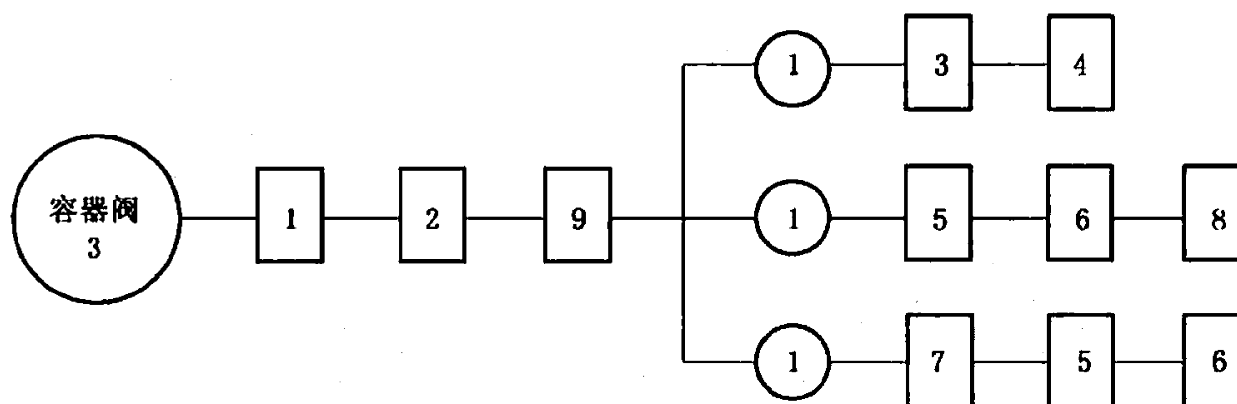
图 F.1 容器阀试验程序图
