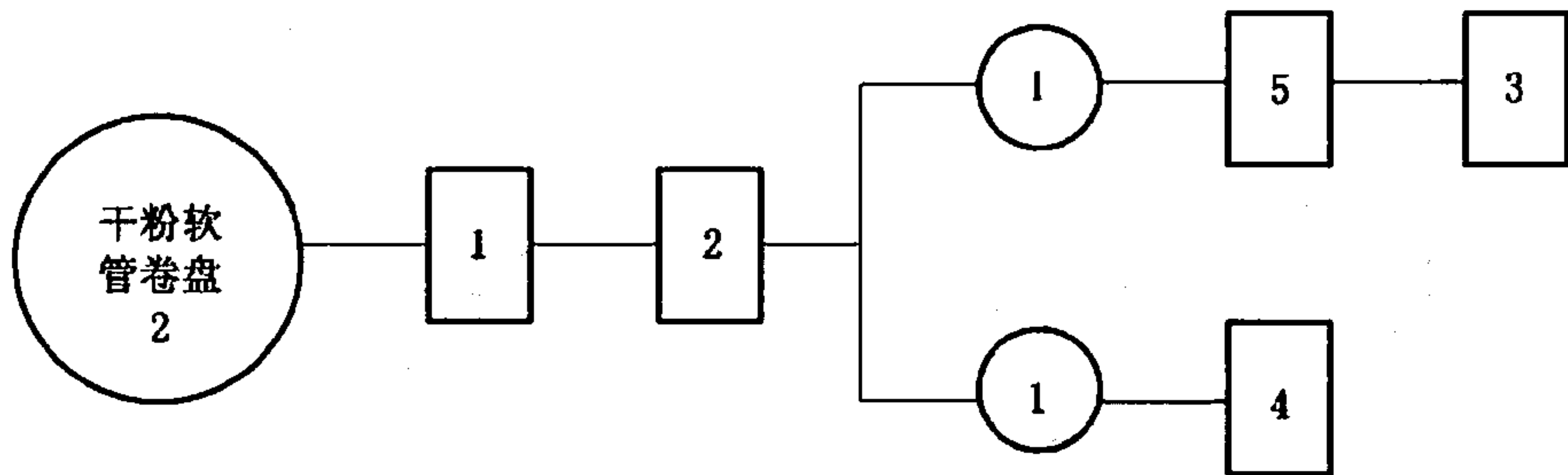
图 T.1 干粉软管卷盘试验程序图
