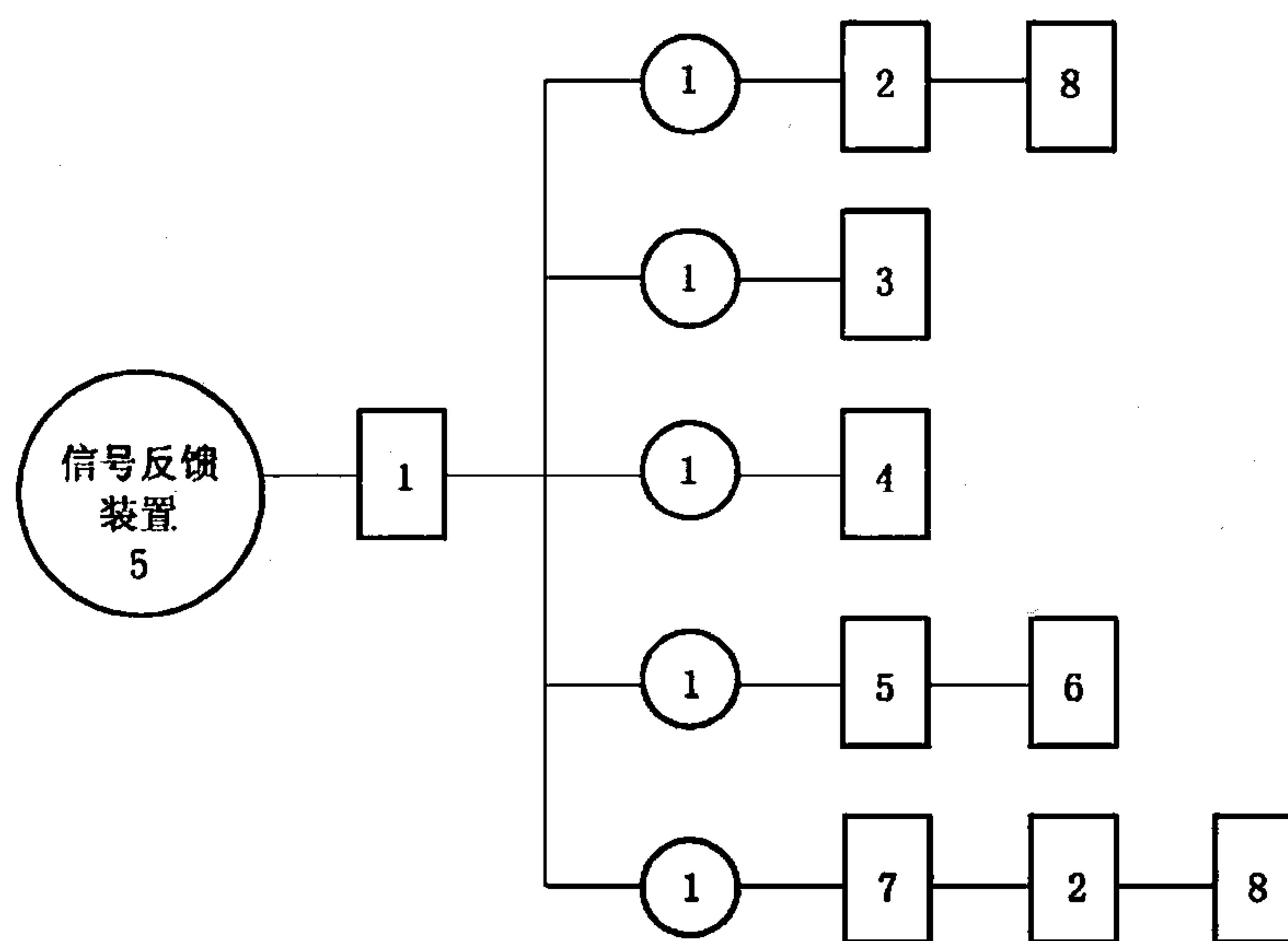
图 Q.1 信号反馈装置试验程序图
