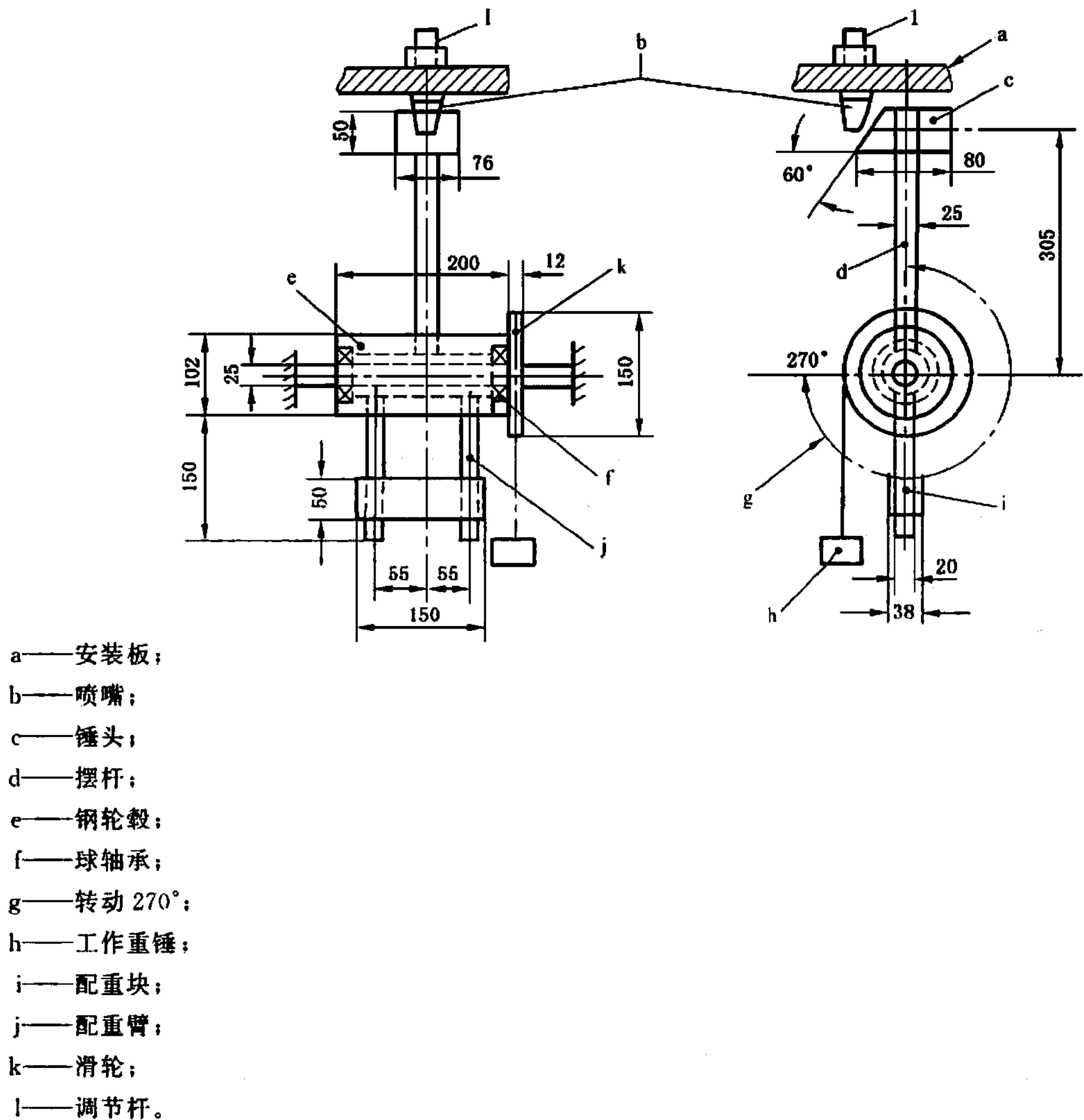
图 3 喷嘴耐冲击试验装置
