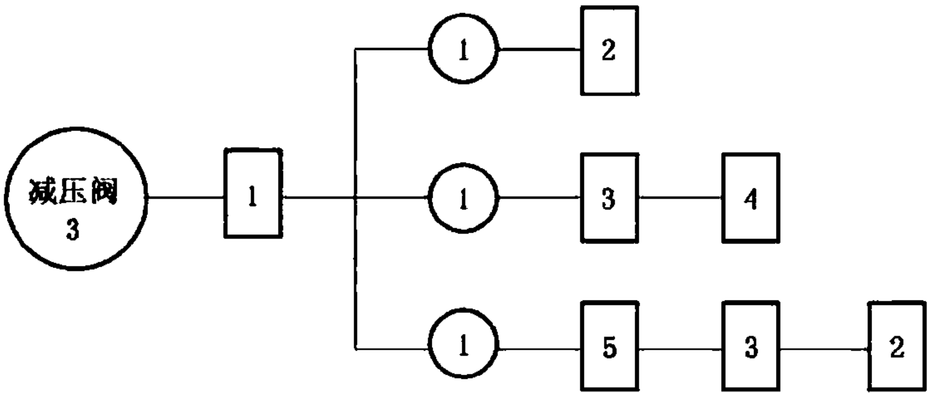
图 R. 1 减压阀试验程序图
