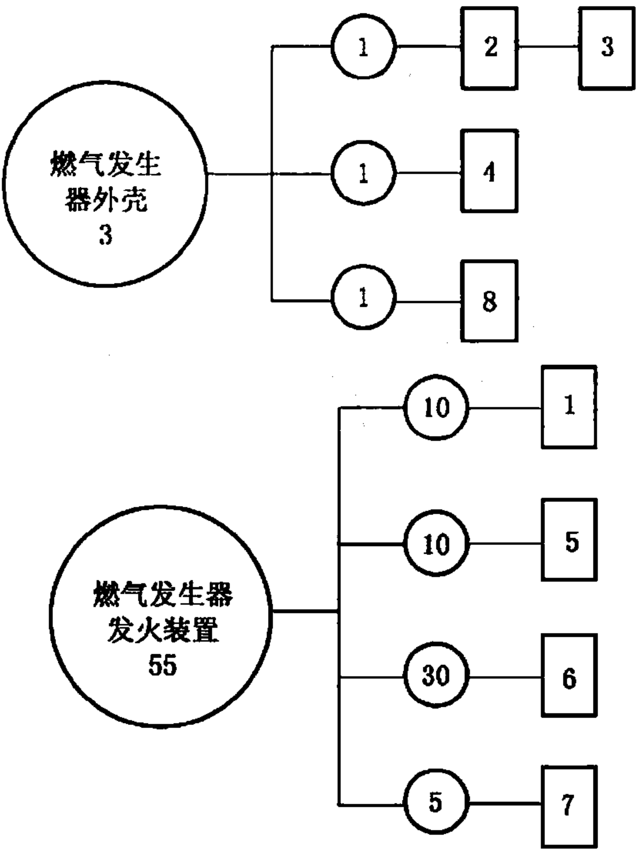
图 P.1 燃气发生器试验程序图
