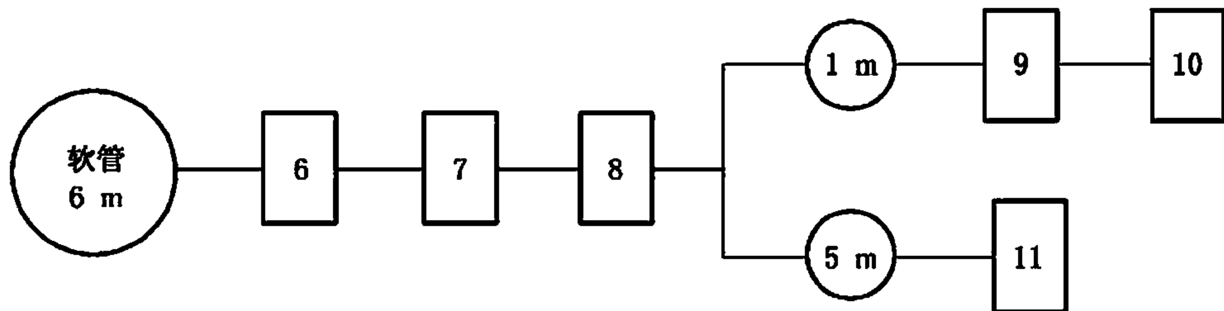
图 T.2 软管试验程序图
