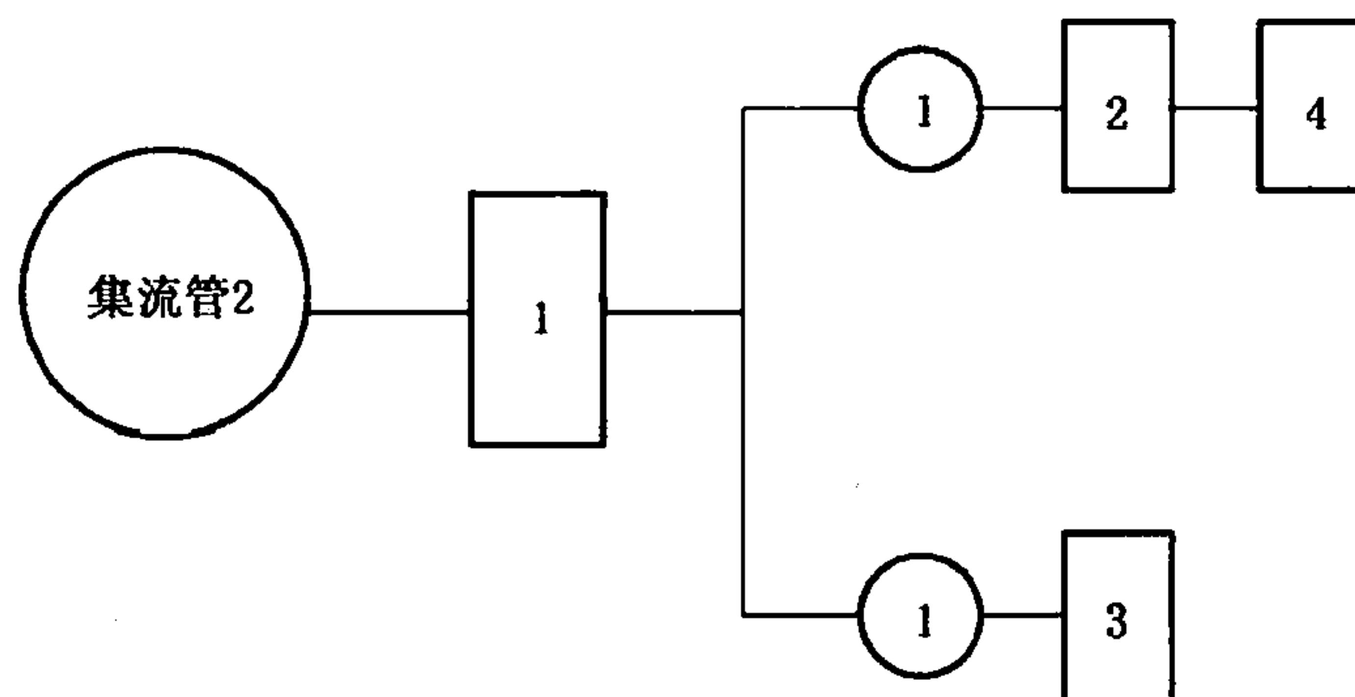
图 H.1 集流管试验程序图
