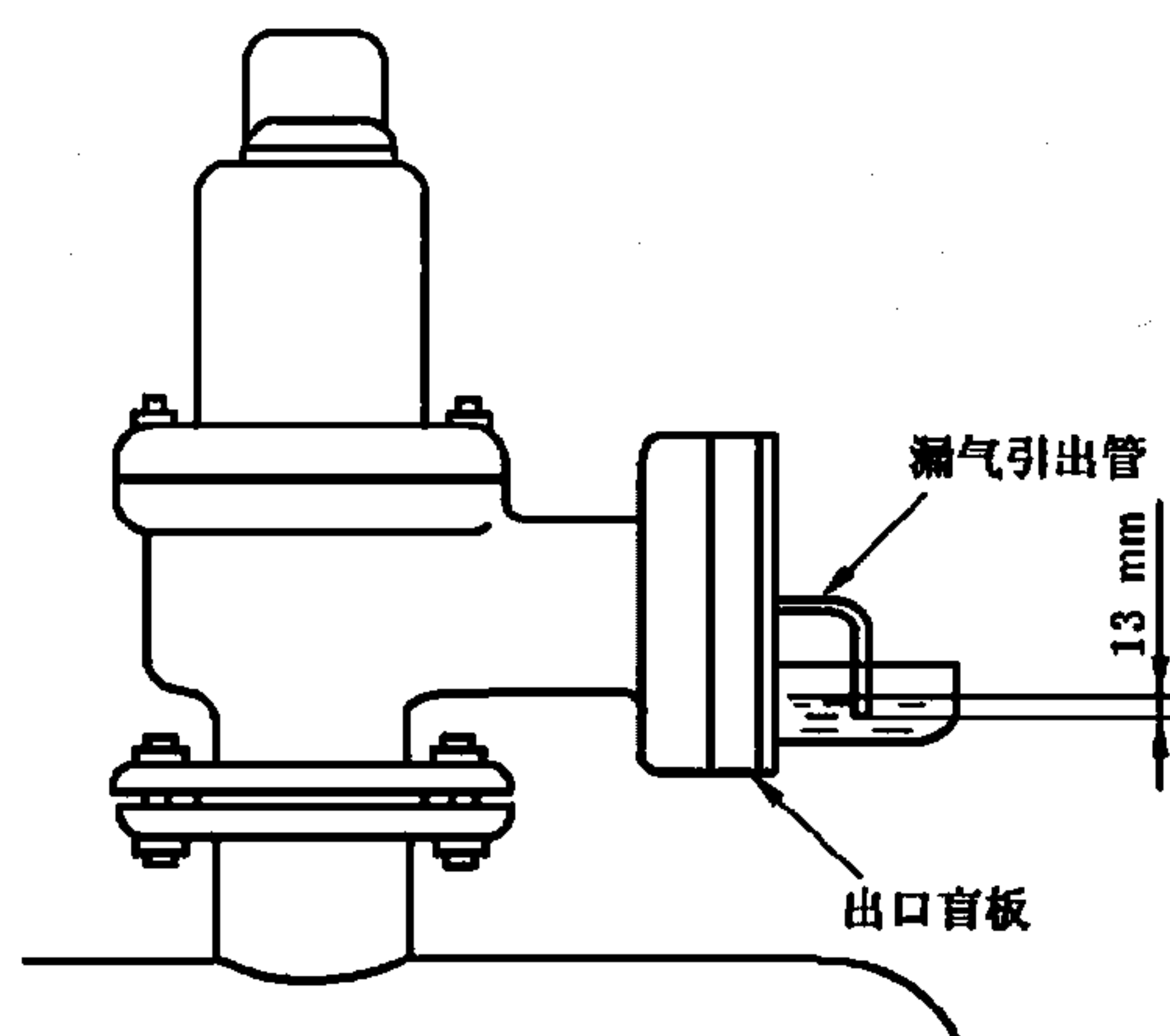
图 1 安全阀密封试验布置图
