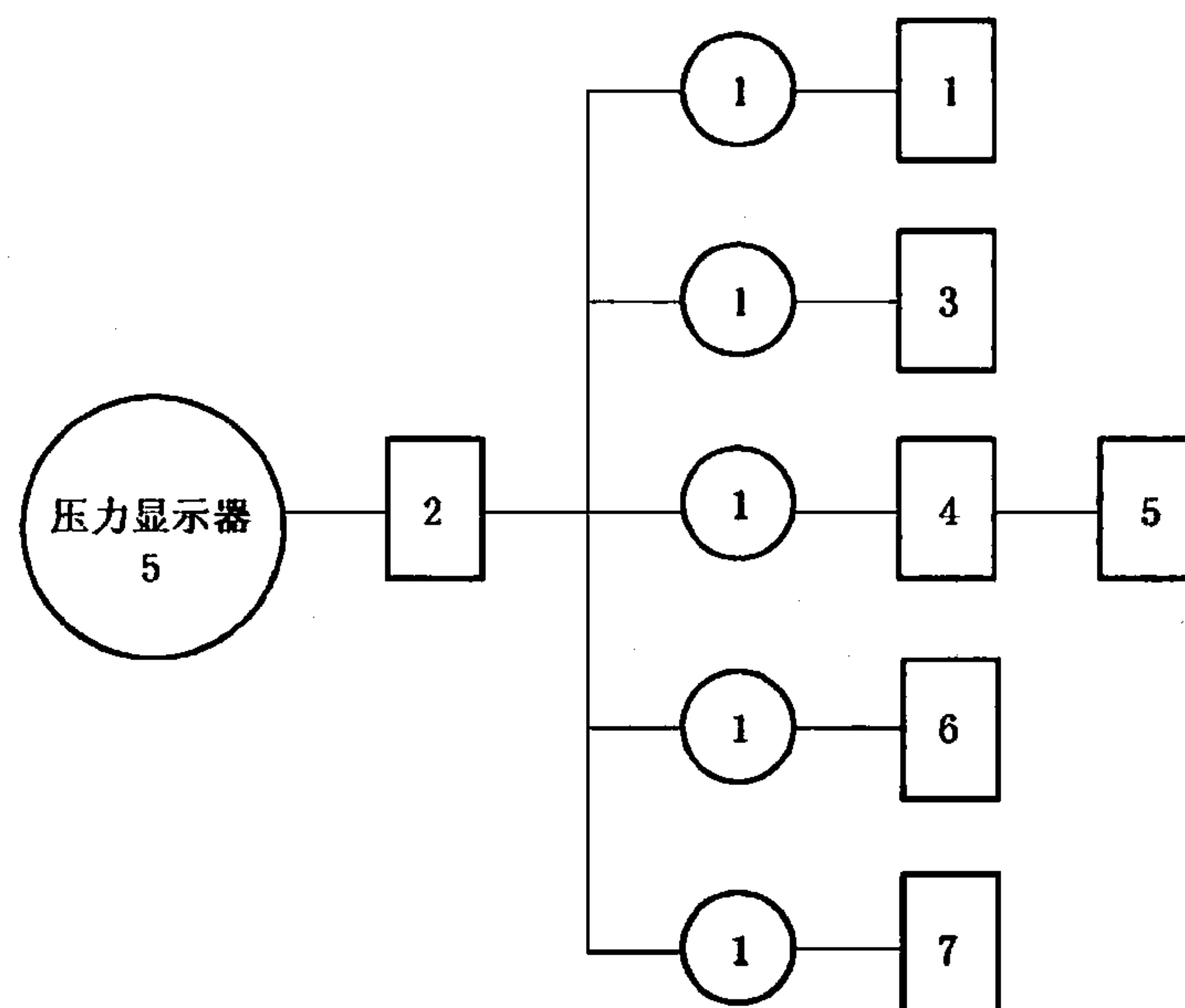
图 L.1 压力显示器试验程序图
