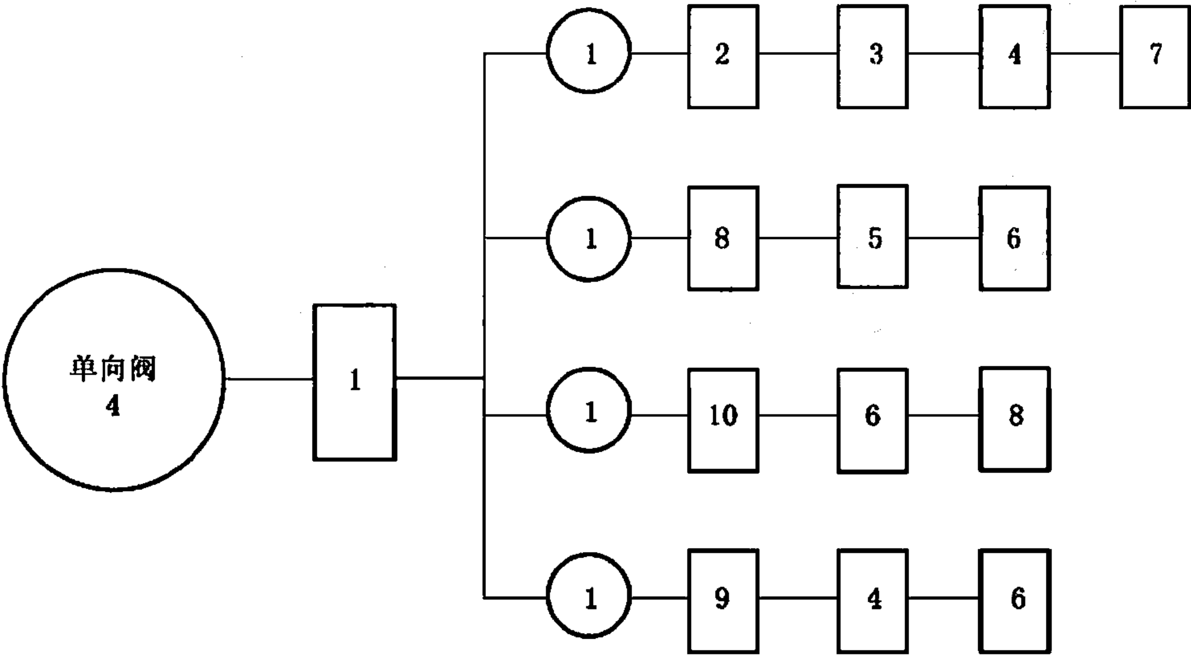
图 G.1 单向阀试验程序图
