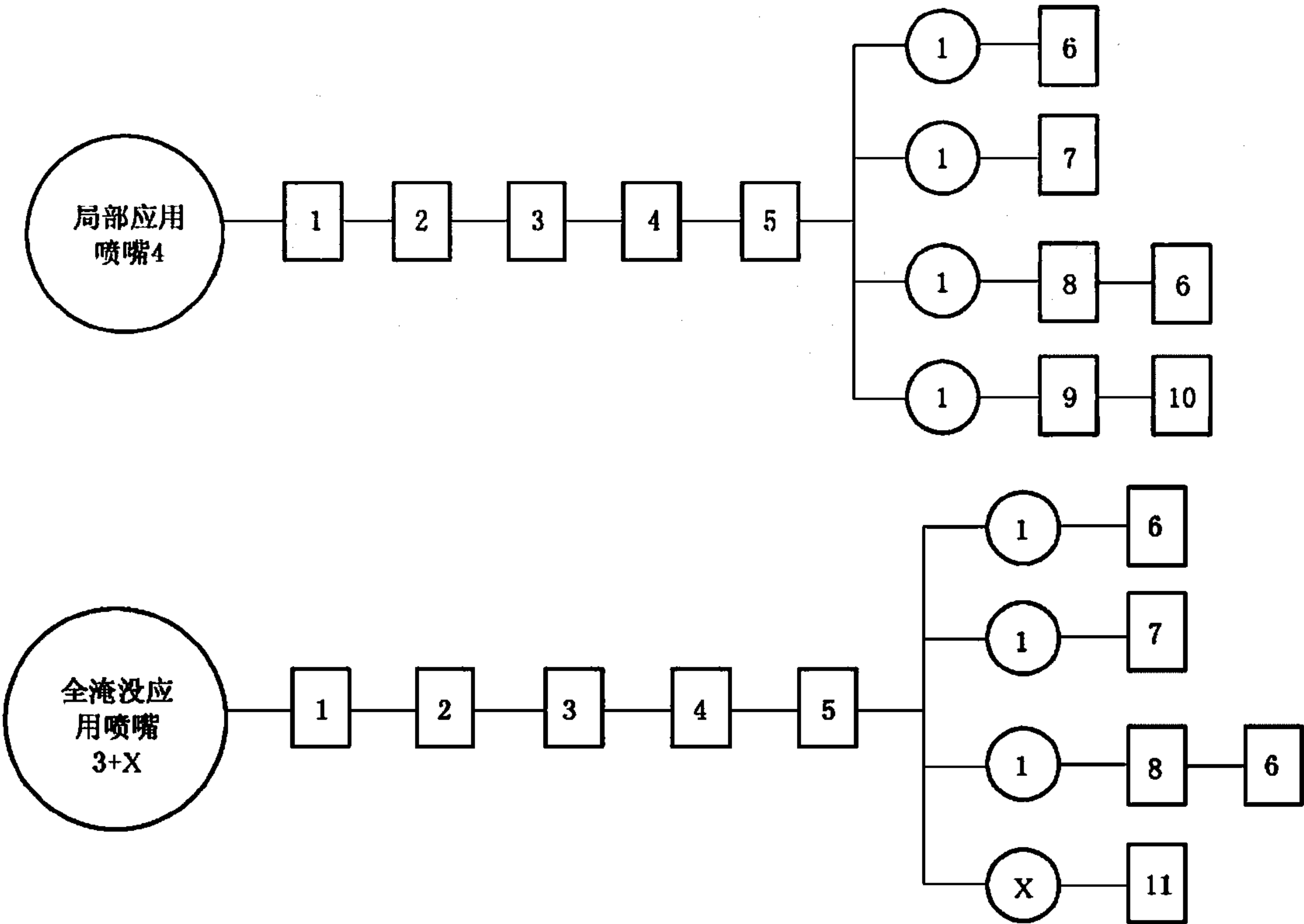
图 S.1 喷嘴试验程序图
