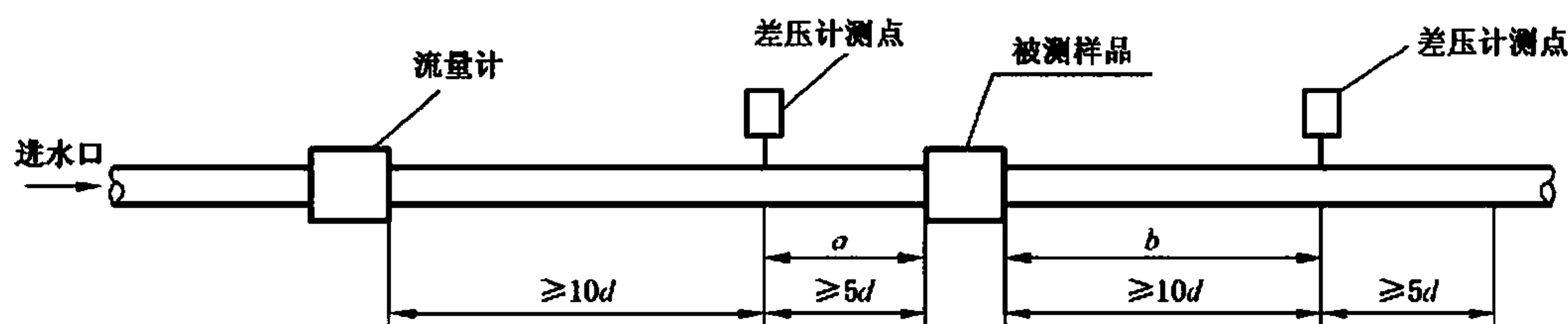
图 2 等效长度试验装置
