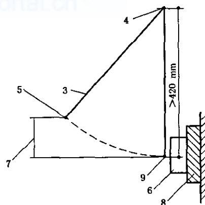
b) 试验装置原理
