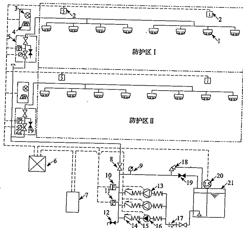
图1 开式系统示意
