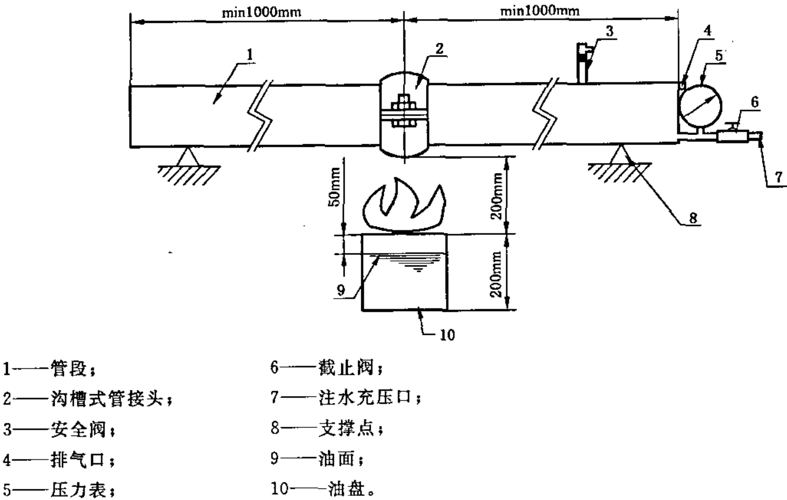
图 6 耐火试验装置图
