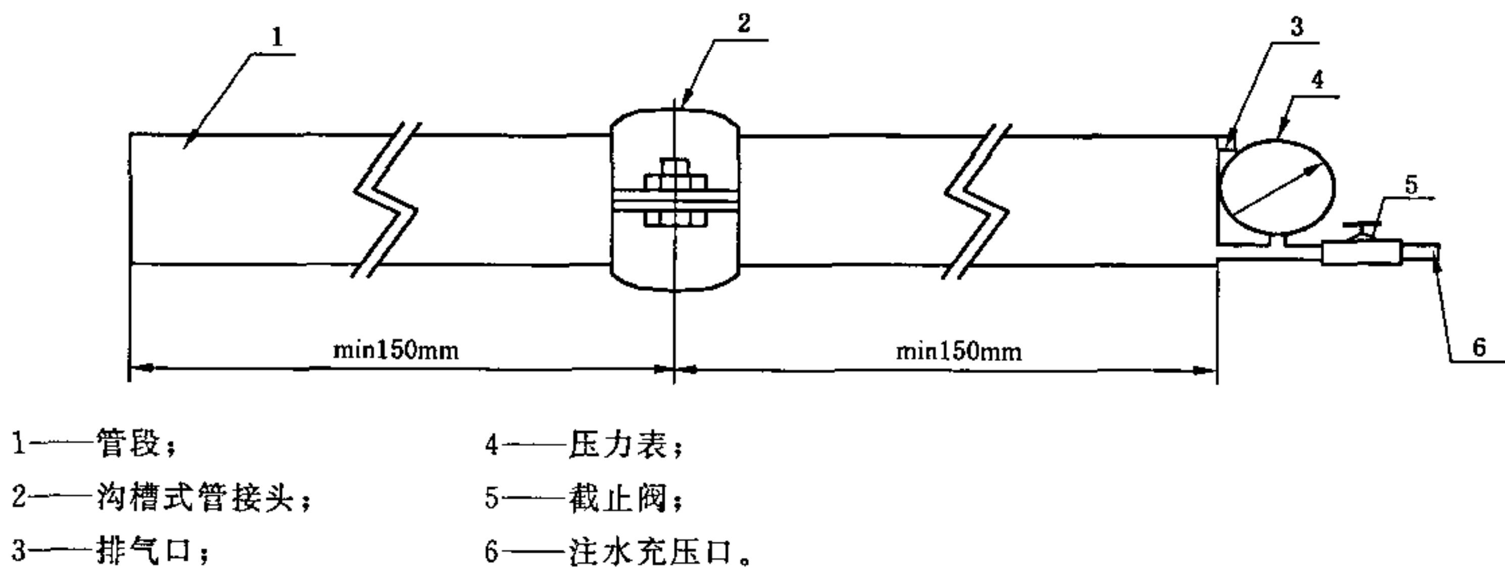
图 2 强度密封试验装置图
