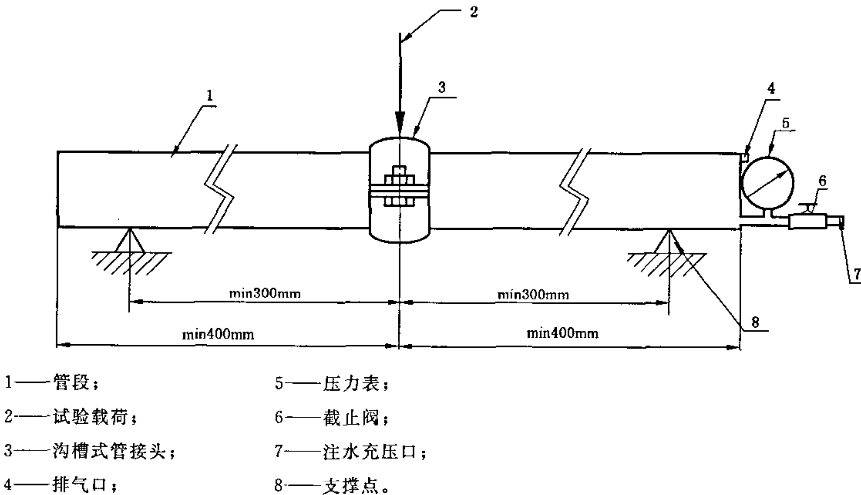
图 3 沟槽式管接头承载力矩试验装置图
