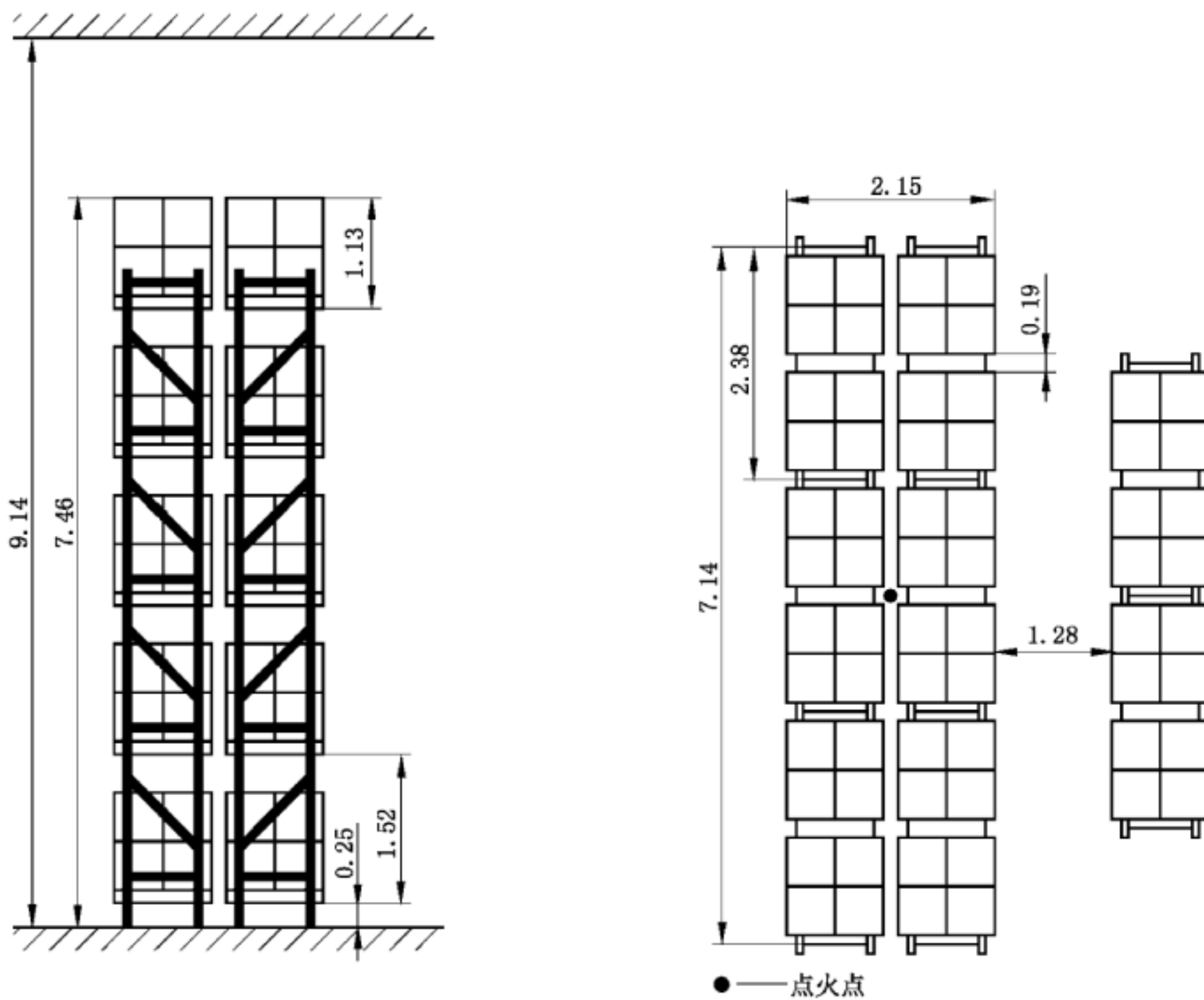
图 19 K 242 直立型 ESFR 喷头灭火试验布置 试验 C
