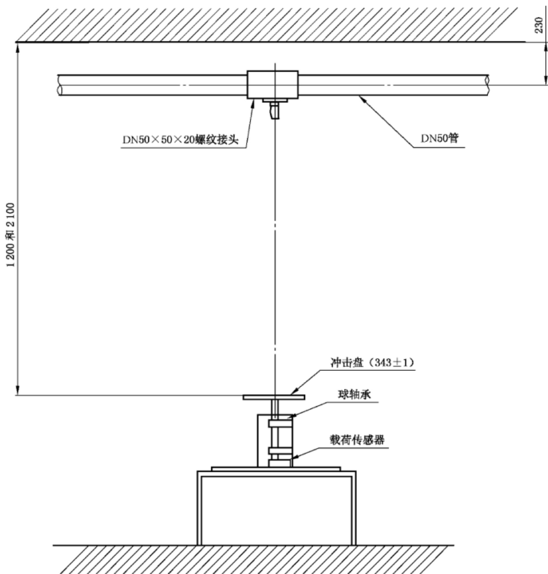
图 11 冲力试验装置
