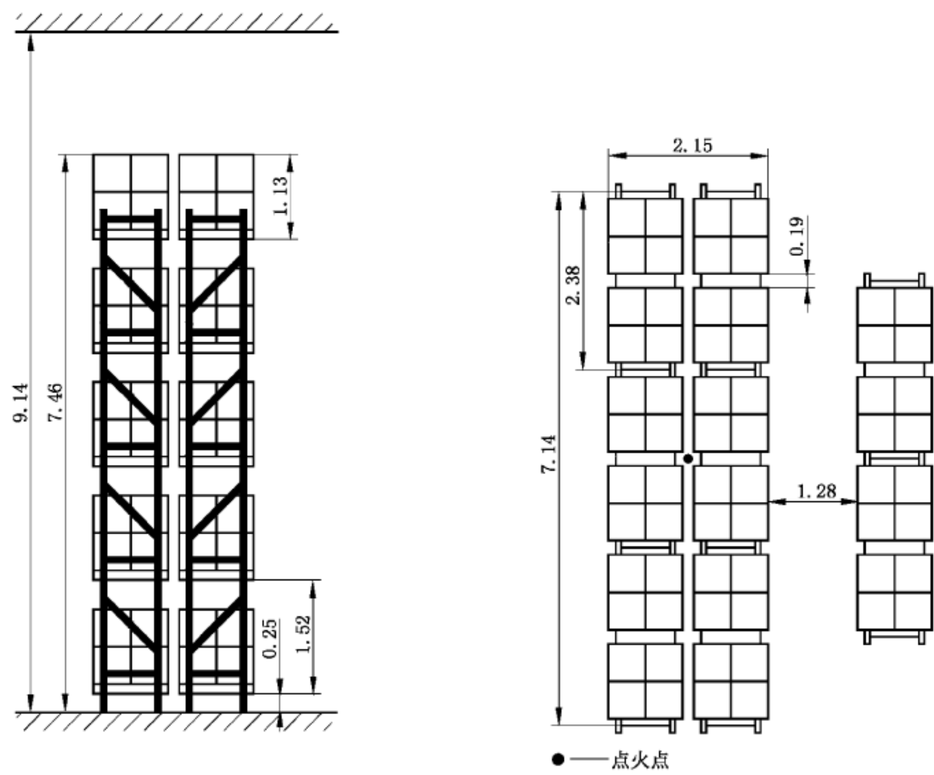
图 18 K 242 直立型 ESFR 喷头灭火试验布置 试验 B
