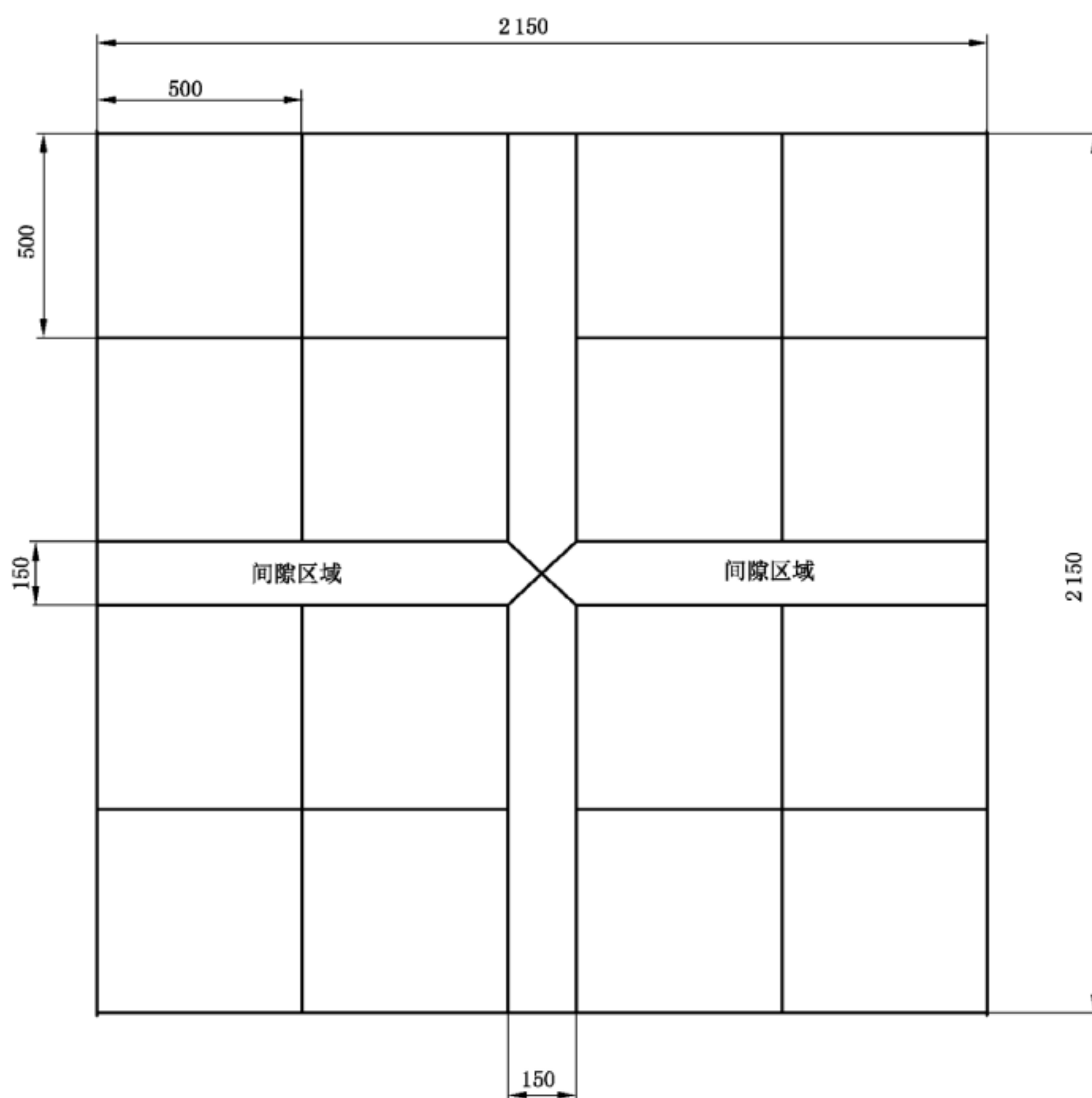
图 7 布水试验装置中集水盒的布置
