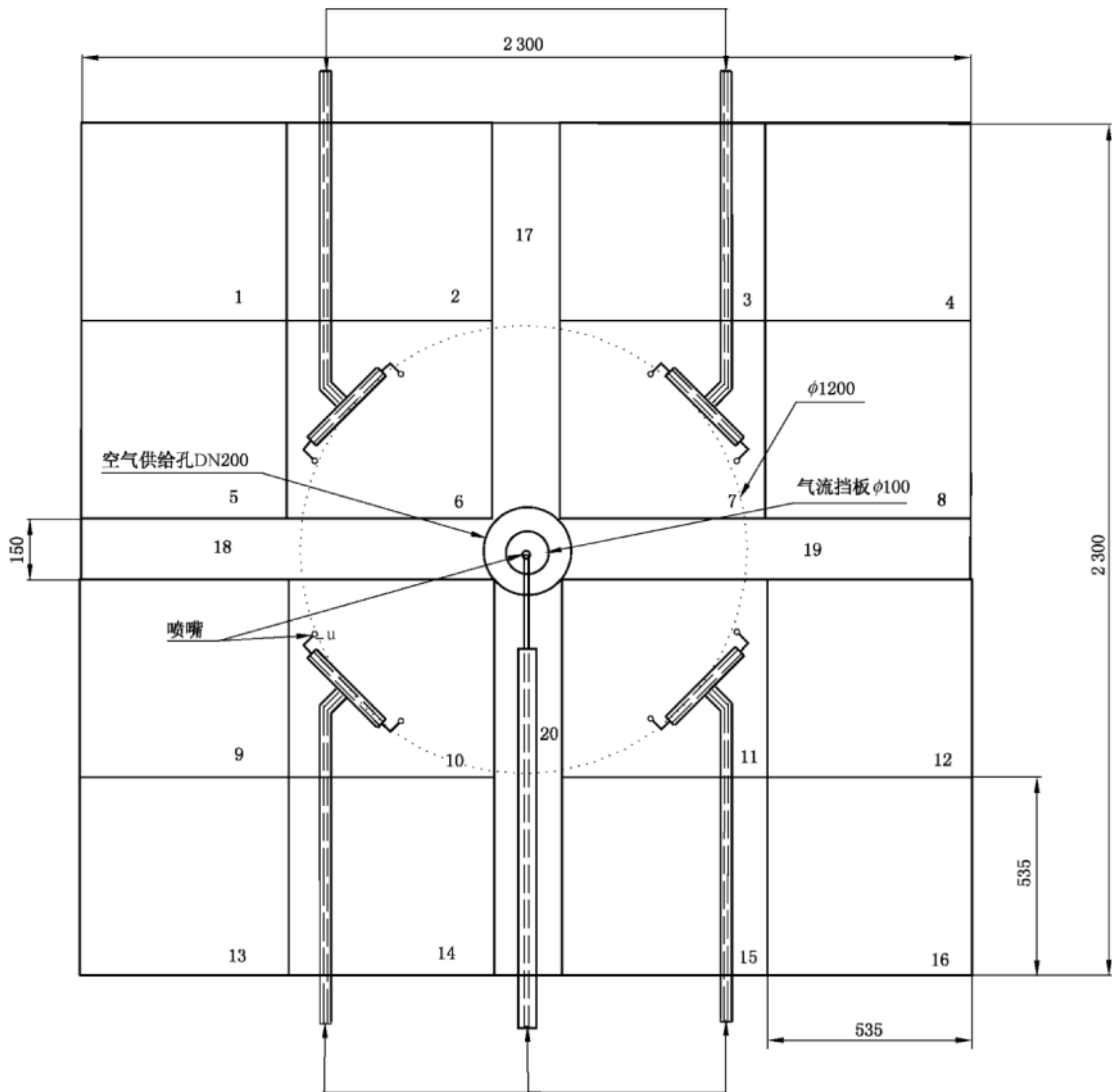
图 10 实际洒水密度(ADD)试验装置
