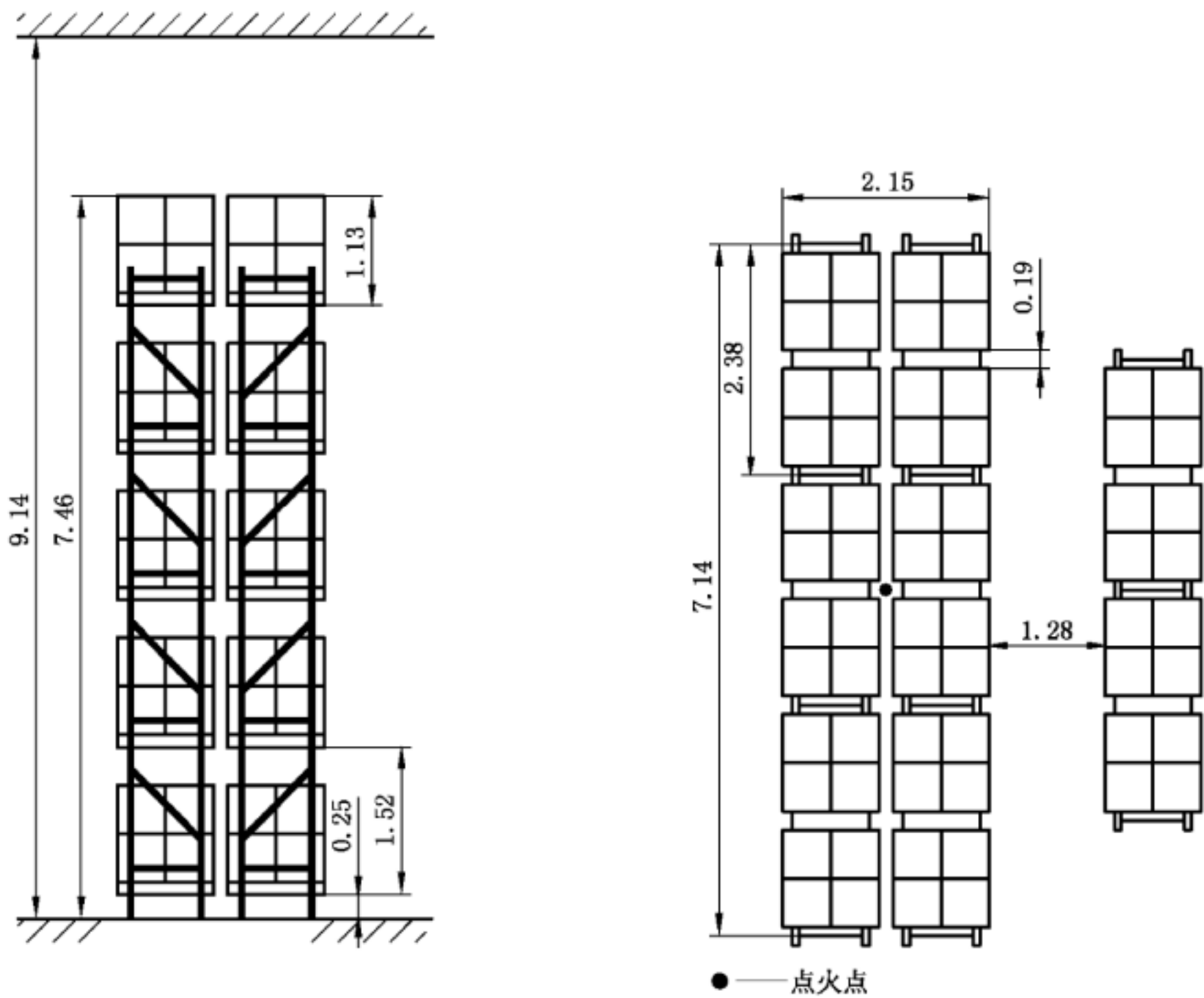
图 13 K 202 直立型 ESFR 喷头灭火试验布置 试验 B
