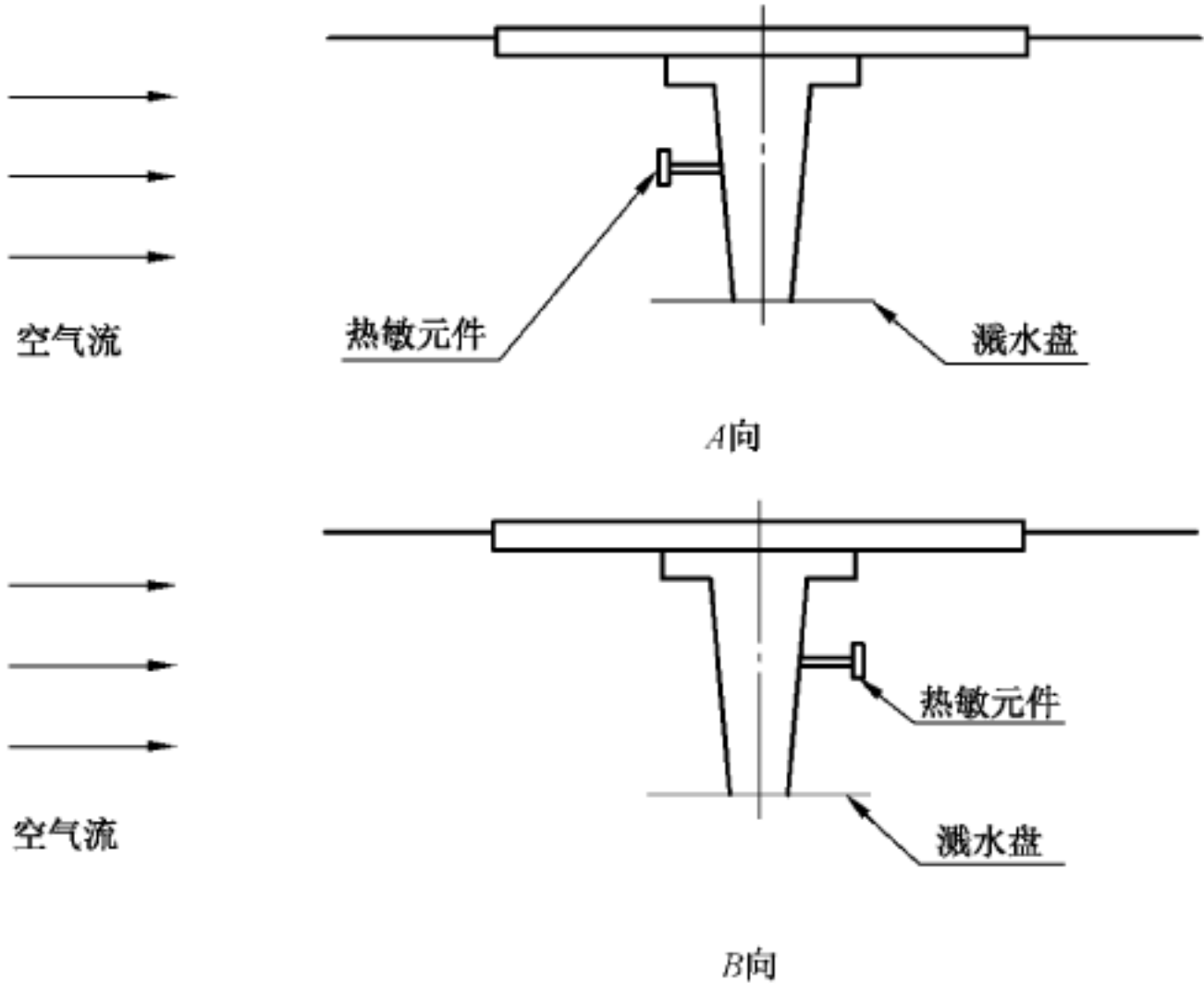
图 9 动态热试验方位
