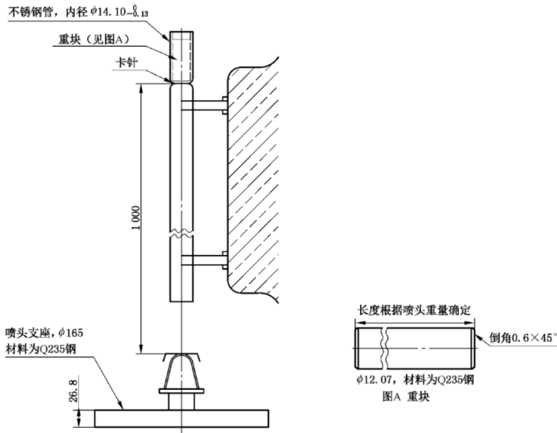
图 8 碰撞试验装置
