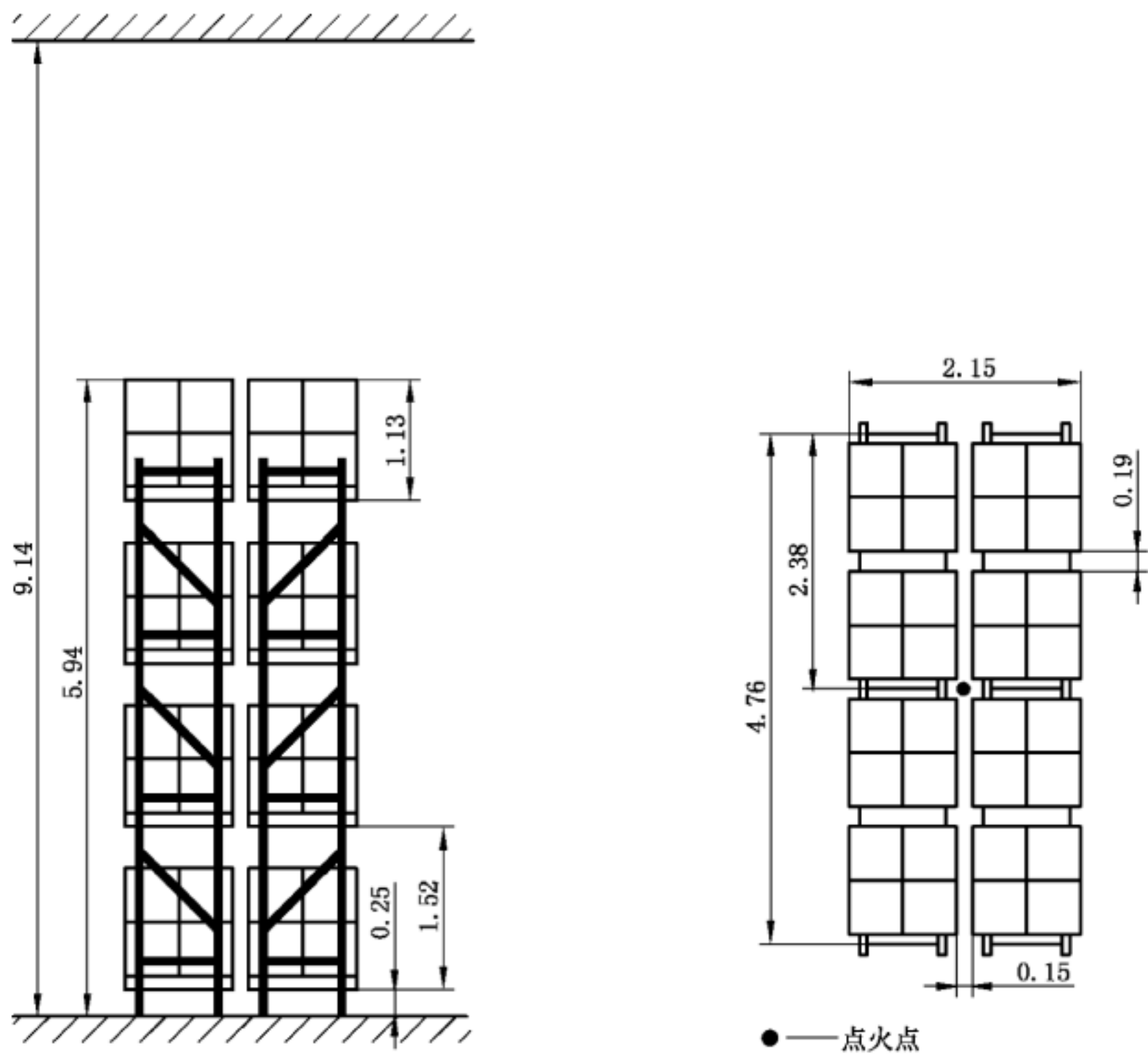
图 12 K 202 直立型 ESFR 喷头灭火试验布置 试验 A
