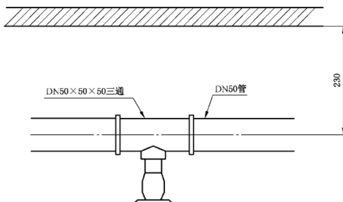
图 6 布水试验装置中管路的安装示意图
