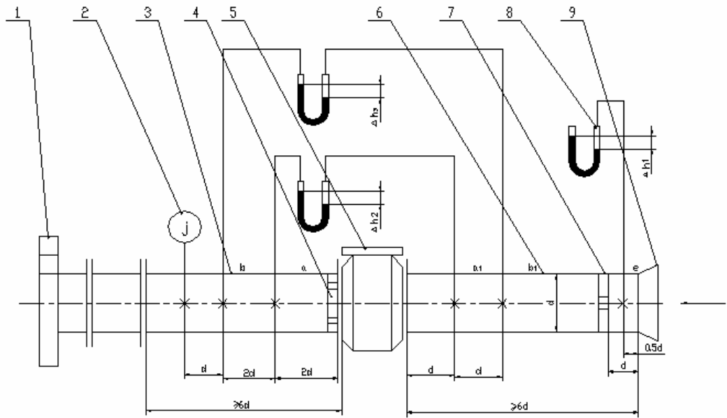
1——风机；2——温度计；3——出气测试管；4——出气整流栅；5——被测阻火器； 6——进气测试管；7——进气整流栅；8——压差计；9——集流器。
