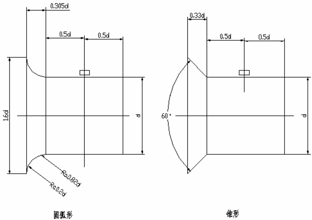
图 4 集流器外形尺寸
