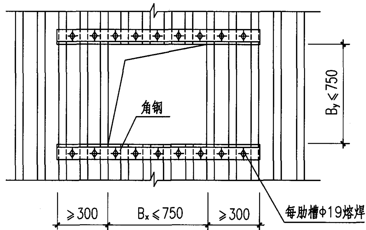
组合楼板开孔 \leq 750 时的加强措施(1)
