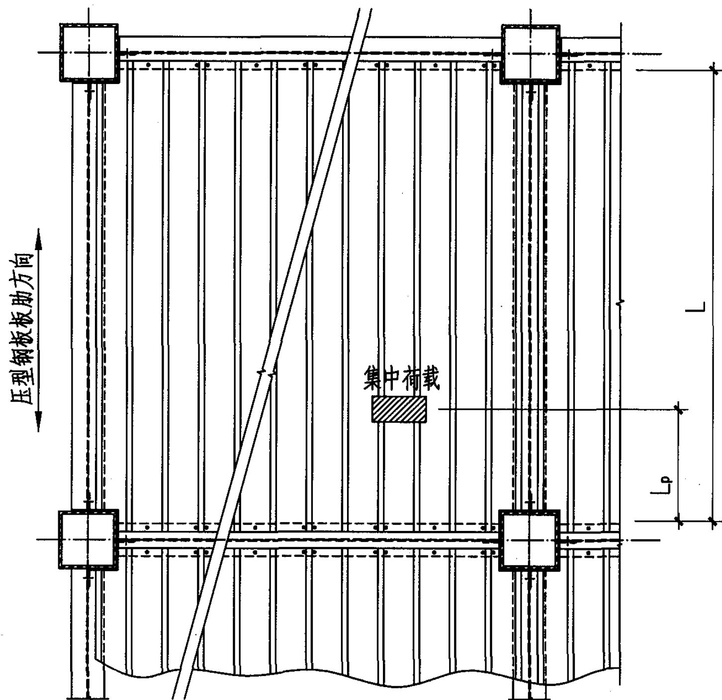
压型钢板铺板平面示意图
