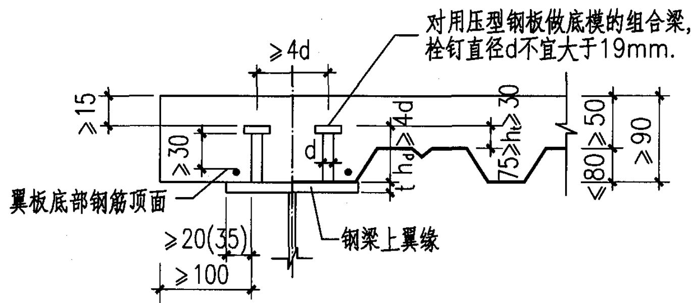
b. 组合梁翼板为压型钢板—混凝土组合楼板
