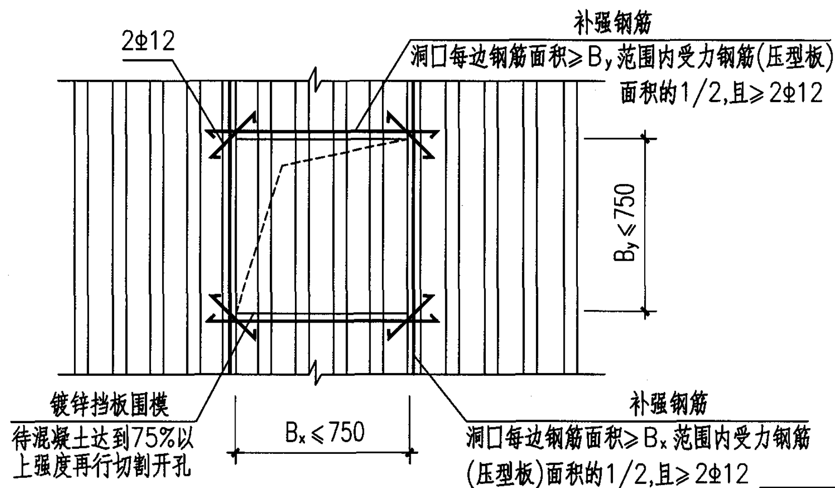
组合楼板开孔 \leq 750 时的加强措施(2)
