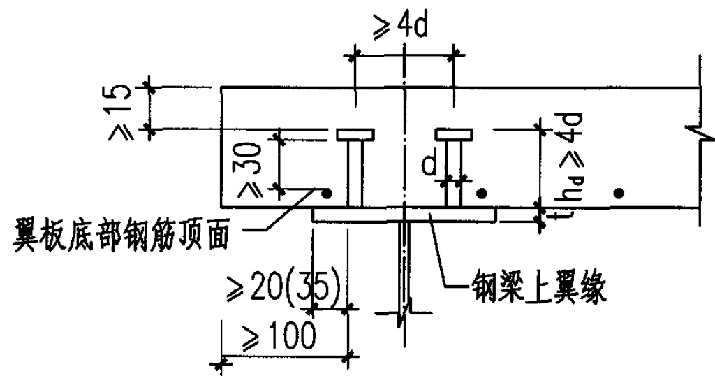
a. 组合梁翼板为现浇混凝土平板
