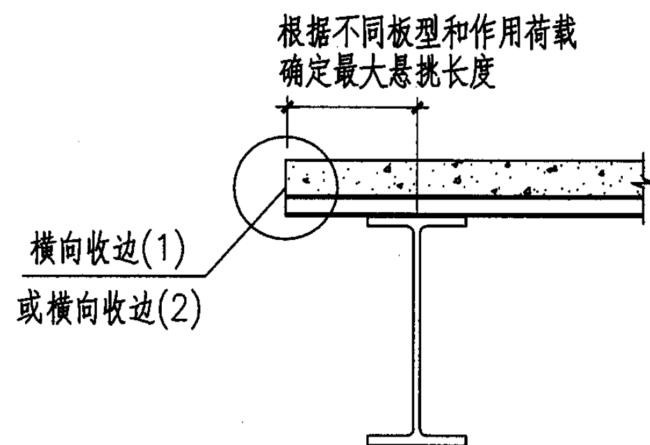
板肋与梁垂直收边构造(1)
