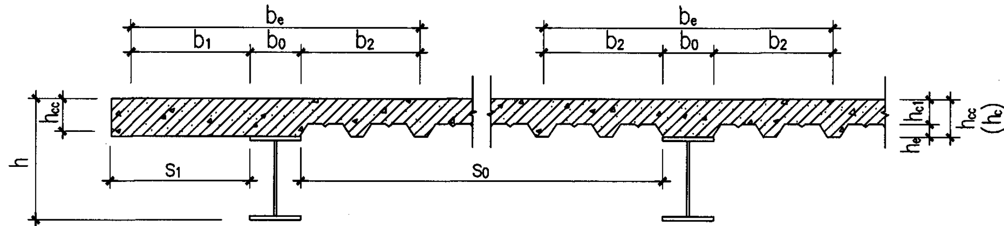
c.翼板为组合楼板
