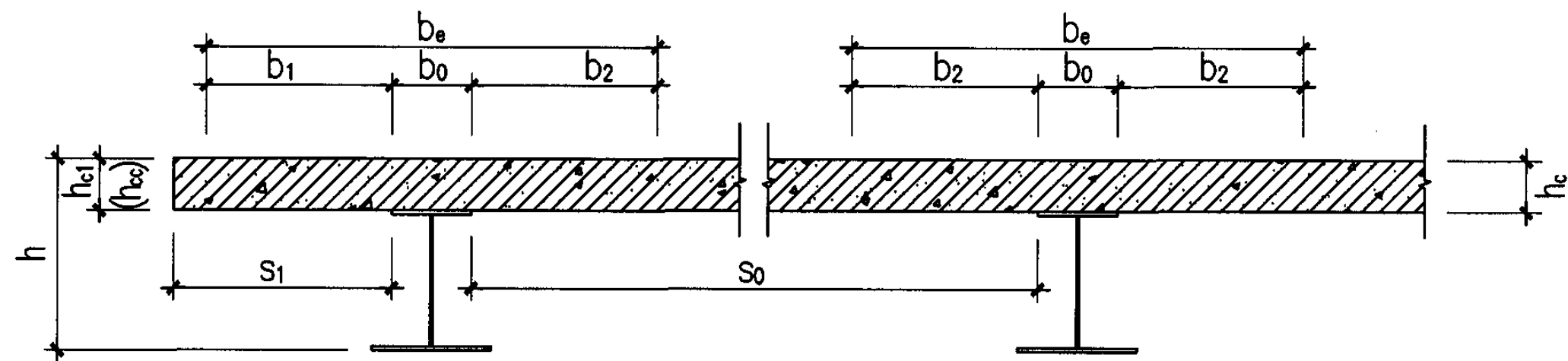
a.翼板为混凝土平板(无板托)
