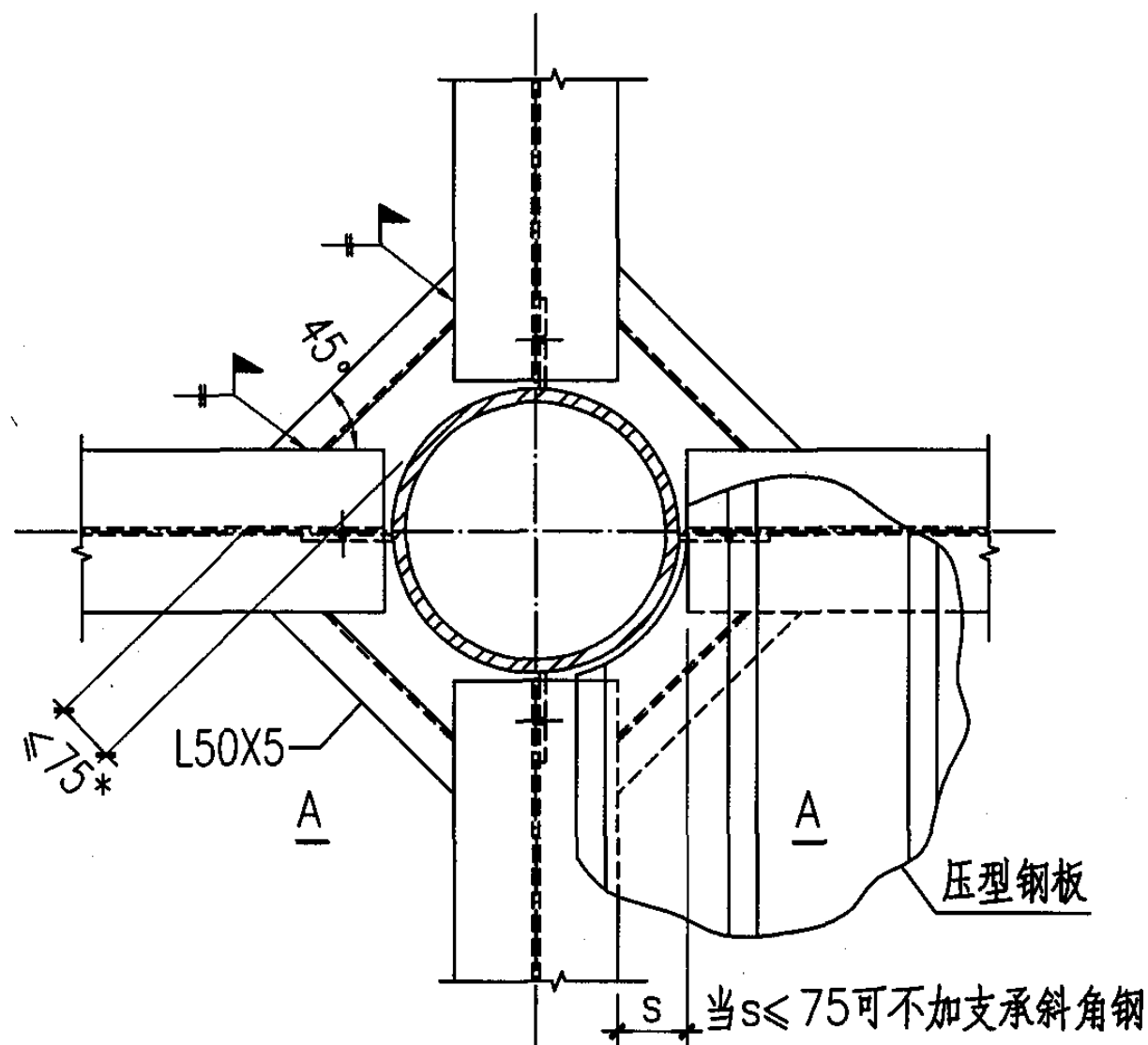
圆柱梁柱节点处压型钢板支托构造
