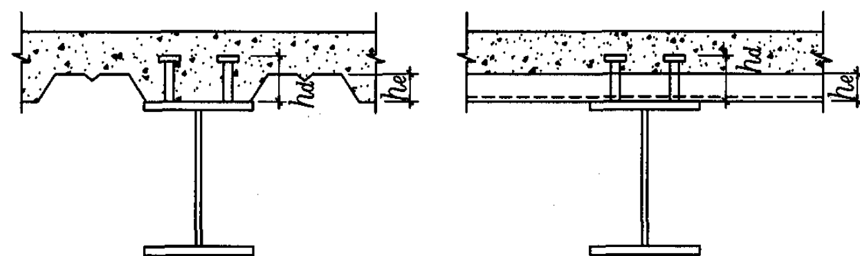
肋与钢梁平行的组合梁截面
