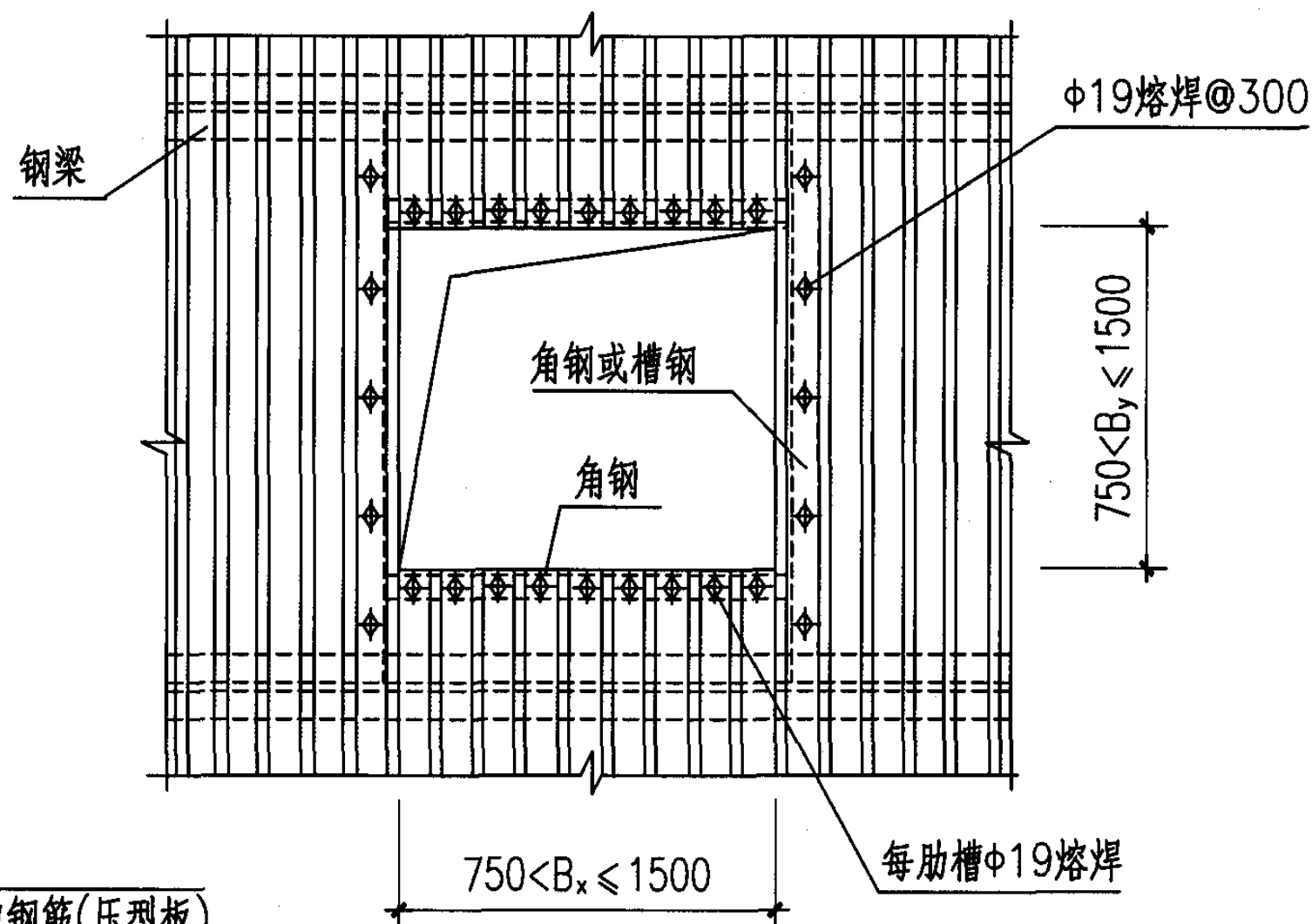
组合楼板开孔750~1500时的加强措施
