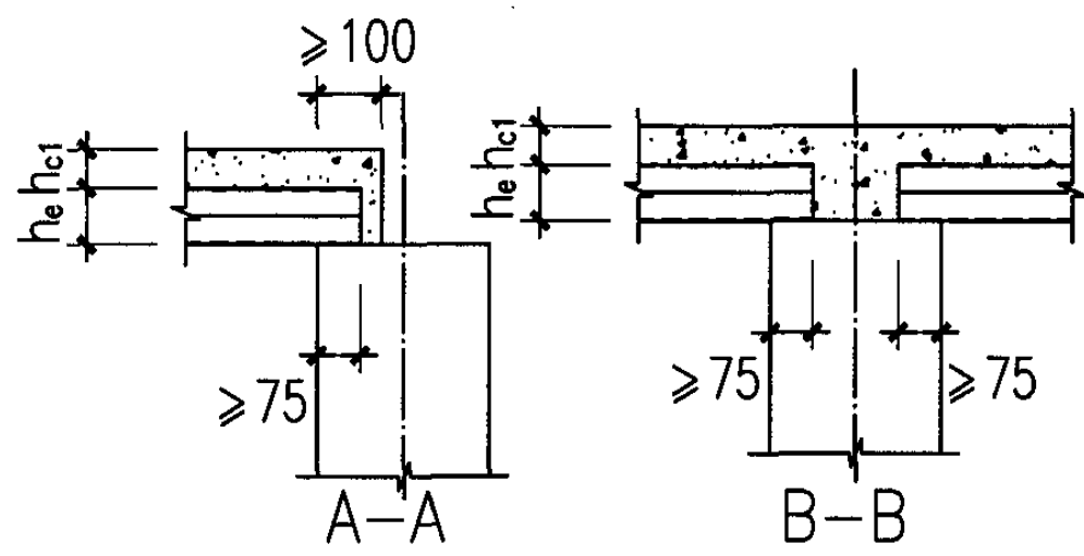
组合楼板支承长度构造要求
