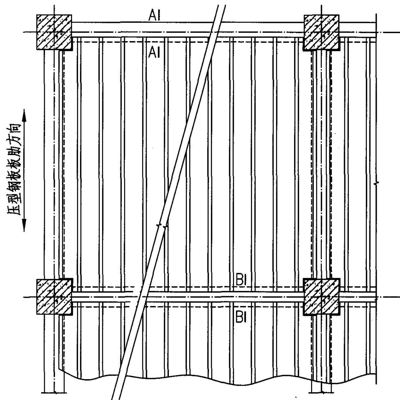
压型钢板铺板平面示意图
