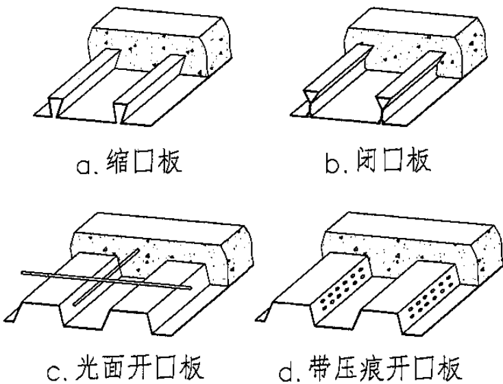
图 6.2-1 压型钢板组合楼板的基本形式
