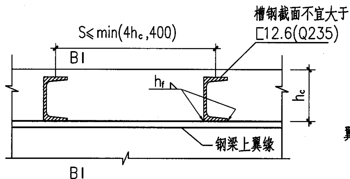
槽钢抗剪连接件构造
