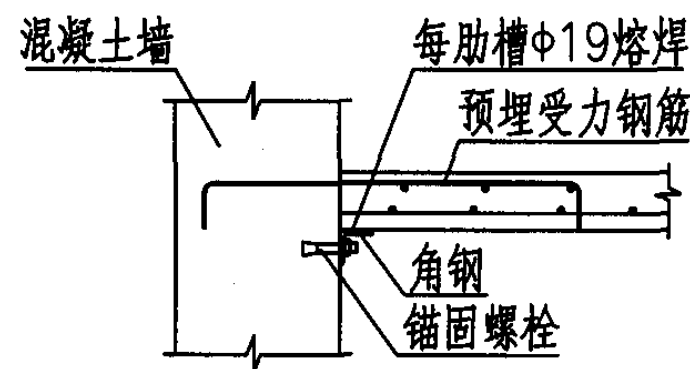
组合楼板与混凝土墙侧面连接做法
