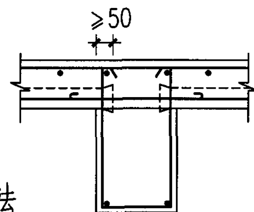
压型钢板锚固方法
