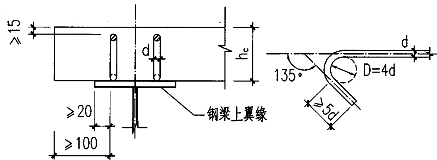
弯筋抗剪连接件弯钩构造 (HPB235级钢筋)
