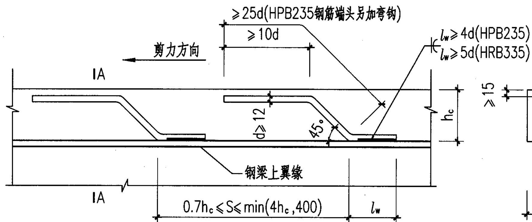
弯筋抗剪连接件构造
