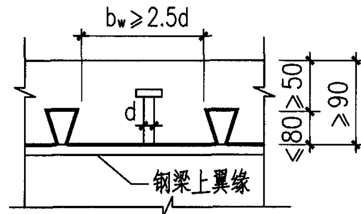
b. 缩口型或闭口型
