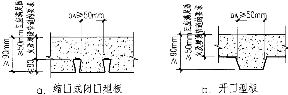
图 6.5-1 对组合楼板截面形状的要求
