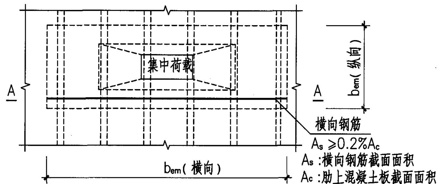
局部集中荷载作用下的横向钢筋
