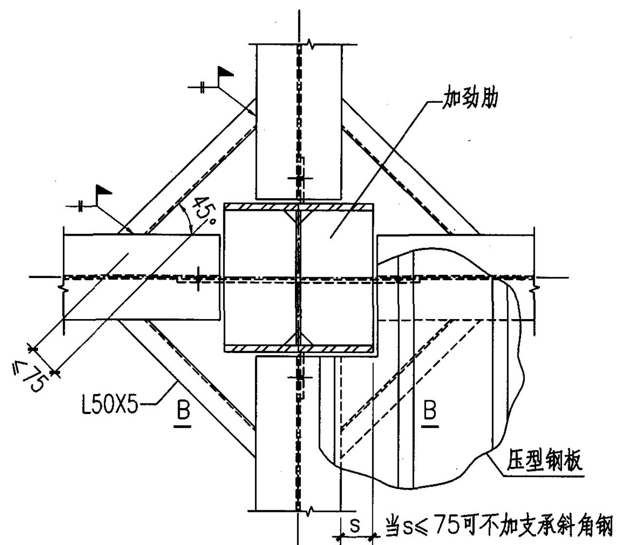
H型钢柱梁柱节点处压型钢板支托构造(2)
