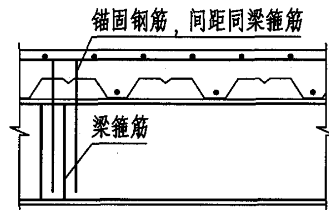
b. 钢筋插入法
