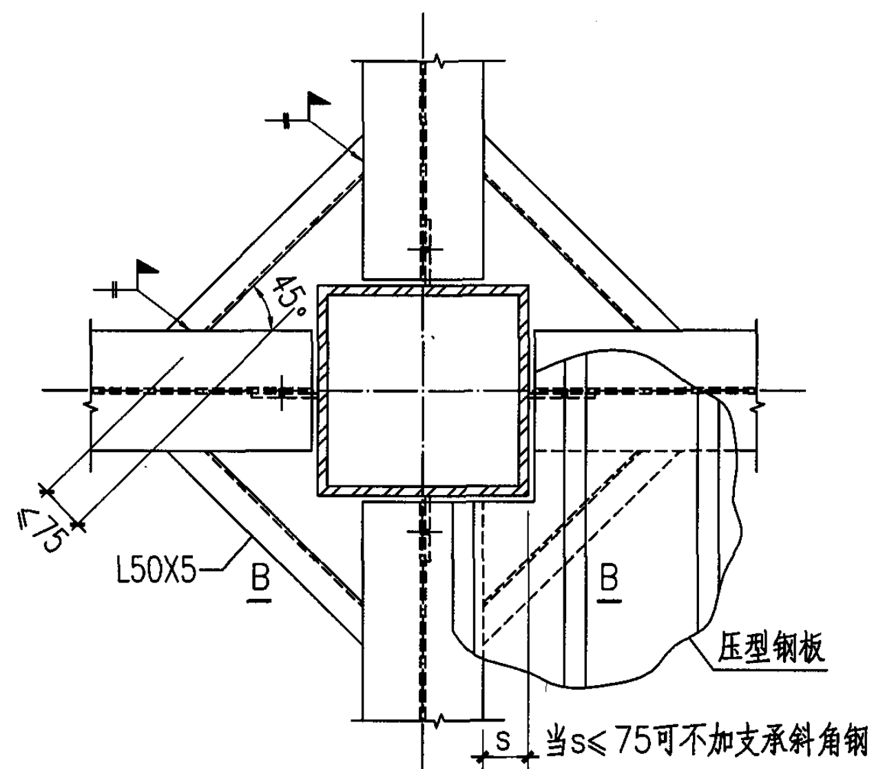
箱型钢柱梁柱节点处压型钢板支托构造(2)
