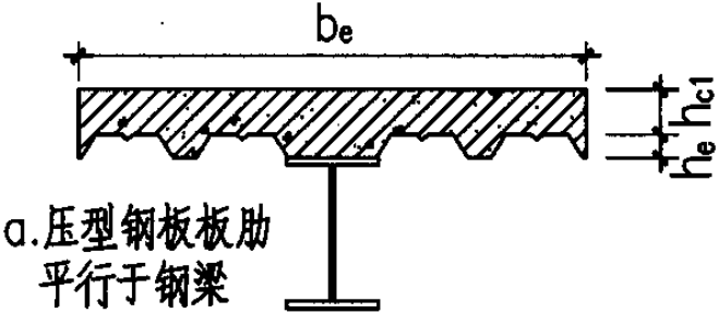
组合梁截面示意图
