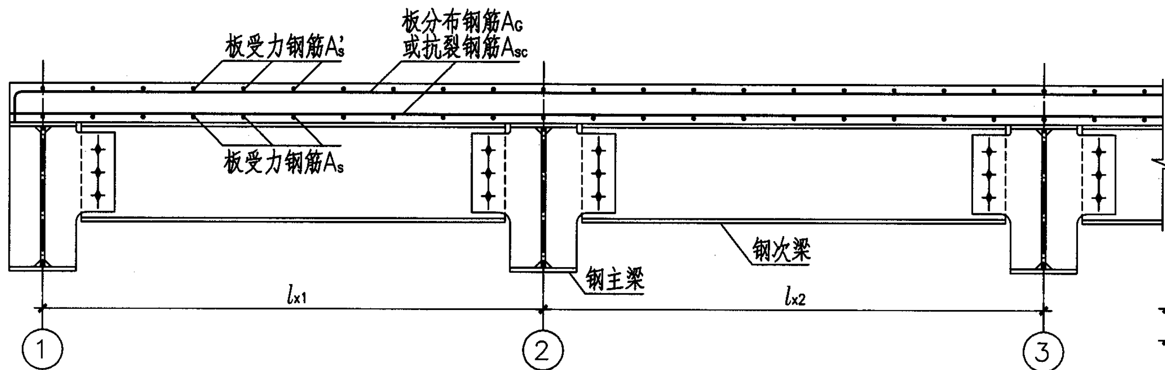
1-1 简支组合梁节点连接及配筋构造
