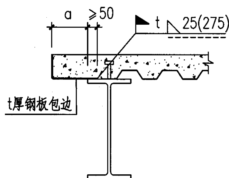
板肋与梁平行收边构造 ( a \leq 250 )
