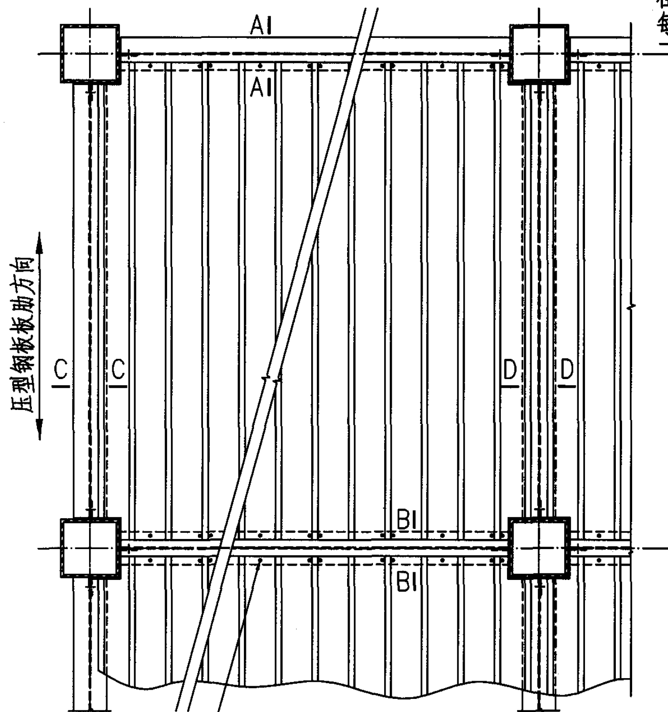
压型钢板铺板平面示意图
