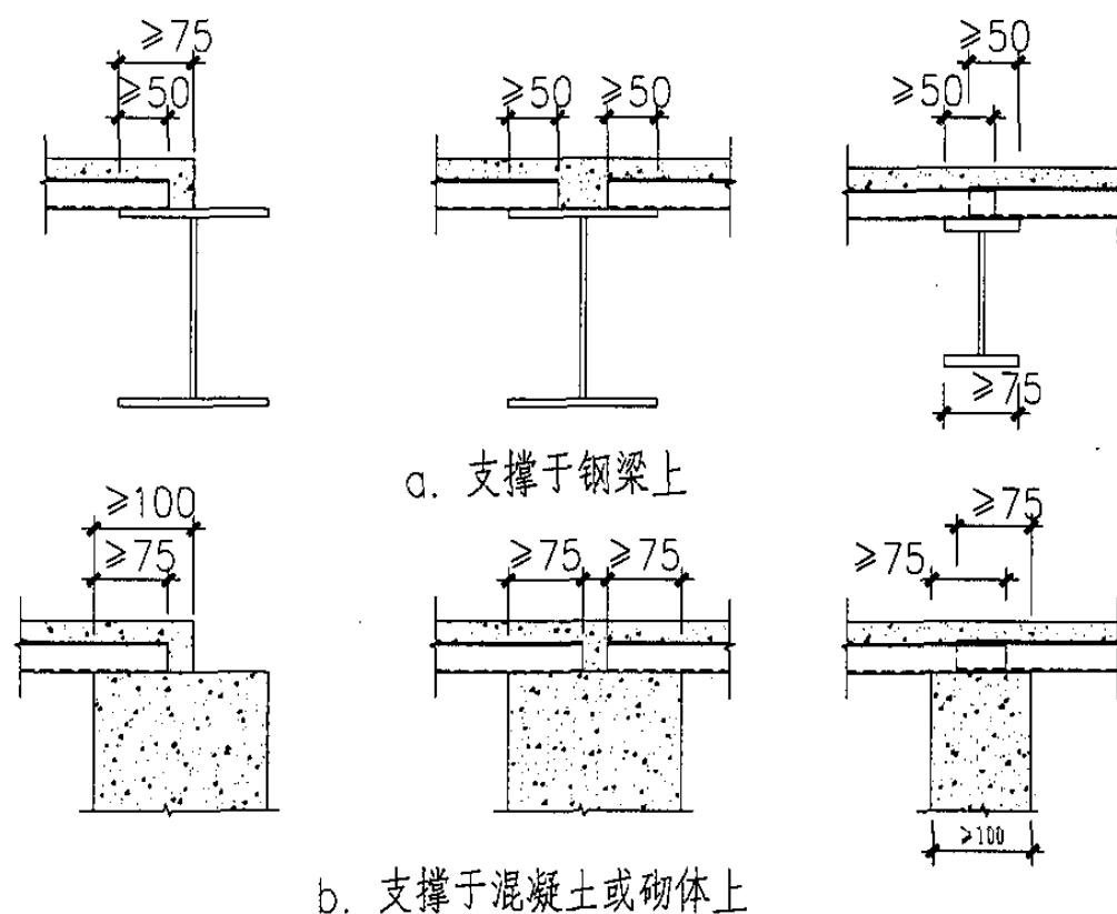
图 6.5-2 组合楼板的支承长度要求
