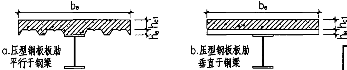
组合梁截面示意图
