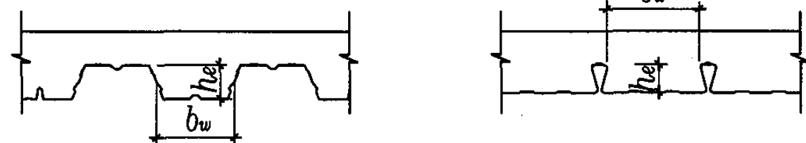
压型钢板组合板剖面
