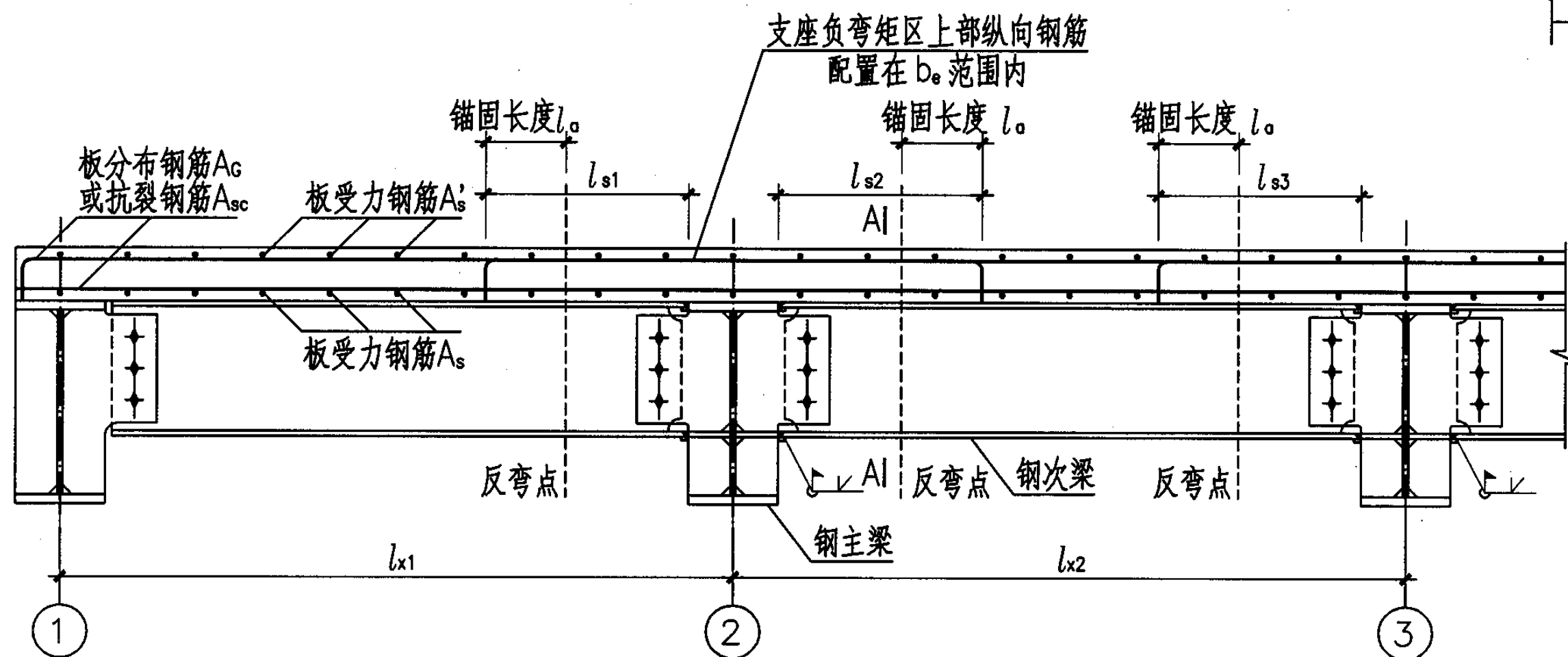
2-2 连续组合梁节点连接及配筋构造
