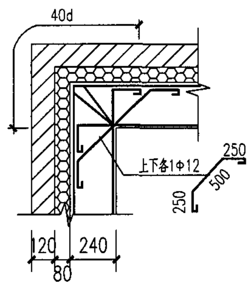
圈梁联接节点(一)
