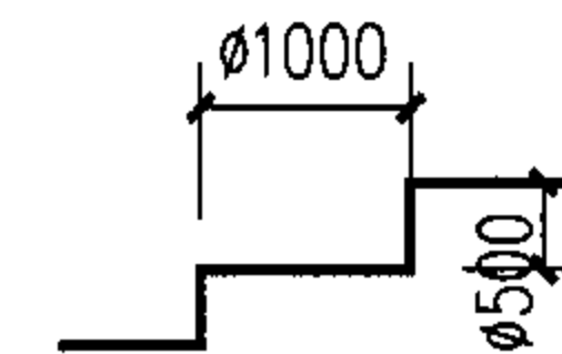
毛石基础放台示意图
