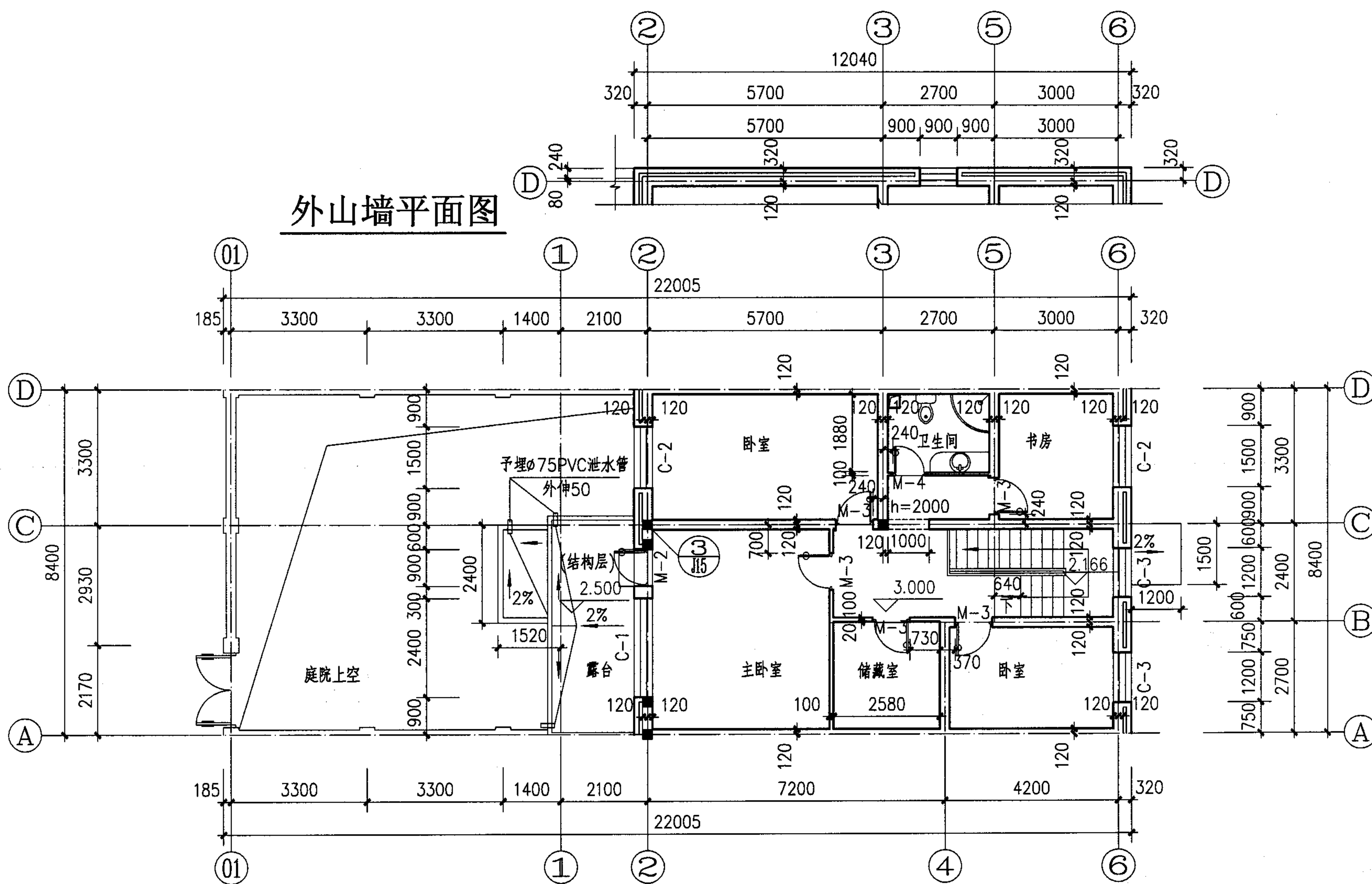
二层平面图
