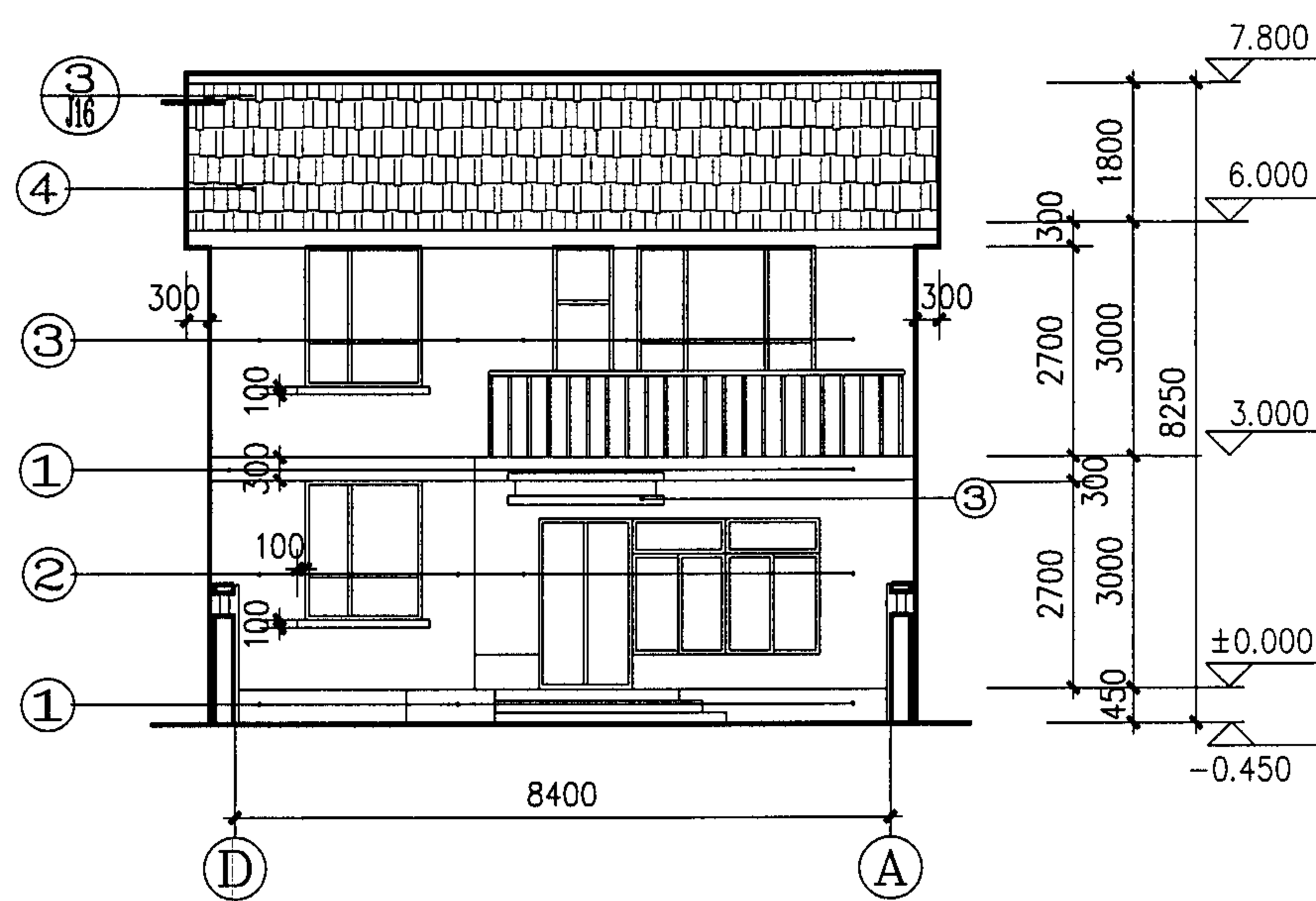
④-①轴立面图
