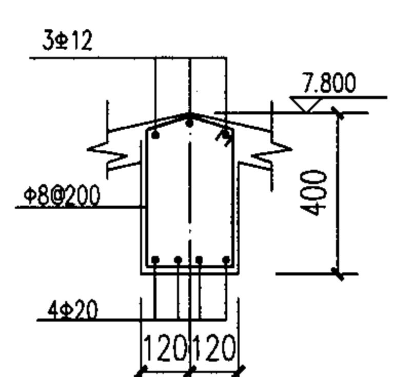
XL-3 梁长=5340
