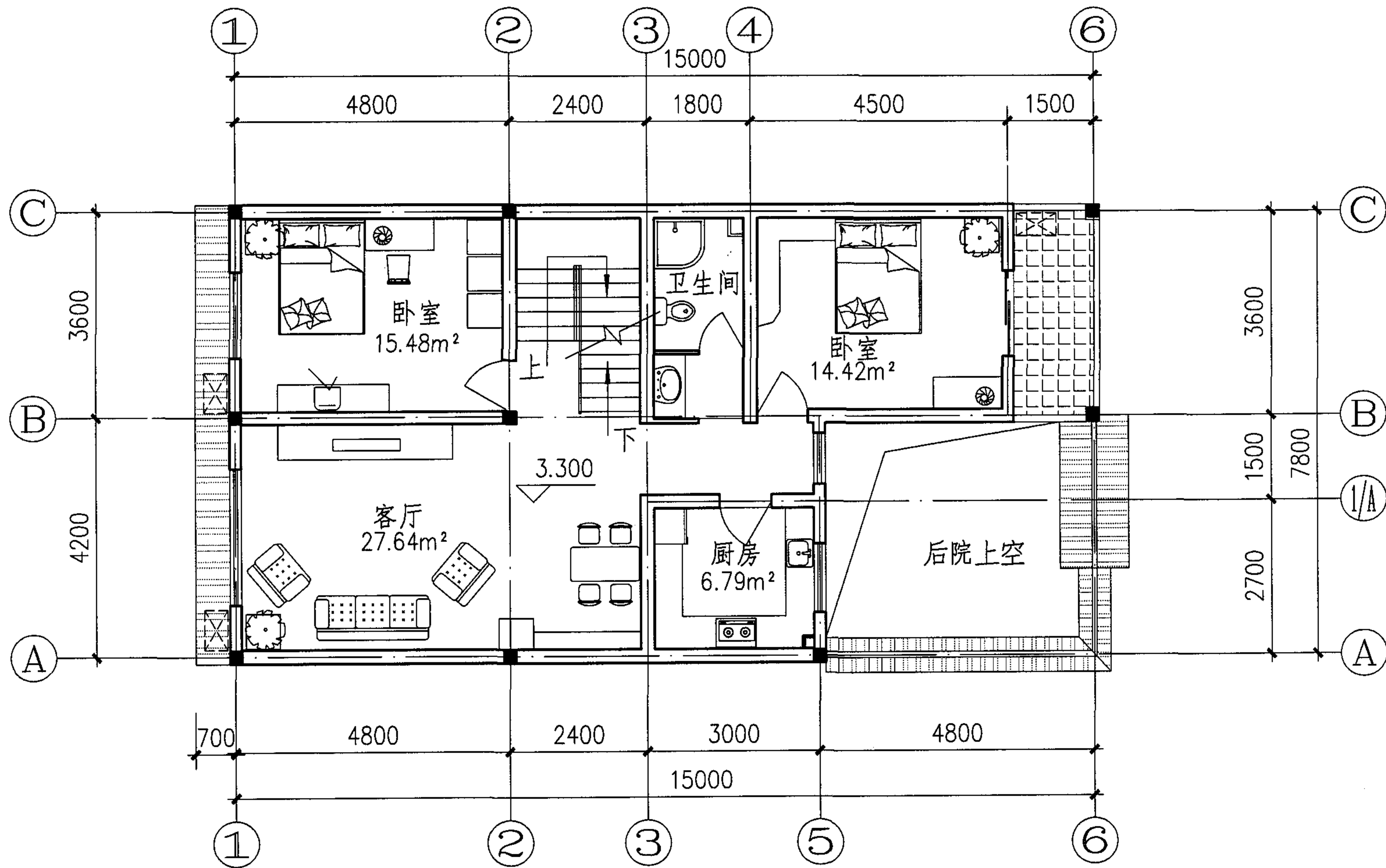
二层平面家具布置示意图
