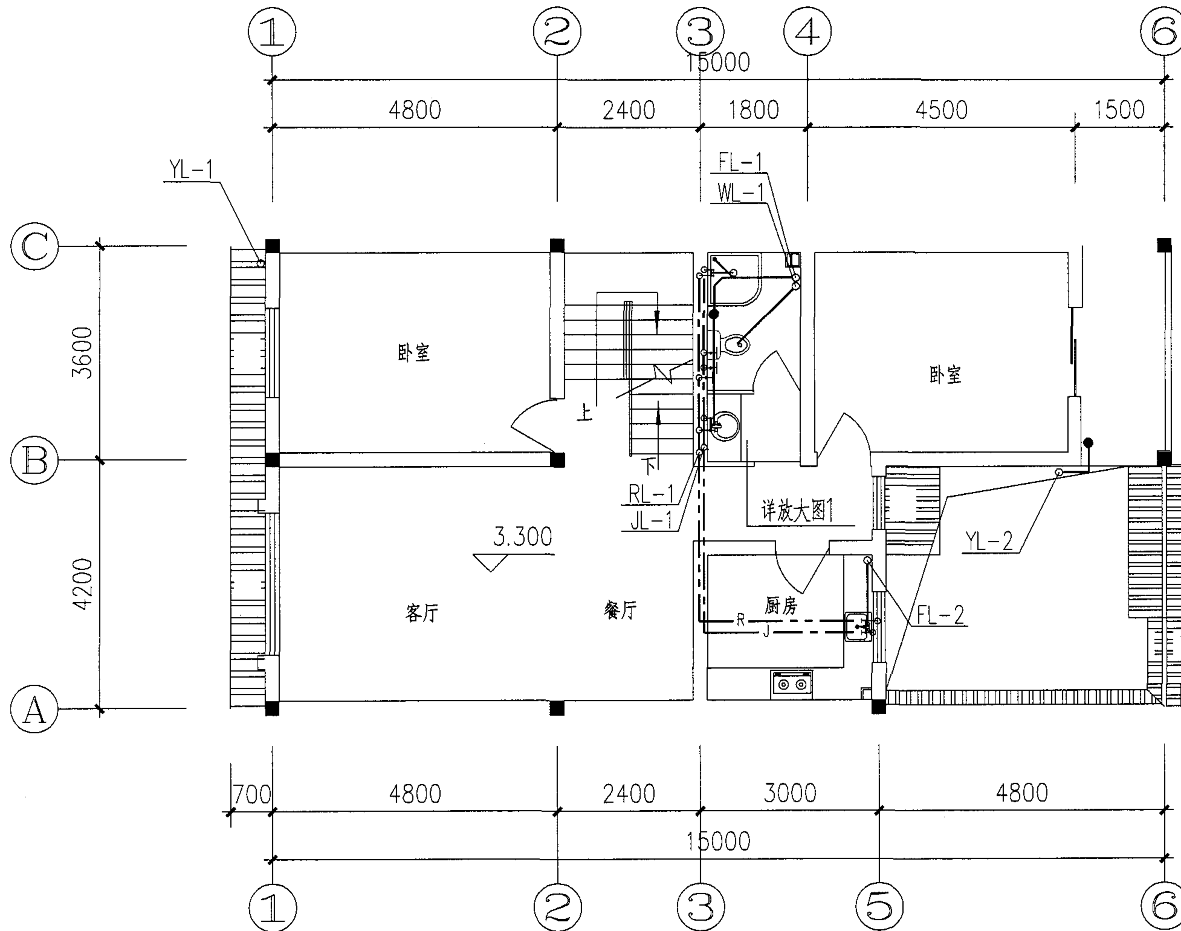
二层给排水平面图
