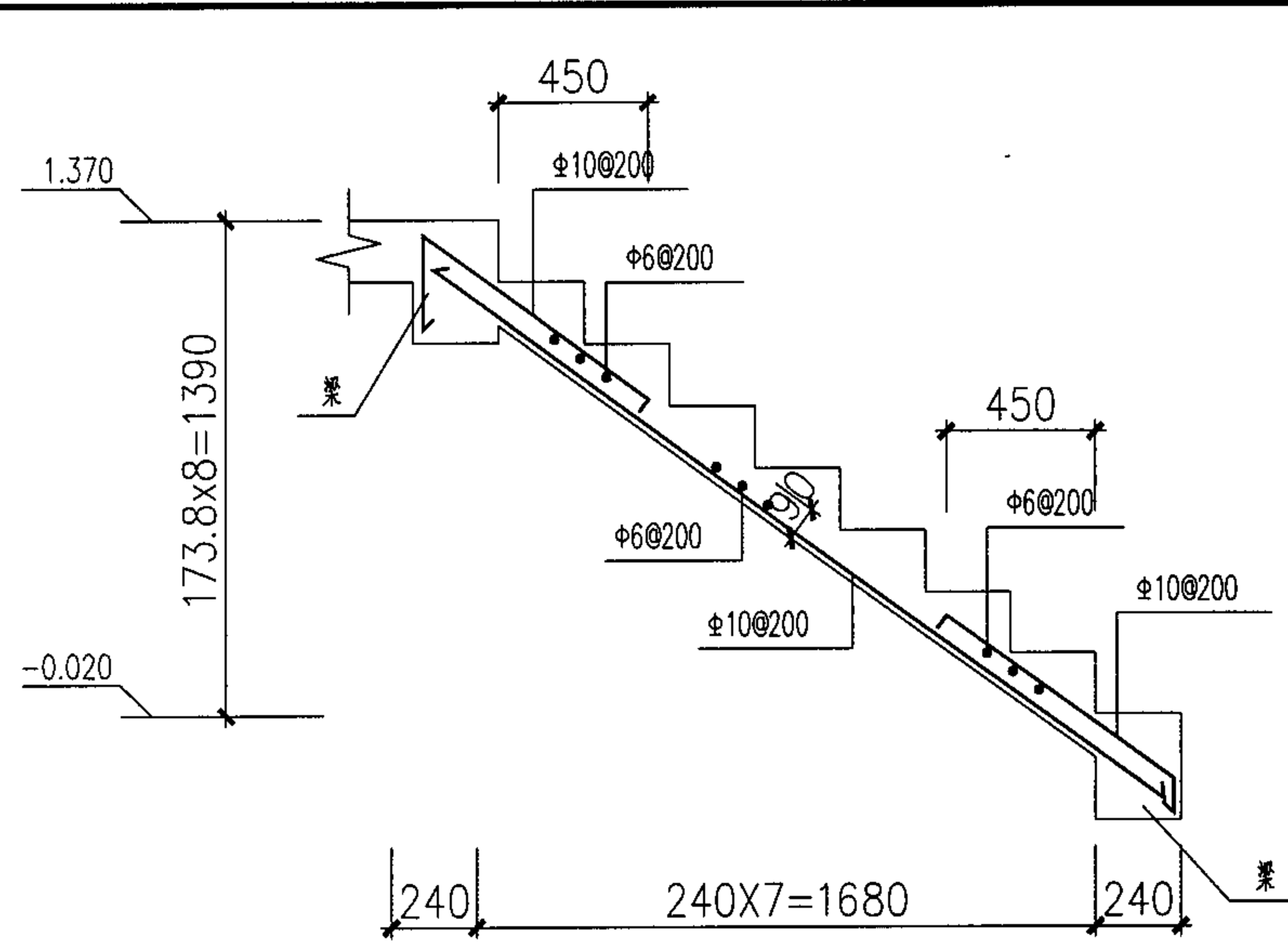
TB-1 板宽1040
