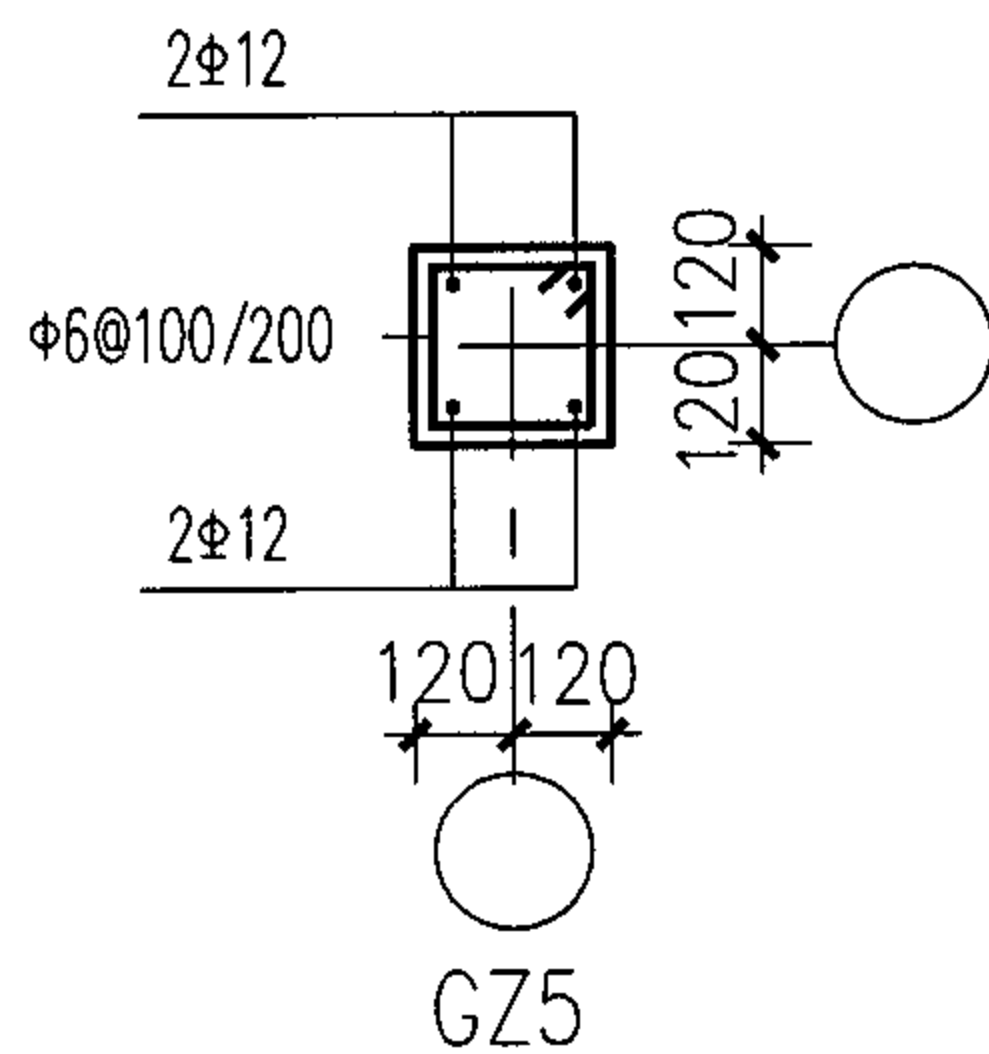
标高:6.280~屋面 (主筋锚入下面梁400)
