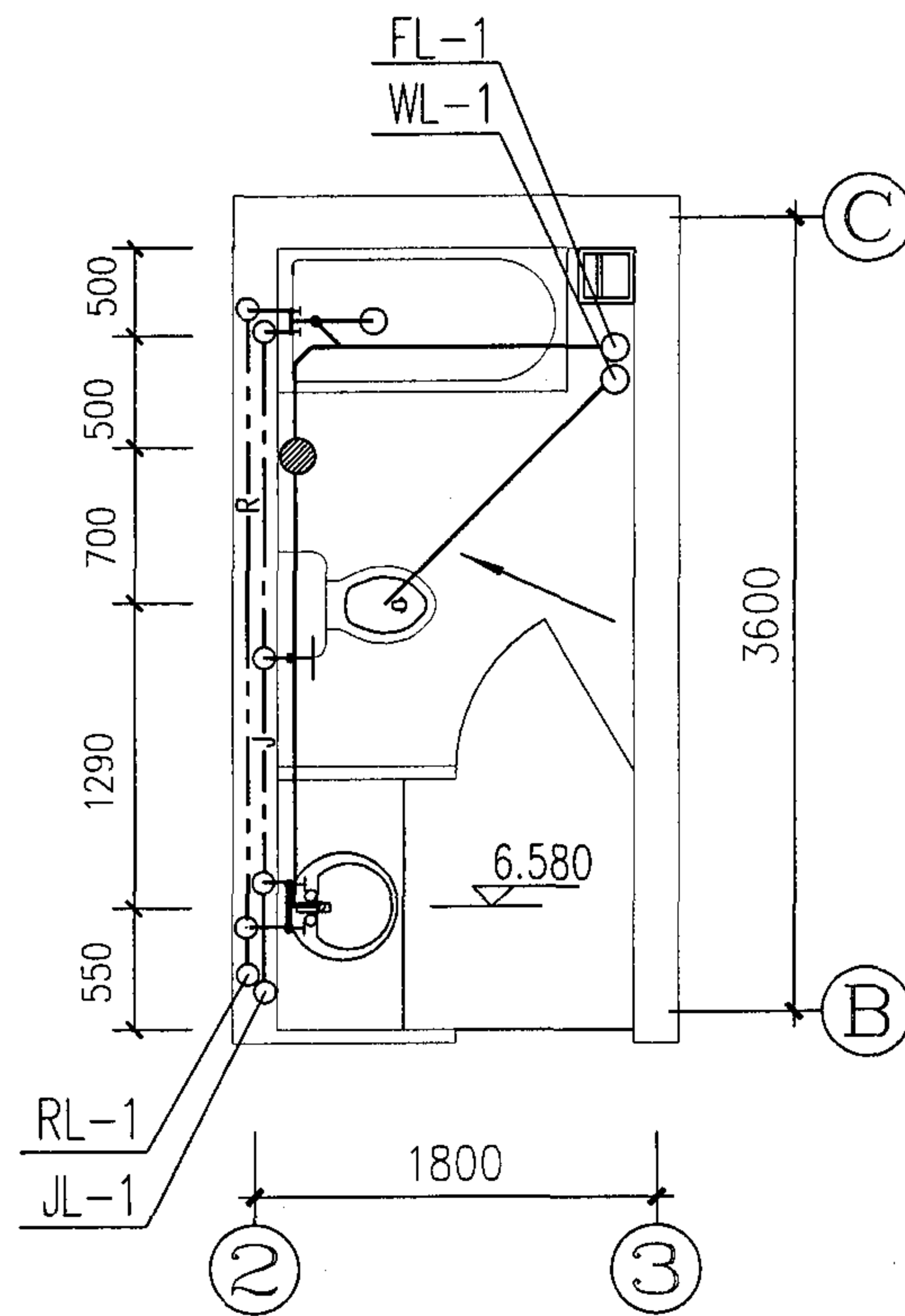
三层卫生间平面放大图
