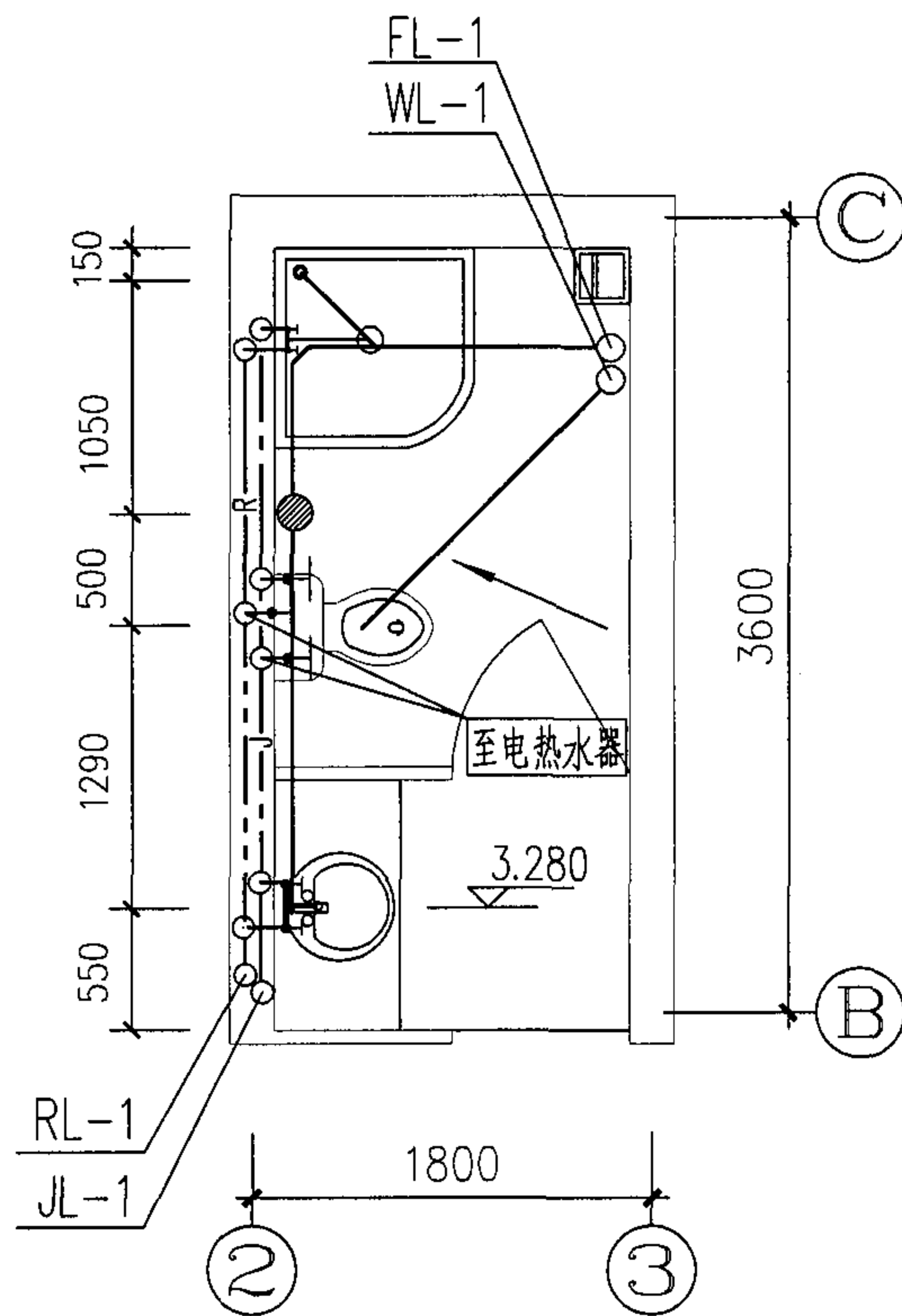
二层卫生间平面放大图
