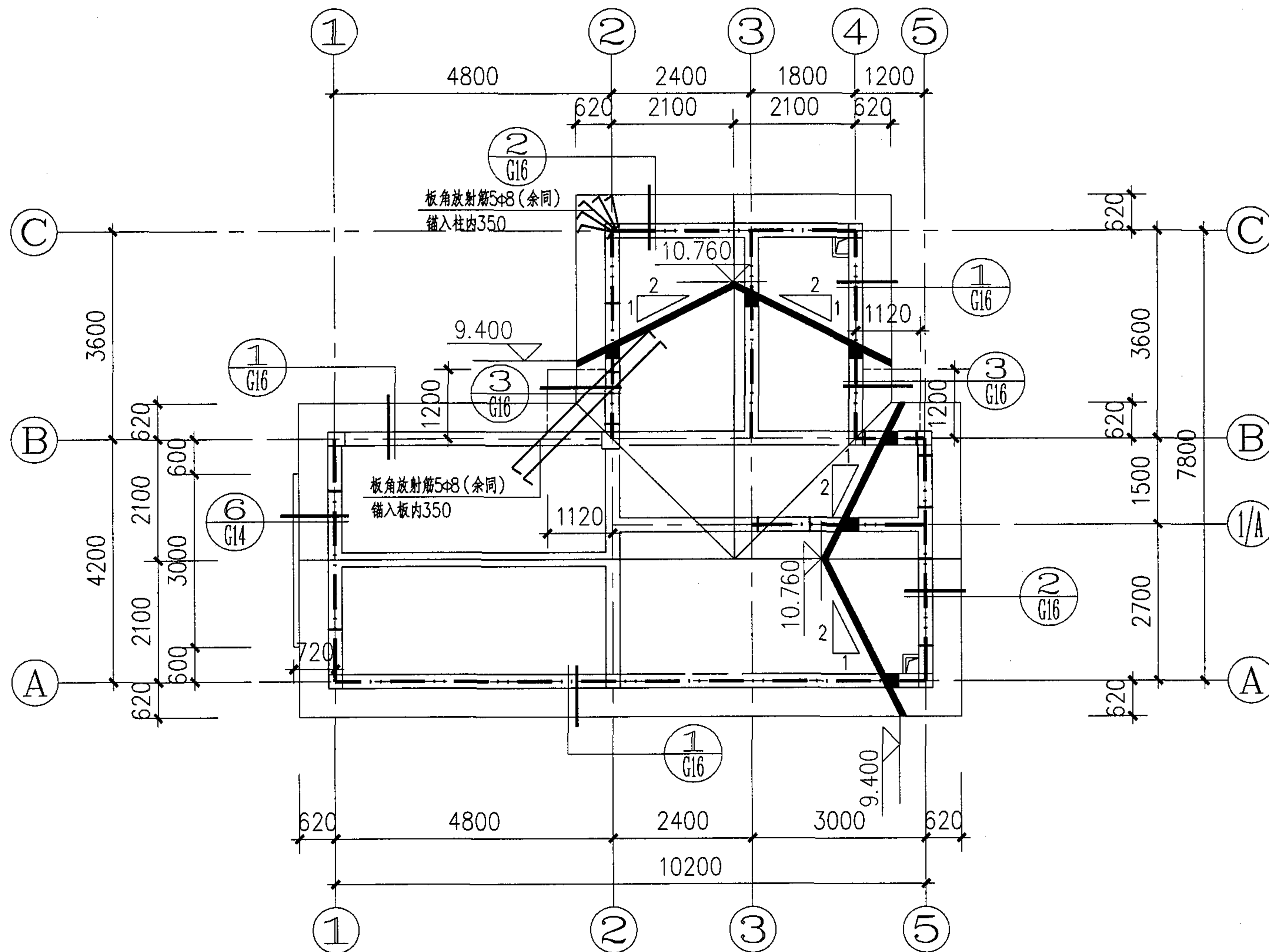
屋面层结构平面布置图
