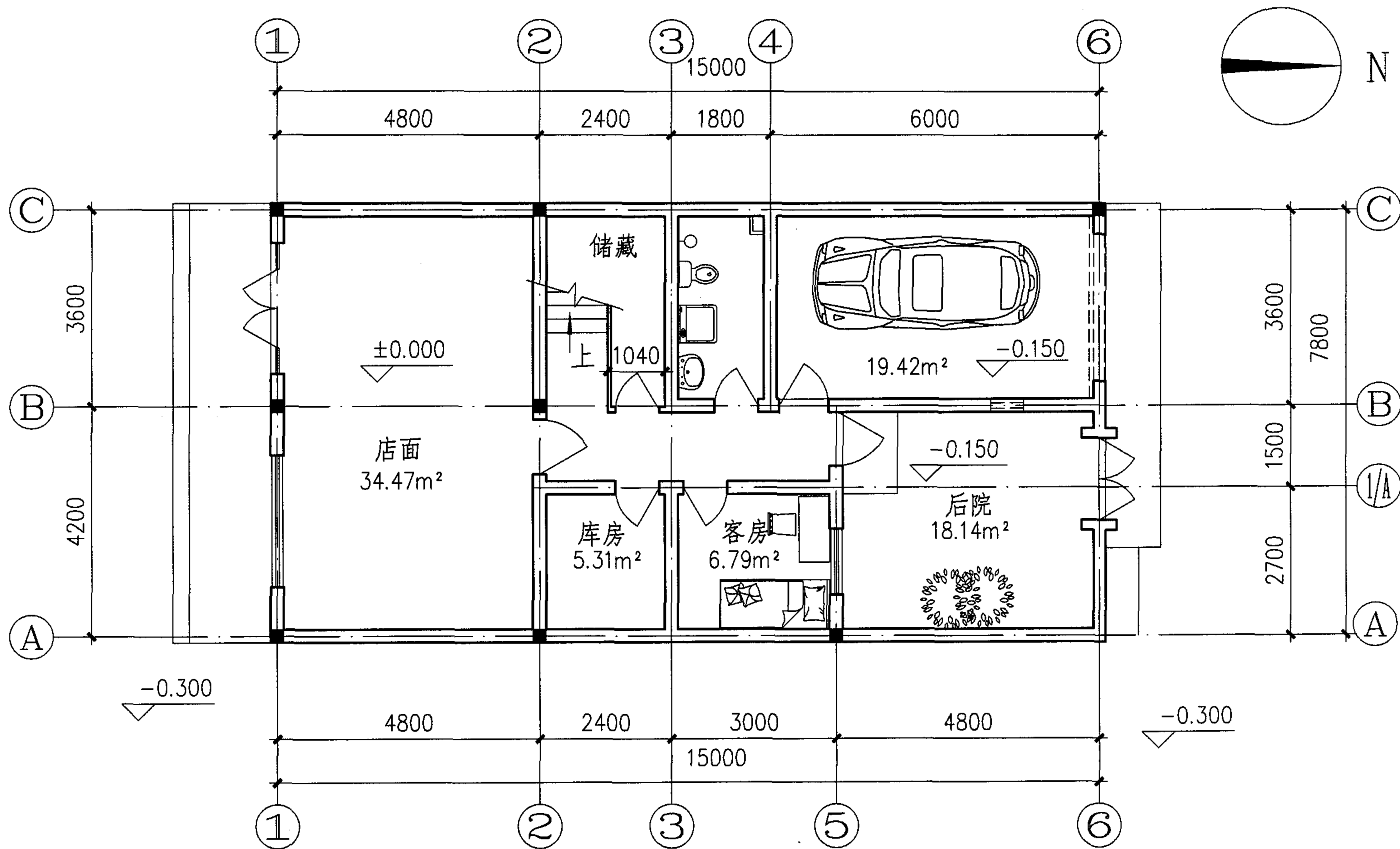
一层平面家具布置示意图
