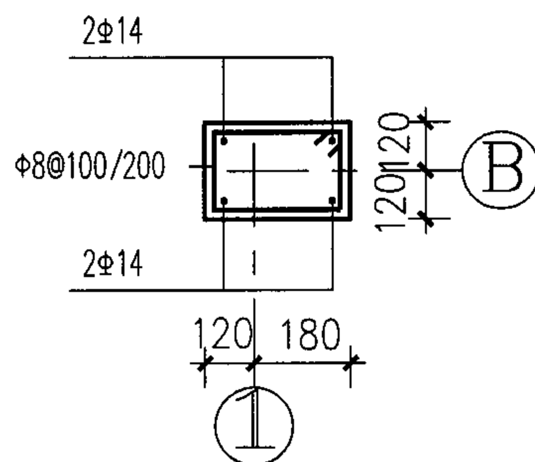
标高:基础梁顶~屋面
