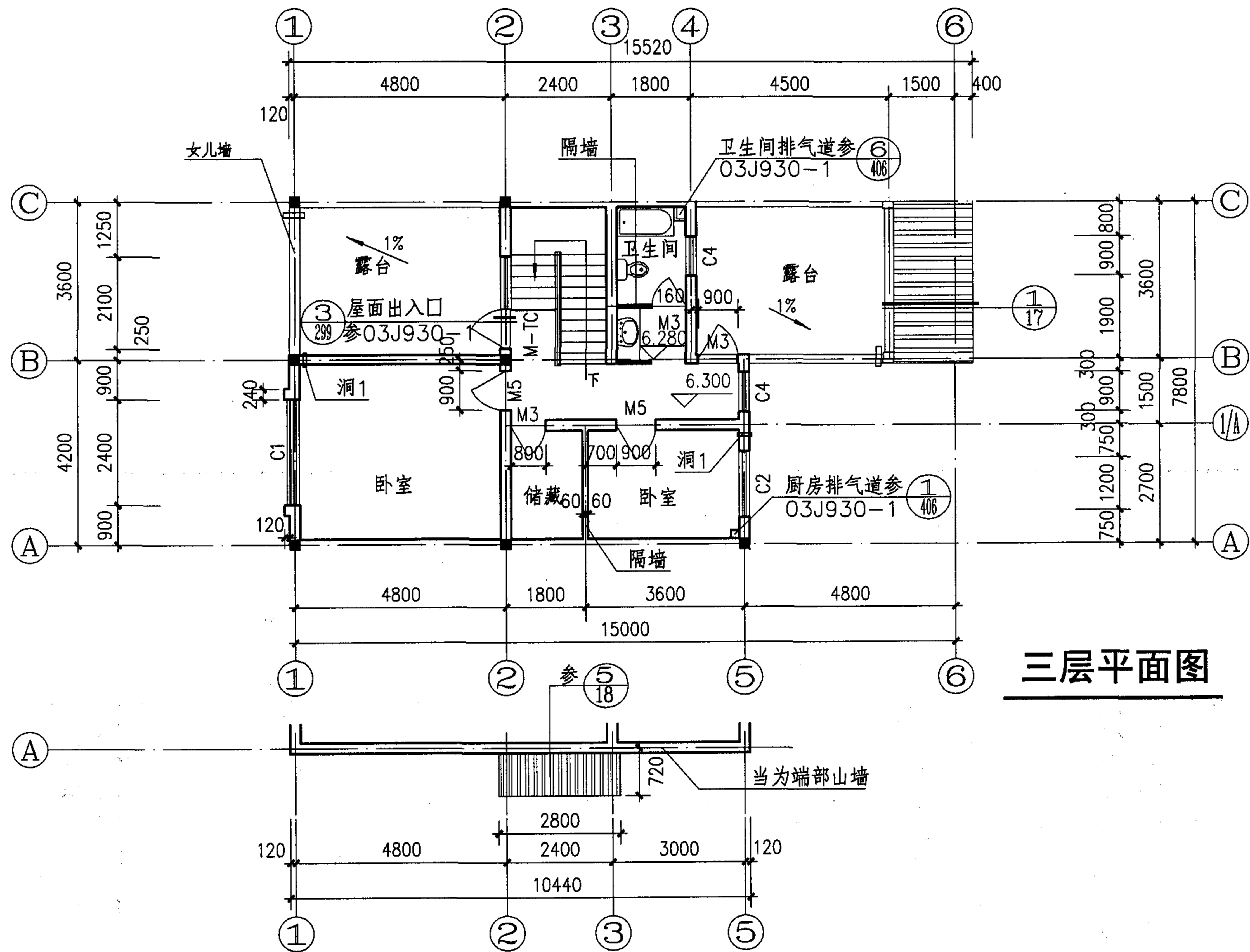
三层平面图
