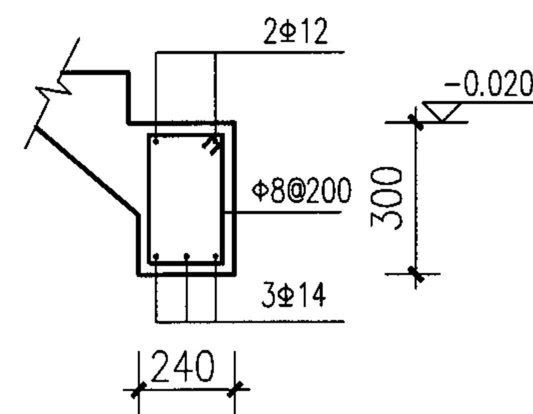
TL-1 梁长L=2640
