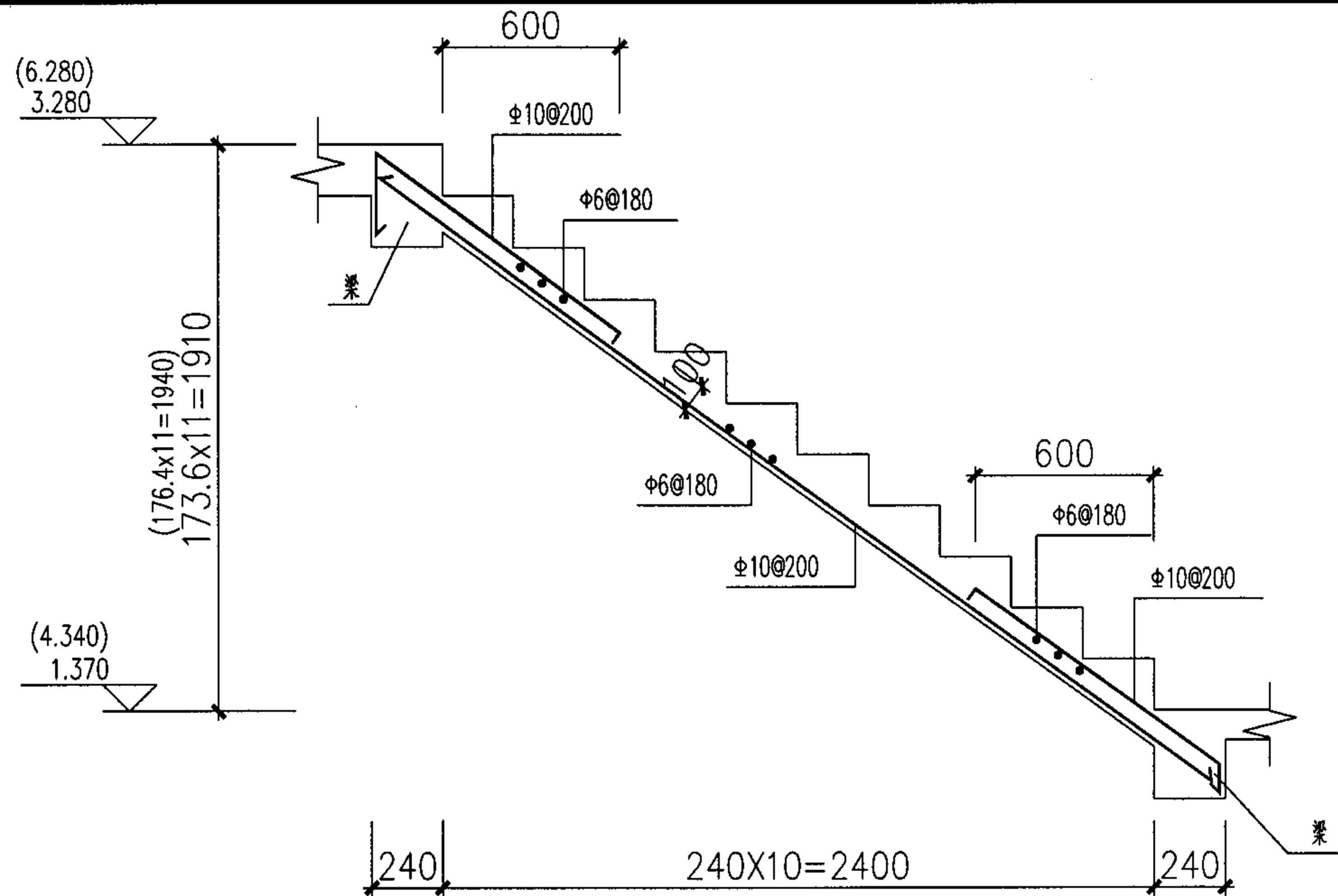
TB-2 (TB-2a) 板宽1040
