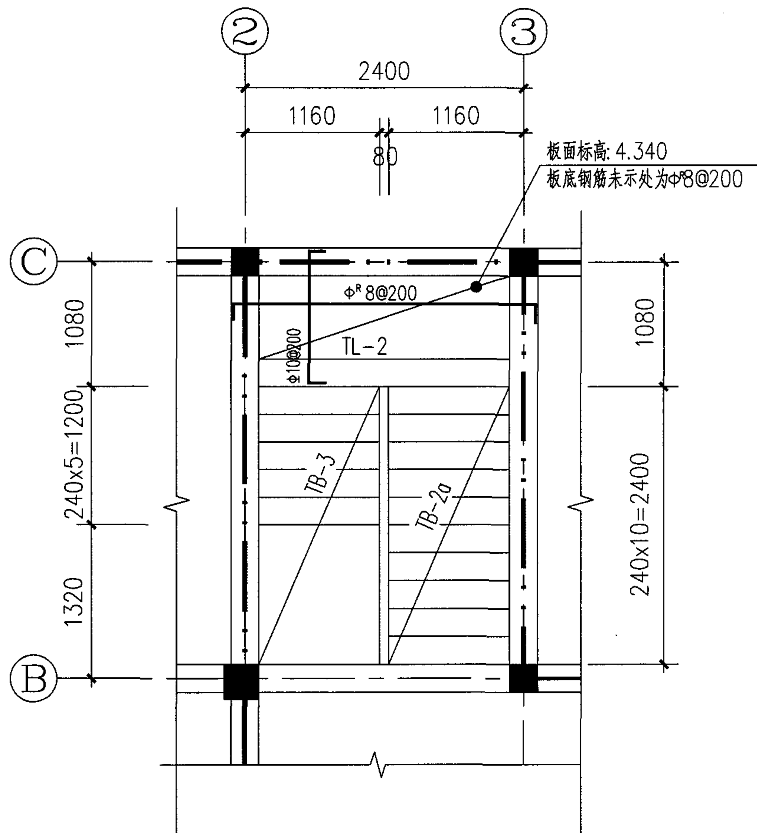
三层楼梯结构平面图
