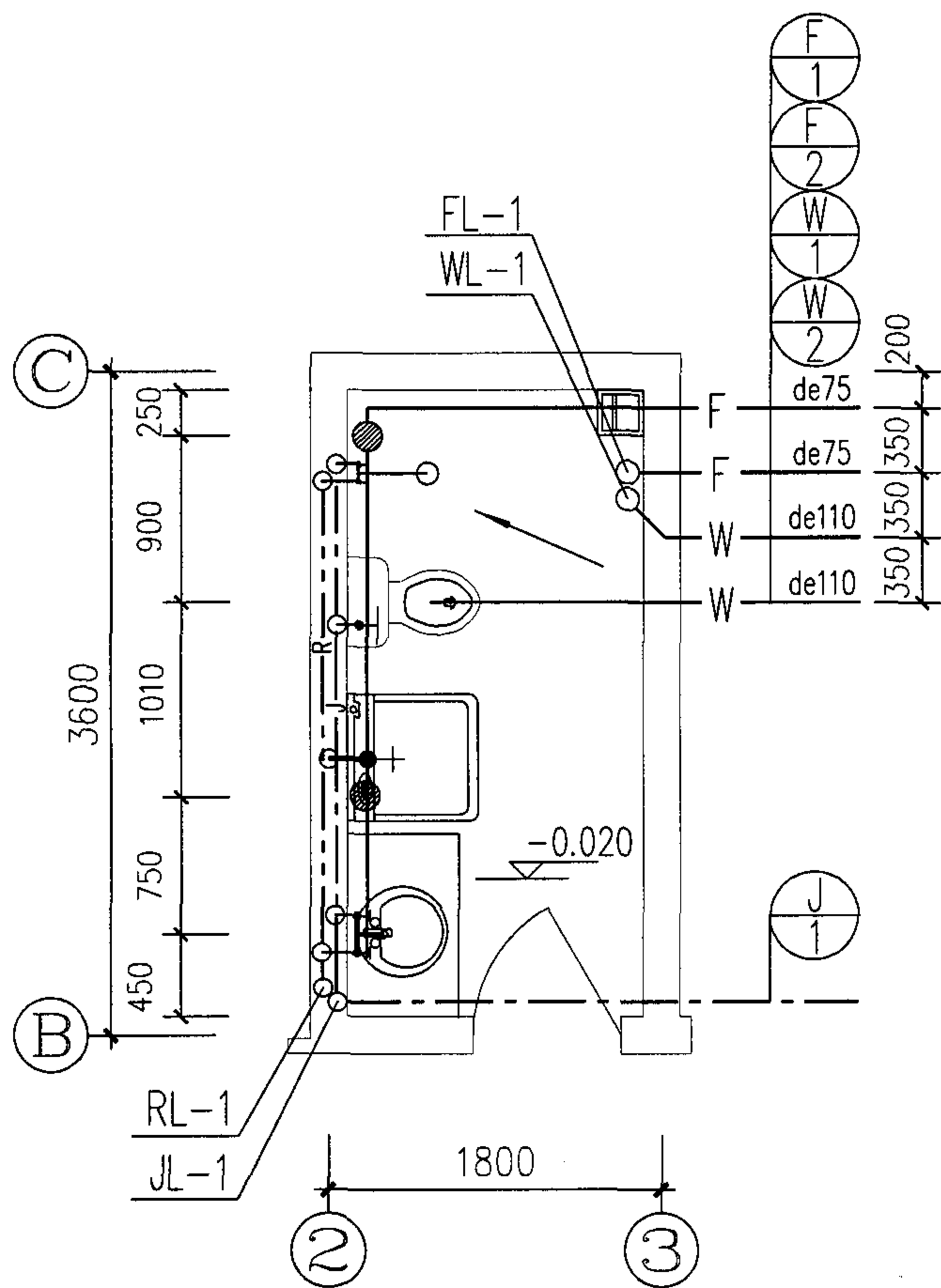
一层卫生间平面放大图
