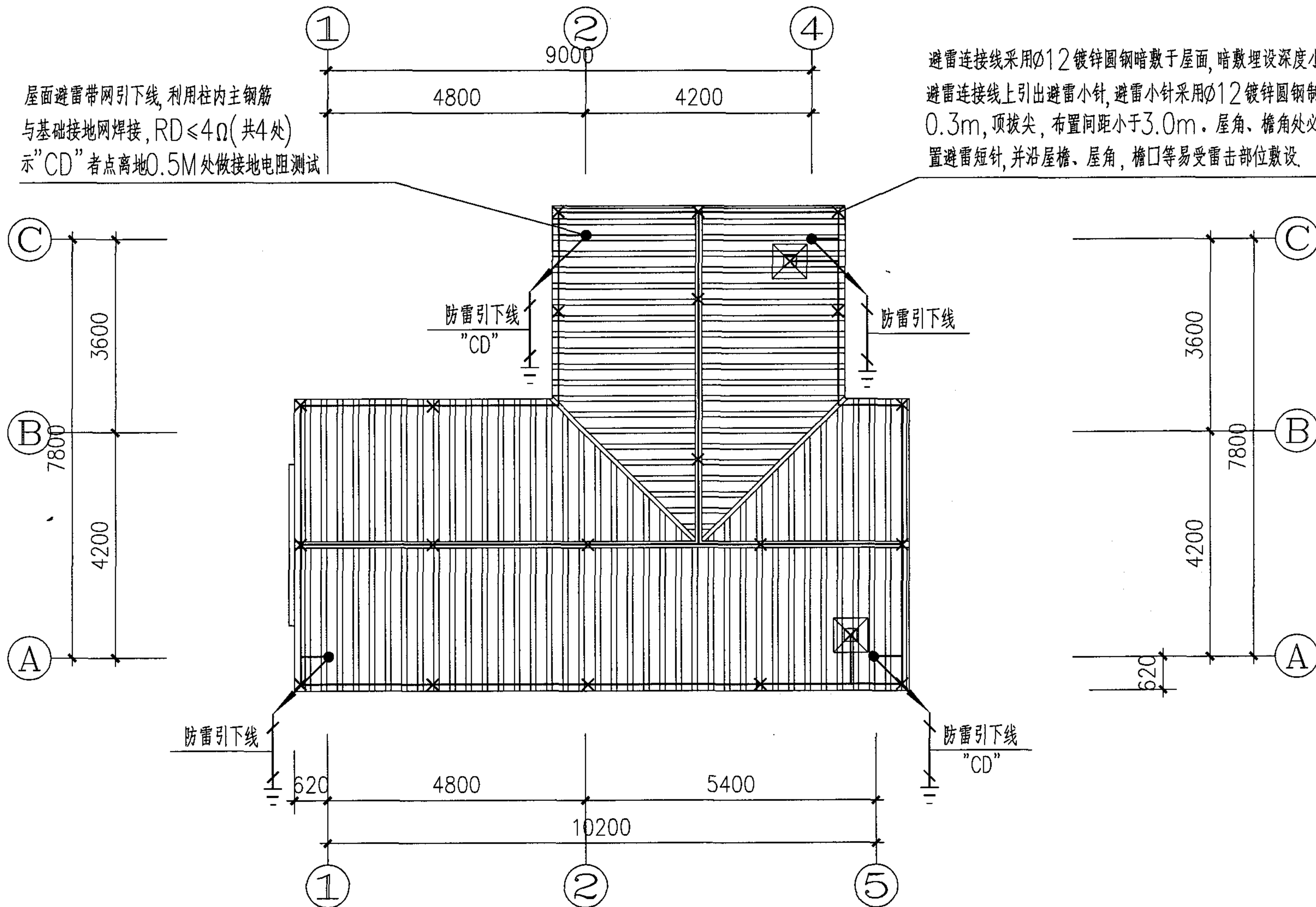
屋面防雷平面图
