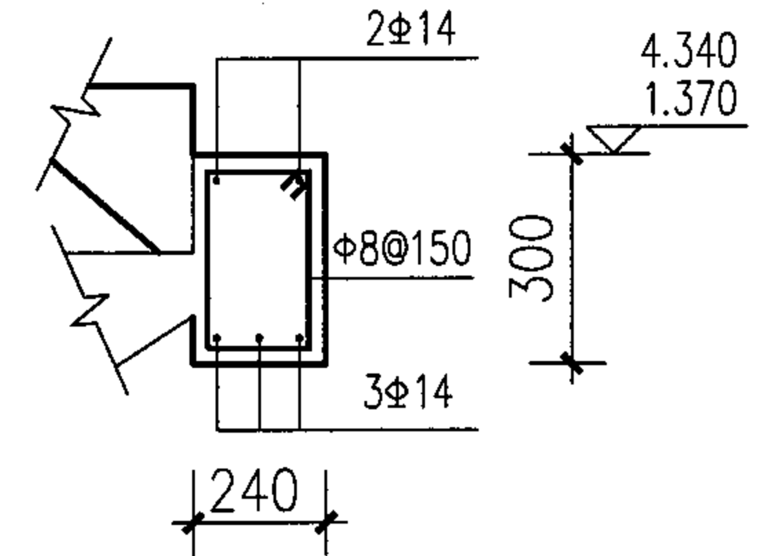
TL-2 梁长L=2640
