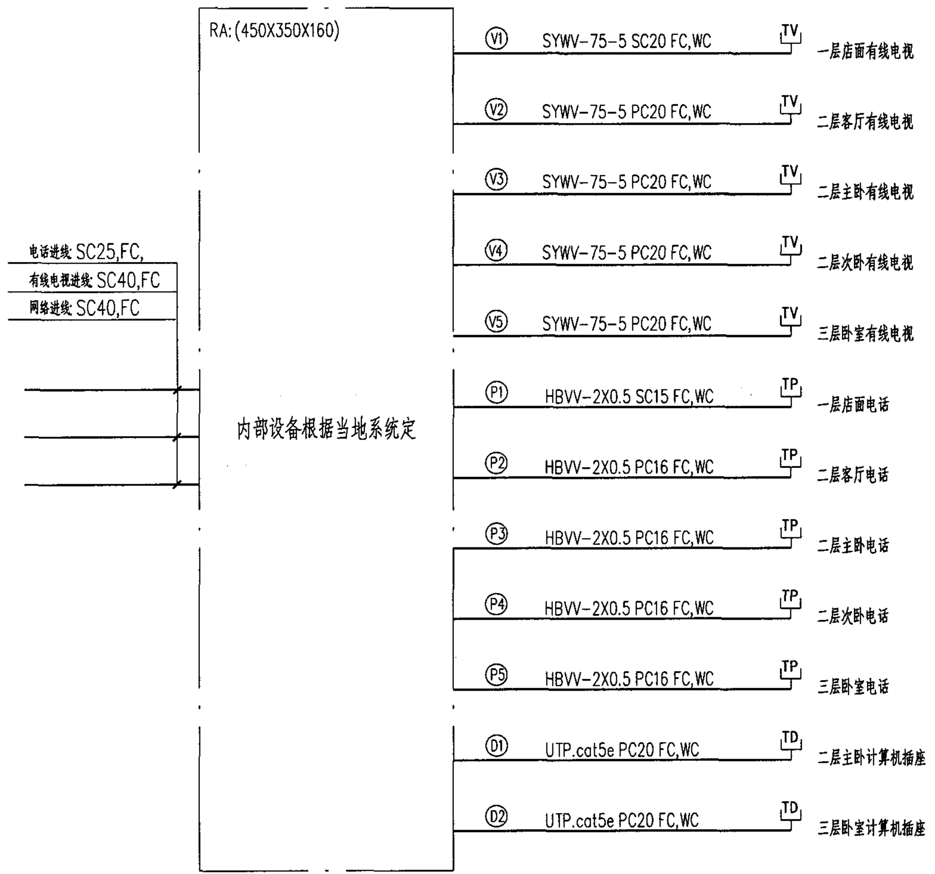
电话、有线、网络布线系统图
