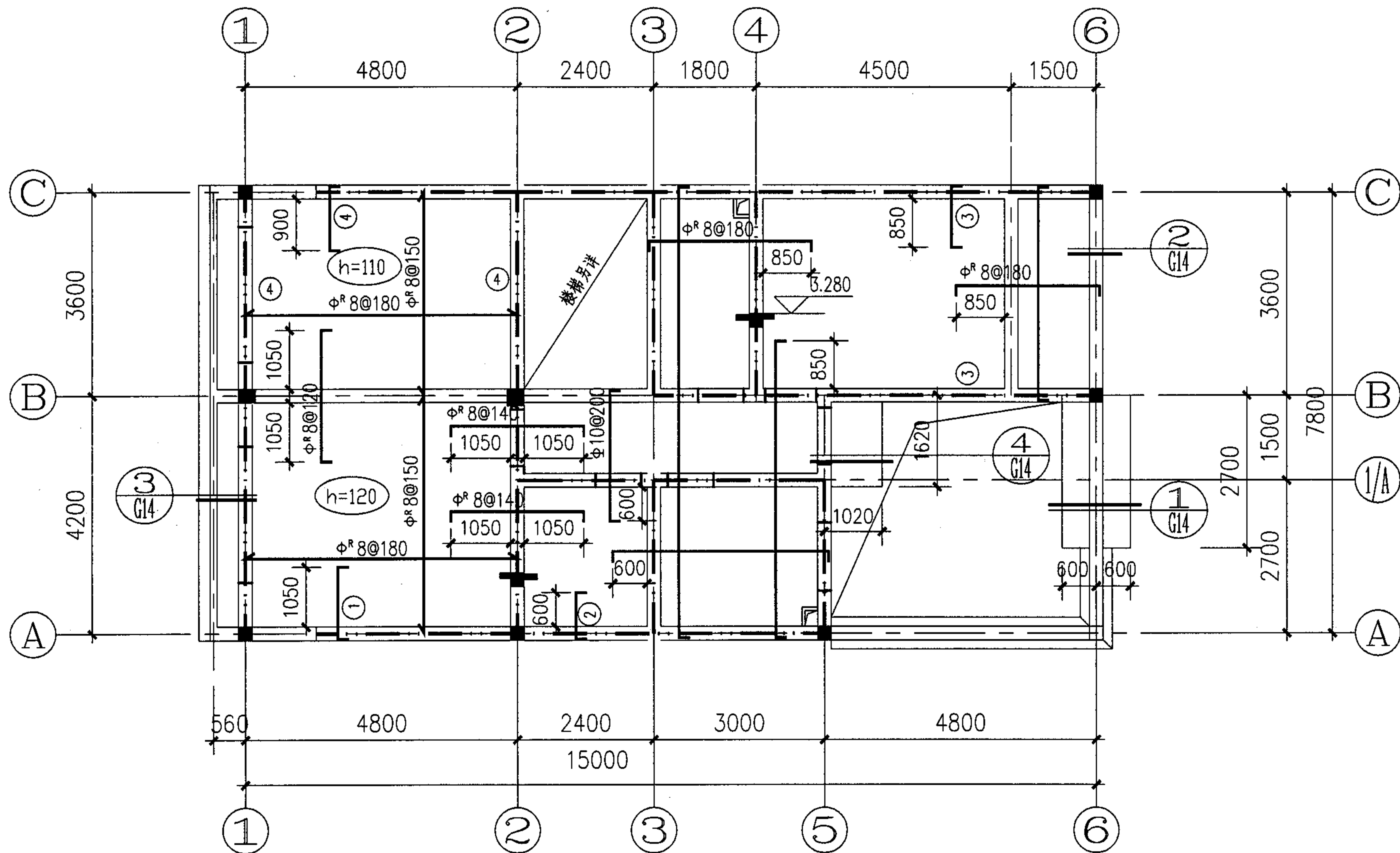
3. 280层结构平面布置图
