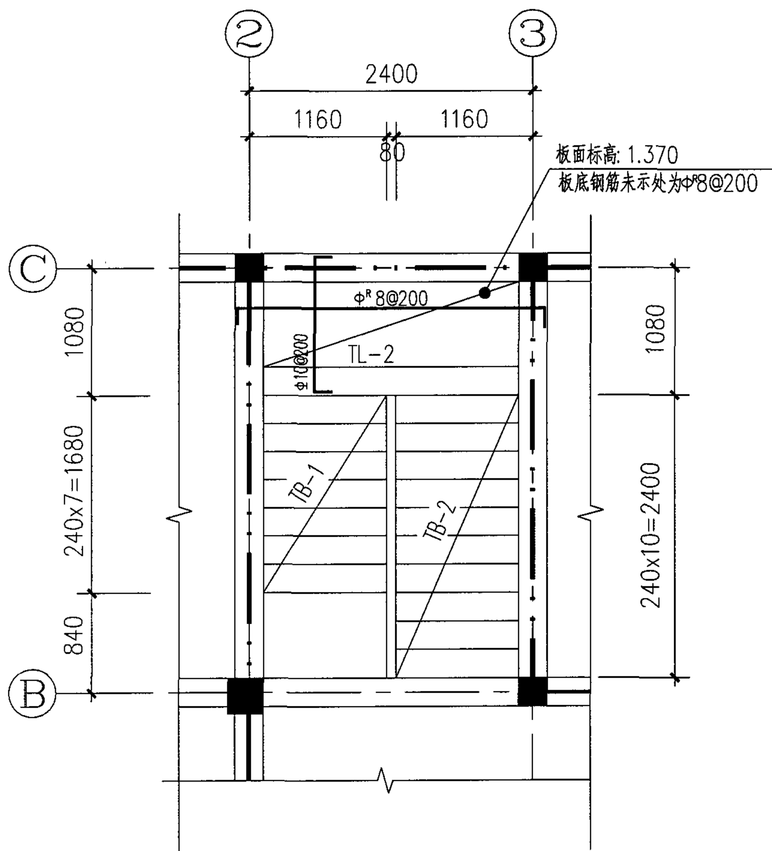
二层楼梯结构平面图
