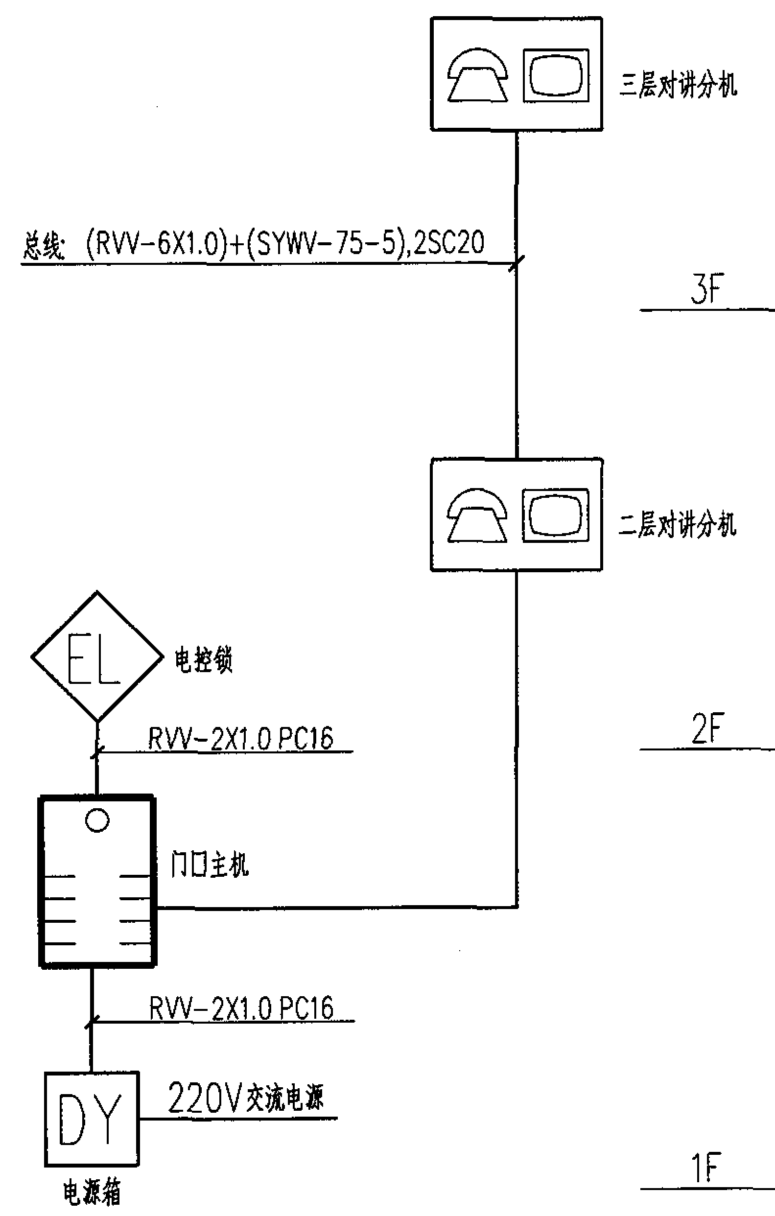
访客对讲系统图
