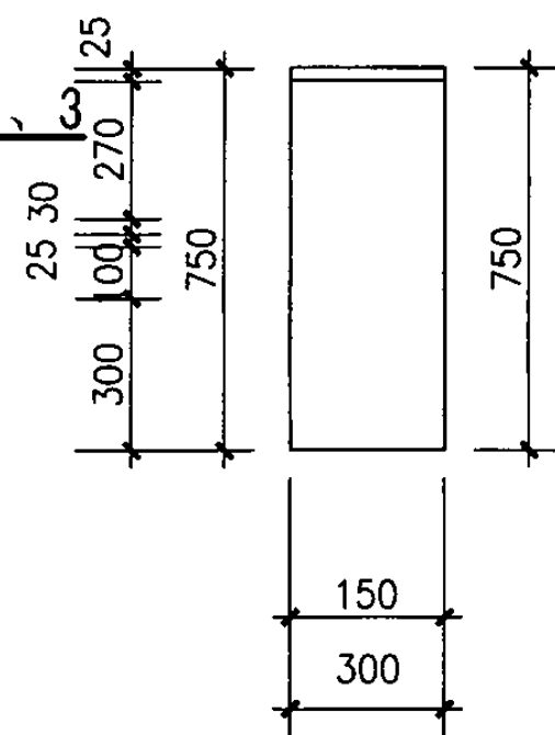
侧立面图
