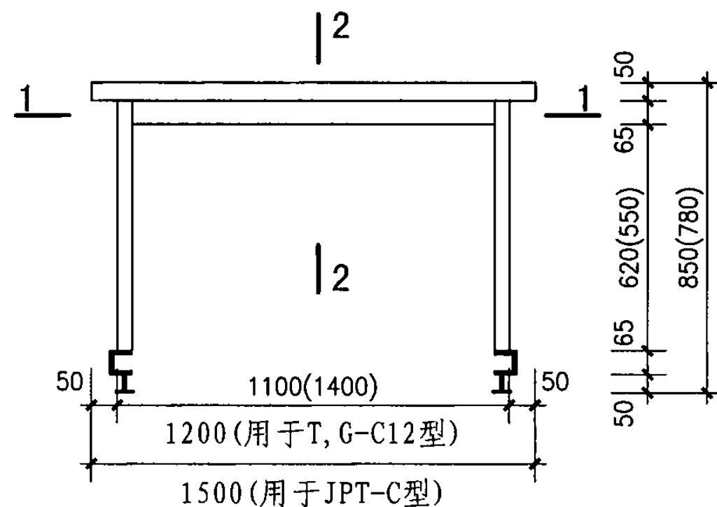
正立面图
