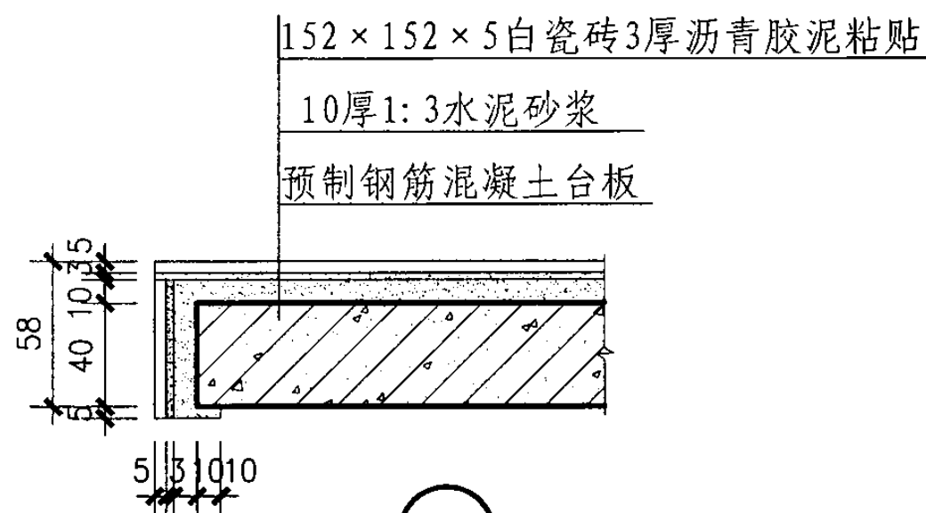
TF-C型单台板
