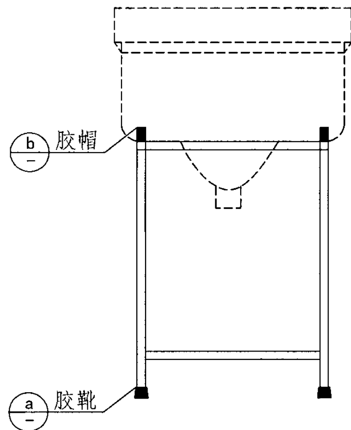
正立面
