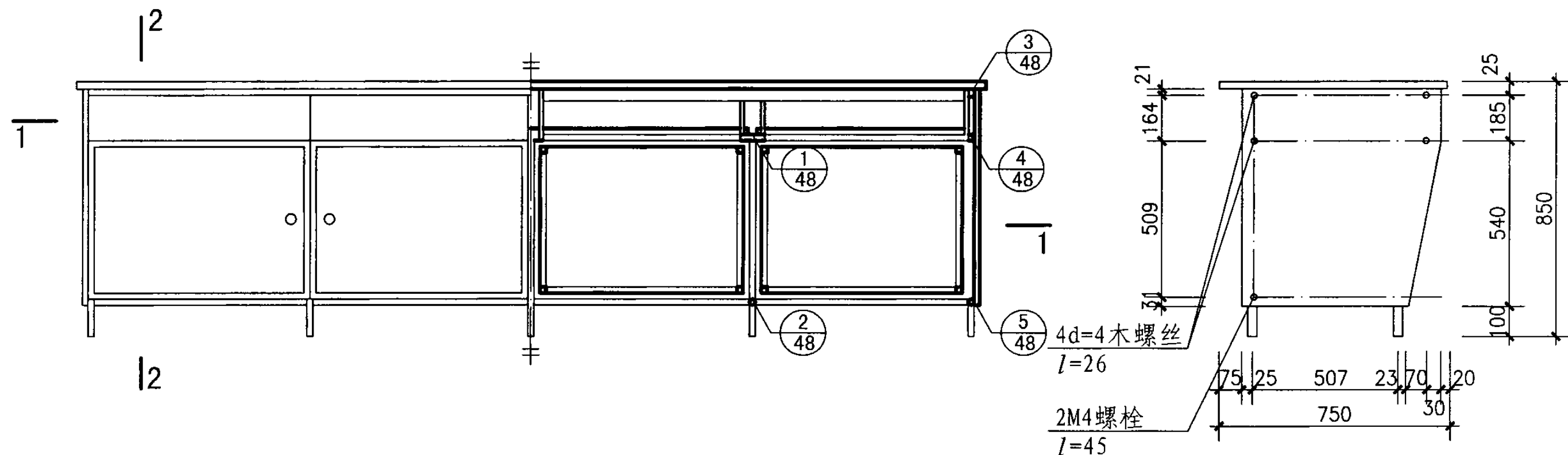
立剖面图
