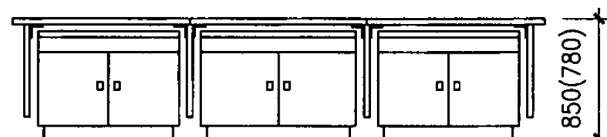
S、T-B36型立面图
