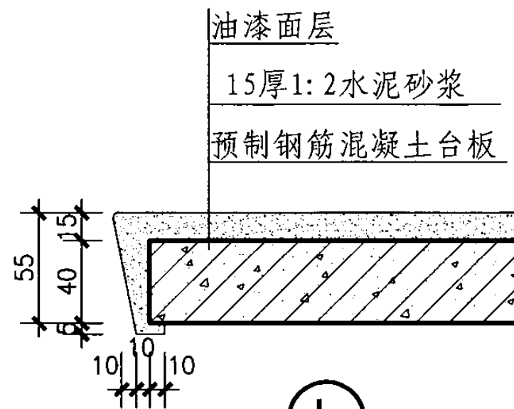
TF-A、B组合式中间台板
