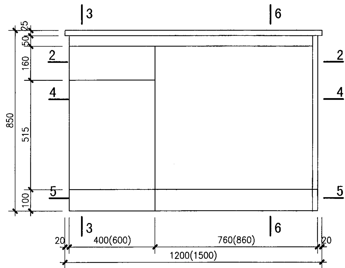
正立面图
