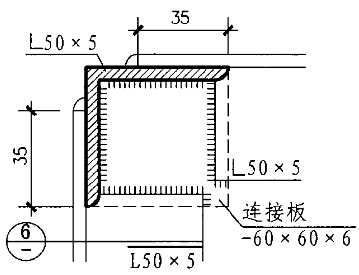
基架组合图
