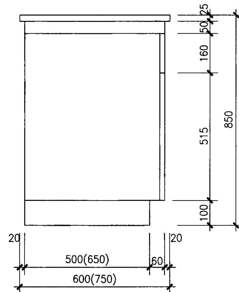
侧立面图
