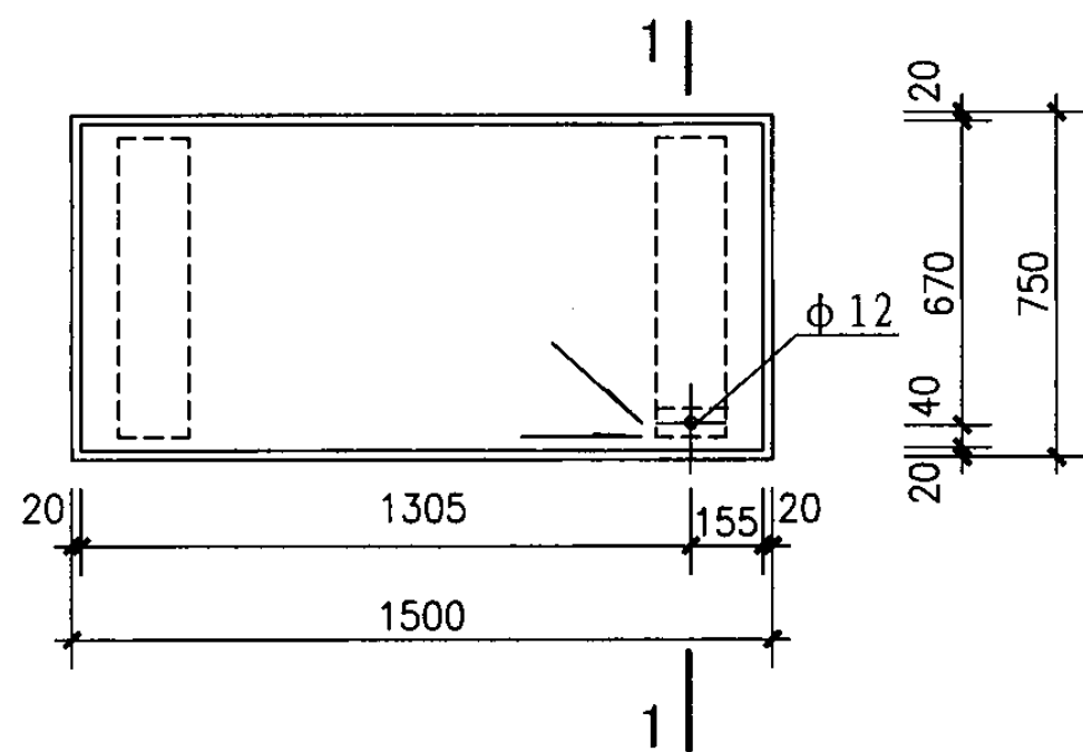
平面图
