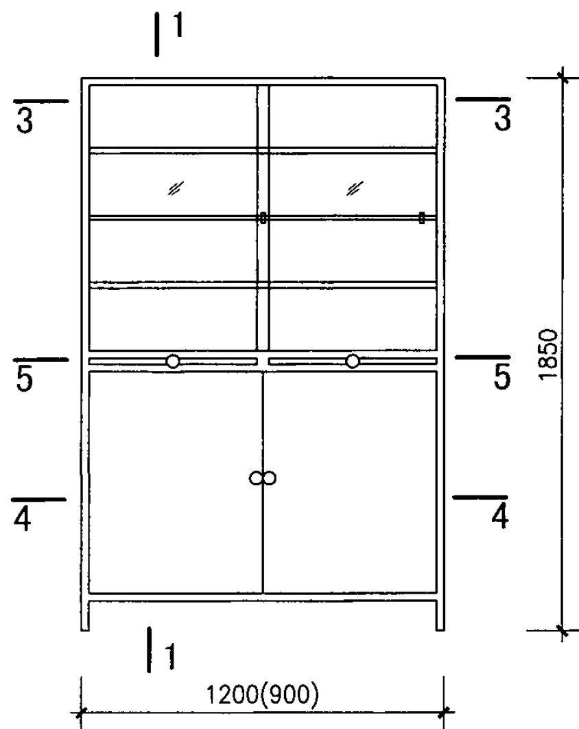
立面图
