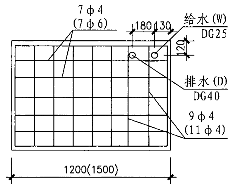
TF-A、B组合式中间台板
