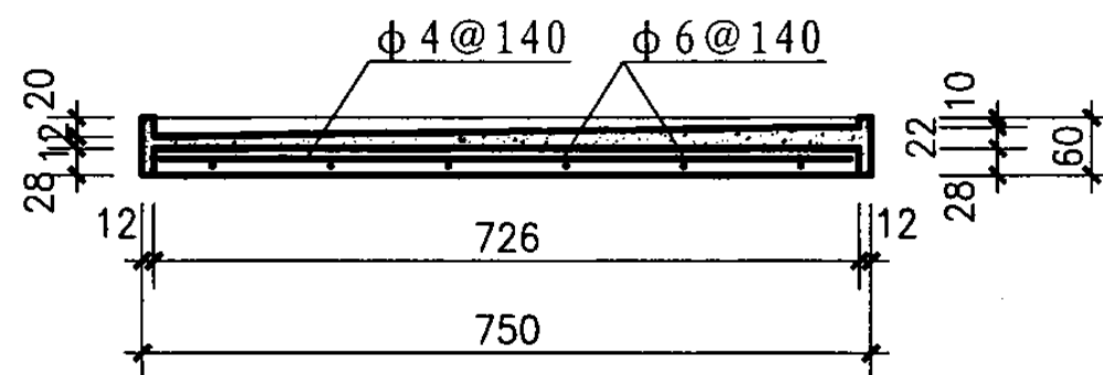
台板配筋图
