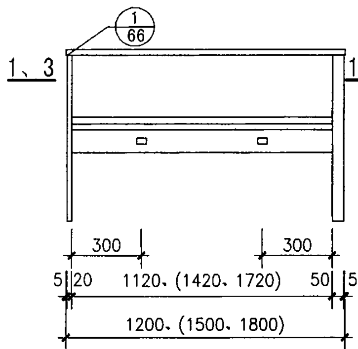
正立面图
