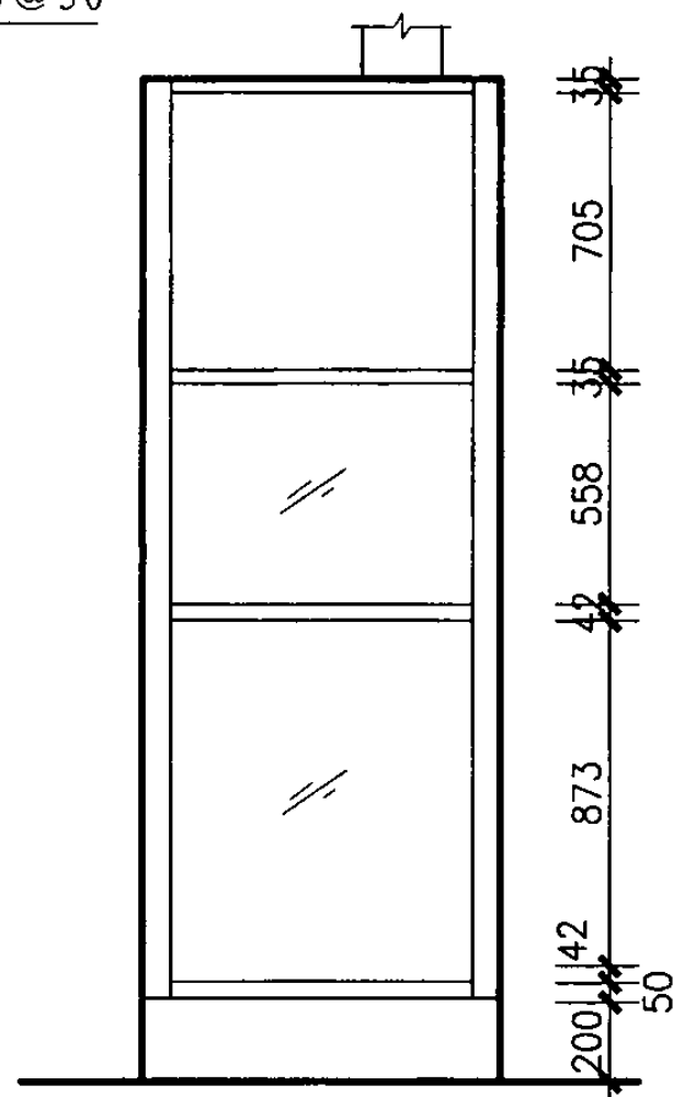
侧立面图
