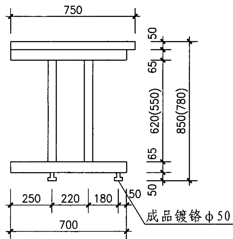
侧立面图
