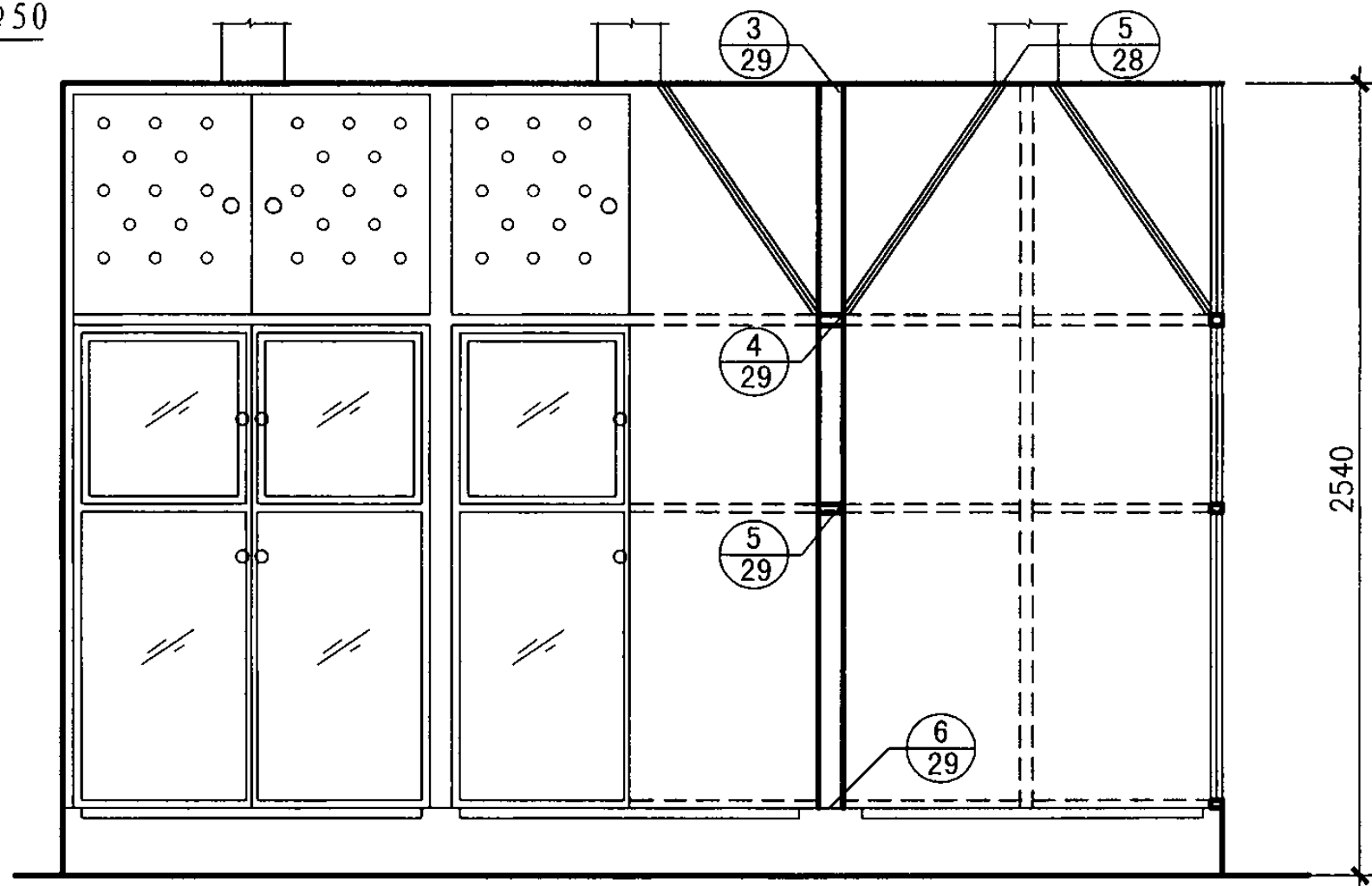
TF-E 36型立面图
