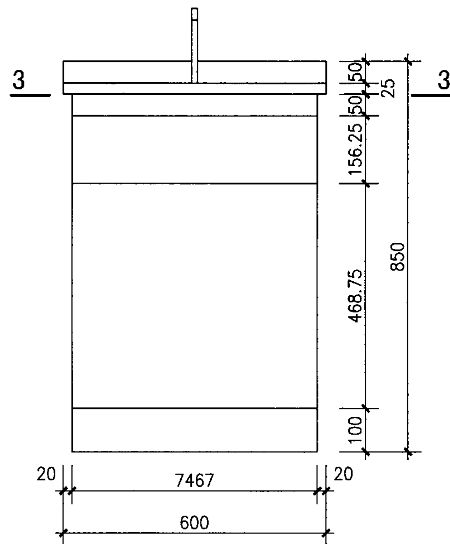
侧立面图
