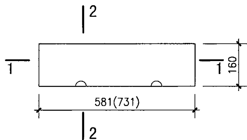
抽屉立面图
