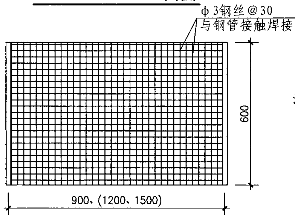
B09、B12、B15立面图
