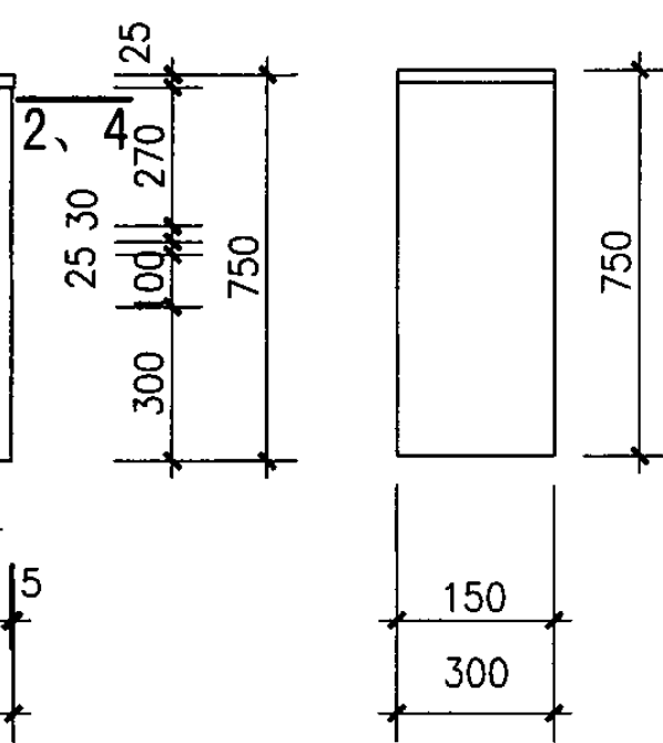
侧立面图
