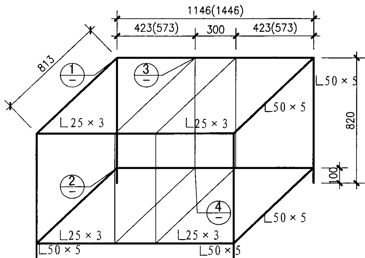
基架组合图
