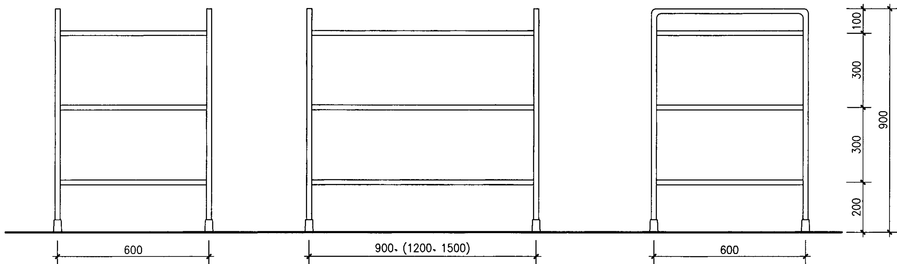
B09、B12、B15立面图
