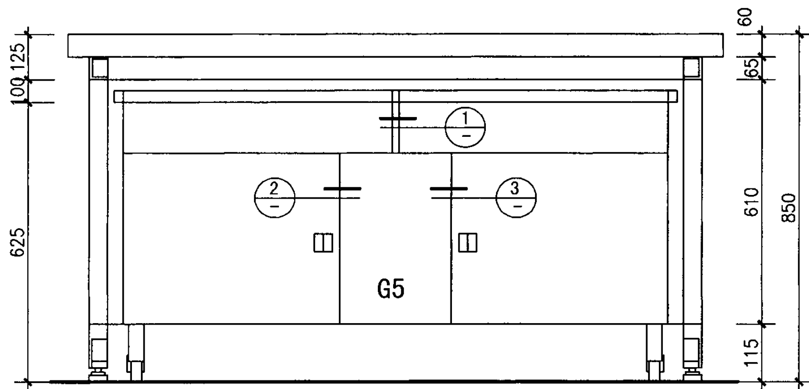
JPT-C型立面图
