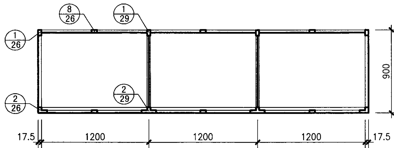
TF-E 36型平面图
