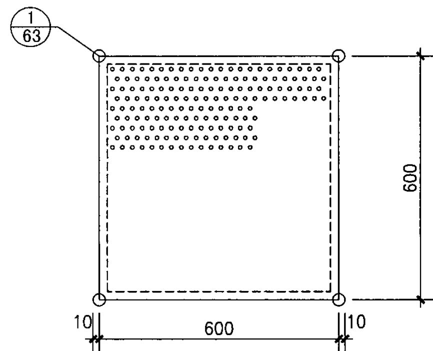
A06立面图
