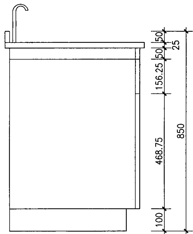
立面图
