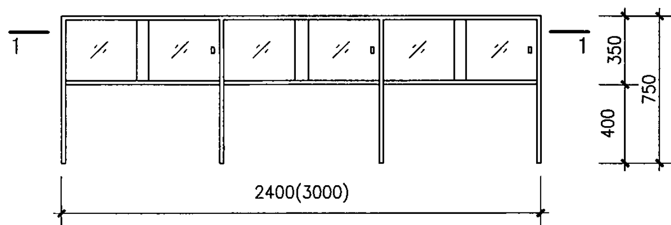
SJJ-E24a、b, E30a、b型立面图
