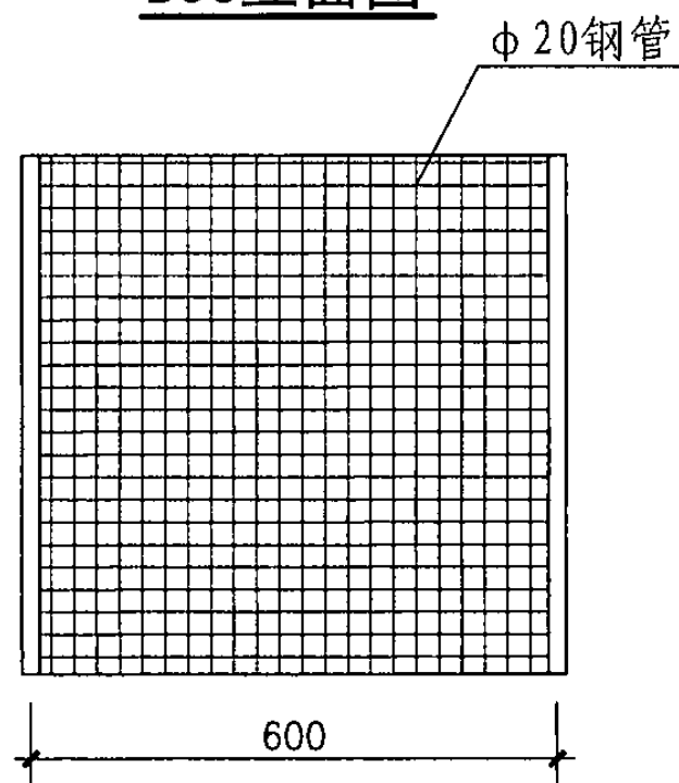
B06立面图
