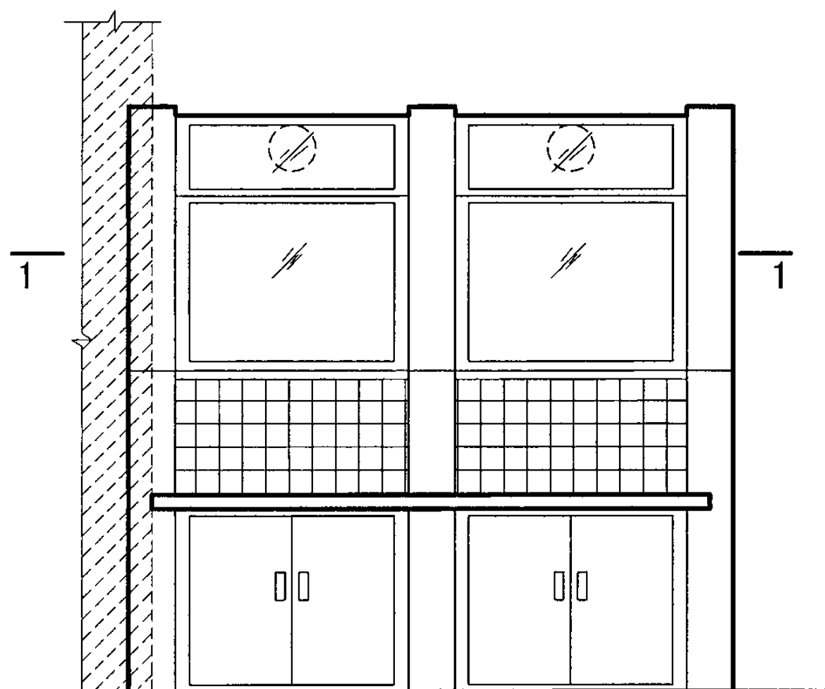
TF-A 24立面图
