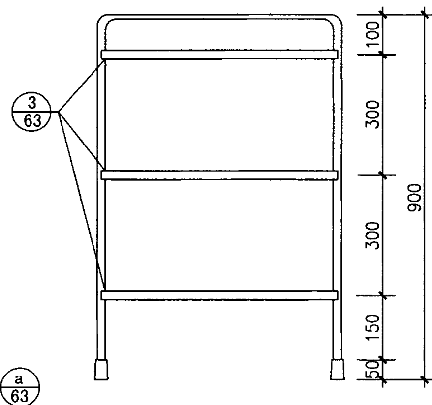
侧立面图
