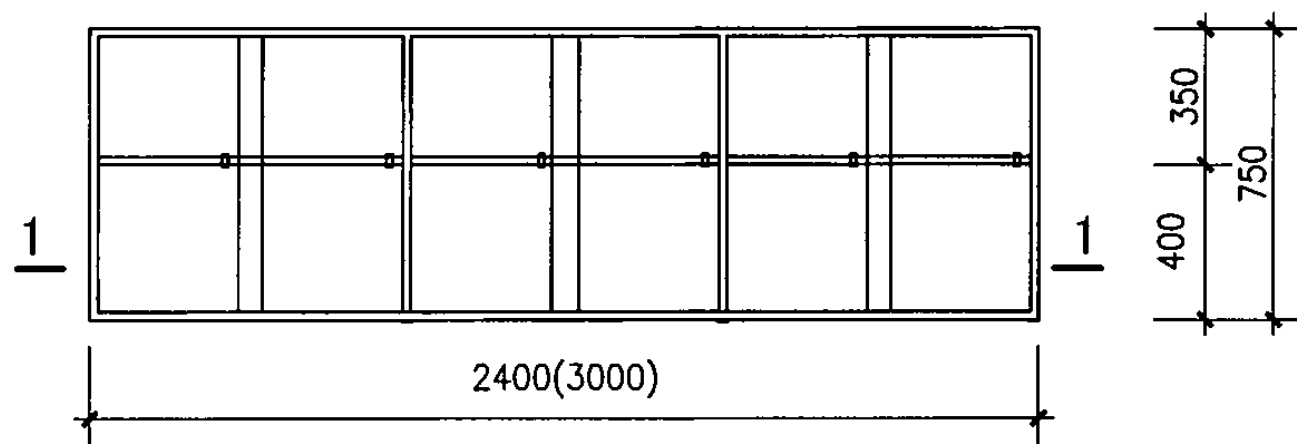
SJJ-F24a、b, F30a、b型立面图
