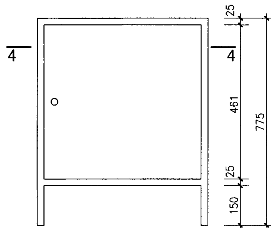
D型柜立面图
