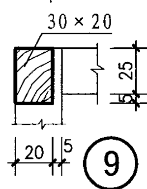
YPG-D 型药品柜节点详图
