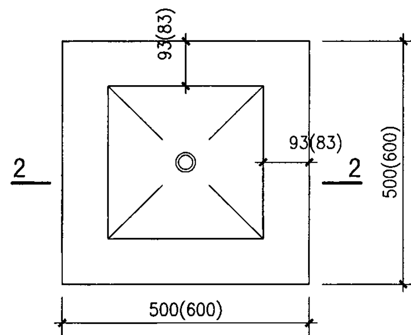
B05、B06型平面图
