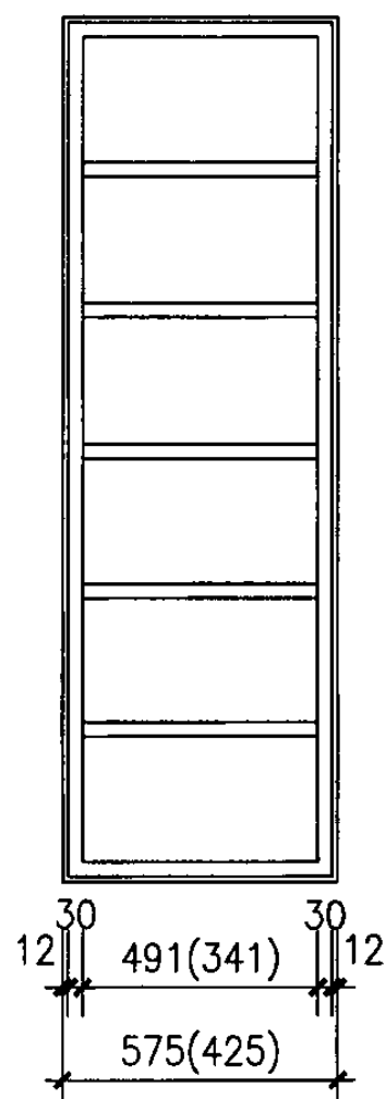
门骨架图
