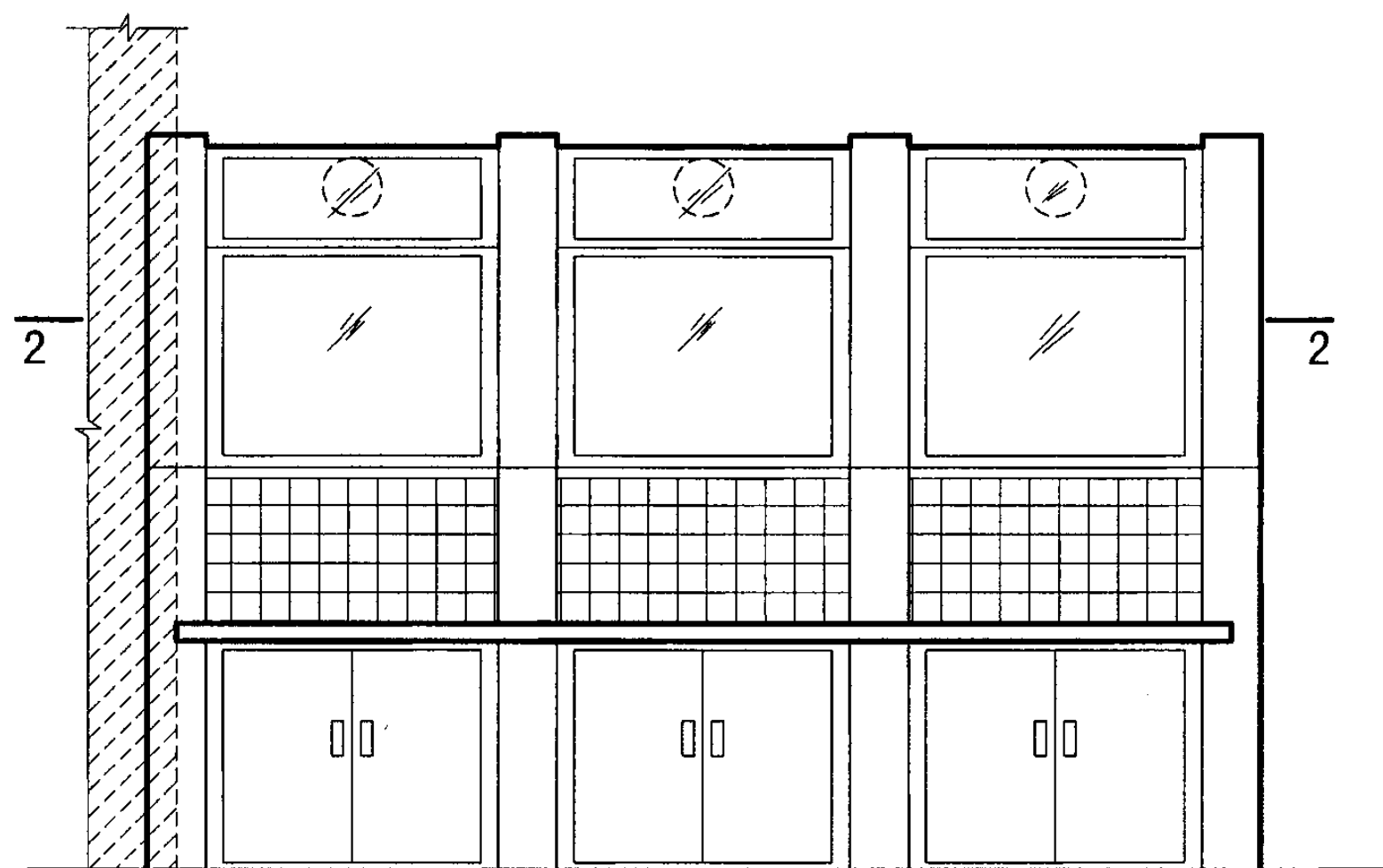
TF-A 36立面图
