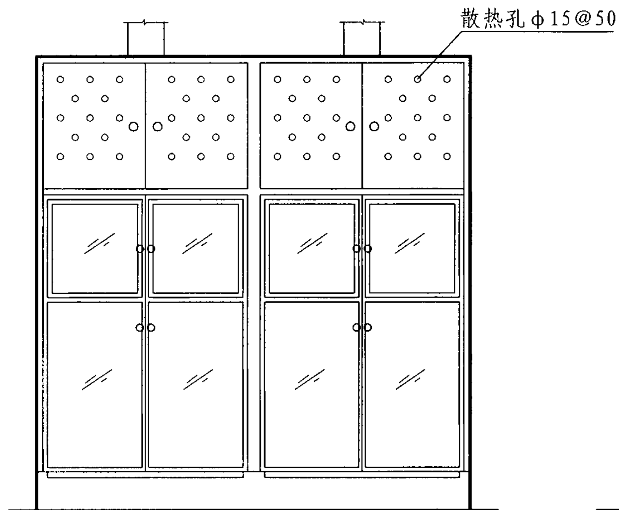
TF-E 24型立面图
