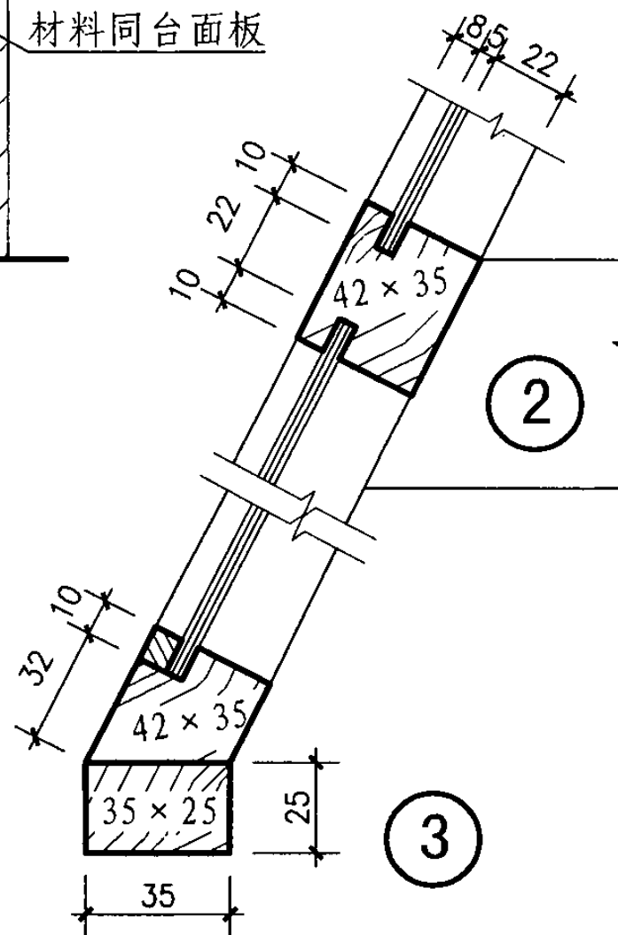
TF-B12型通风柜详图
