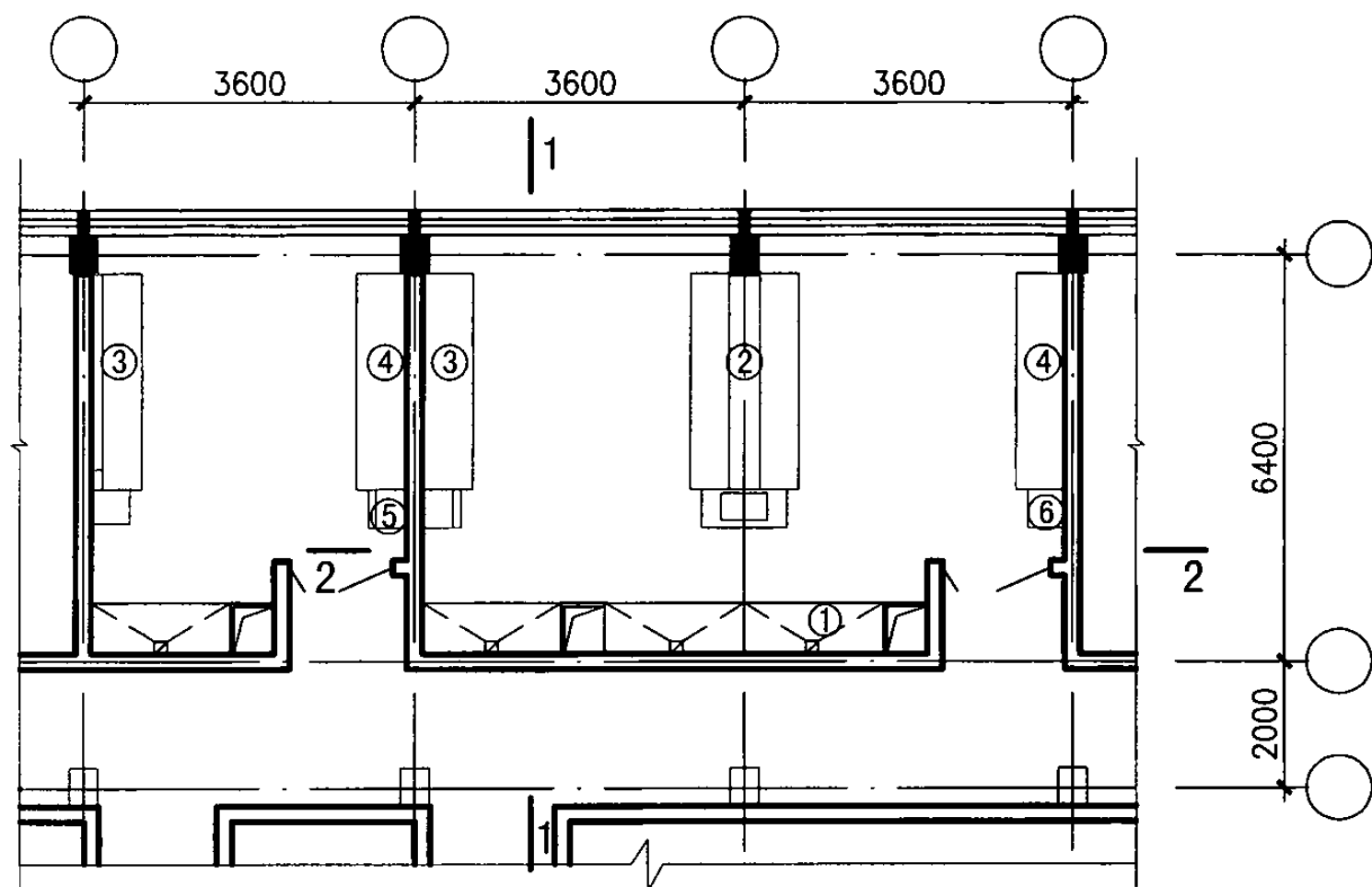
平面布置图
