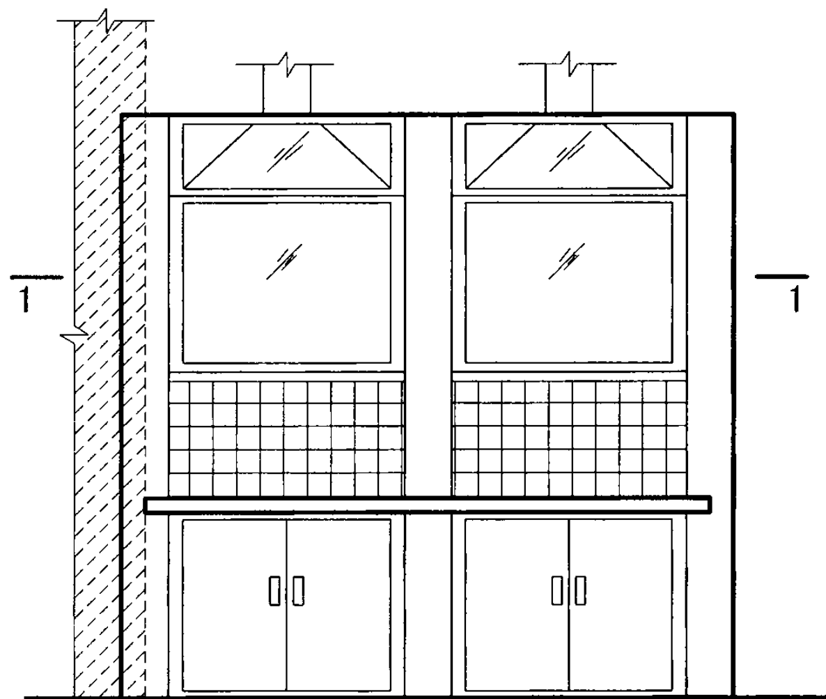
TF-B 24立面图
