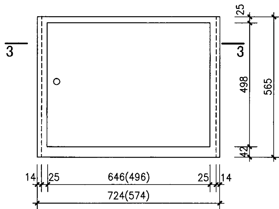
B24, B30型柜立面图
