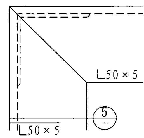
基架组合图
