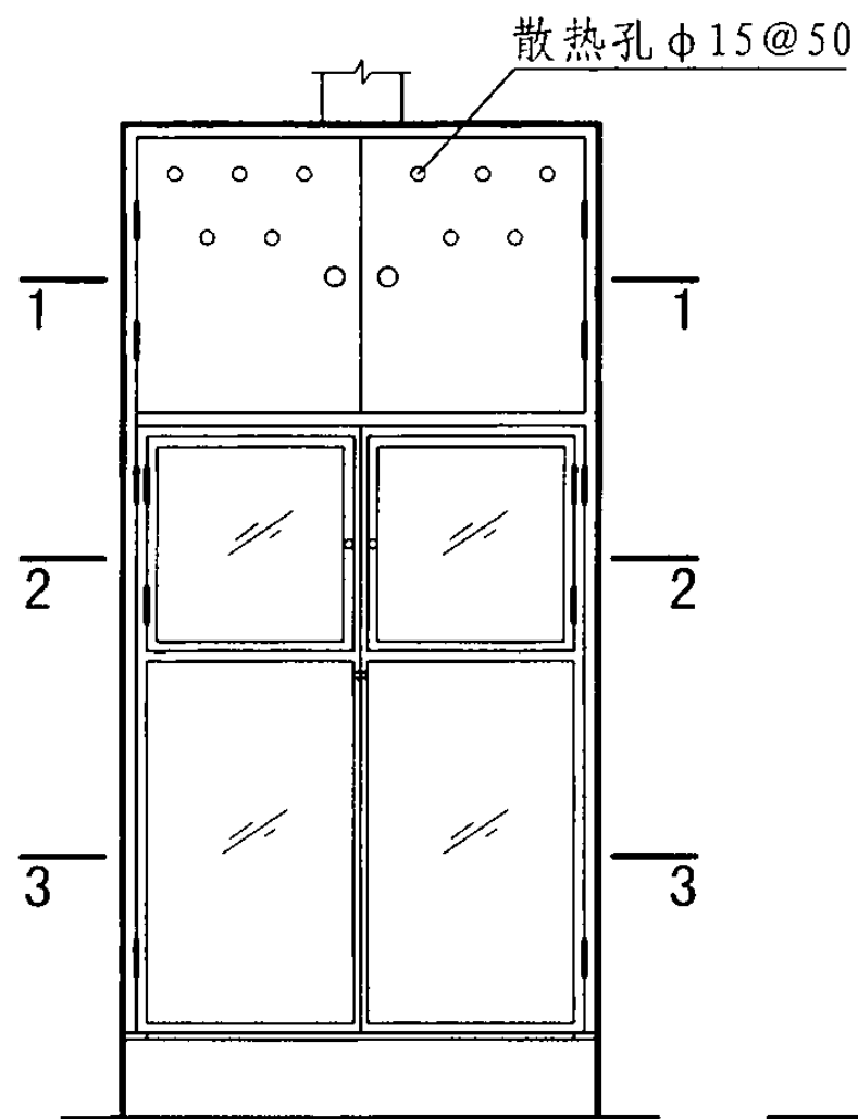
立面图
