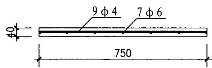
台板配筋图
