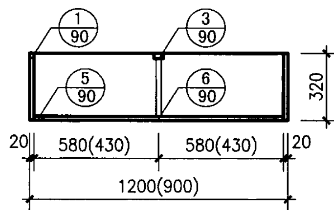
侧立面图
