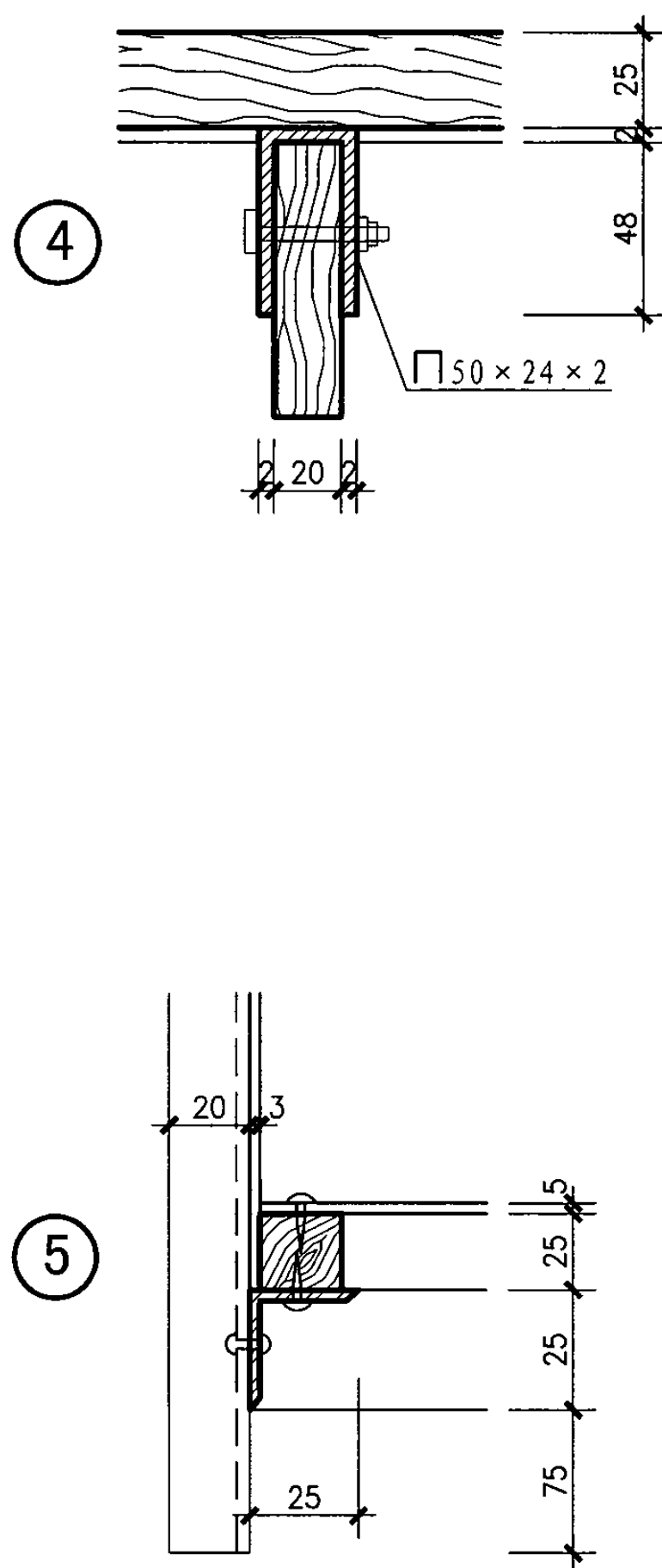
SYT-a、b、c、d型实验台节点详图 (一)
