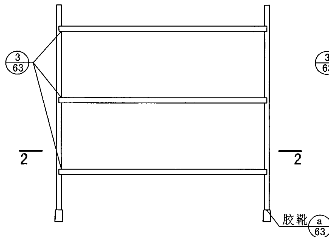
A09、A12、A15立面图
