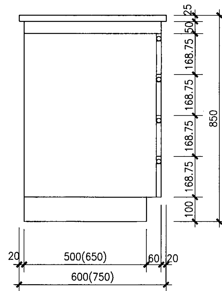
侧立面图
