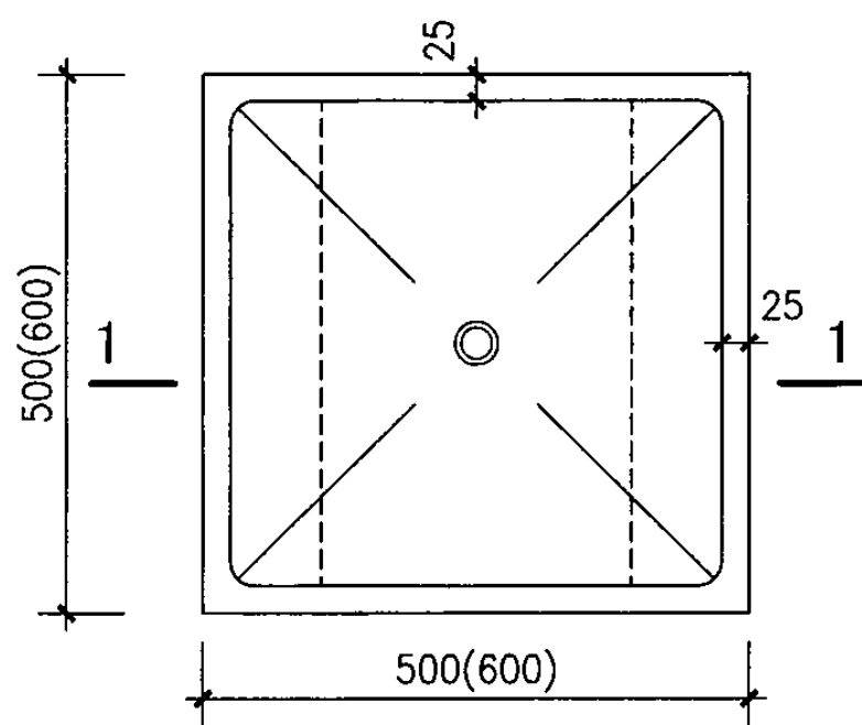
A05、A06型平面图
