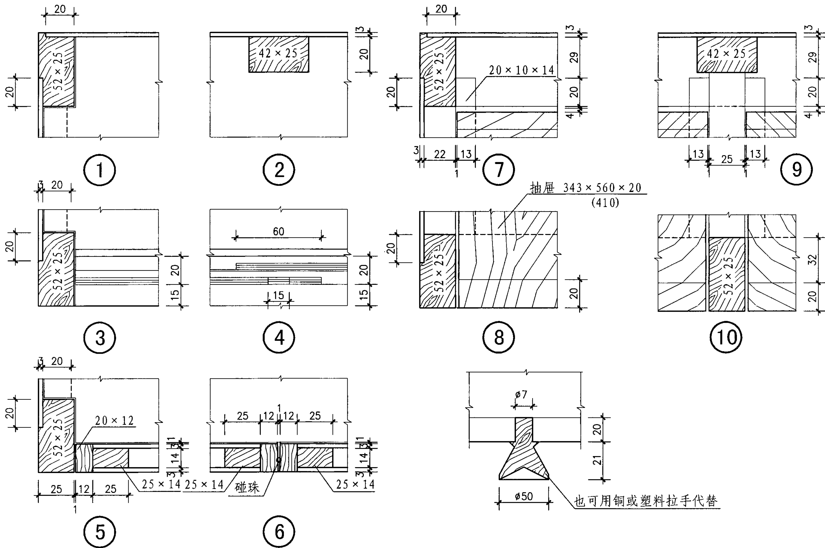
YPG-A、B、C型药品柜节点详图 (一)
