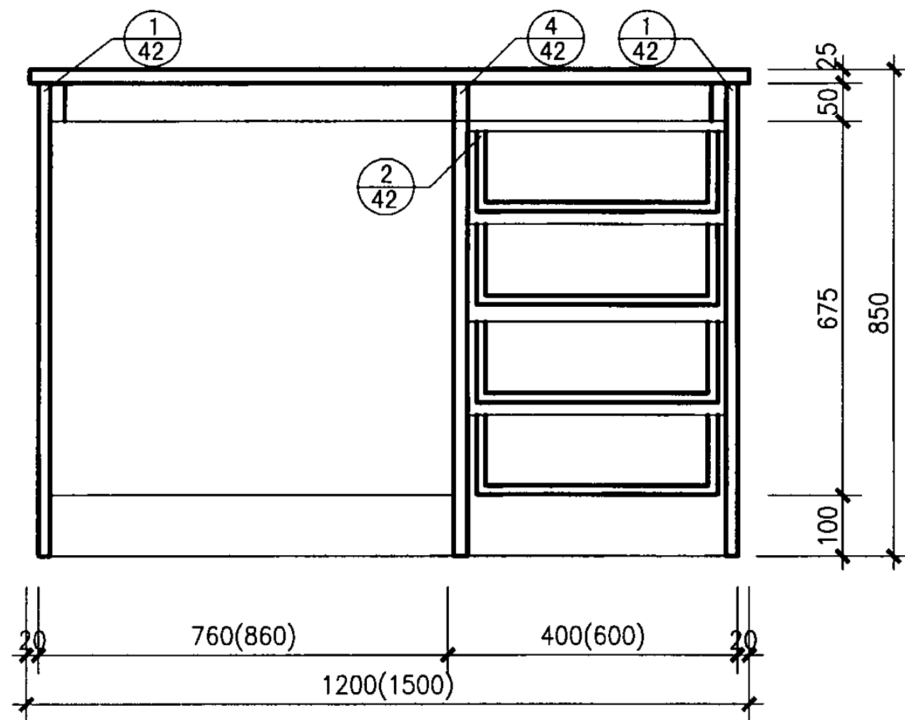
1-1
