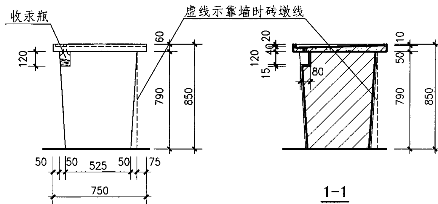
侧立面图
