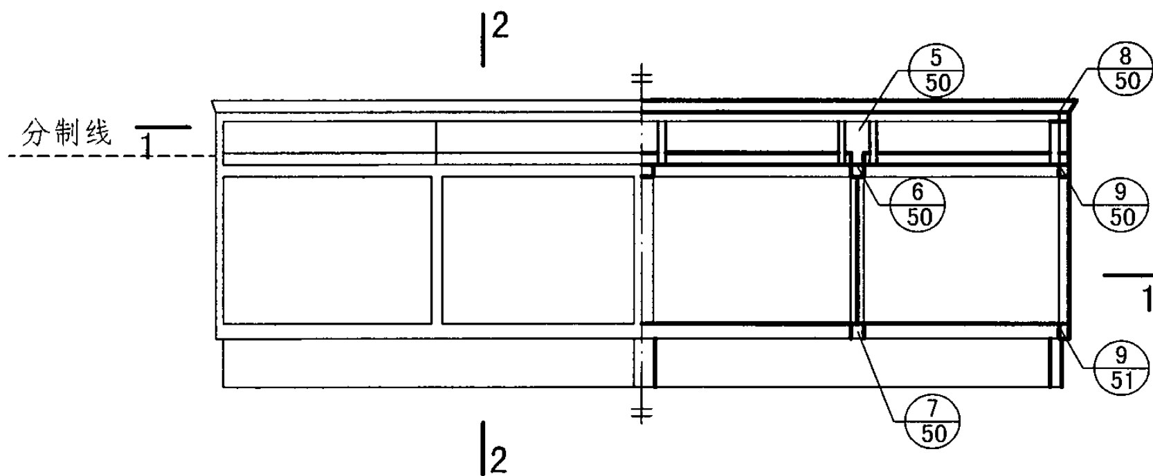
立剖面图
