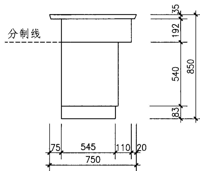
侧立面图
