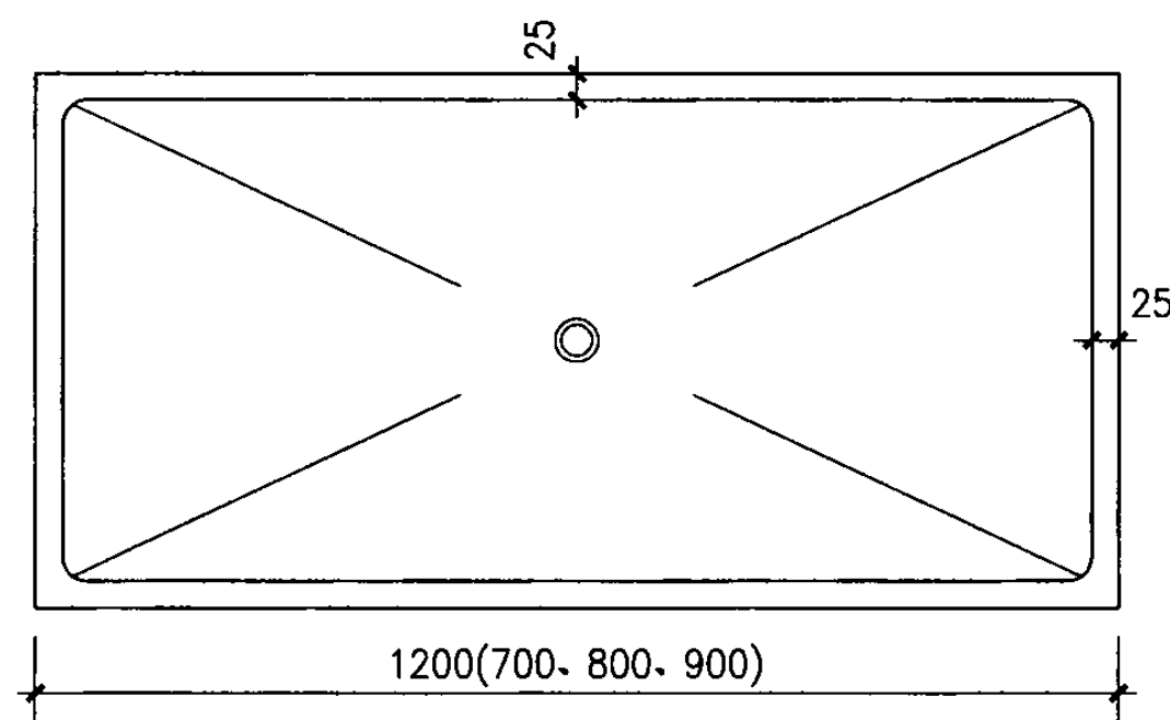
A07、A08、A09、A12型平面图
