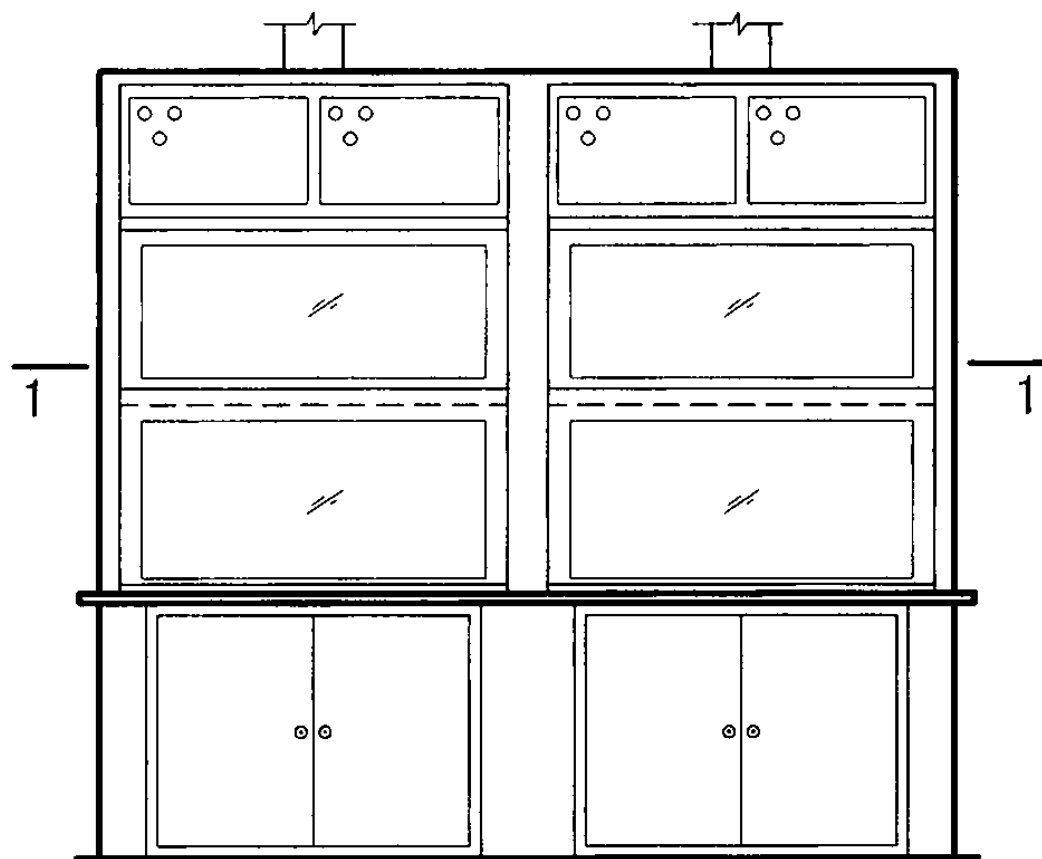
TF-C 24立面图
