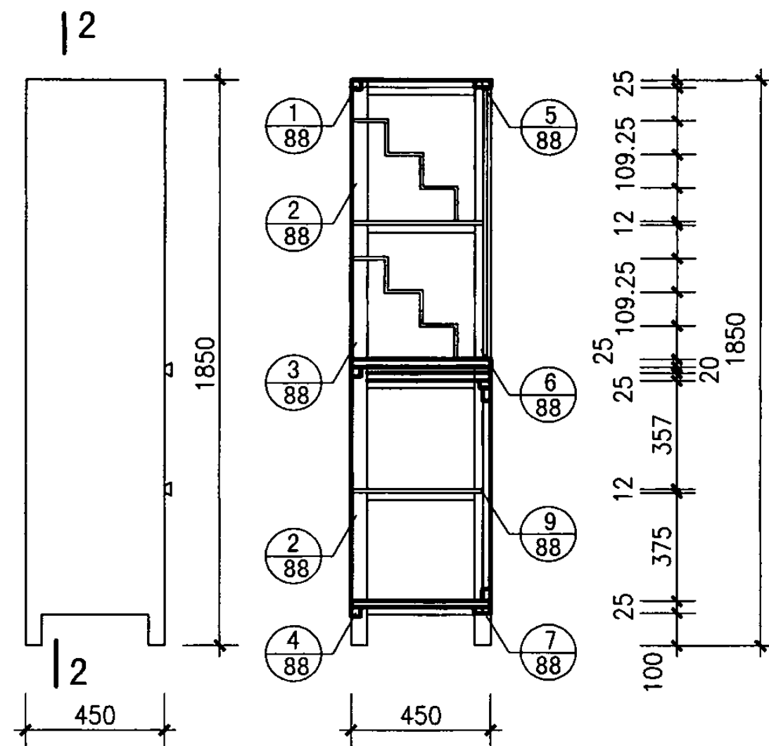
侧立面图
