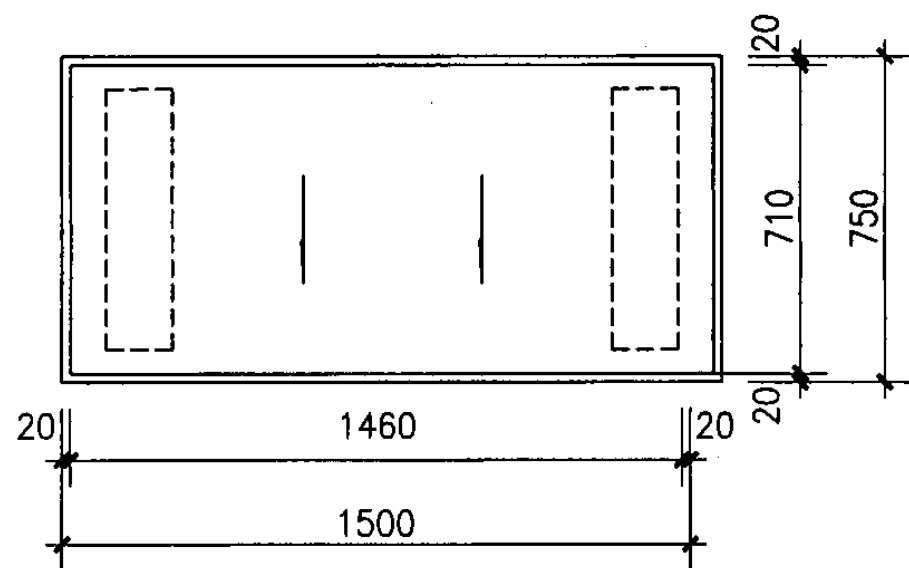
平面图
