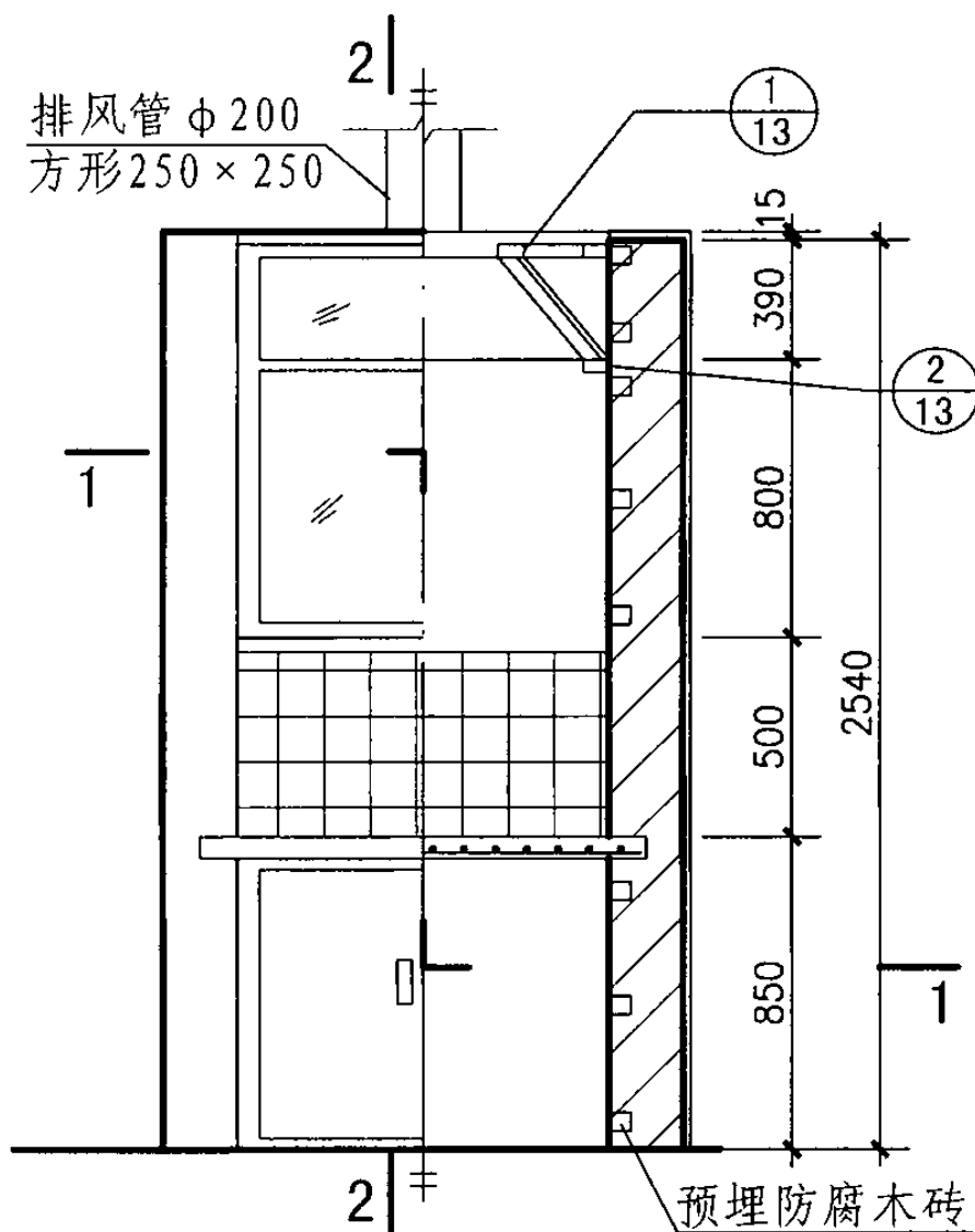
立剖面图
