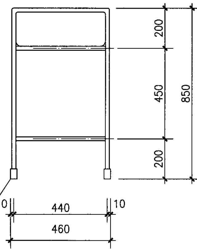
侧立面图
