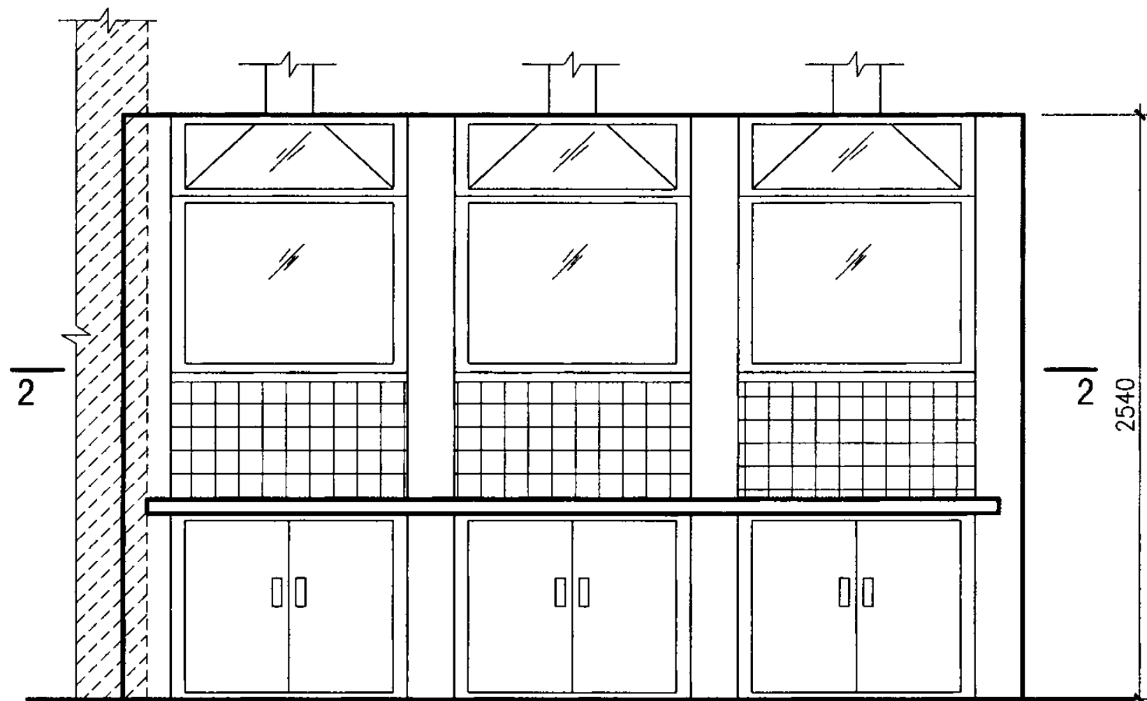
TF-B 36立面图
