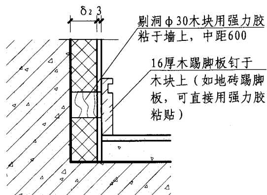
4 踢脚 (室内)
