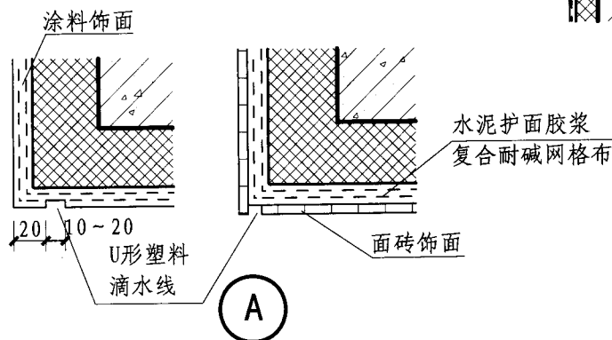
平窗口及滴水线
