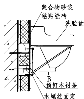
洗脸盆安装
