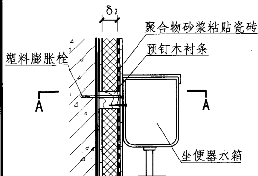
坐便器水箱安装
