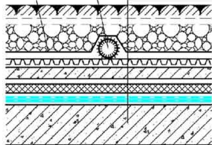
① 排水管与排水板组合排水 滤水管间距见具体工程设计
