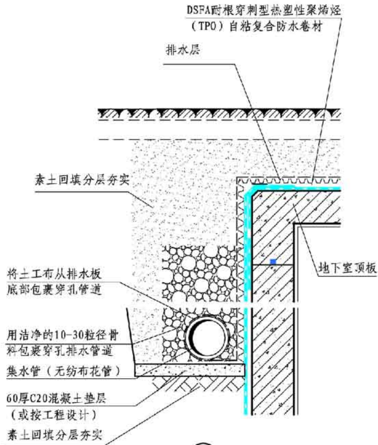
② 盲沟排水(二)
