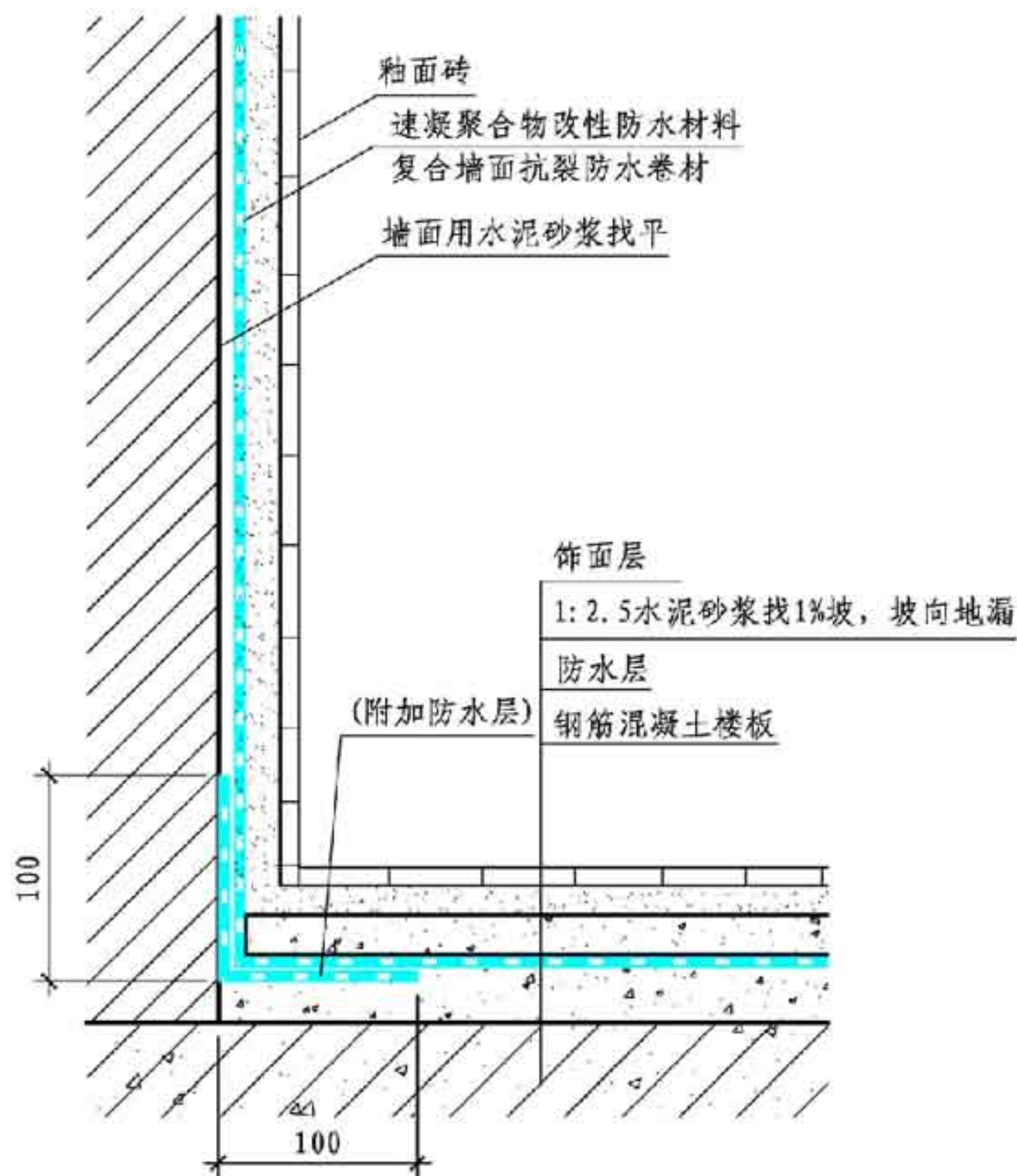
① 厕浴间墙地面防水做法
