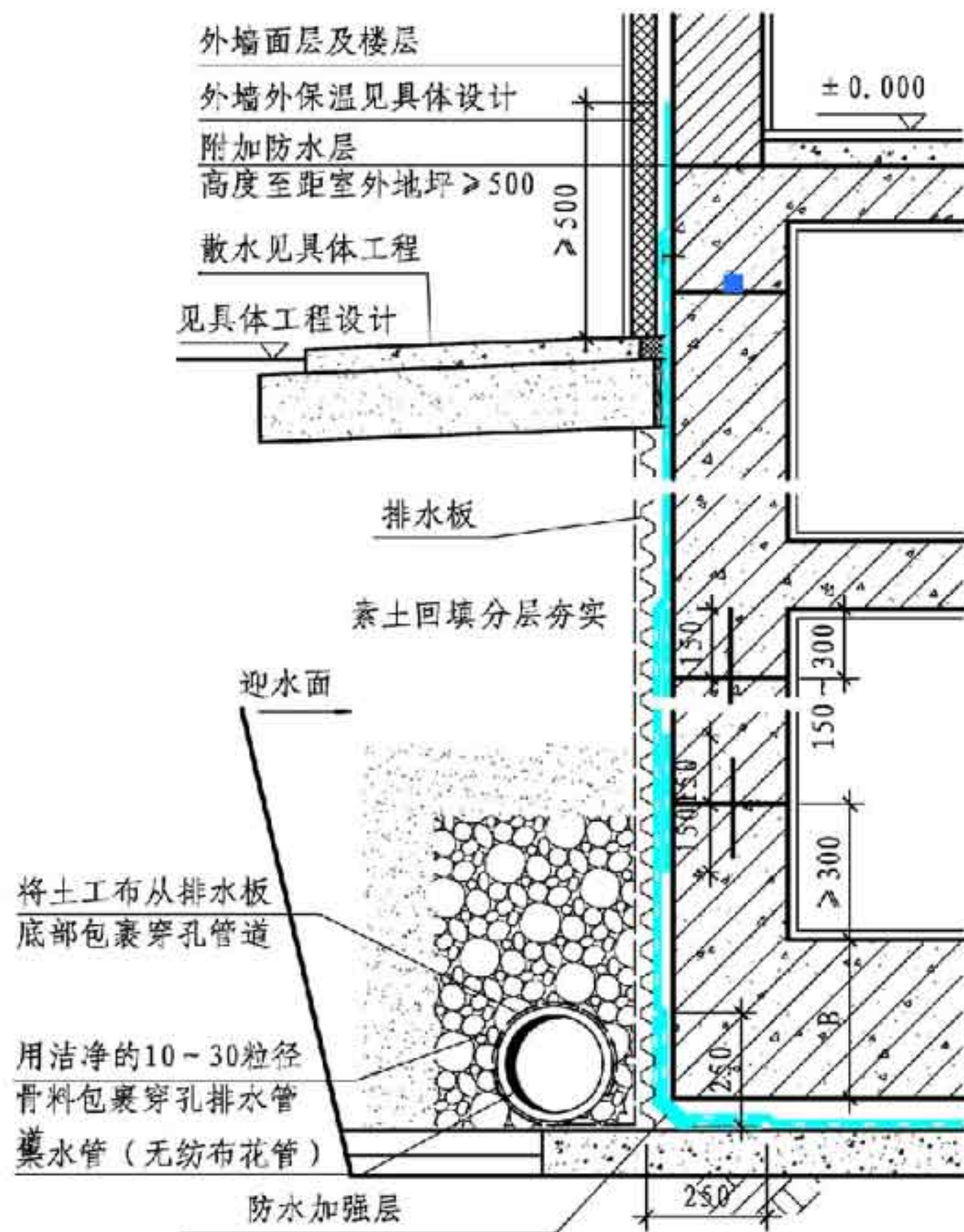
① 盲沟排水(一)
