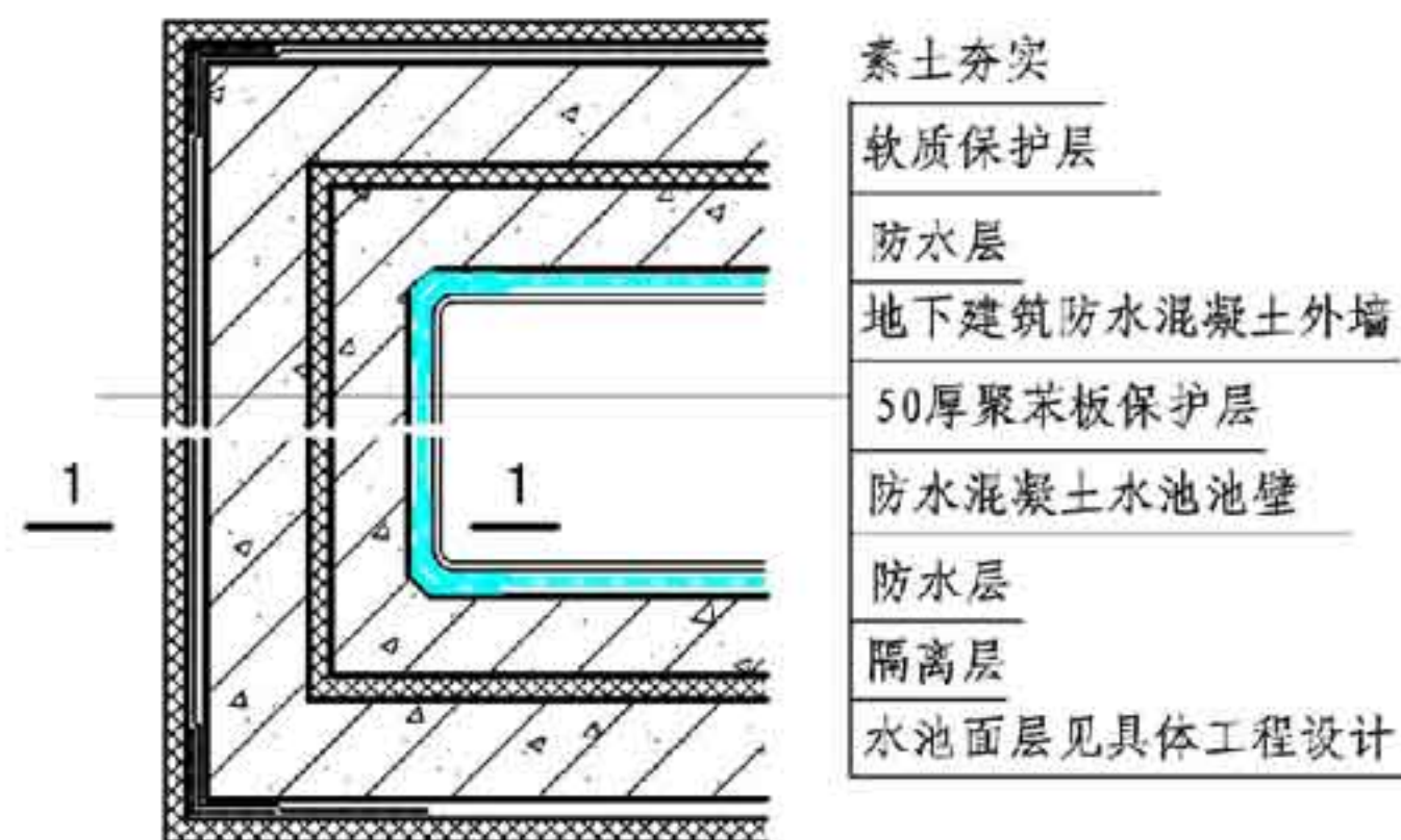
② 地下水池平面图
