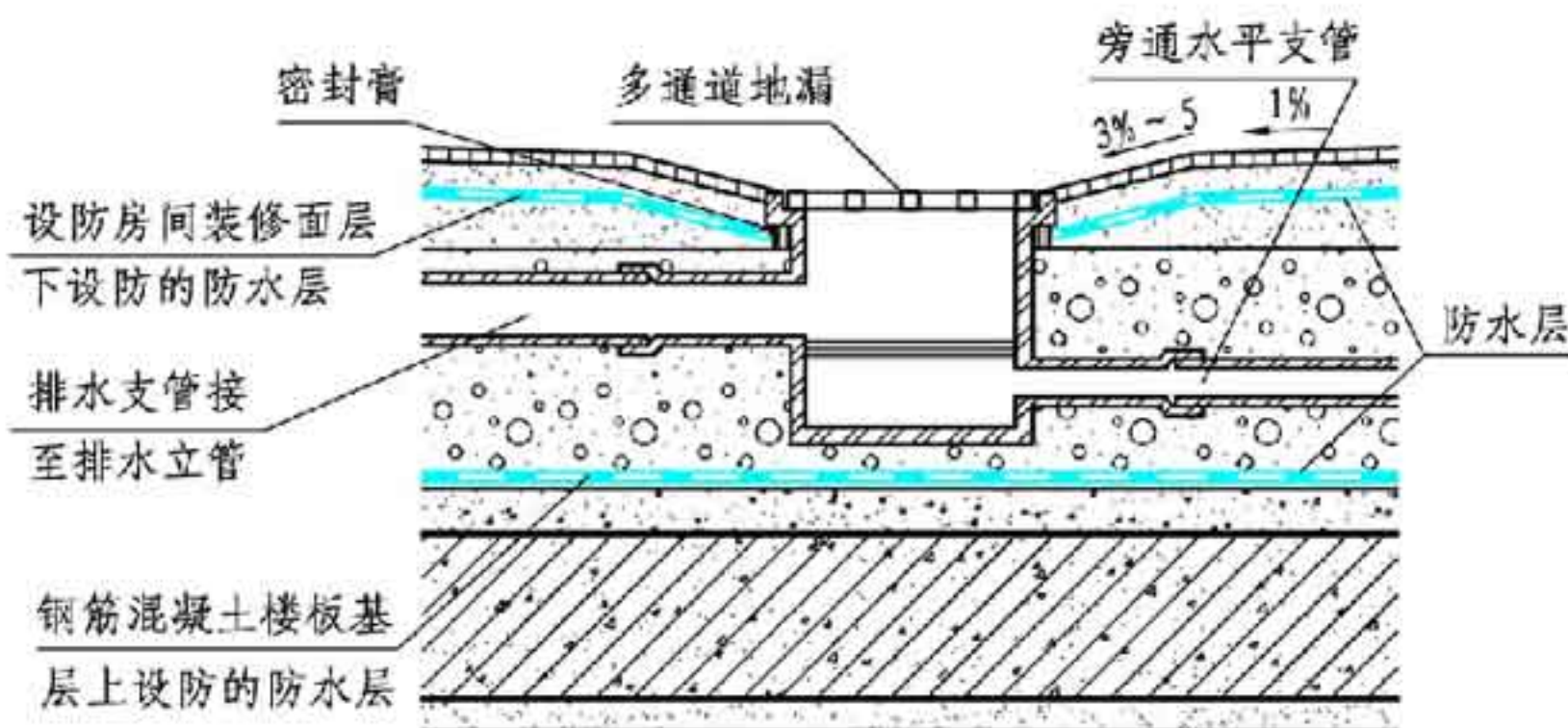
② 同层排水时的地漏防水构造
