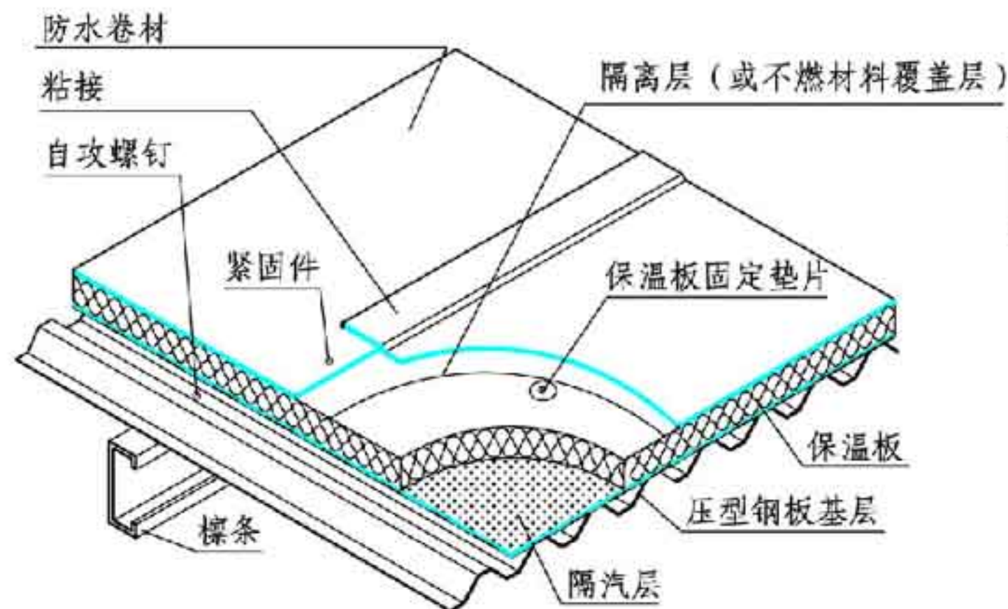
压型钢板屋面防水构造示意图
