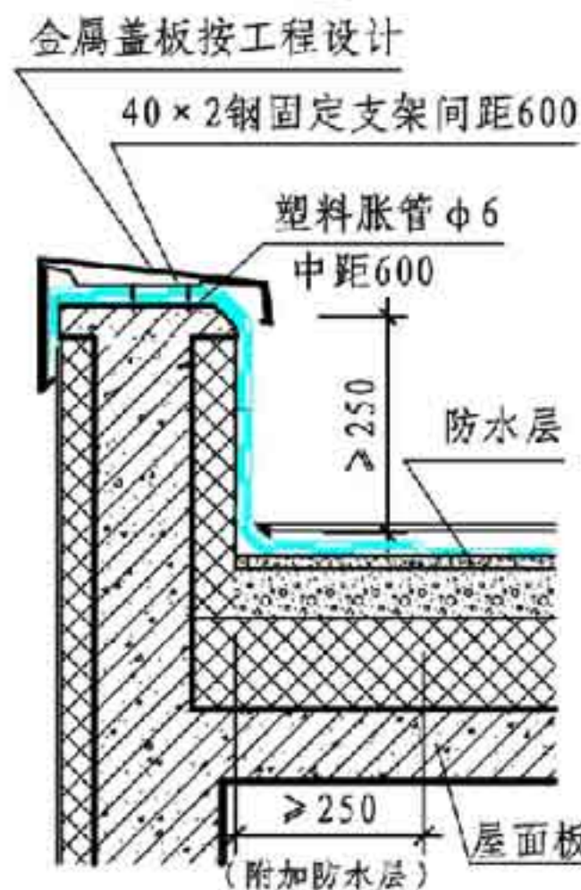
③ 女儿墙(二)
