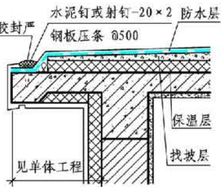
② 檐口
