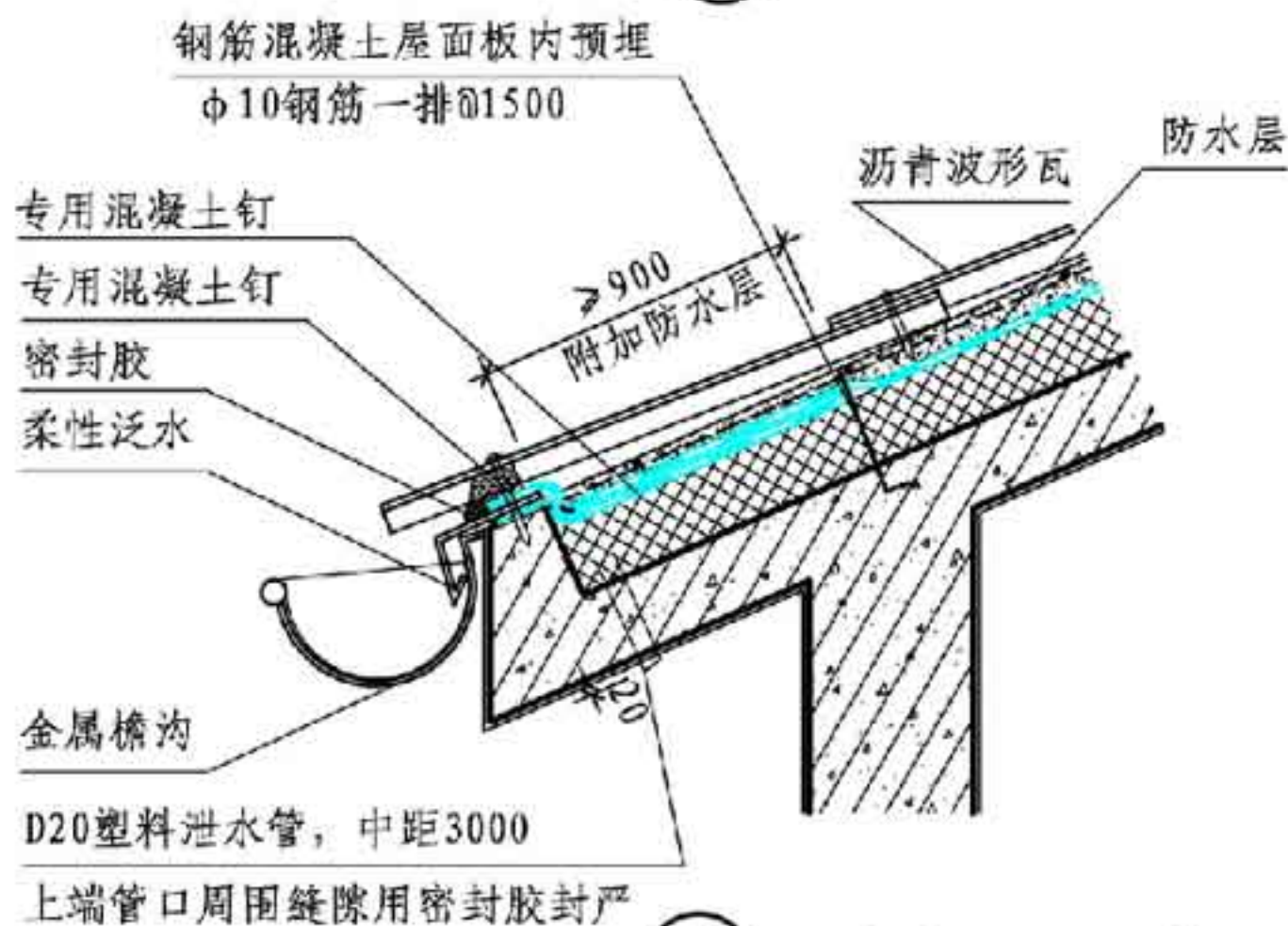
② 沥青波形瓦屋面檐口
