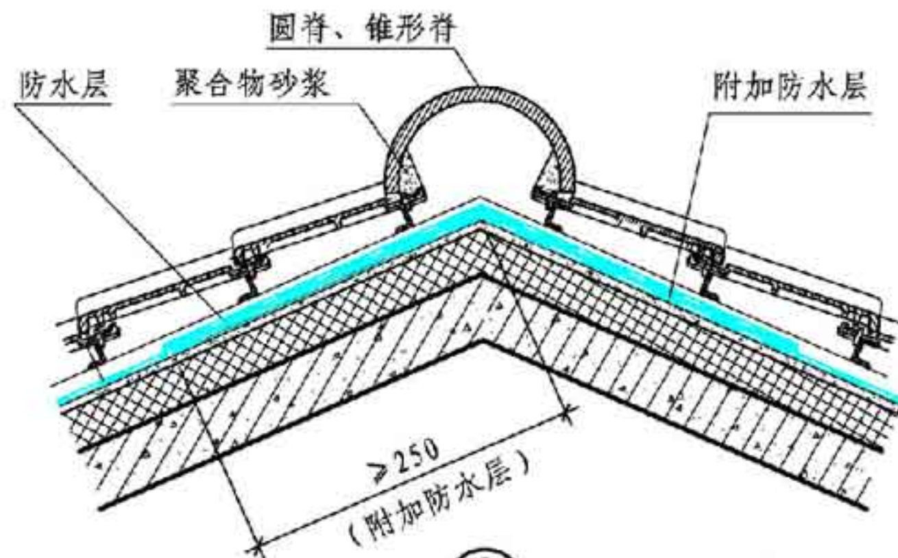
③ 平瓦屋面屋脊
