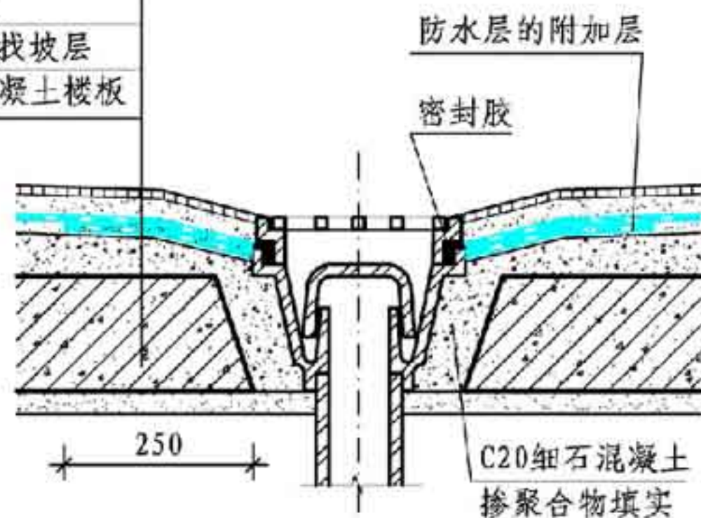
① 地漏防水构造
