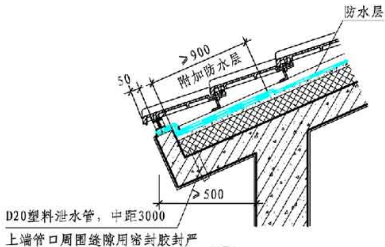
④ 平瓦屋面檐口
