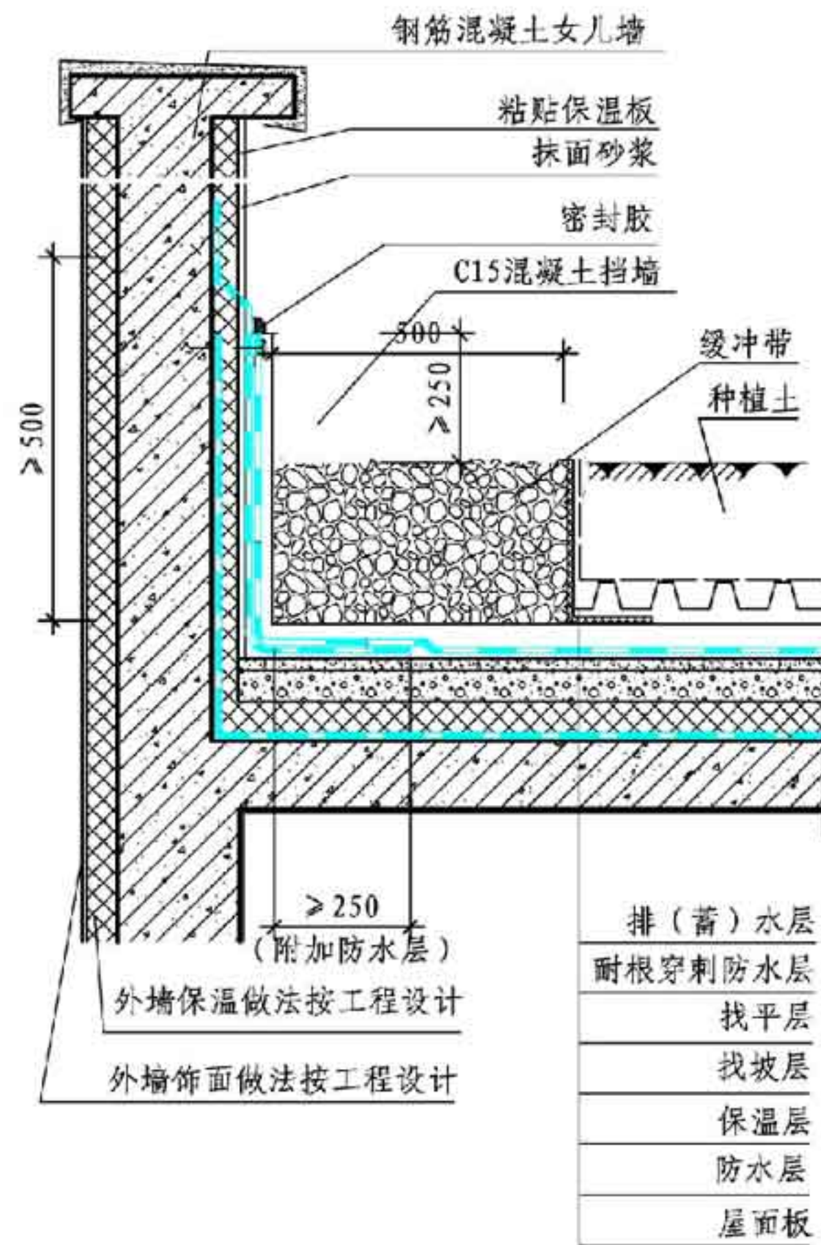
④ 种植屋面女儿墙
