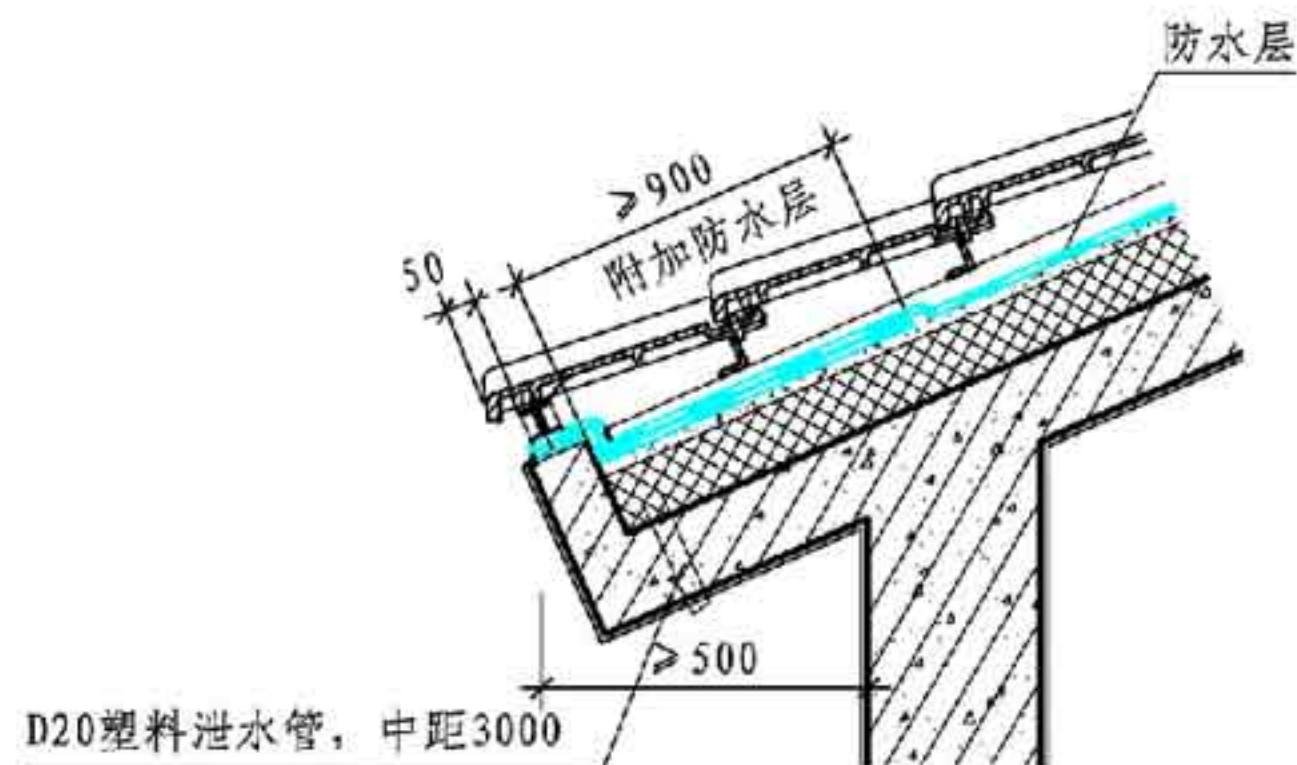
① 平瓦屋面檐口
