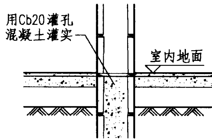
① 无芯柱
