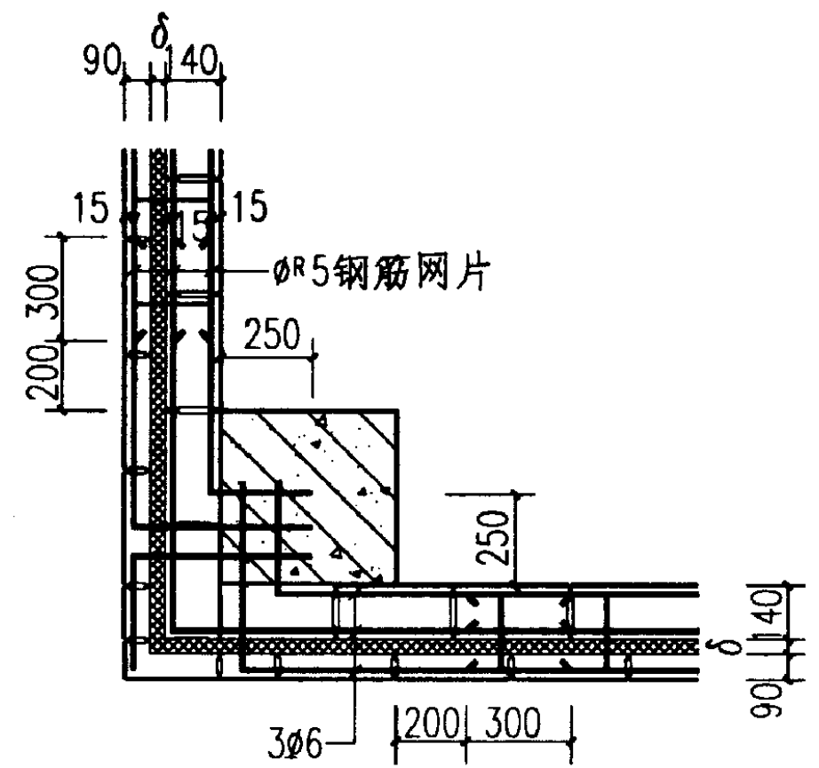
④ 转角夹芯墙
