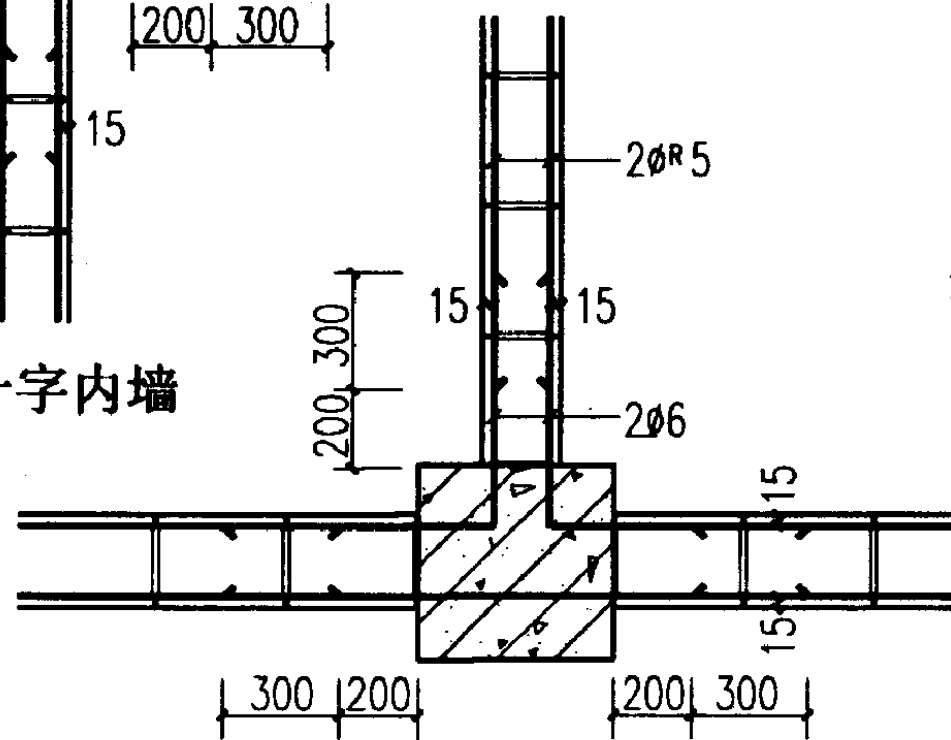
⑥ 丁字内墙
