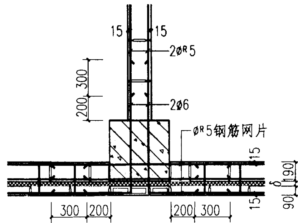
5 丁字夹芯墙
