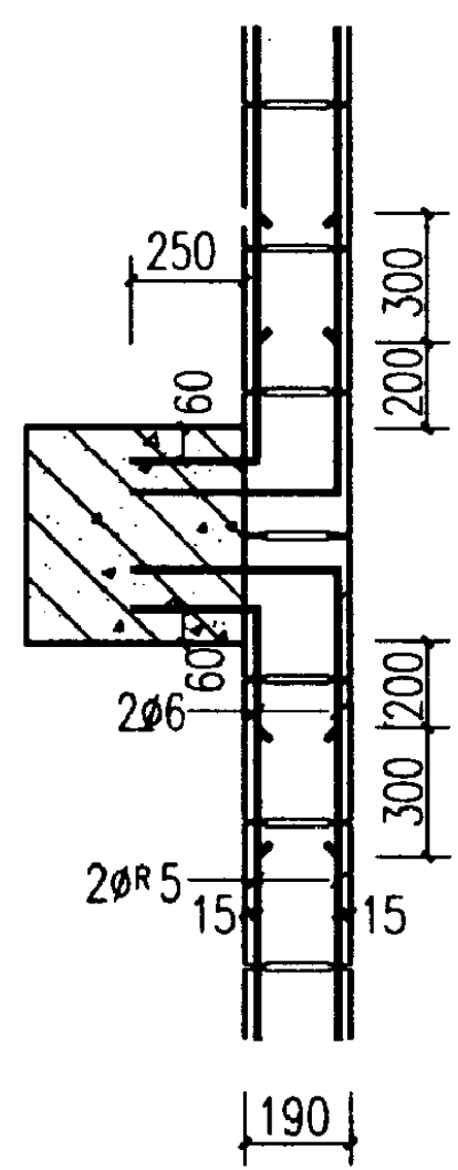
③ 一字墙
