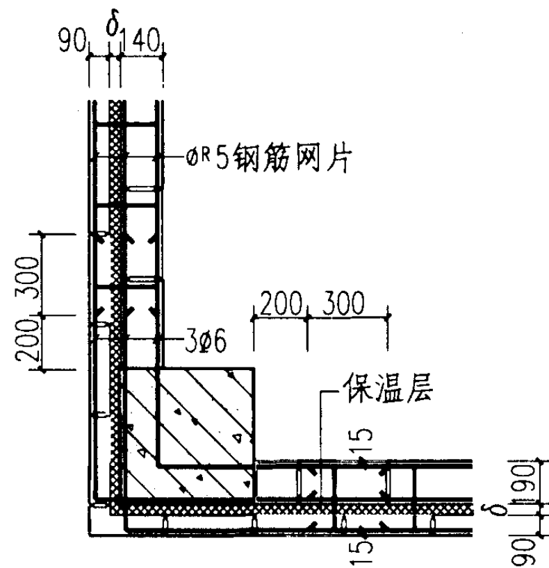
4 转角夹芯墙
