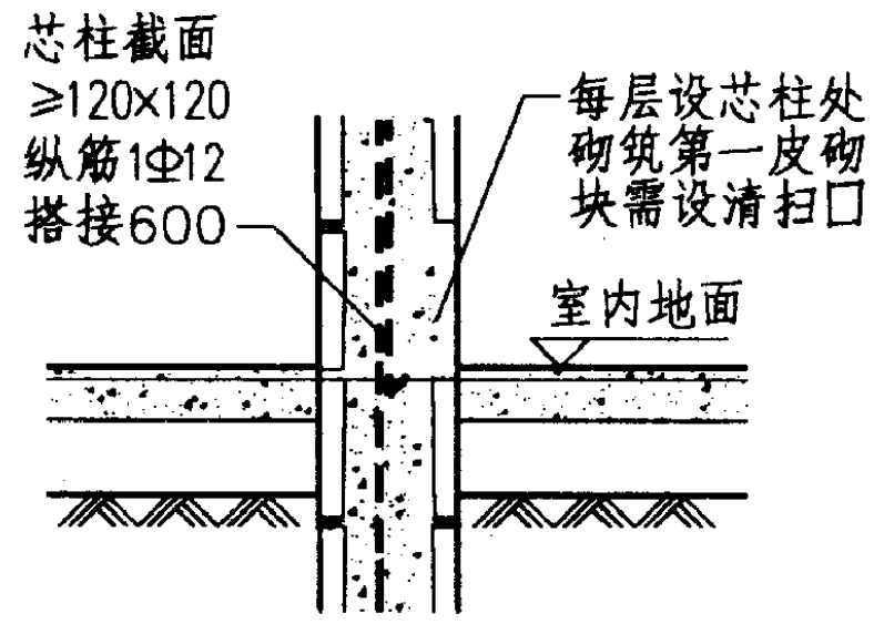
② 设芯柱
