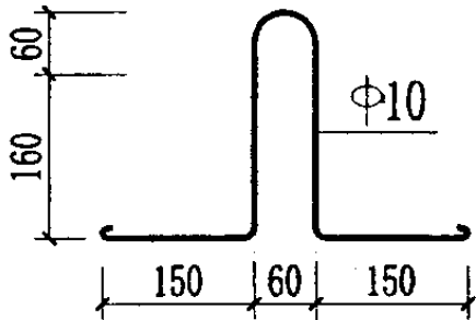
图 7.12 吊钩大样
