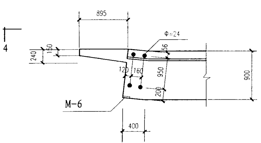
自由落水端节点模板图
