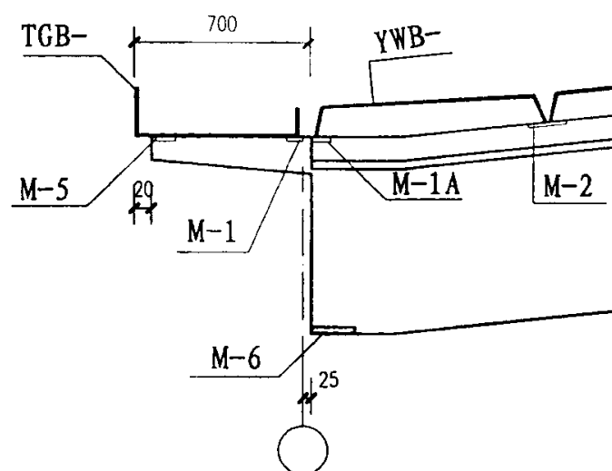
外天沟端部排板示意
