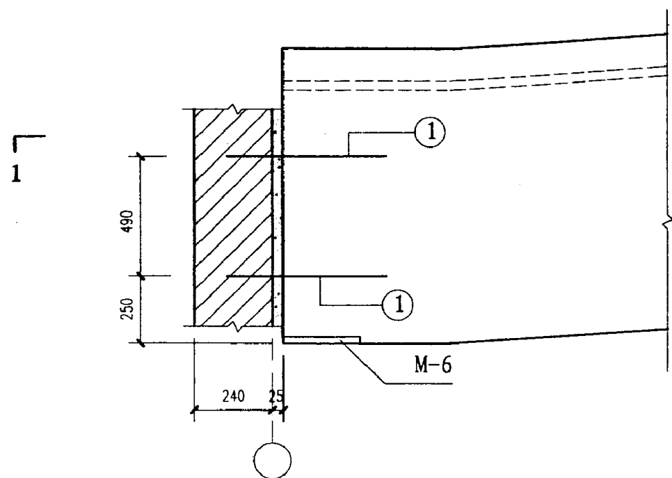
无天沟梁端预埋锚固钢筋
