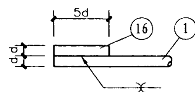
16号与1号焊接详图
