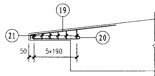
自由落水端节点配筋图
