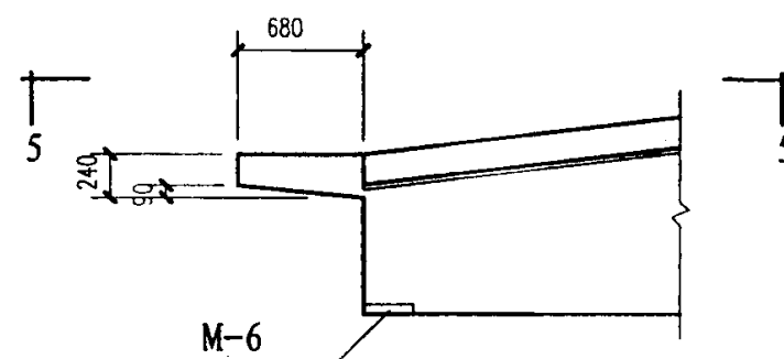
外天沟端节点模板图
