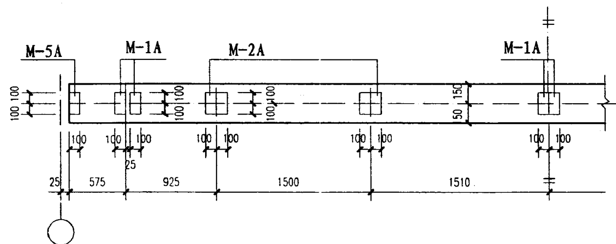
内天沟时屋面梁上翼缘预埋件位置图
