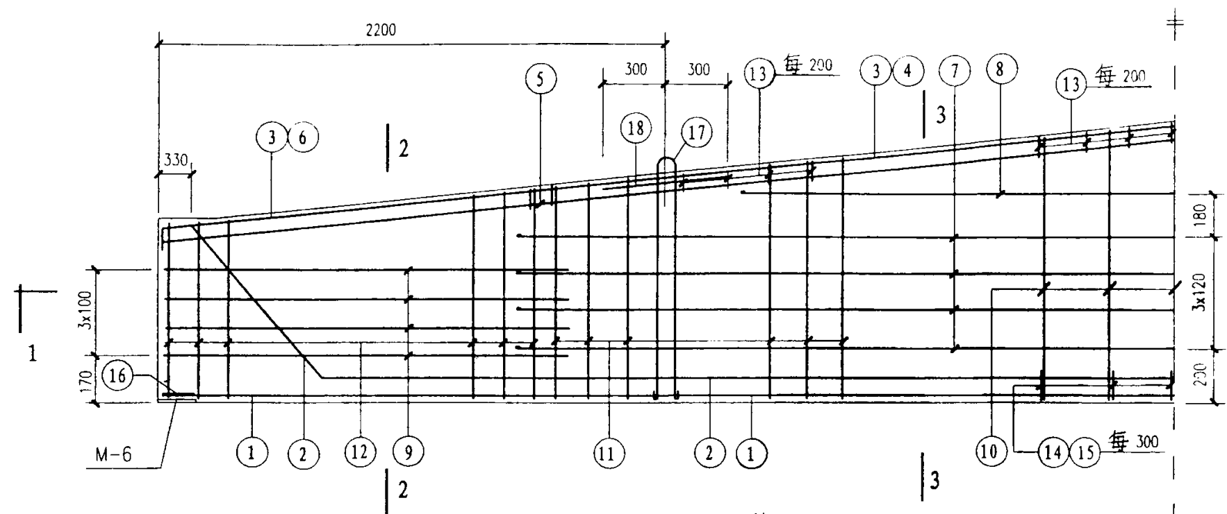
配筋图
