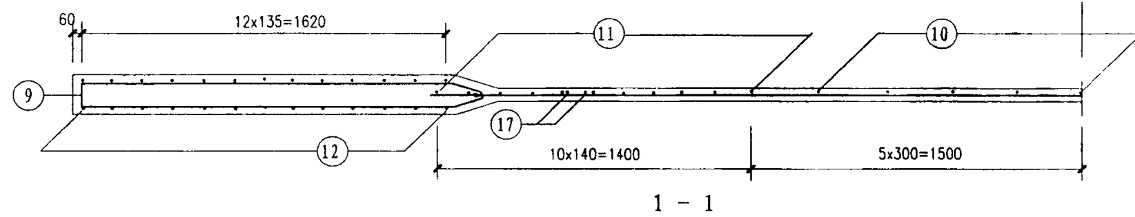
配筋图
