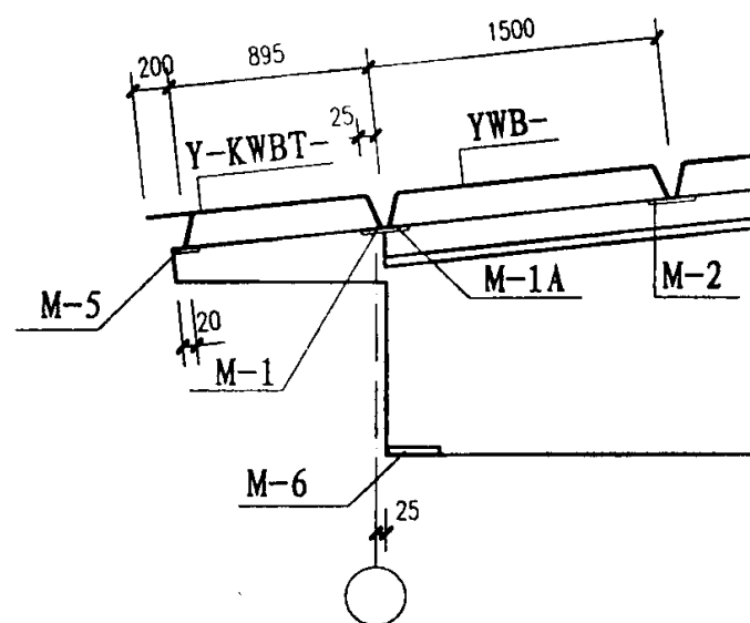
自由落水端部排板示意
