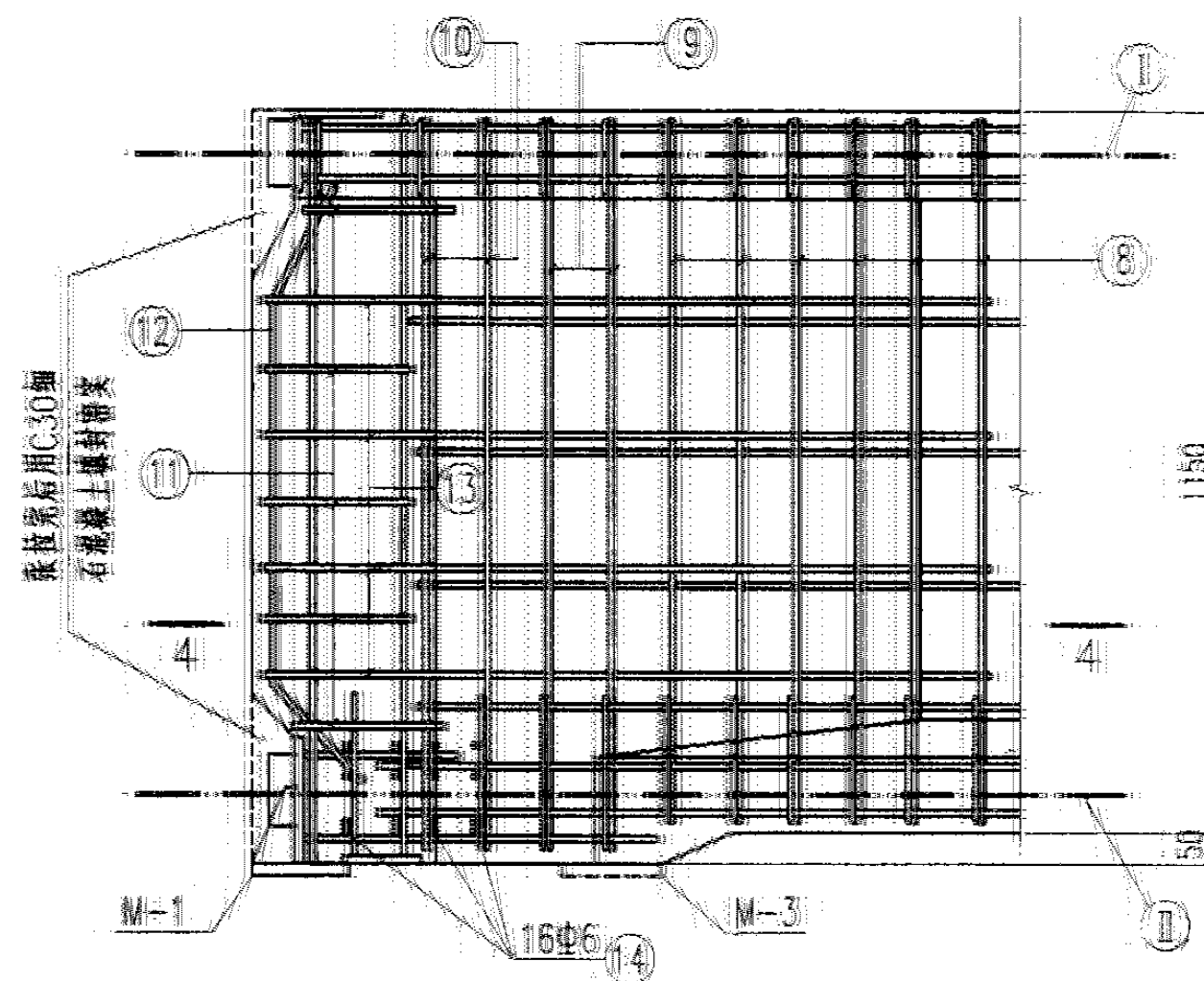
端部配筋大样图
