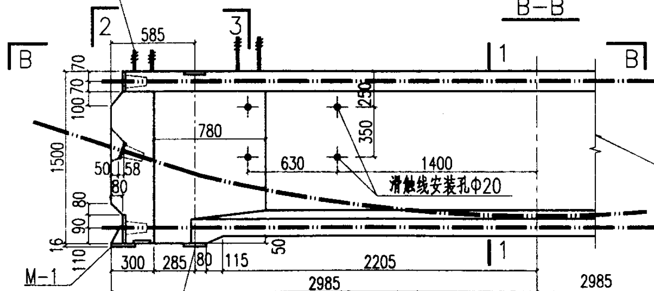
YDL-5s.B 模板图
