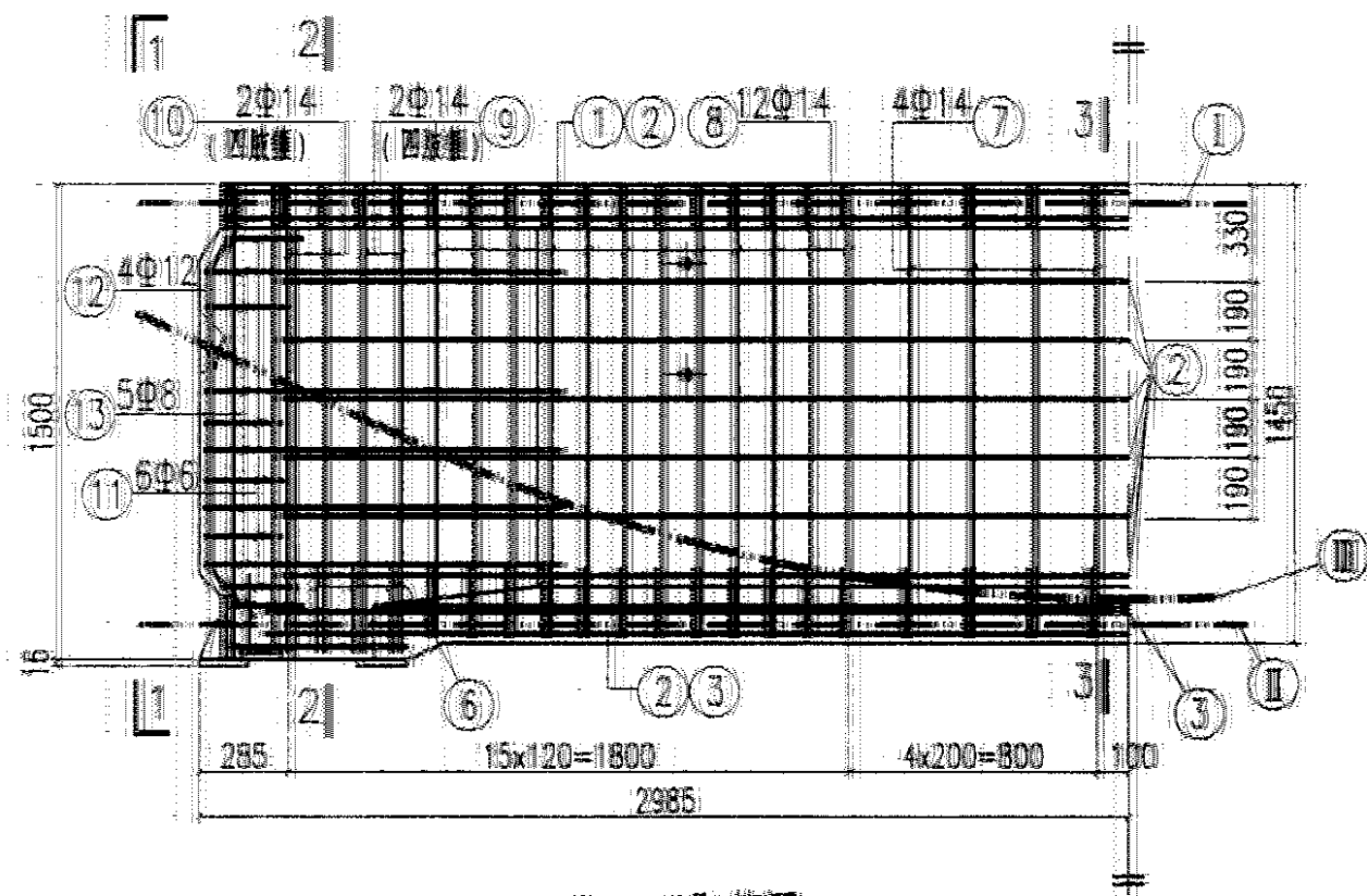
YDL-6配筋图
