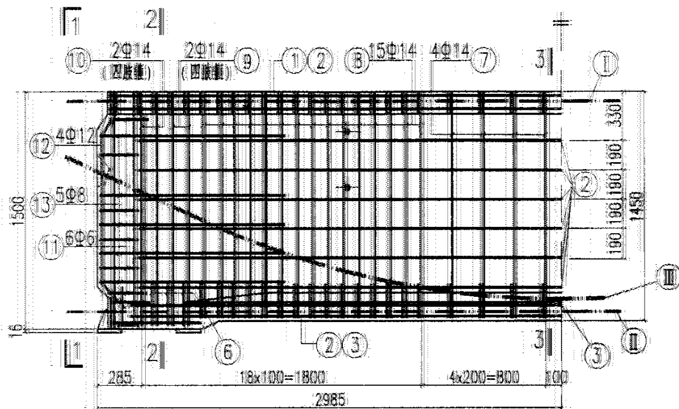
YDL-7配筋图
