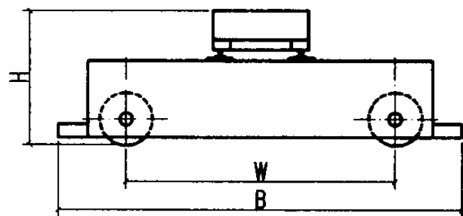
10~50t(10.5~25.5)吊车侧面示意图
