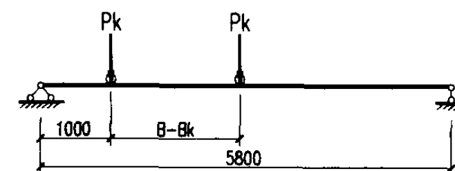
最大剪力位置图
