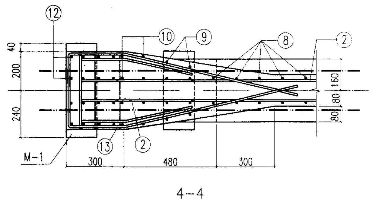
端部配筋大样图
