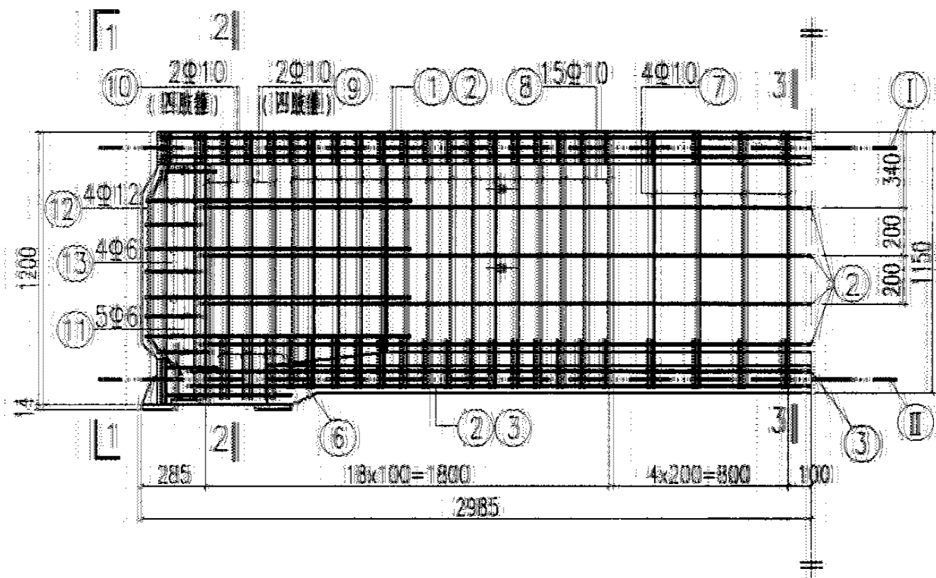
YDL-2配筋图
