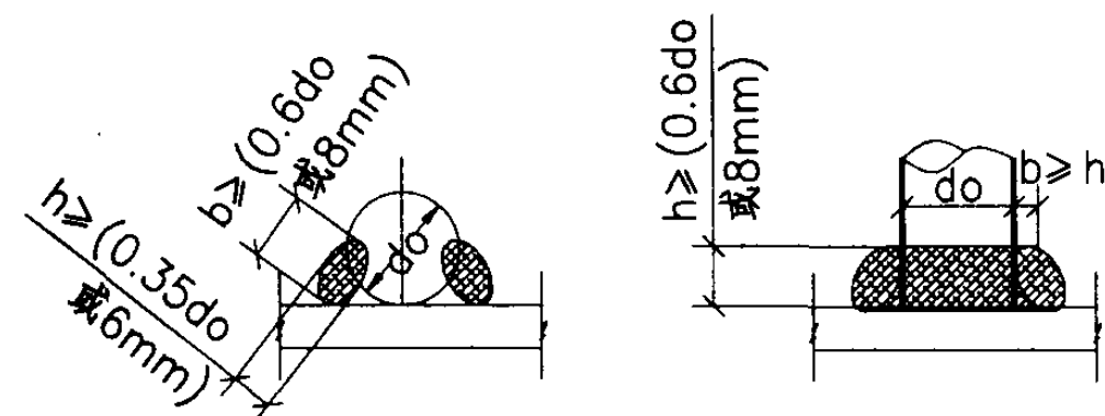
钢筋与钢板搭接焊
