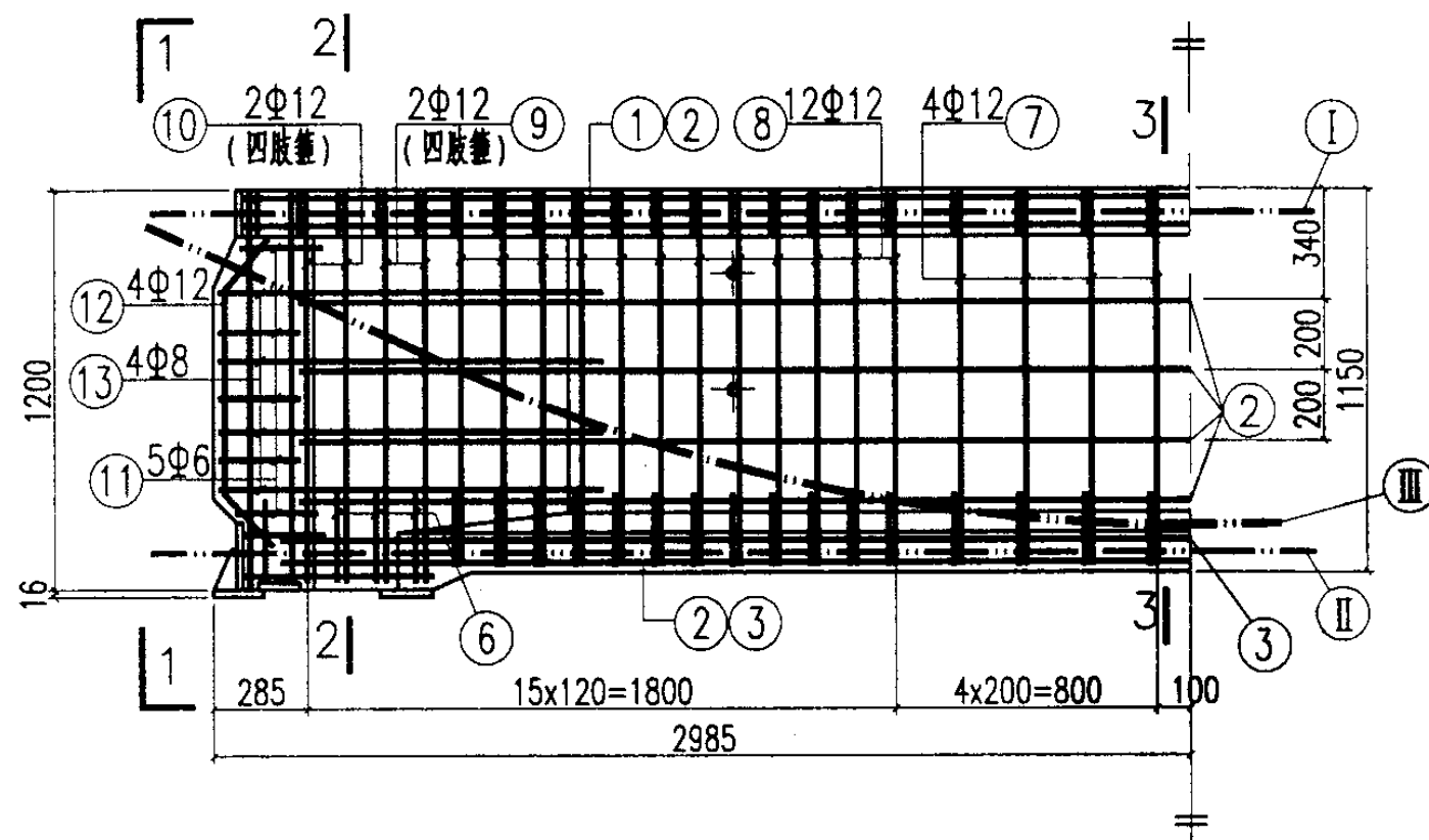
YDL-3配筋图
