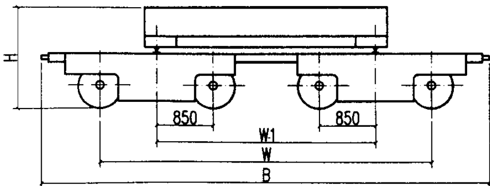
75/20~125/30t吊车侧面示意图
