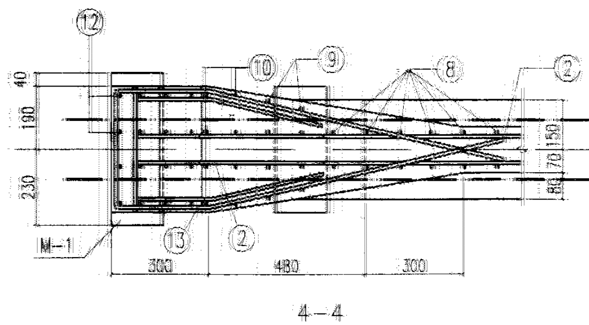
端部配筋大样图
