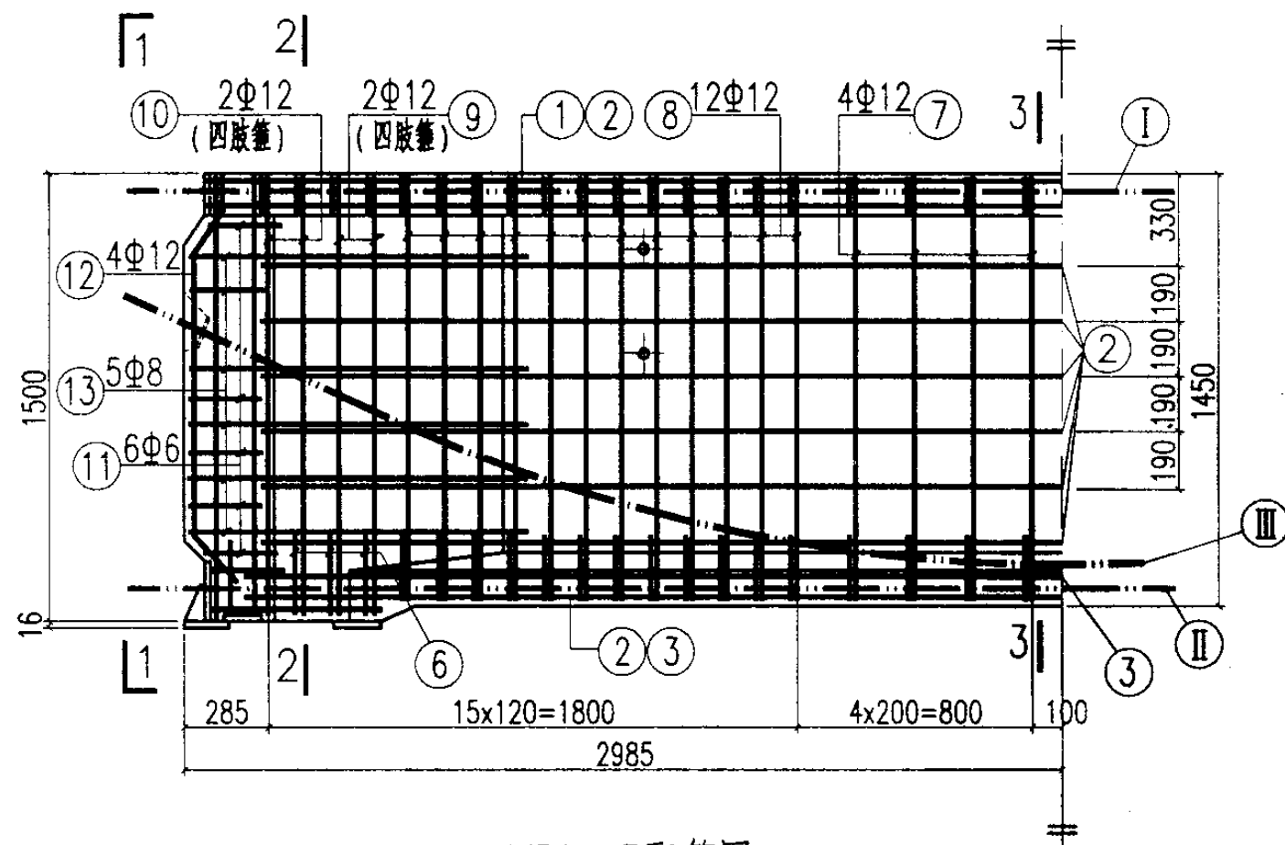
YDL-5配筋图
