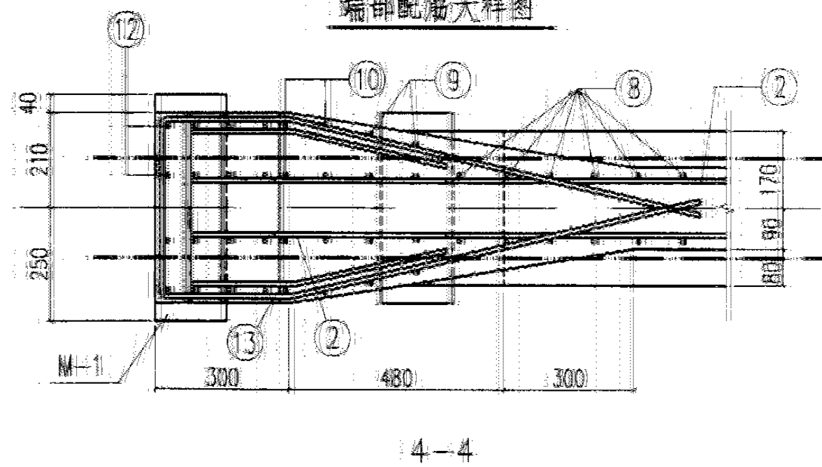
端部配筋大样图
