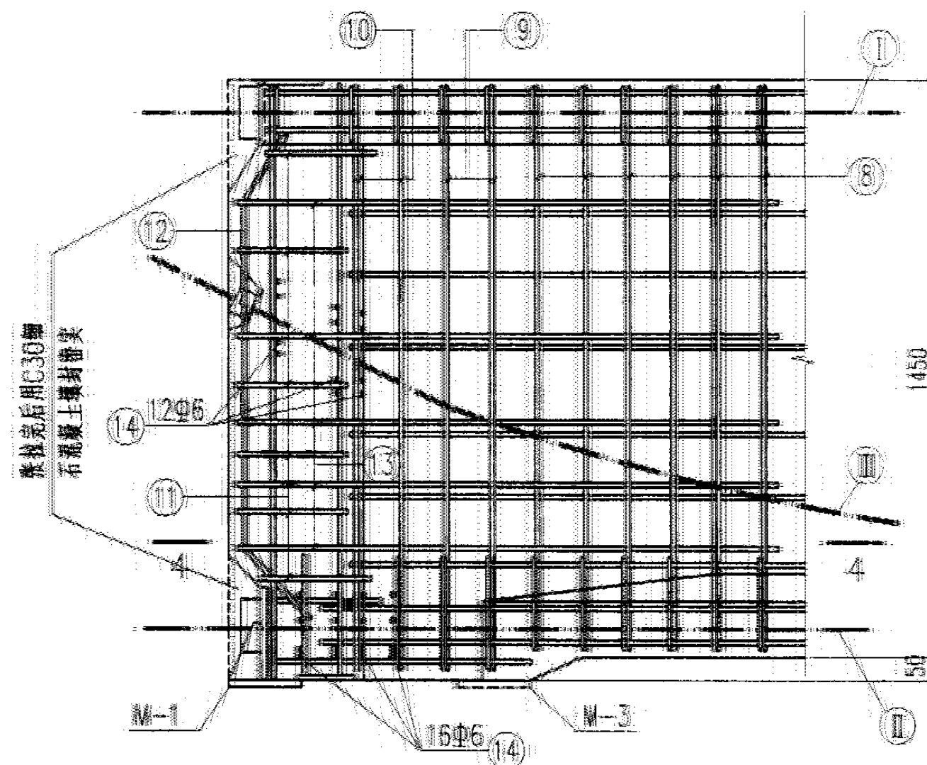
端部配筋大样图
