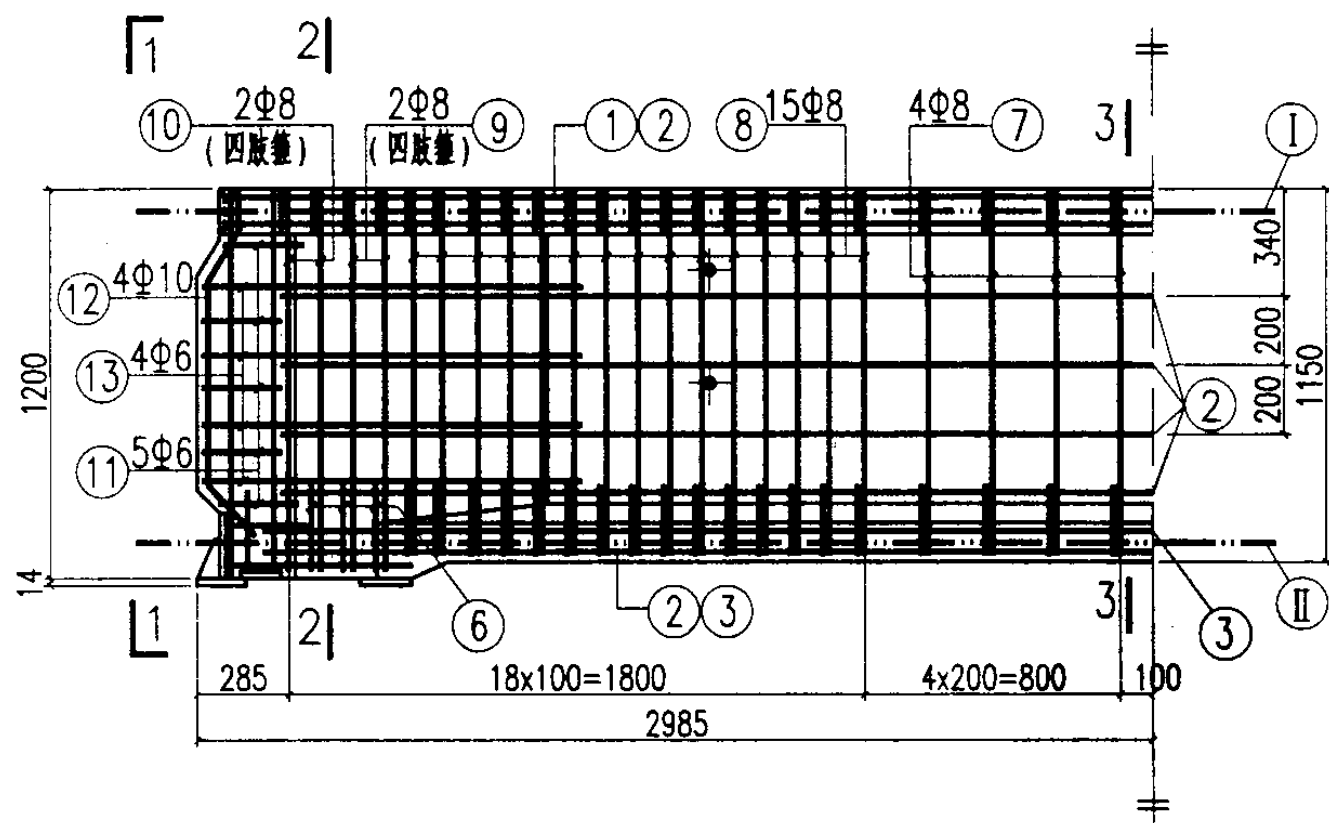
YDL-1 配筋图
