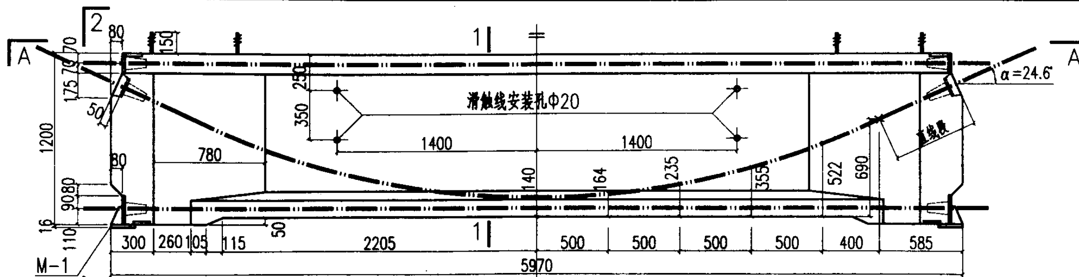
YDL-3 z 模板图
