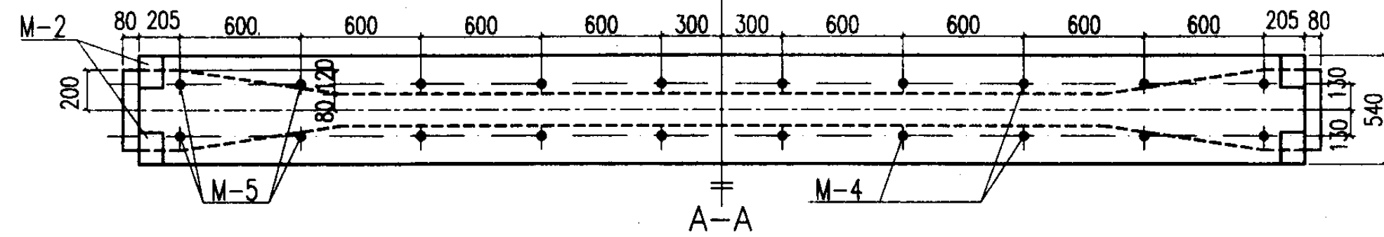
YDL-3 z 模板图
