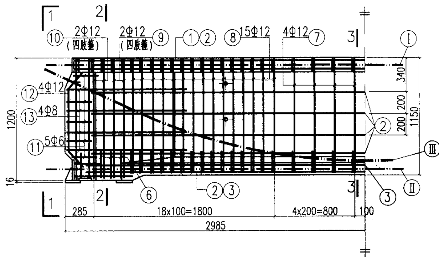
YDL-4配筋图
