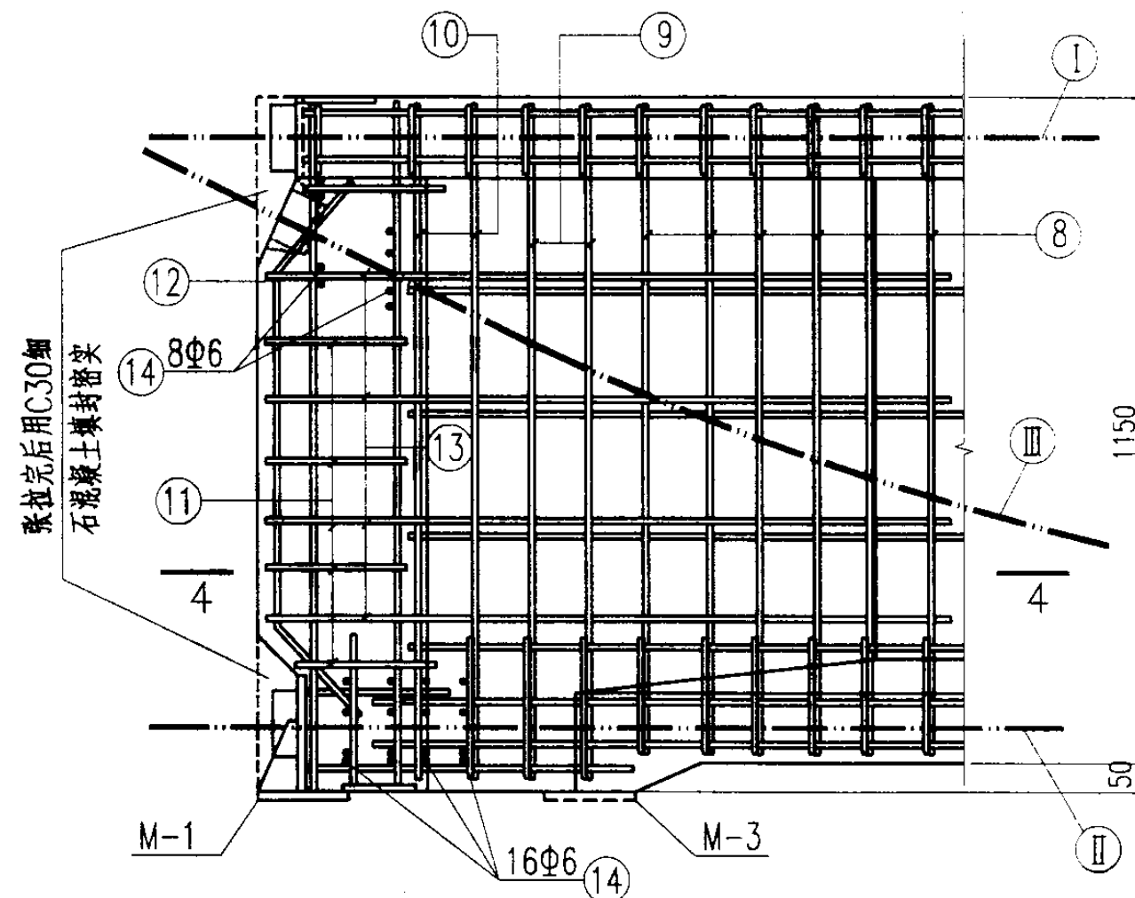
端部配筋大样图
