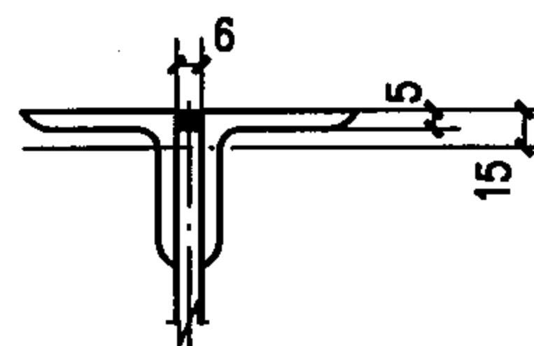
上弦塞焊示意
