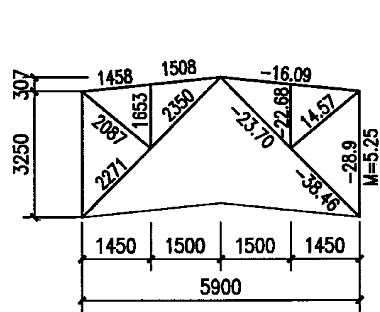
几何尺寸及内力图
