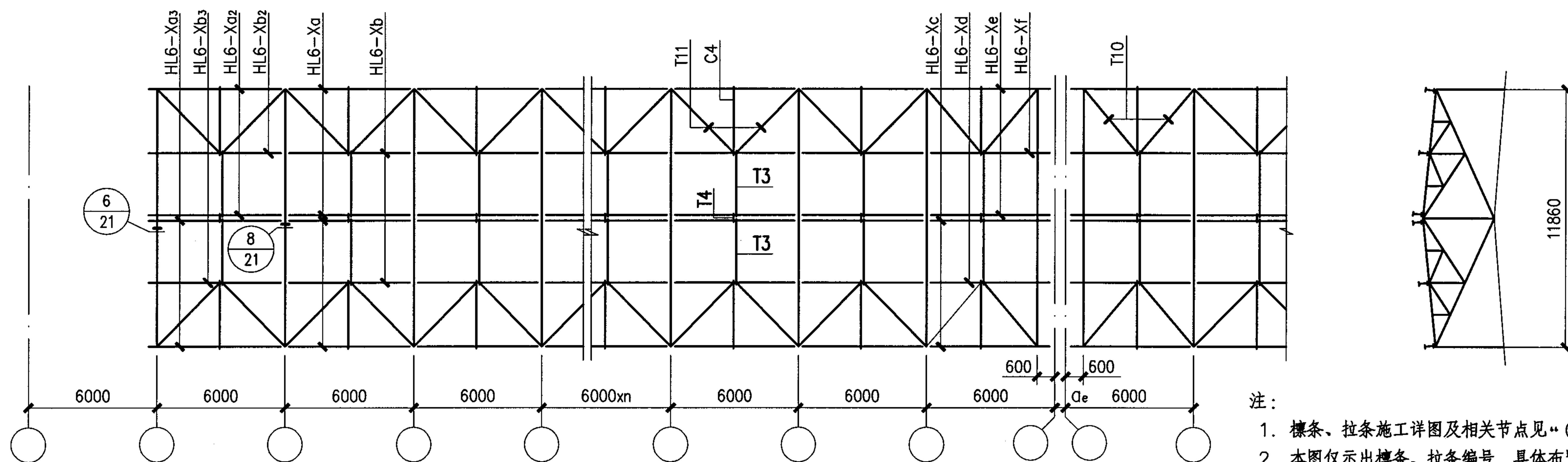
檩条、拉条平面布置图 (二)
