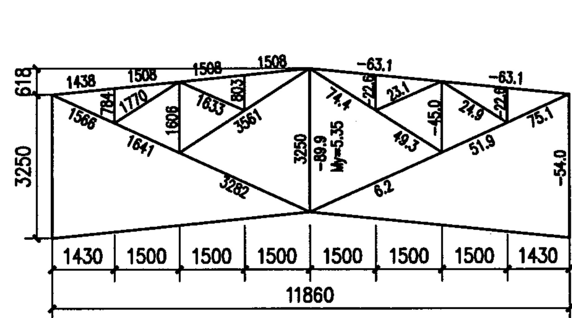
几何尺寸及内力图
