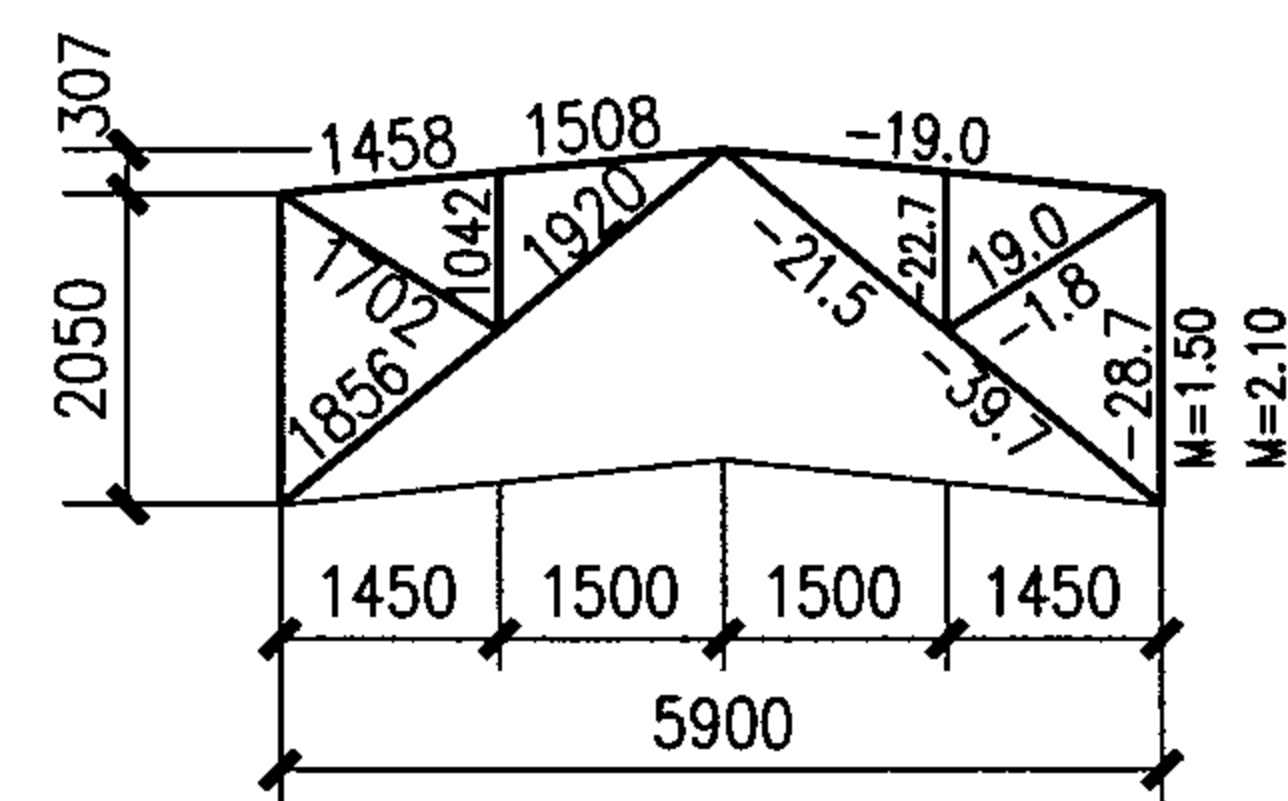
几何尺寸及内力图
