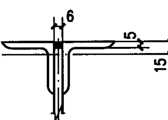
上弦塞焊示意
