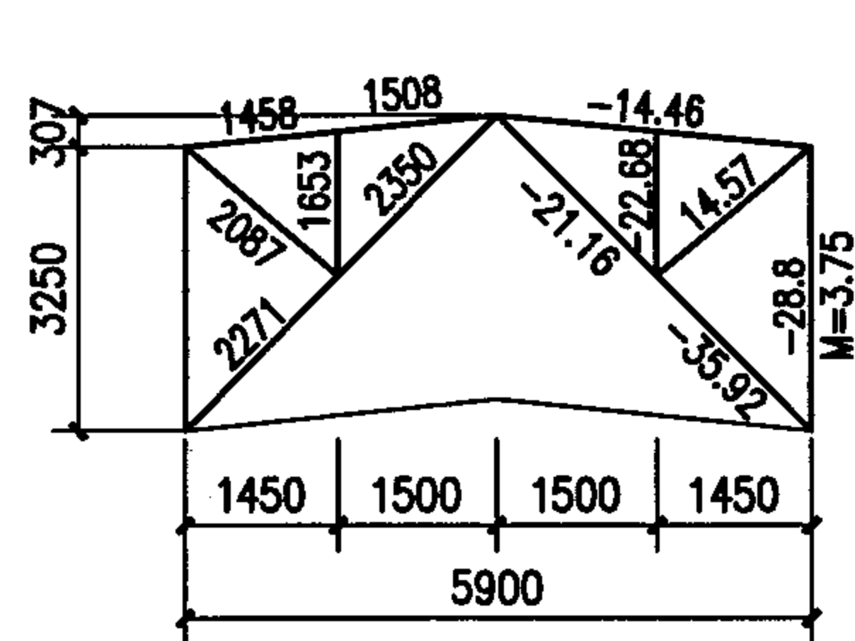
几何尺寸及内力图
