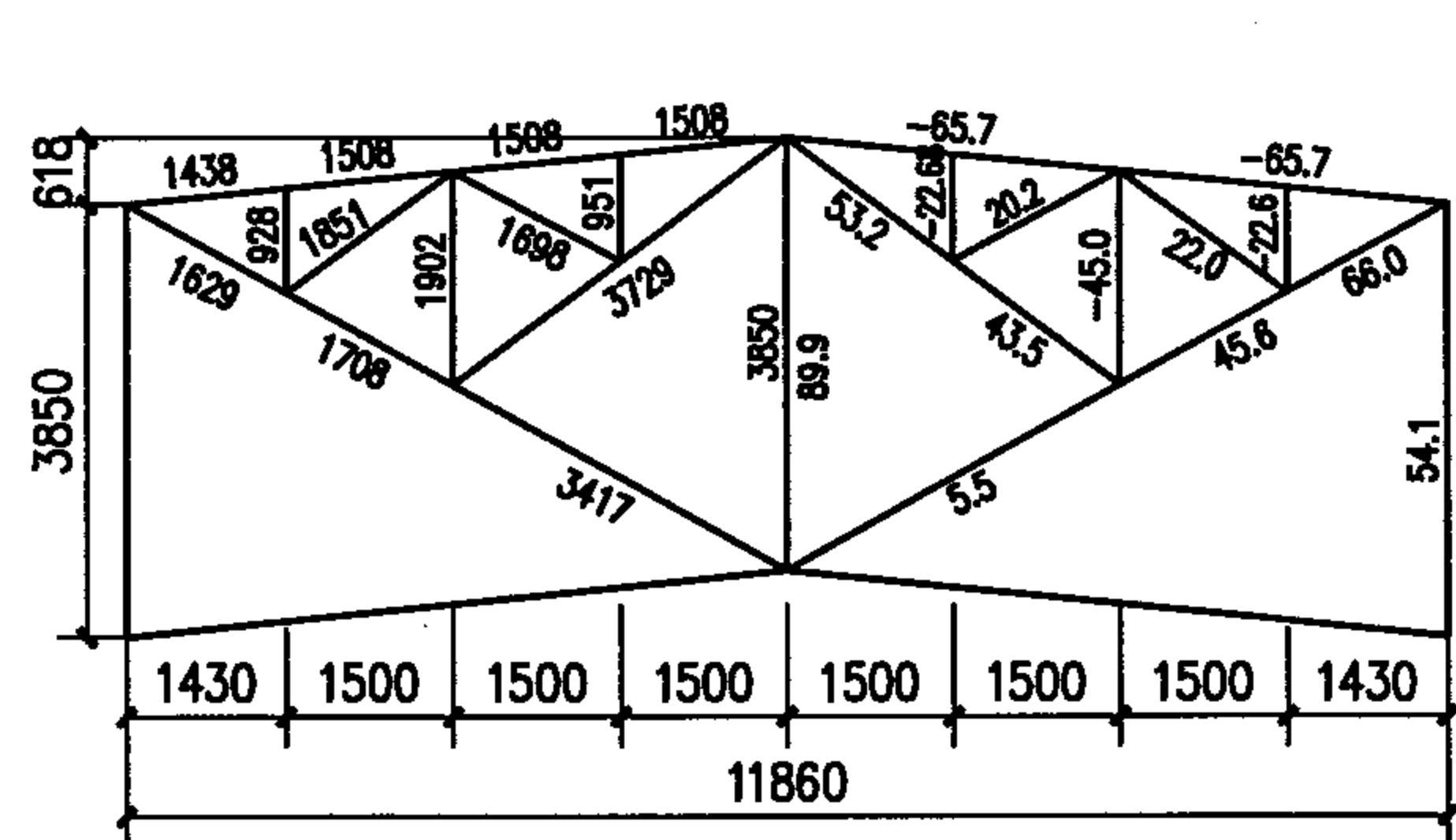
几何尺寸及内力图
