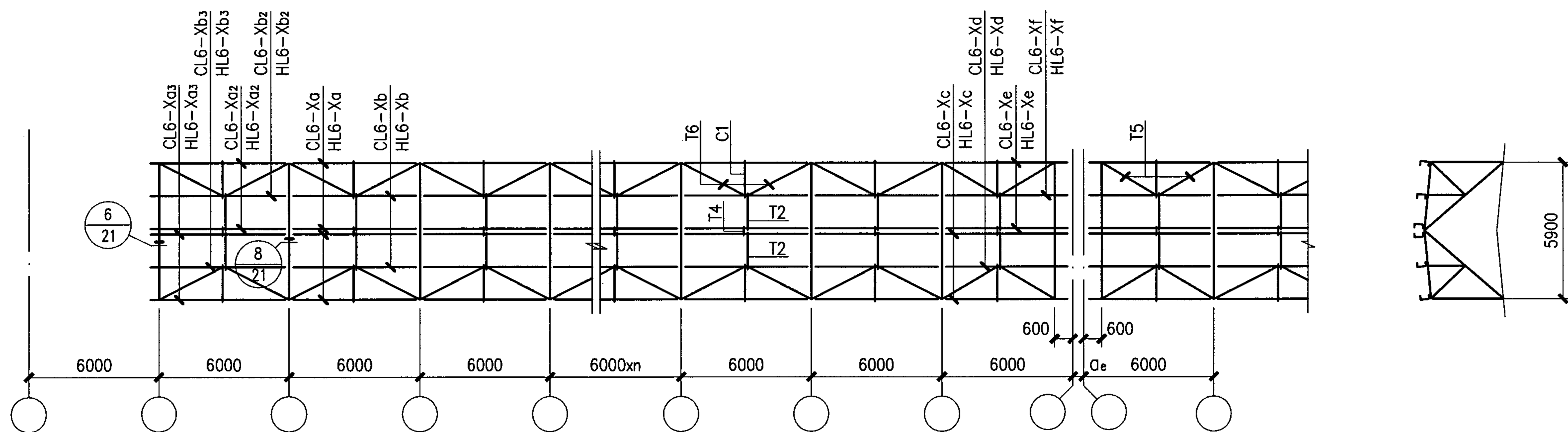
標条、拉条平面布置图（一）
