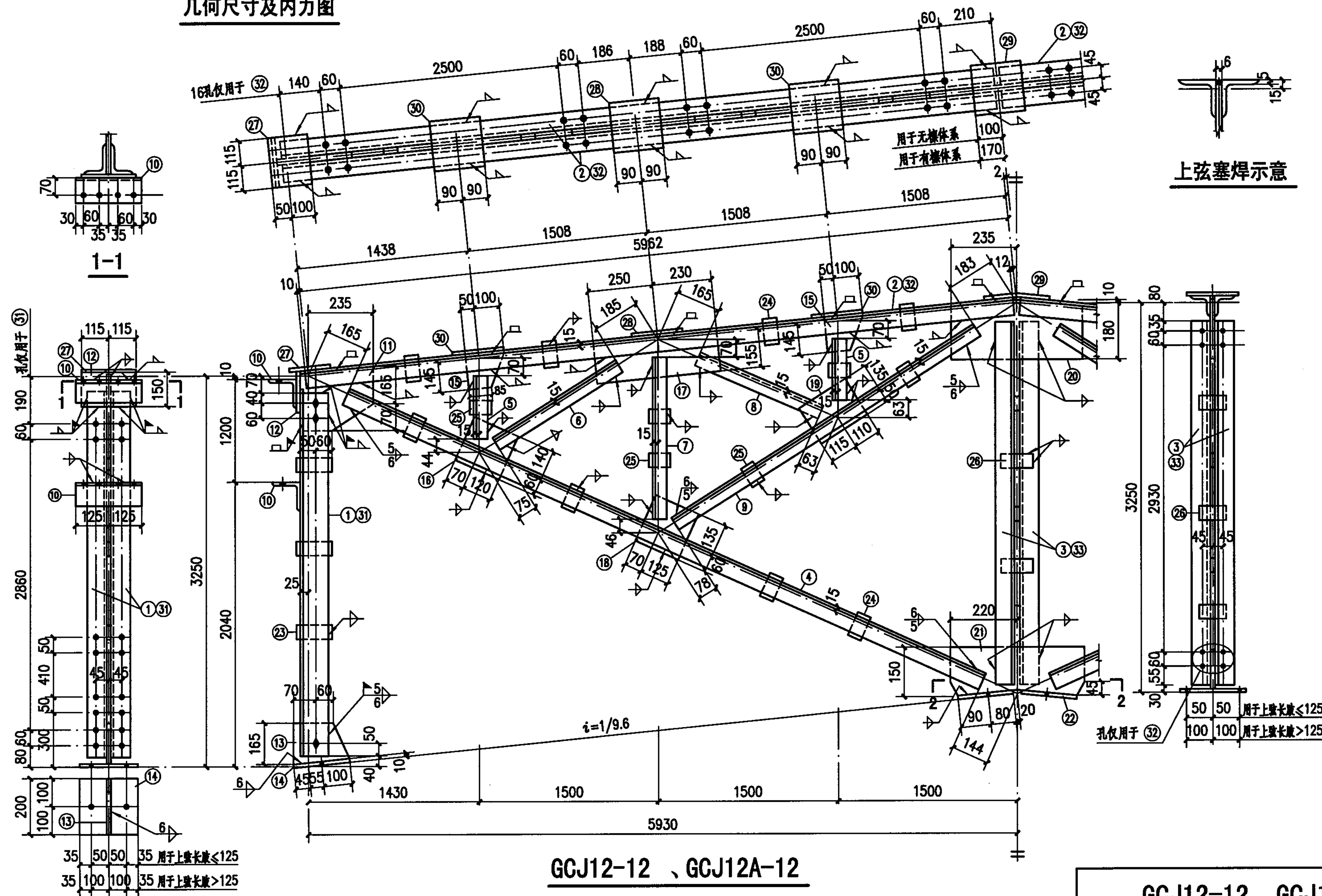
几何尺寸及内力图
