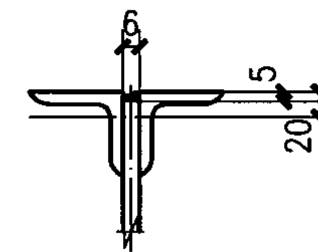
上弦塞焊示意
