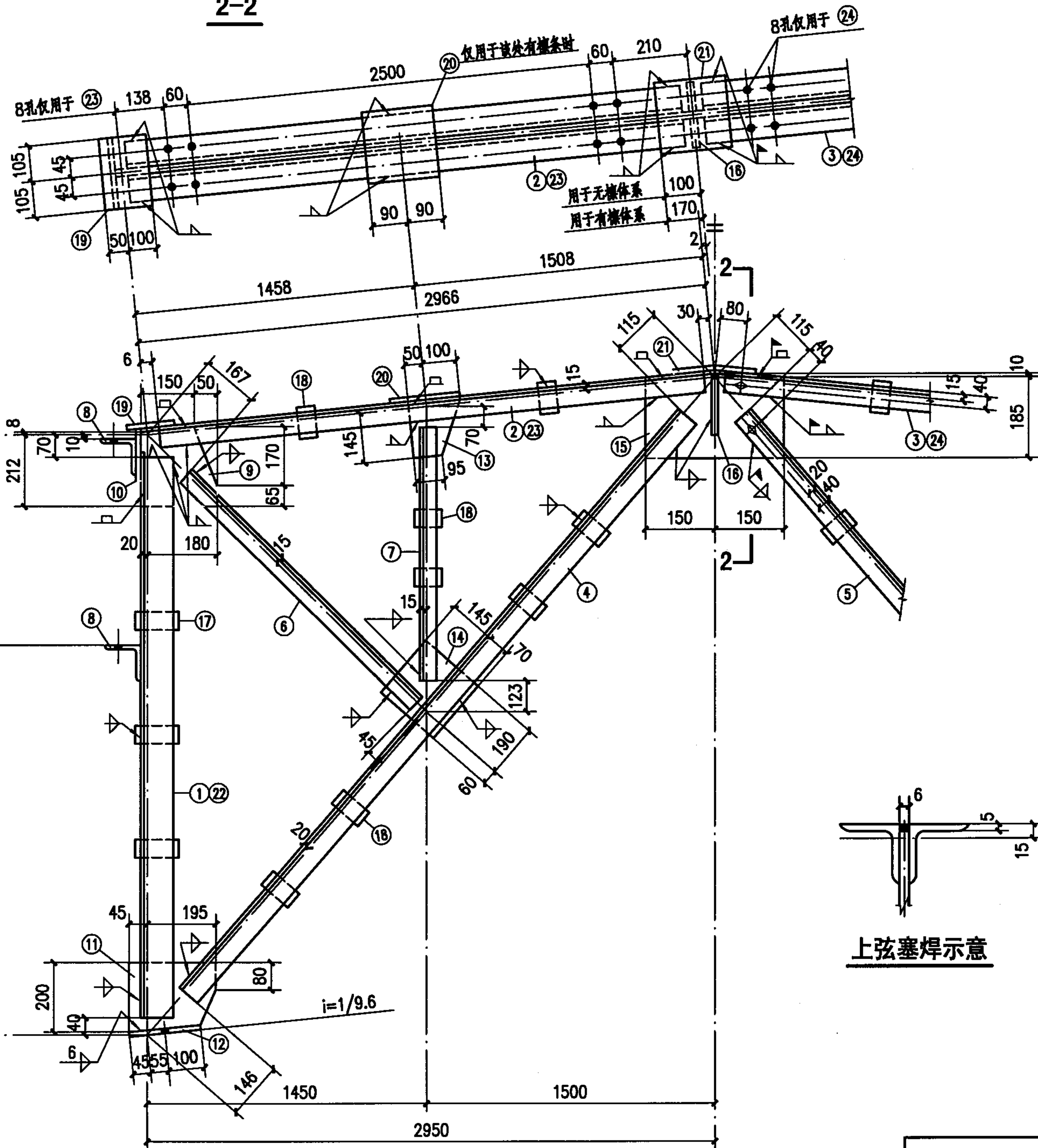
GCJ6-41、GCJ6A-41
