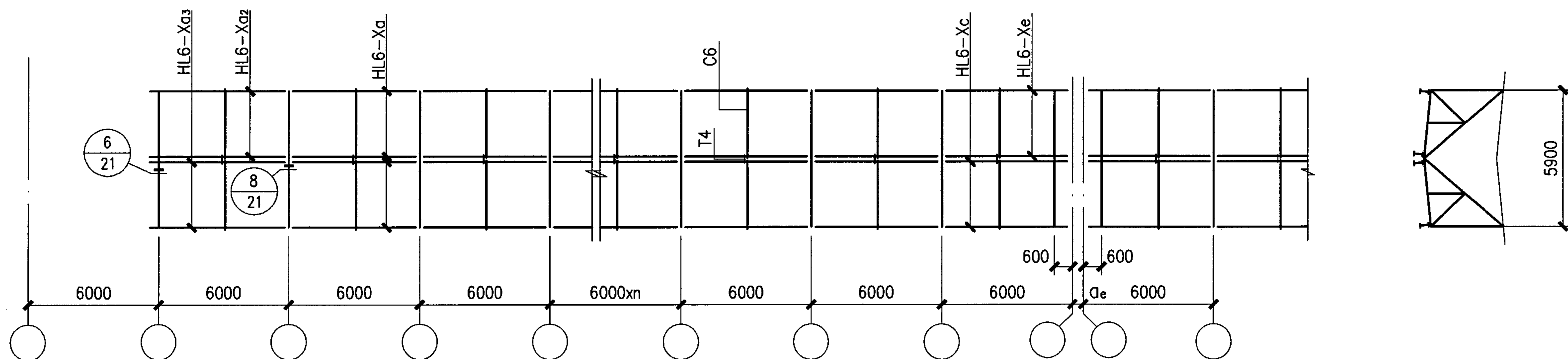
標条、拉条平面布置图（二）
