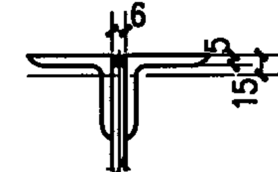
上弦塞焊示意
