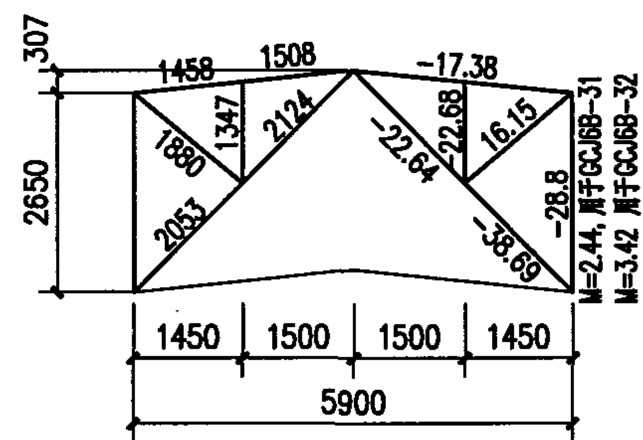
几何尺寸及内力图
