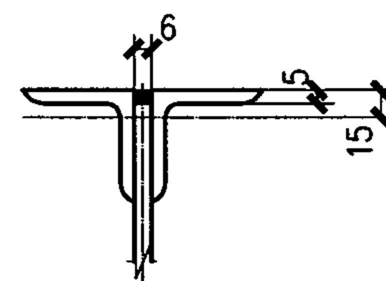
上弦塞焊示意
