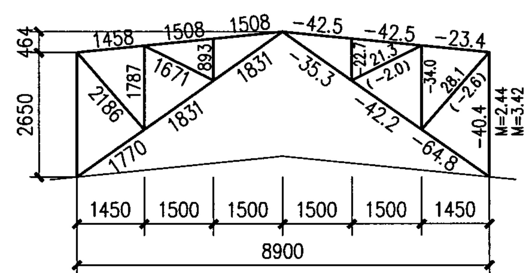
几何尺寸及内力图
