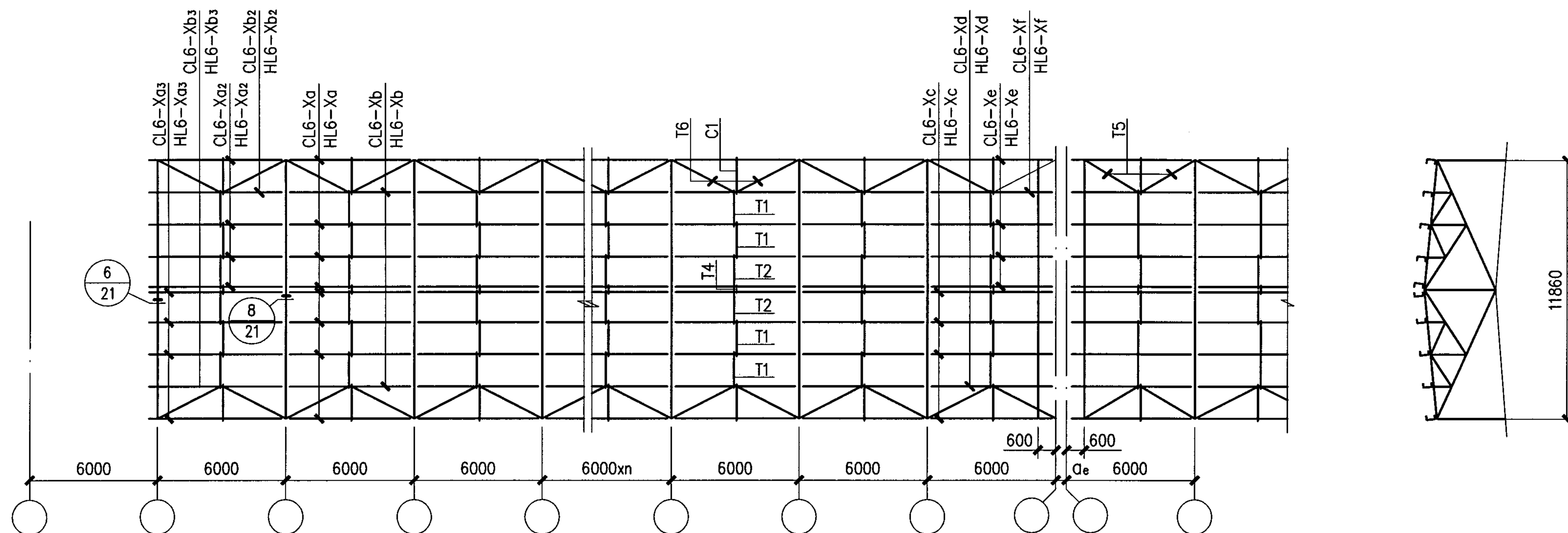
檩条、拉条平面布置图 (一)
