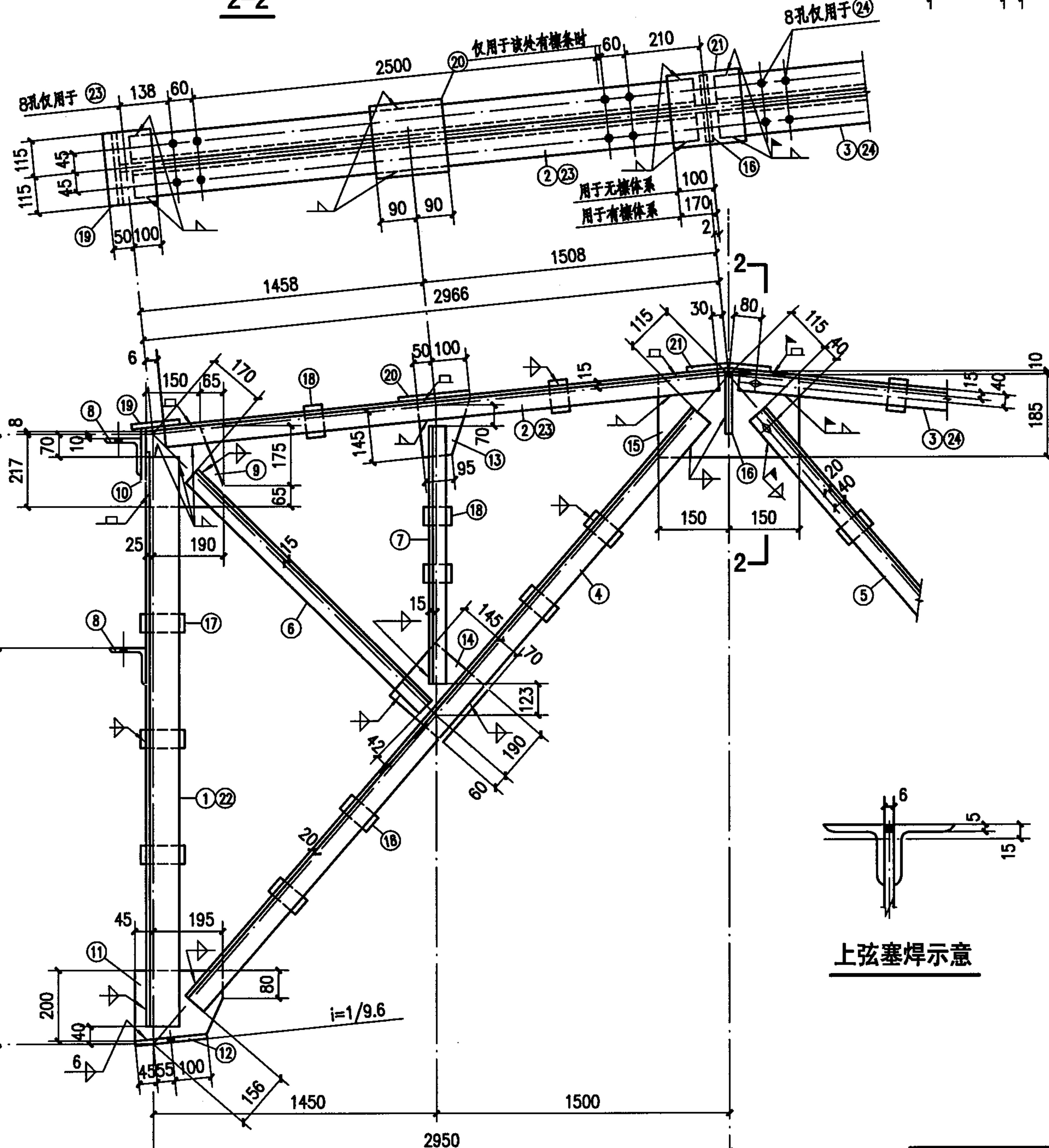
GCJ6-42、GCJ6A-42
