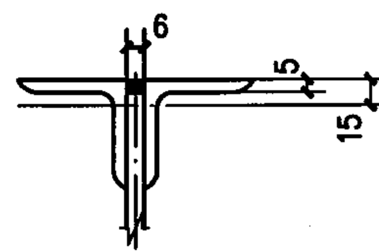
上弦塞焊示意
