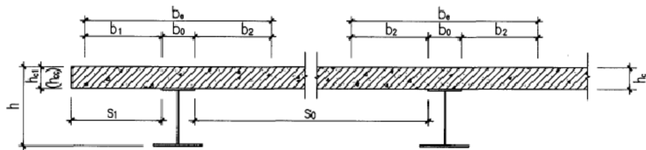
a.翼板为混凝土平板(无板托)
