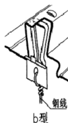
缩口型压型钢板悬吊系统构造
