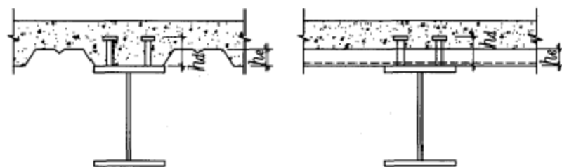
肋与钢梁平行的组合梁截面
