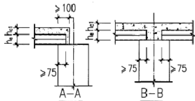
组合楼板支承长度构造要求
