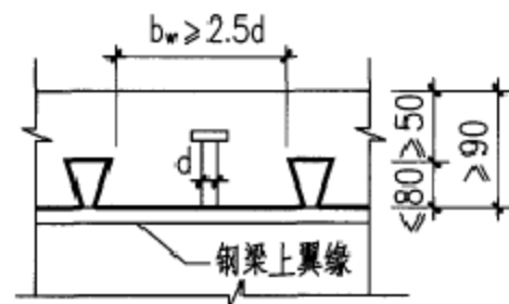
b. 缩口型或闭口型
