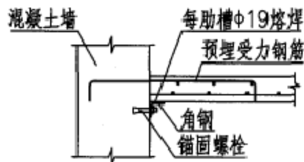
组合楼板与混凝土墙侧面连接做法
