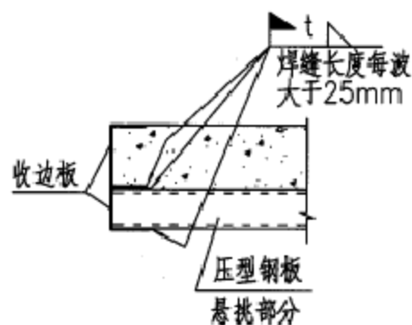
横向收边(1)
