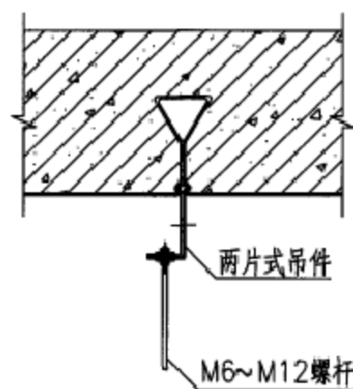
闭口型压型钢板悬吊系统构造
