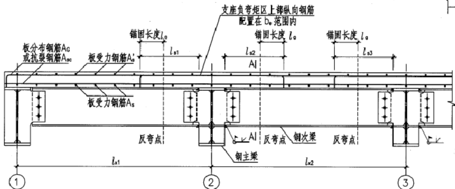
2-2 连续组合梁节点连接及配筋构造
