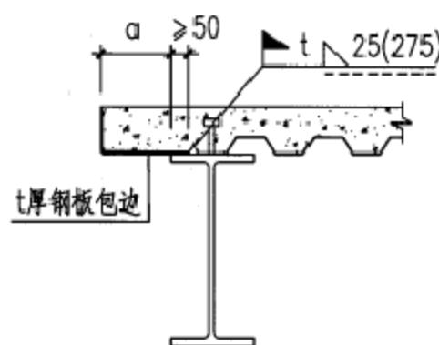
板肋与梁平行收边构造 ( a \leq 250 )
