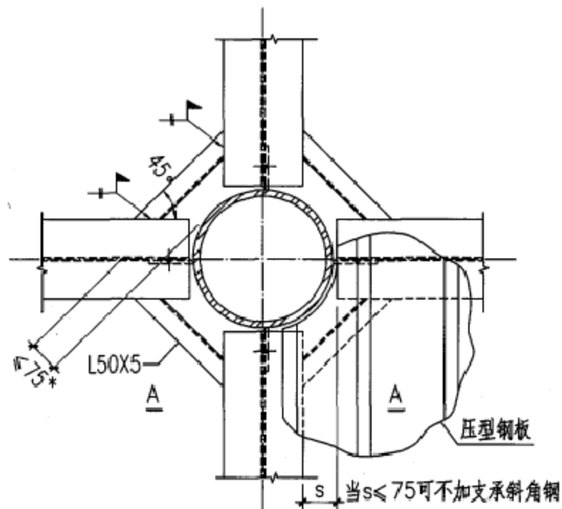
圆柱梁柱节点处压型钢板支托构造
