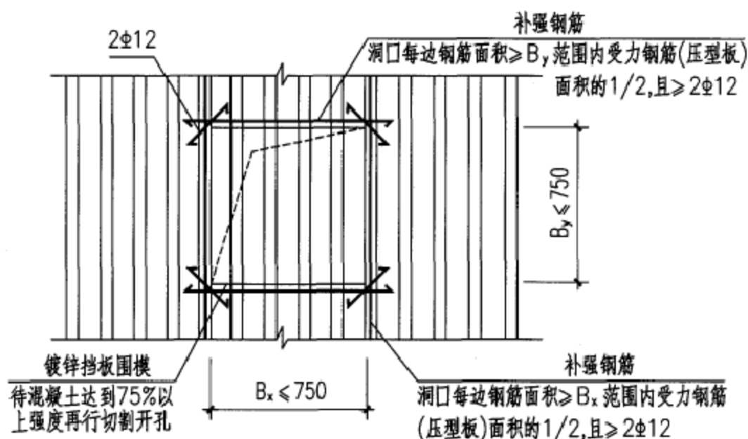
组合楼板开孔 \leq 750 时的加强措施(2)
