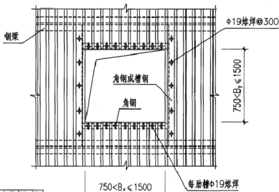
组合楼板开孔750~1500时的加强措施
