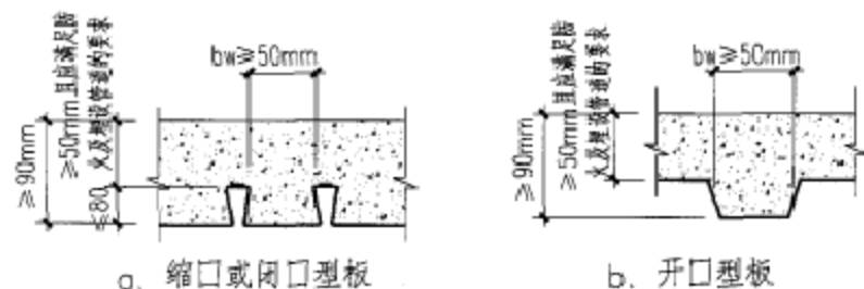
图 6.5-1 对组合楼板截面形状的要求
