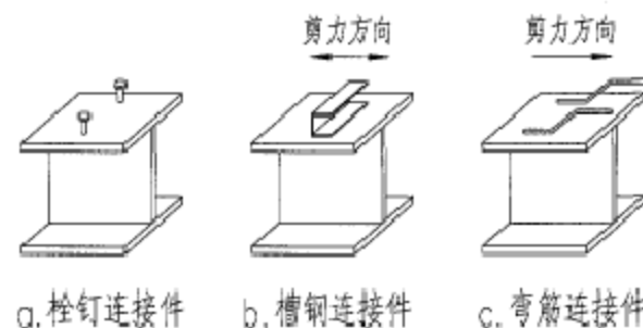
图5.2-1 连接件的形式及布置方向
