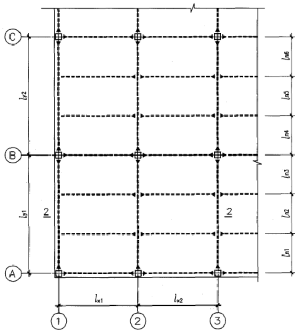
连续组合梁平面布置示意图
