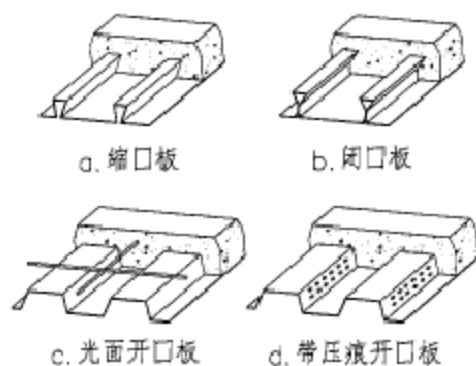
图 6.2-1 压型钢板组合楼板的基本形式
