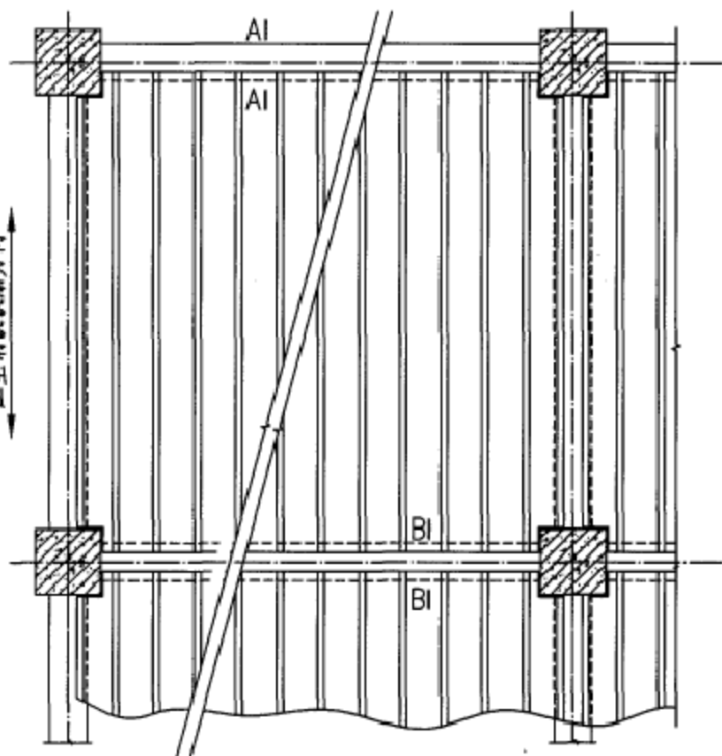
压型钢板铺板平面示意图
