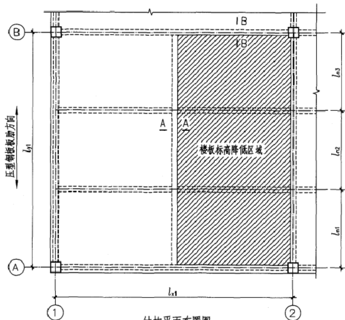
结构平面布置图
