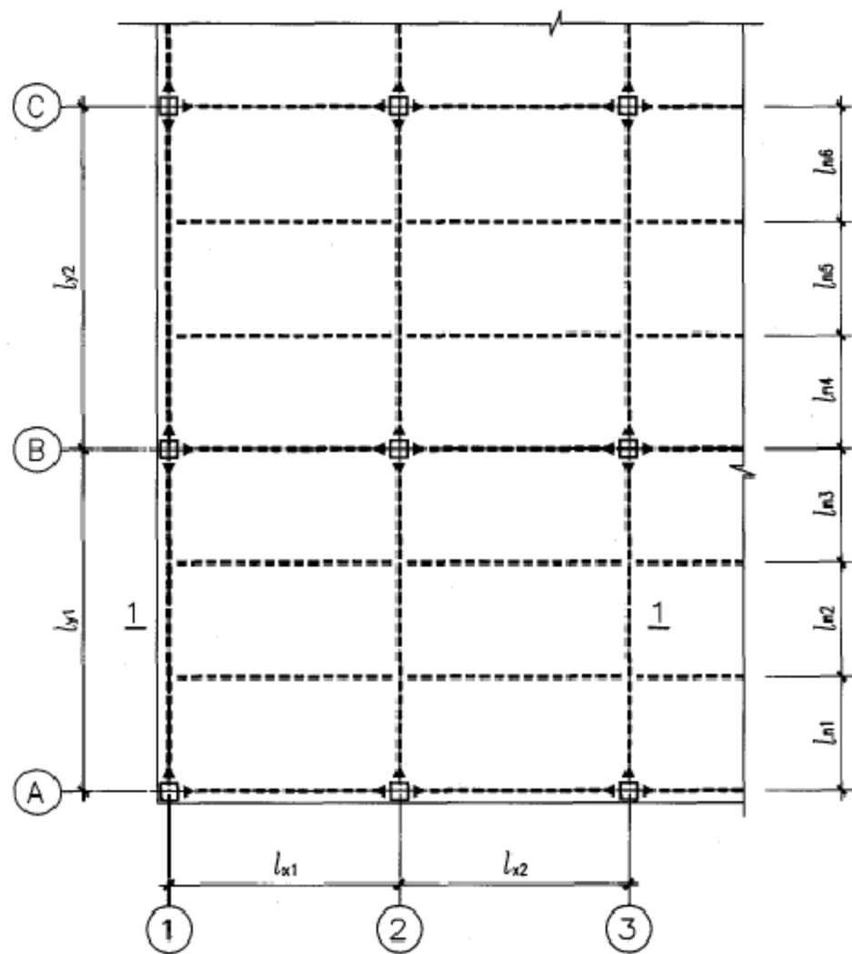
简支组合梁平面布置示意图
