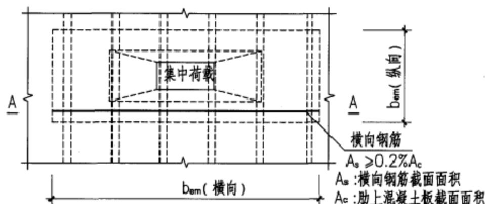
局部集中荷载作用下的横向钢筋
