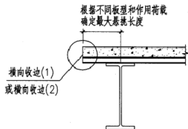
板肋与梁垂直收边构造(1)
