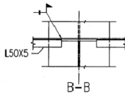
H型钢柱梁柱节点处压型钢板支托构造(2)
