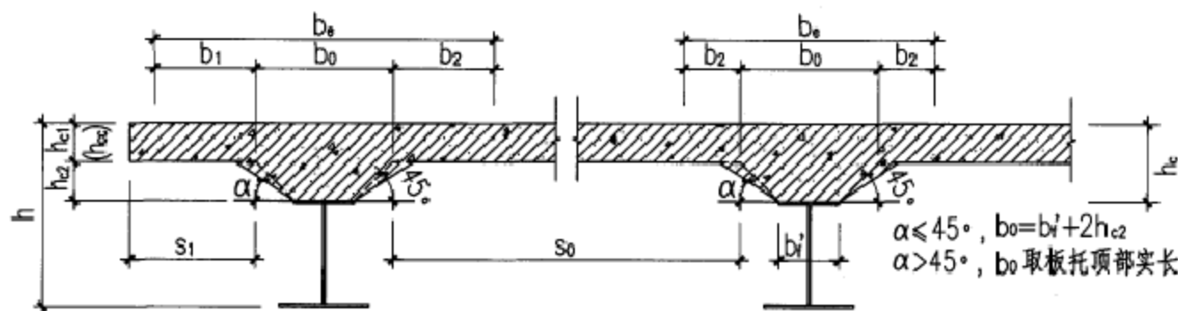
b.翼板为混凝土平板(有板托)
