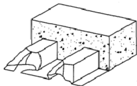
压型钢板端头压扁式收边
