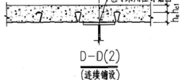
组合楼板端部支承构造一 (支承于钢梁上)
