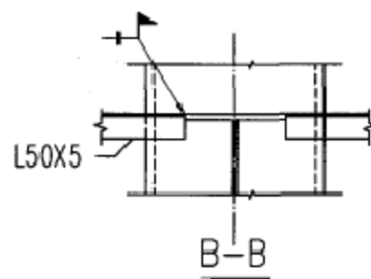
箱型钢柱梁柱节点处压型钢板支托构造(2)
