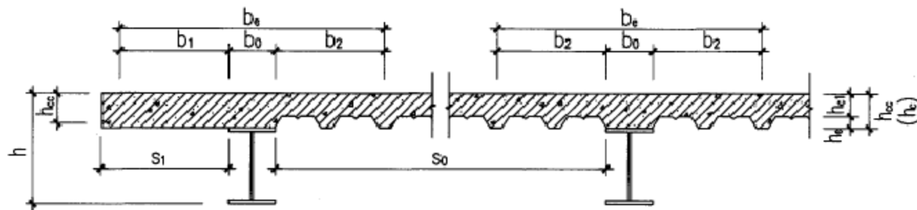
c.翼板为组合楼板
