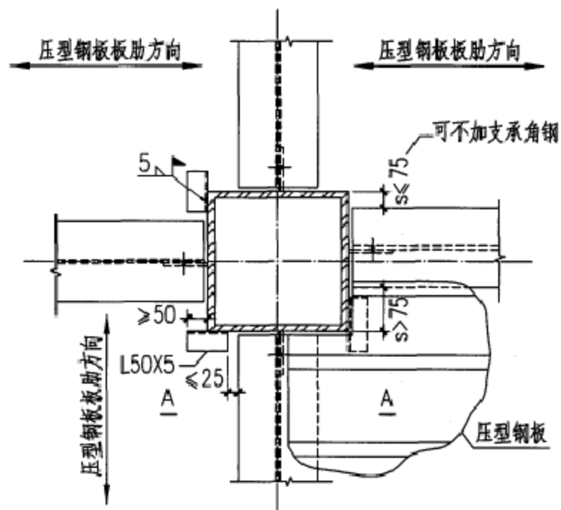
箱型钢柱梁柱节点处压型钢板支托构造(1)
