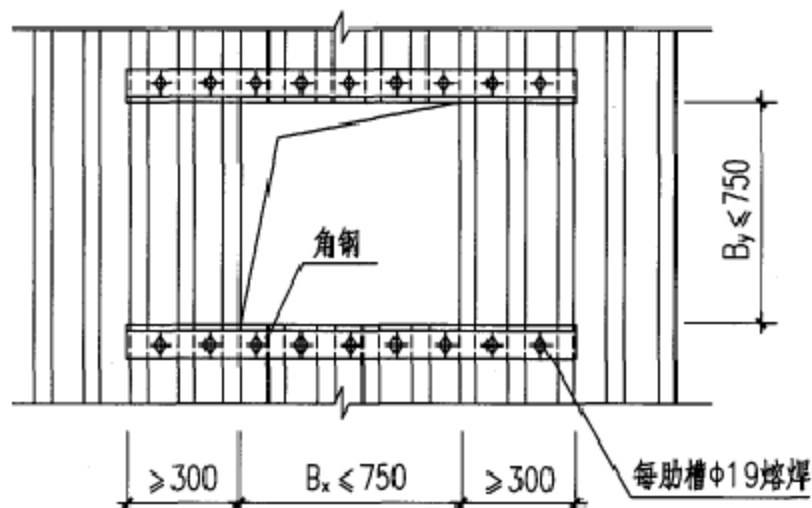
组合楼板开孔 \leq 750 时的加强措施(1)
