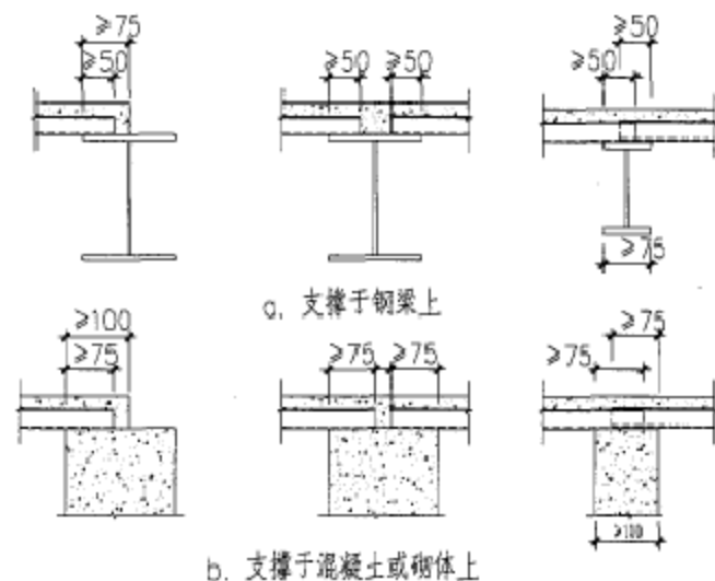
图 6.5-2 组合楼板的支承长度要求
