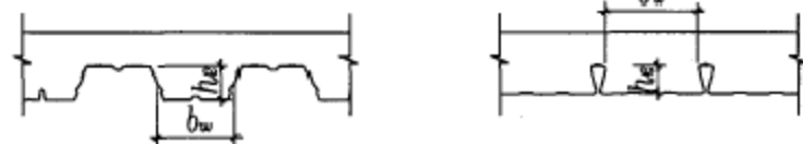
压型钢板组合板剖面
