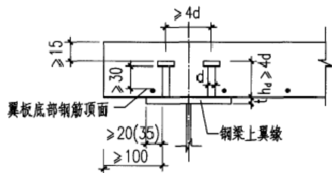
a. 组合梁翼板为现浇混凝土平板
