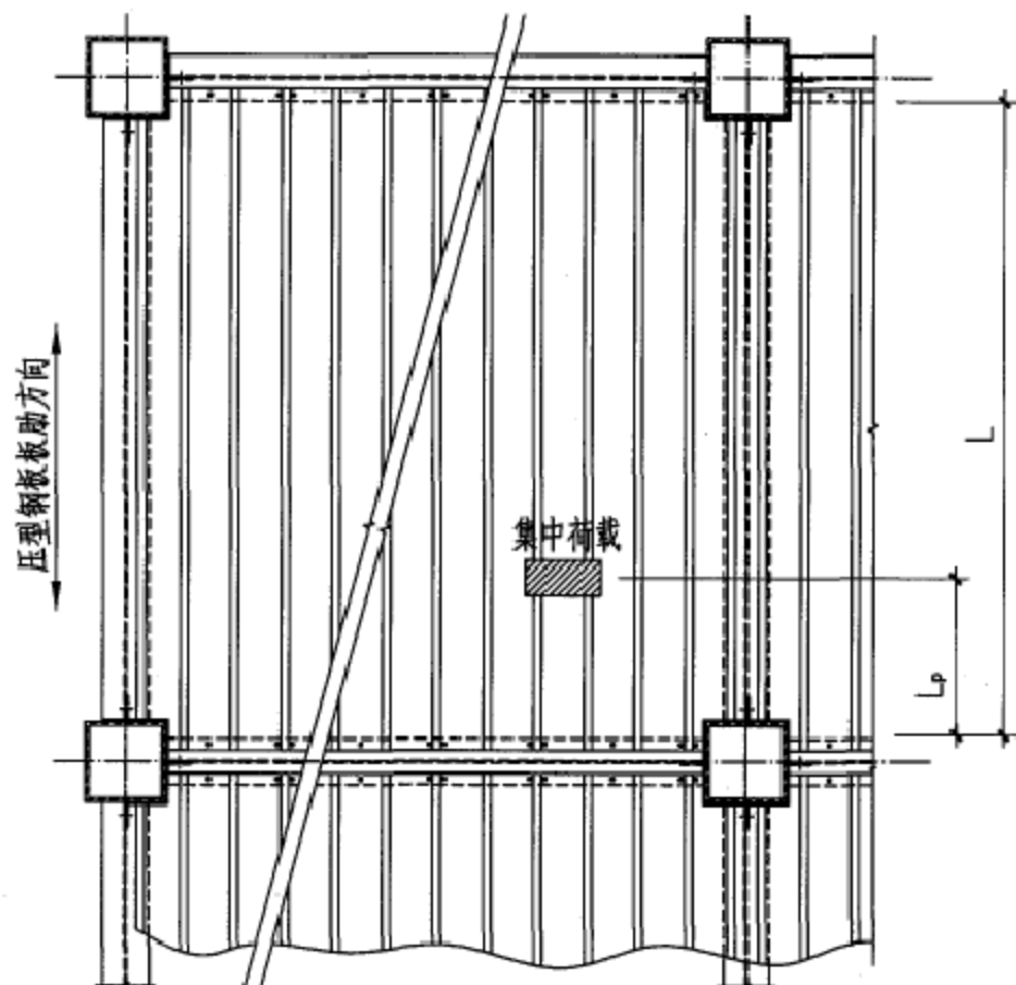
压型钢板铺板平面示意图
