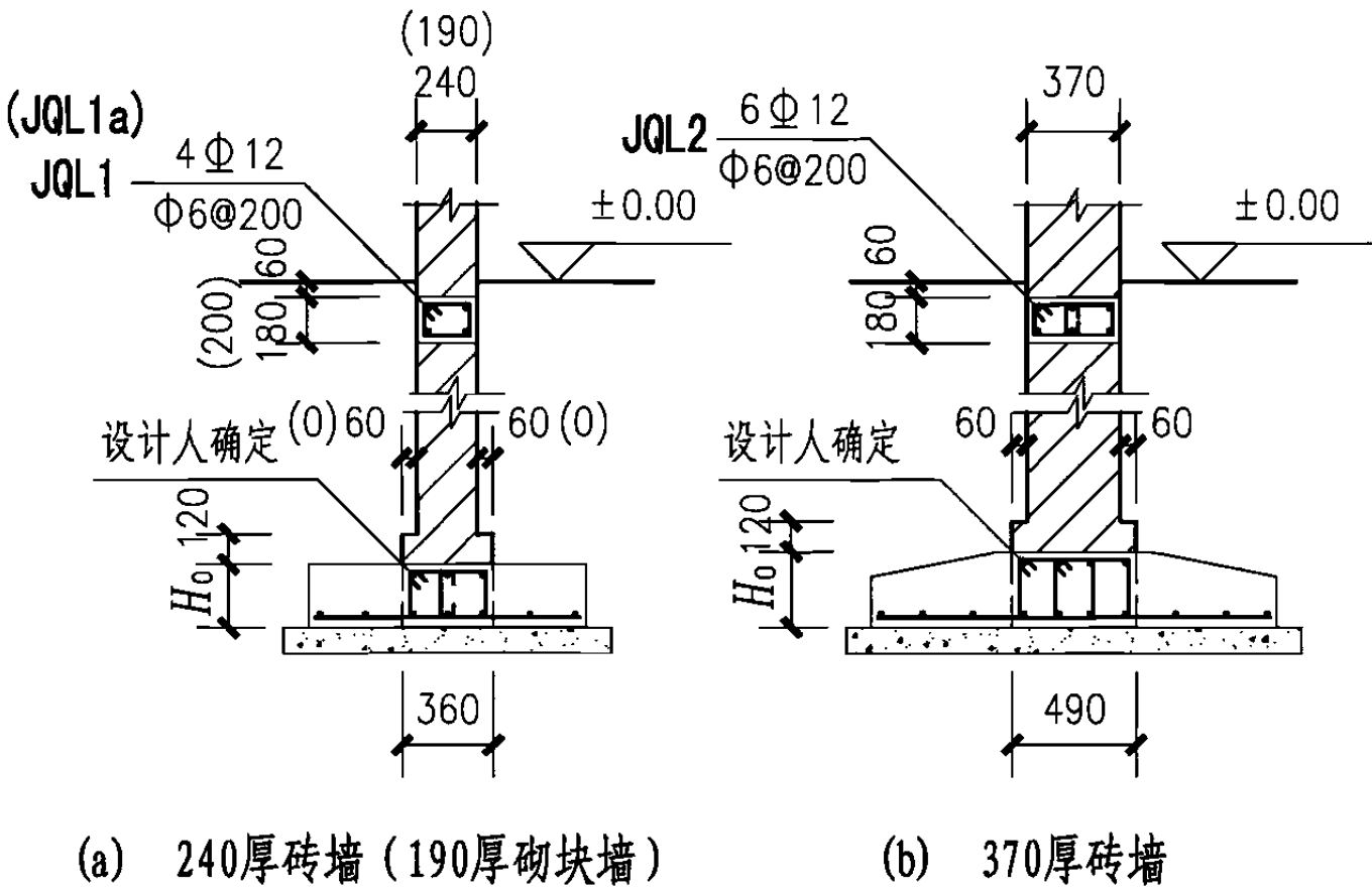
图9.2-2 基础圈梁、暗梁
