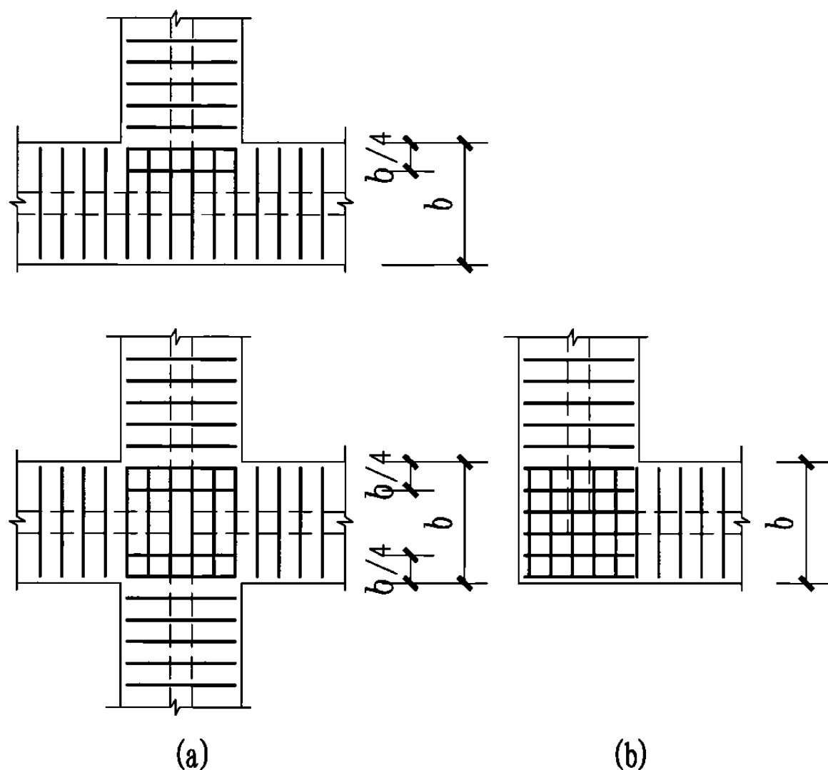
图9.14 钢筋混凝土条形基础底板受力钢筋布置示意
