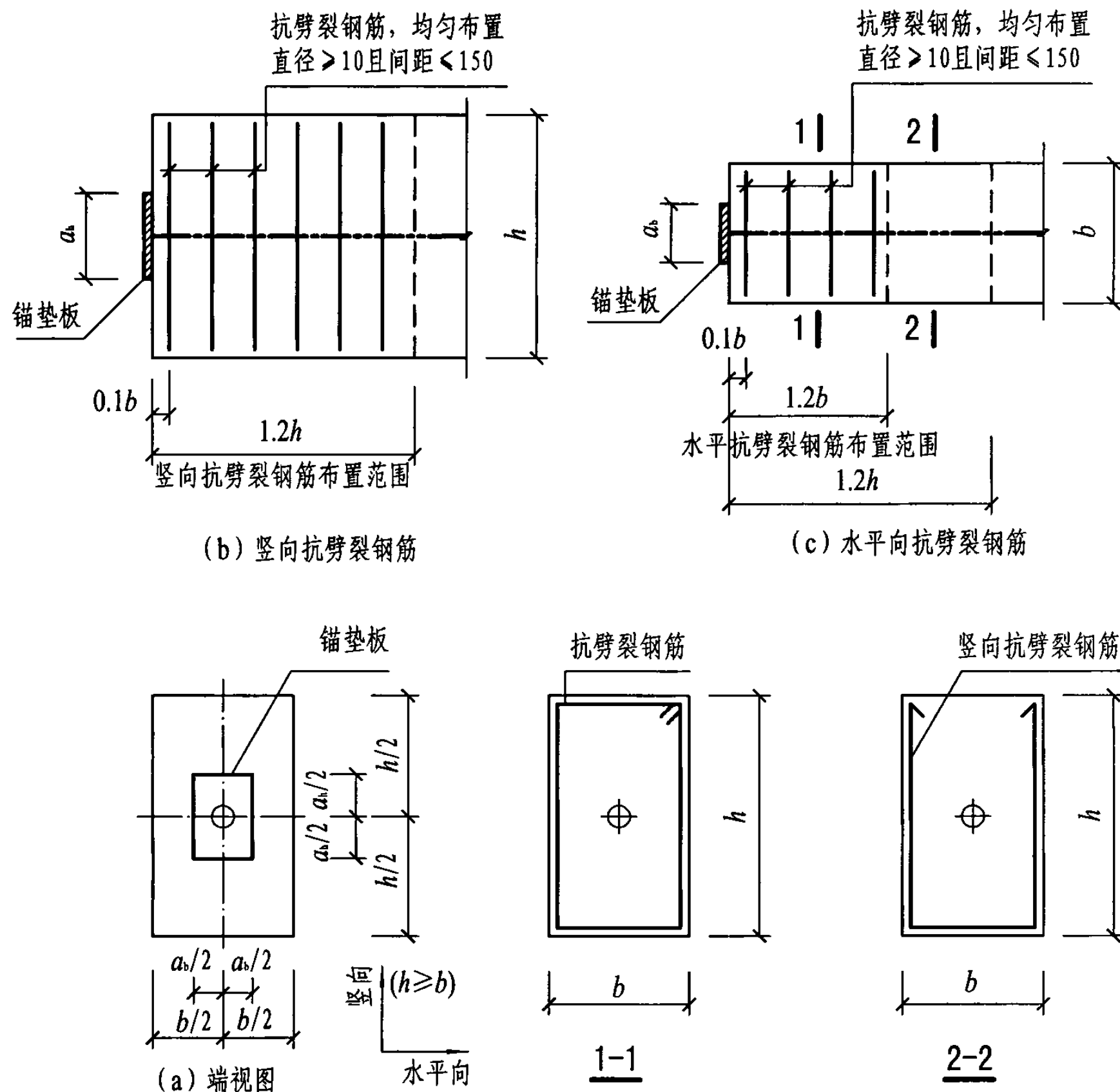
图2.4-3 中置锚具锚固区抗劈裂钢筋构造
