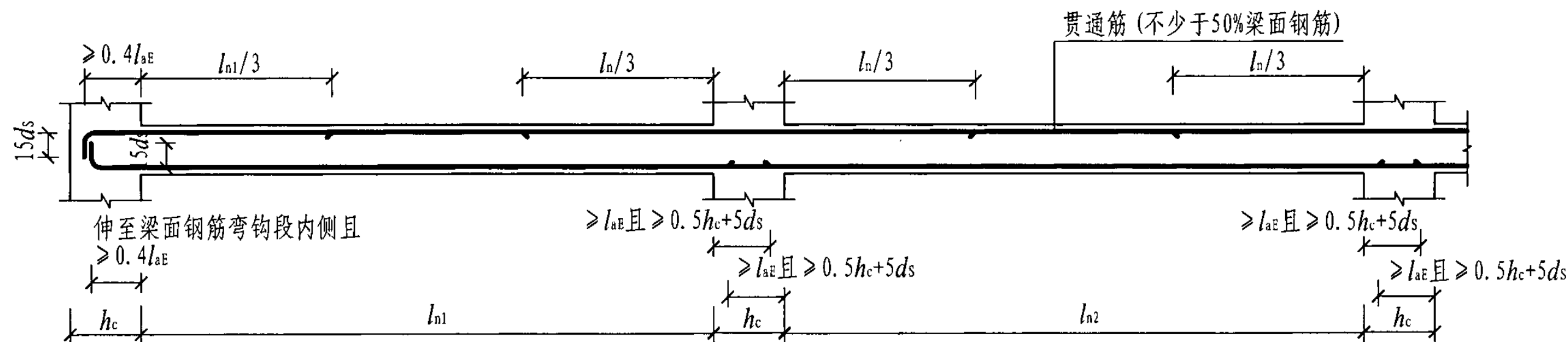
图2.3-9 抗震板柱结构楼层框架暗梁纵向钢筋构造（端支座弯锚）
