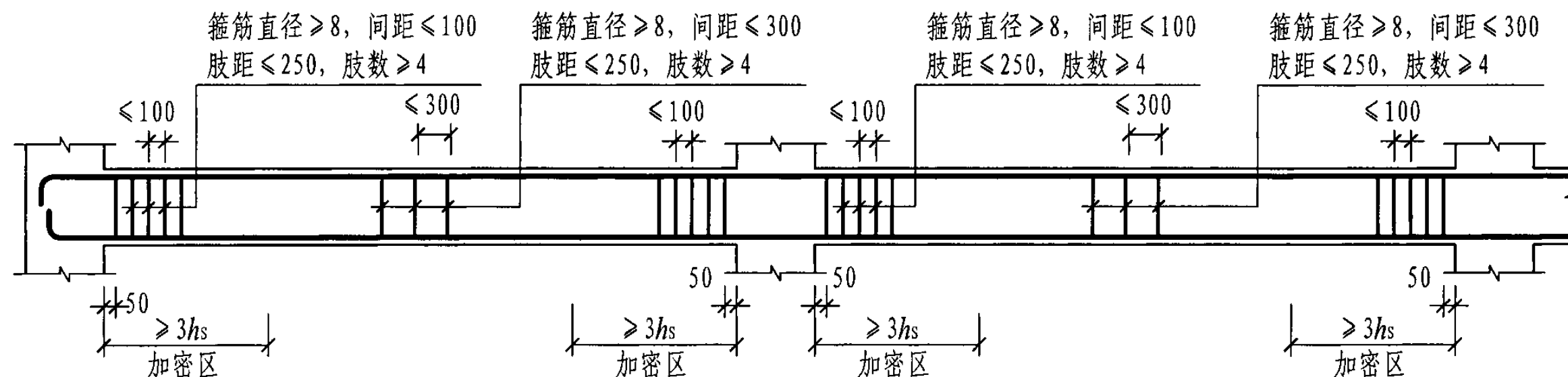
图2.3-8 抗震板柱结构框架暗梁箍筋构造
