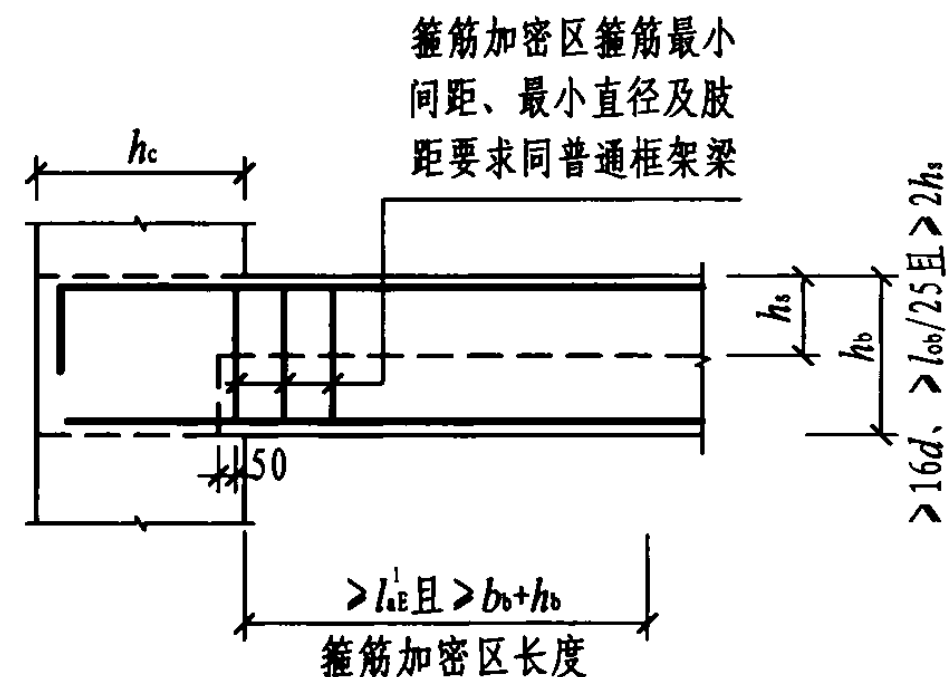
1-1 箍筋加密区
