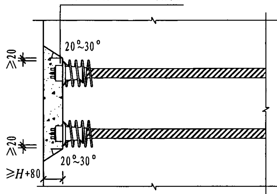
图2.4-23 有粘结预应力筋内凹式封锚构造
