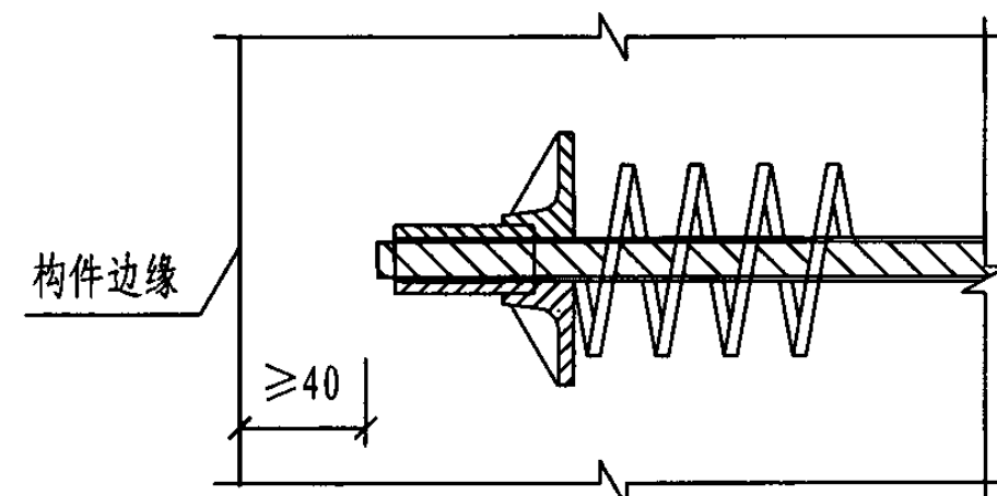
(c) 挤压锚具固定端保护措施
