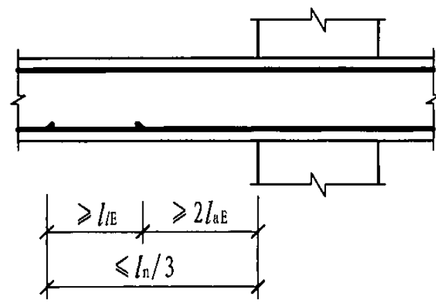
(b) 暗梁支座范围外的下部纵筋搭接
