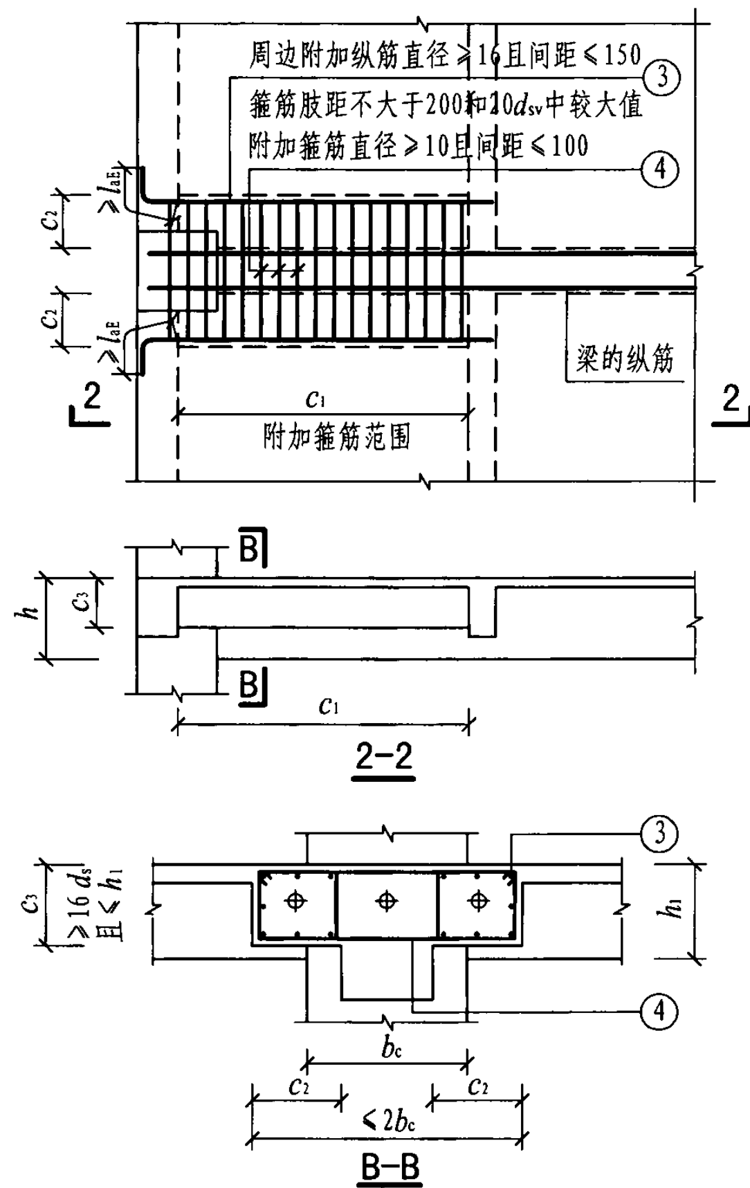
图2.2-5 梁端宽加腋YBb
