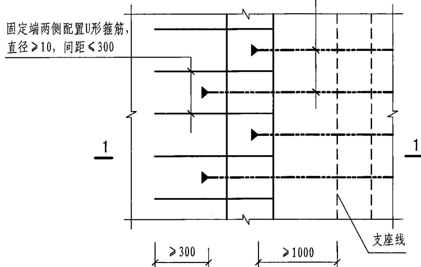
图2.4-20 板中固定端构造配筋
