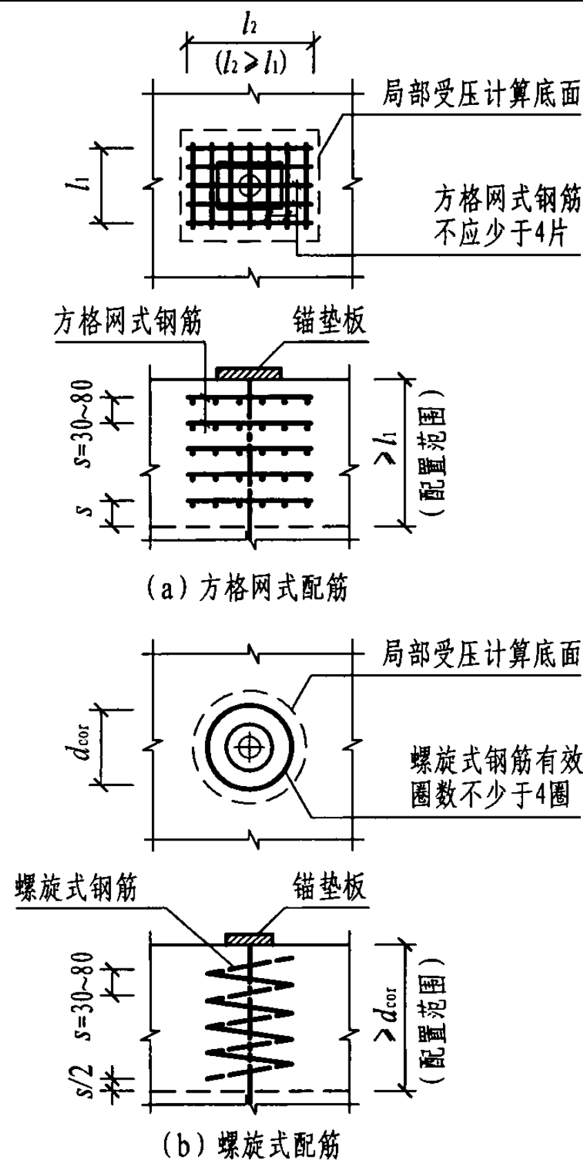
图2.4-2 局部受压区的间接钢筋构造
