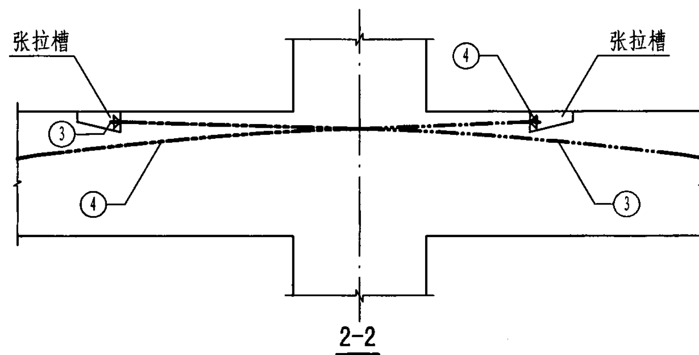
图2.2-12 梁面留槽张拉搭接(二)
