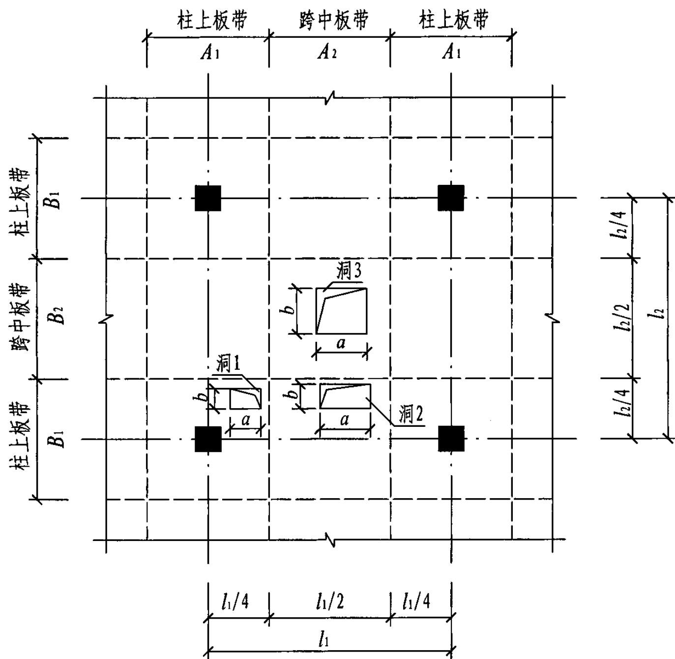
(a) 板柱结构楼板开洞要求
