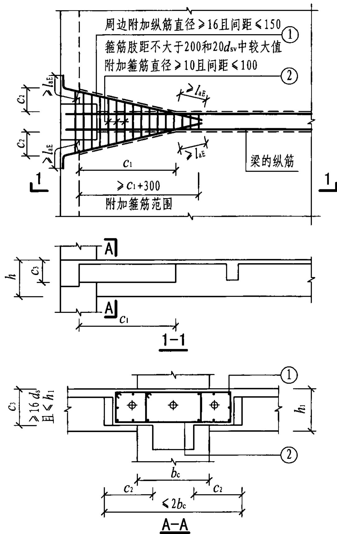
图2.2-4 梁端宽加腋YBa
