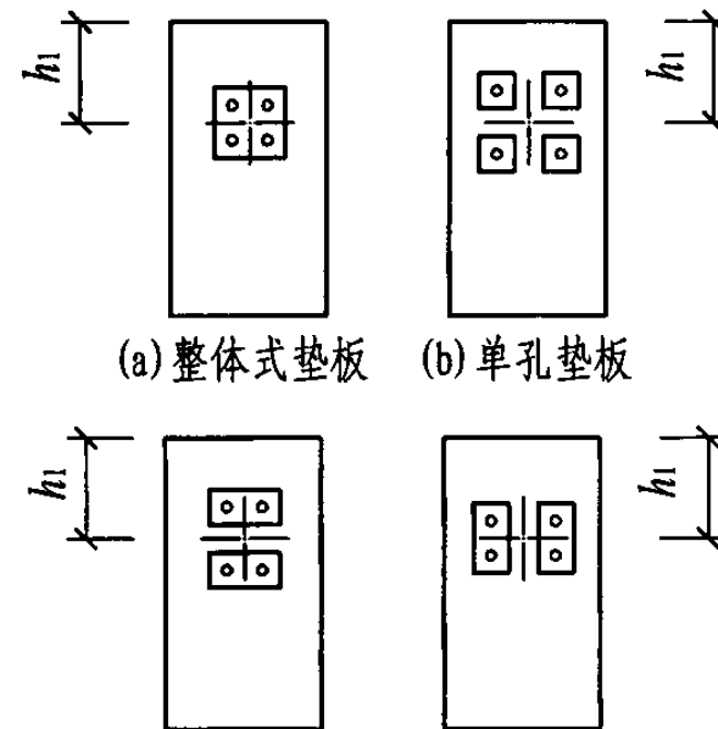
图2.4-17 垫板布置示例 (4孔)
