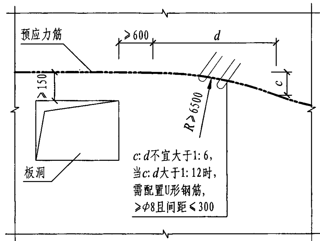
(b) 板洞口预应力筋布置要求
