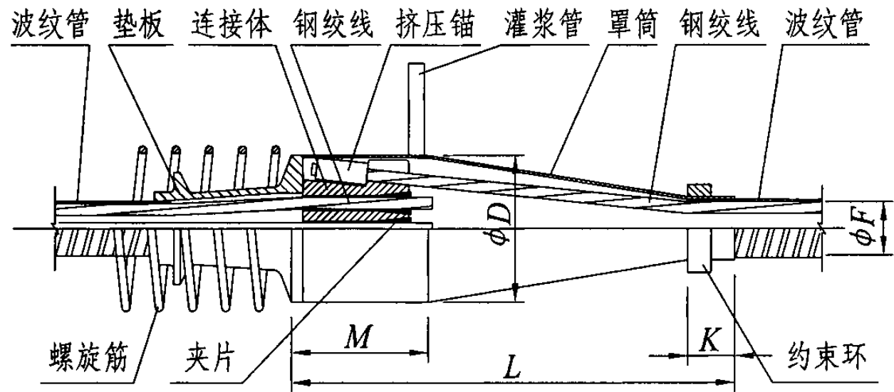
图3.5.1 周边悬挂挤压式连接器构造
