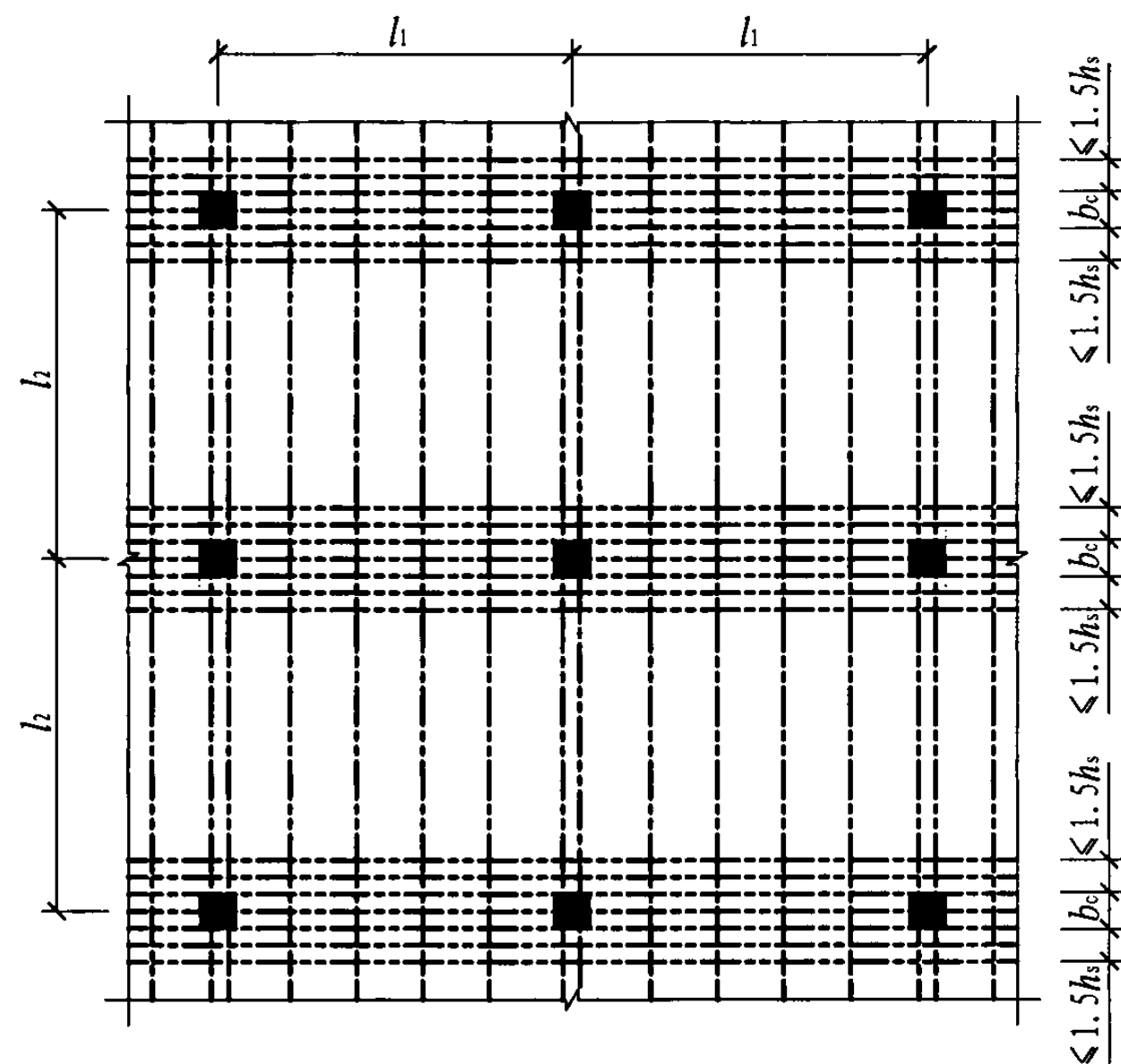
(b) 一向集中, 另一向均匀布置
