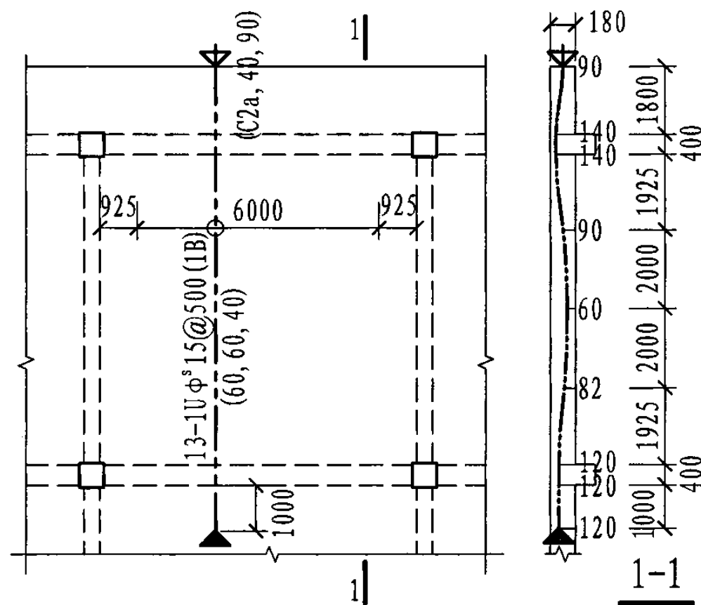
图1.5.5 板内预应力筋线形平面标注示例
