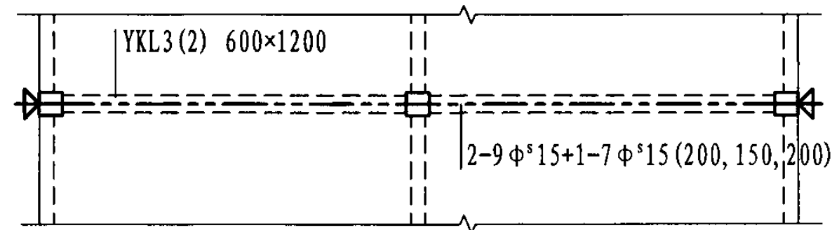
图1.4.5-3 梁内预应力筋平面注写示例(三)
