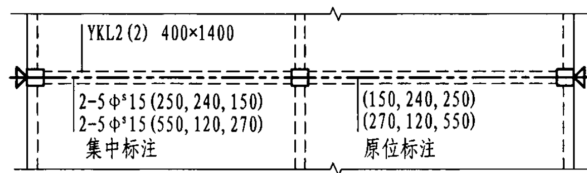
图1.4.5-2 梁内预应力筋平面注写示例(二)
