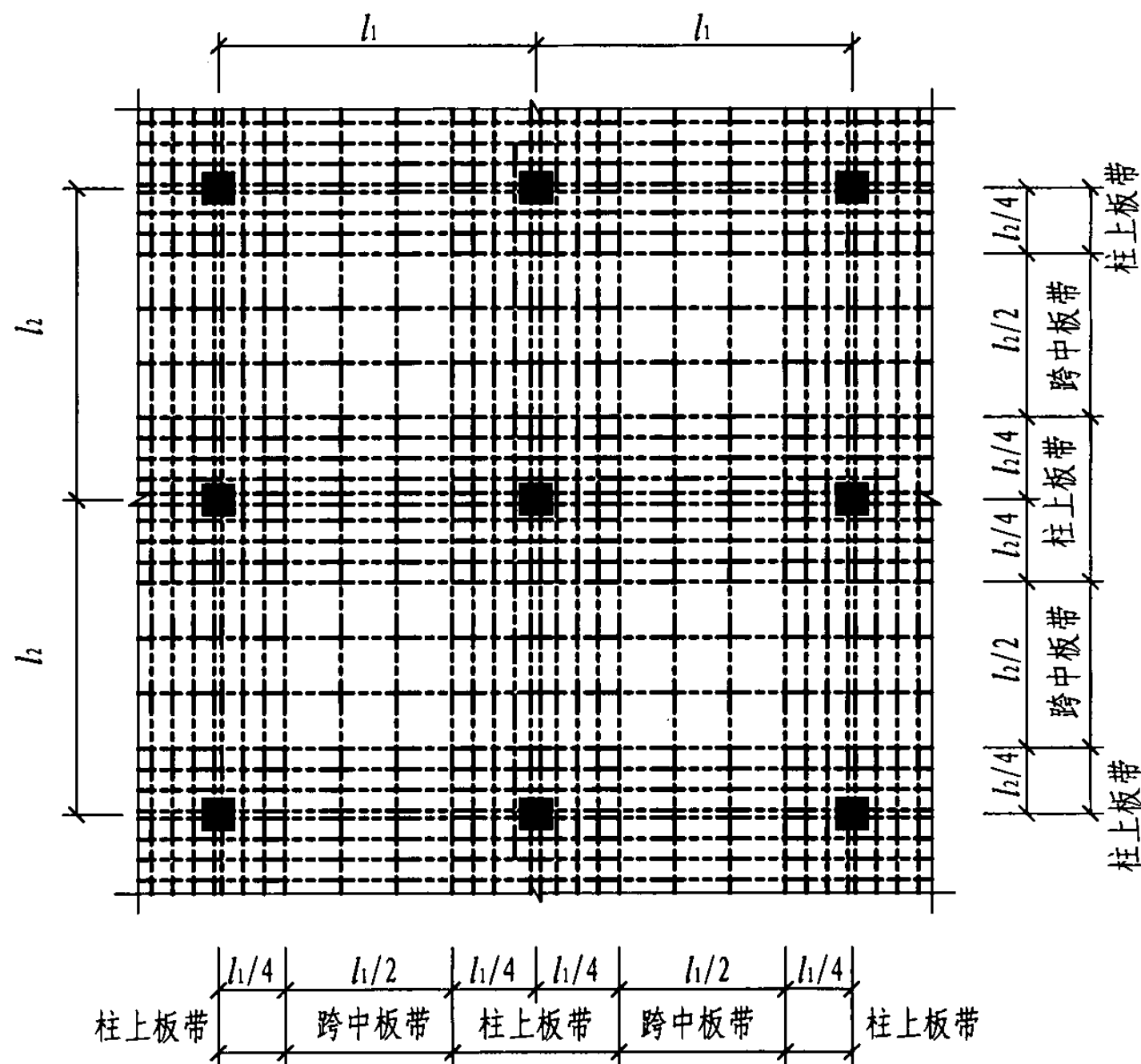
(a) 按柱上板带和跨中板带布置
