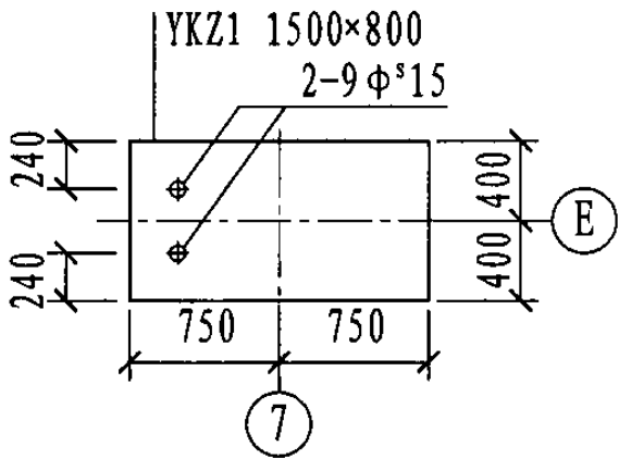
(b) 截面注写表达
