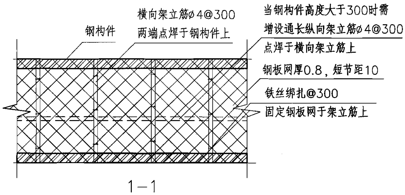
槽形钢柱空心包裹法
