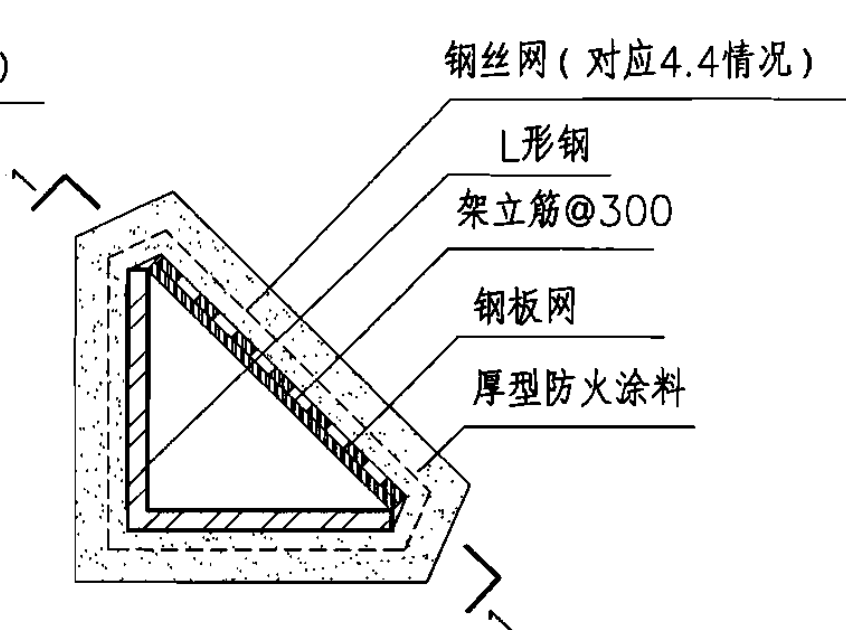
L形钢柱空心包裹法
